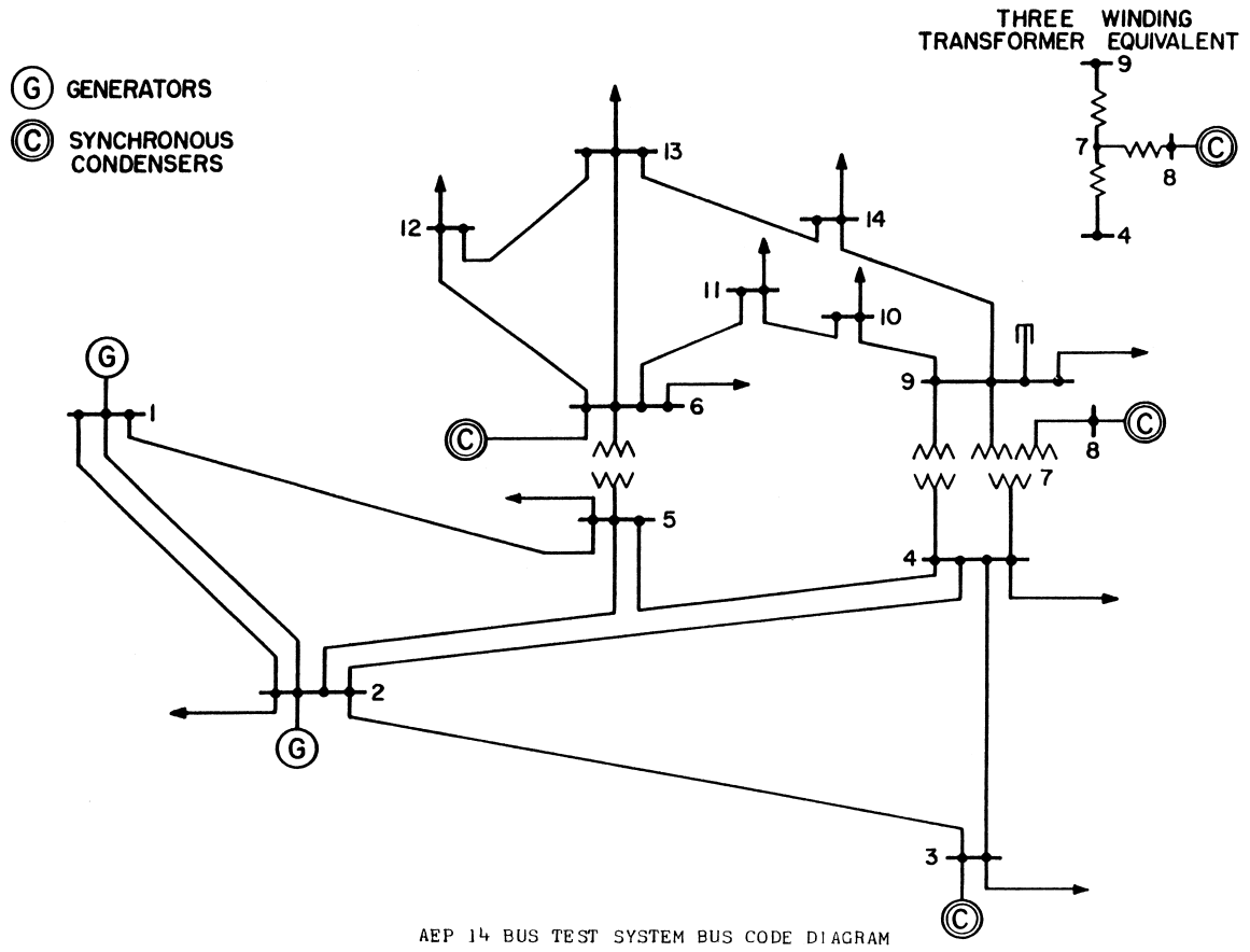
Figura 2.10– Sistema IEEE com 14 barras (UNIVERSIDADE DE WASHINGTON, 2007).
