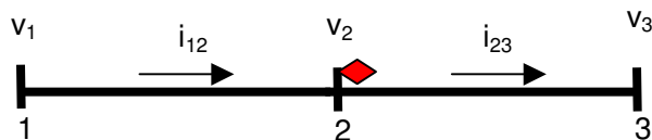
Figura 4.1 – Rede de 3 barras com monitor de QEE instalado na barra 2 considerando custos de instalação iguais em cada barra.
