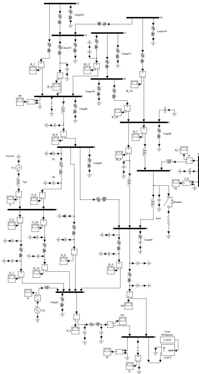
Figura 5.2 – Rede IEEE 14 barras.
