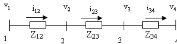
Figura 2.5 – Rede esquemática.
