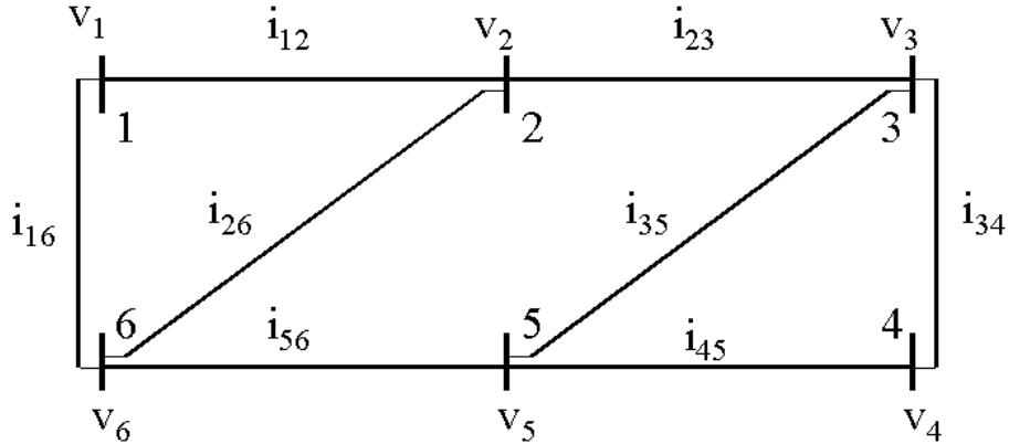
Figura 2.8 – Sistema com 6 barras desconhecidas (ELDERY ET AL. , 2004, 2006).
