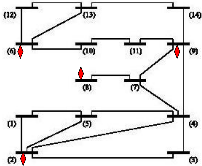
Figura 4.2 – Rede IEEE 14 barras com monitores de QEE instalados nas barras 2, 6, 8 e 9 considerando custos de instalação iguais em cada barra.
