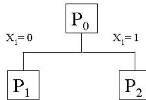
Fig. 3.5 - Árvore branch and bound com os nós correspondentes a P_0 , P_1 e P_2 .
