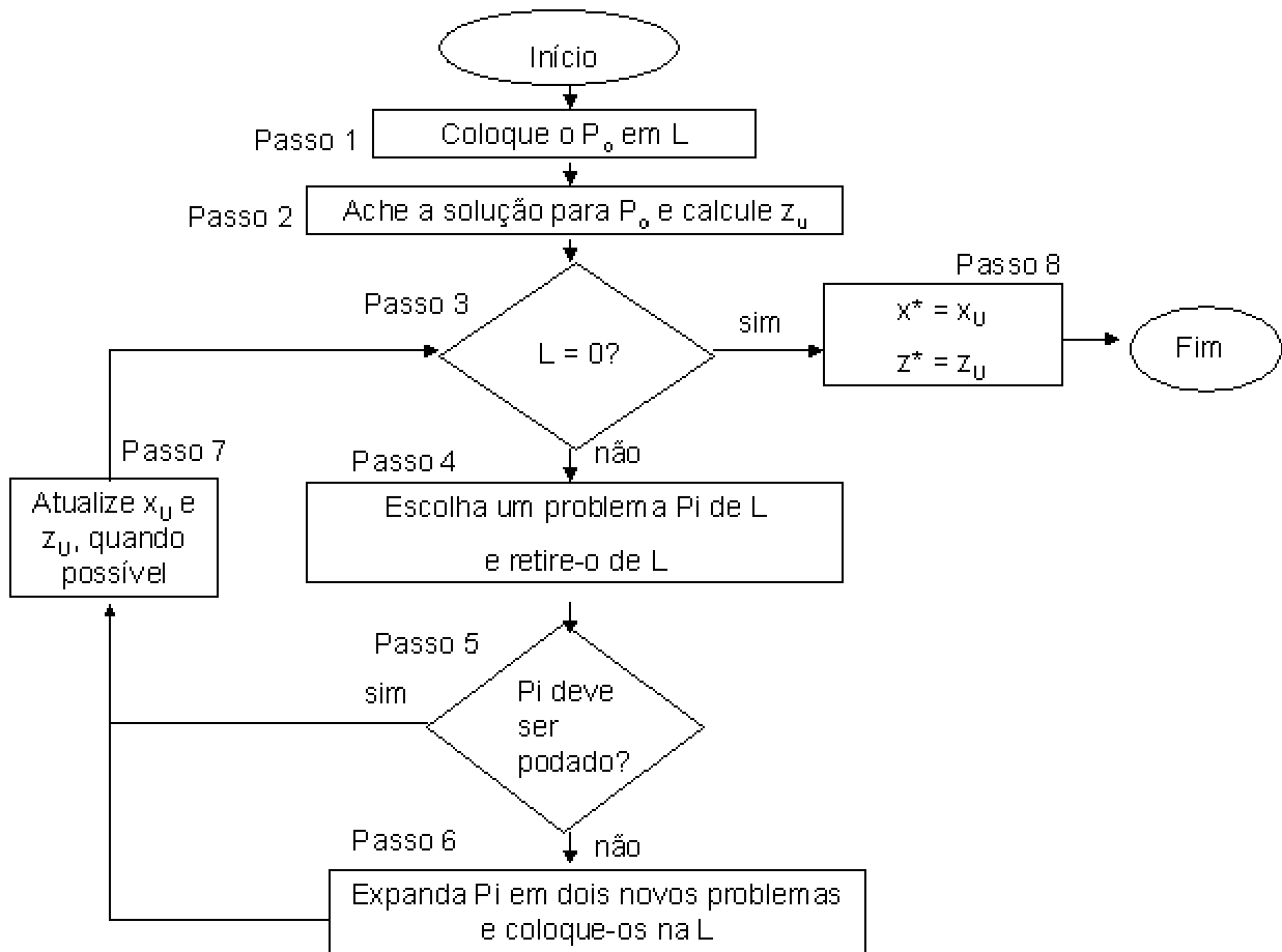
Fig. 3.3 – Fluxograma geral para resolver um PR
