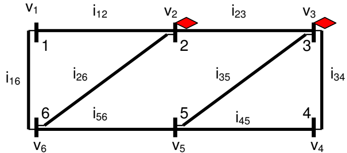
Figura 4.3 - Rede de 6 barras com monitores de QEE instalados na barra 2 e 3 considerando custos de instalação iguais em cada barra.
