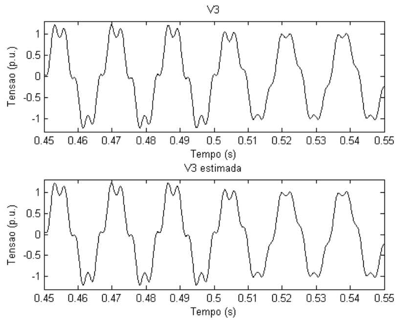
Figura 5.4 – Tensões: real e estimada na barra 3 com carga não-linear nas barras 3 e 7.
