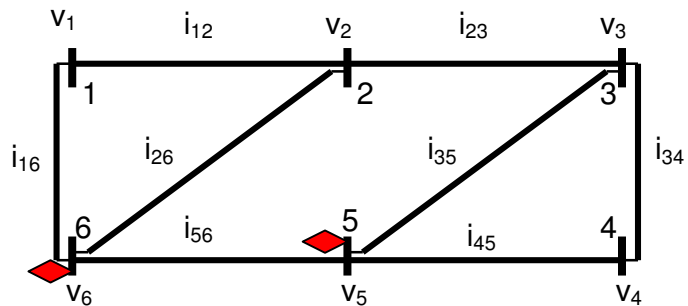
Figura 4.4 - Rede de 6 barras com monitores de QEE instalados na barra 5 e 6 considerando custos de instalação iguais em cada barra.
