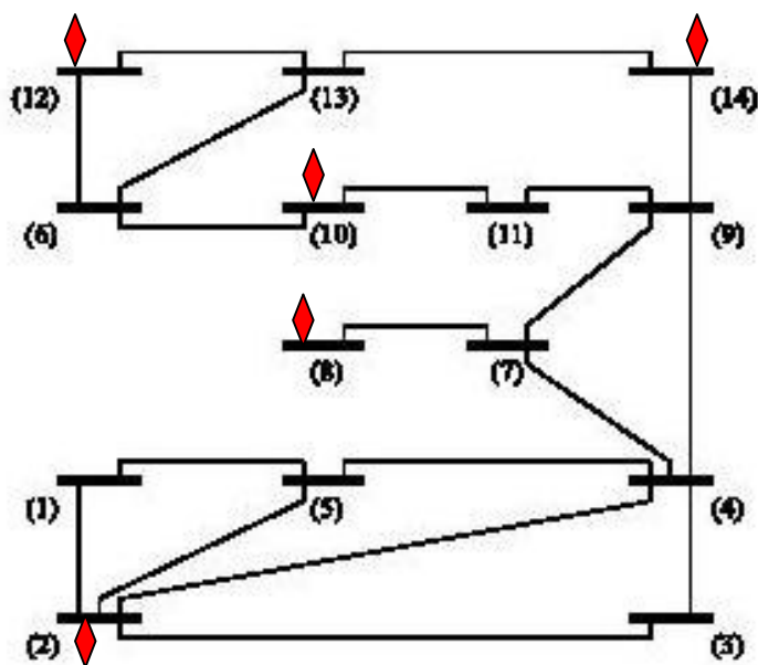
Figura 4.6 – Rede IEEE 14 barras com monitores de QEE instalados considerando custos de instalação diferentes em cada barra.
