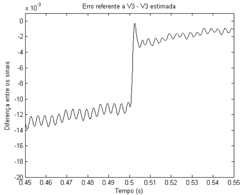
Figura 5.5 – Erro absoluto obtido para a tensão na barra 3 com afundamento de tensão provocado por carga na barra 7 e carga harmônica na barra 3.
