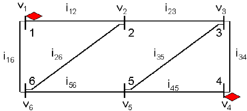
Figura 5.1 - Rede de 6 barras com monitores de QEE instalados na barra 1 e 4.
