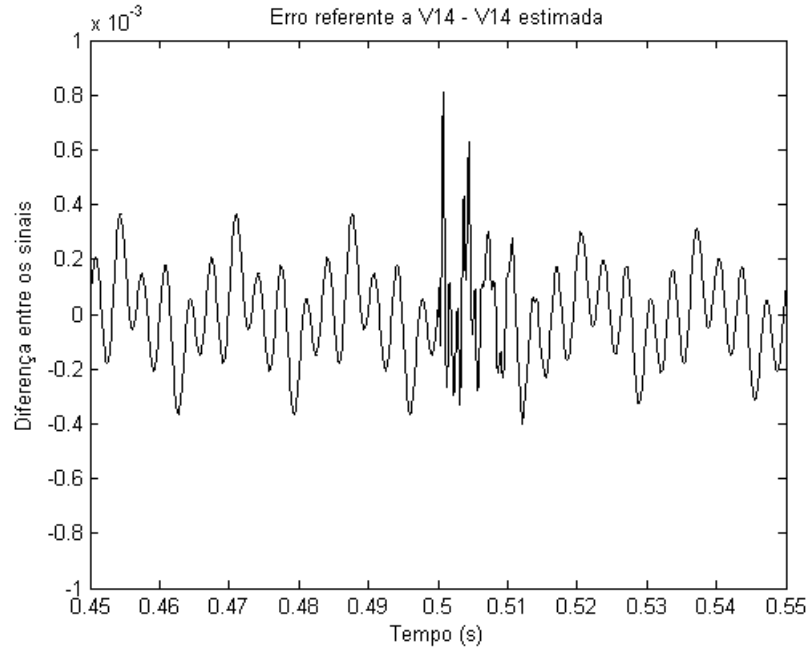
Figura 5.7 – Erro absoluto obtido para a tensão na barra 14 com afundamento de tensão provocado por carga na barra 7 e carga harmônica na barra 3.
