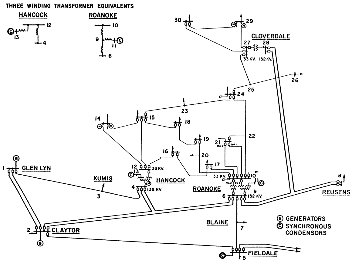
Figura 2.11– Sistema IEEE com 30 barras (UNIVERSIDADE DE WASHINGTON, 2007).
