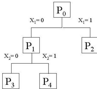
Figura 3.6 – Árvore B & B com os nós correspondentes a P_0 , P_1 e P_2 ; P_3 ; e P_4 .
