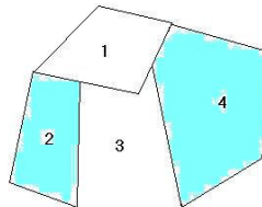
Figura 2.4 - Solução 3: Instalação nas regiões 2 e 4, atendendo às regiões 1 e 3.
