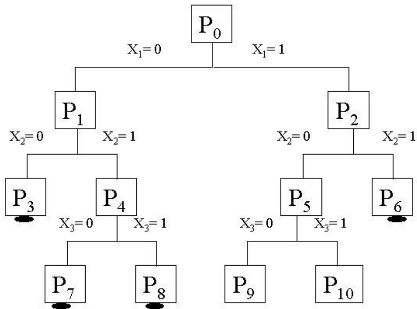
Figura 3.9 – Árvore B & B com os nós correspondentes a P_0 , P_1 e P_2 ; P_3 ; e P_4 ; P_5 e P_6 ; P_7 e P_8 e P_9 e P_{10} .
