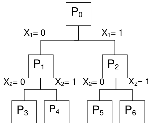
Fig. 3.2 - Árvore de particionamento com os nós correspondentes a P_0 , P_1 e P_2 ; P_3 e P_4 ; e P_5 e P_6 .
