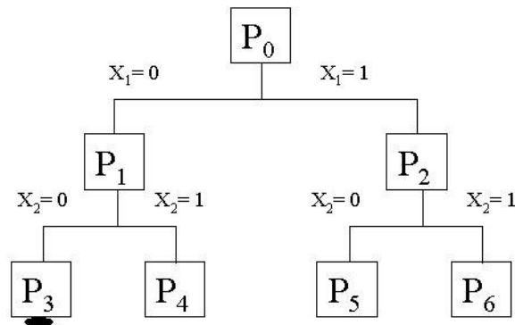
Figura 3.7 – Árvore B & B com os nós correspondentes a P_0 , P_1 e P_2 ; P_3 ; e P_4 ; e P_5 e P_6 .
