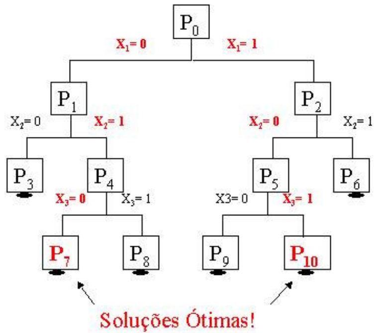
Figura 3.10– Árvore final para o problema.
