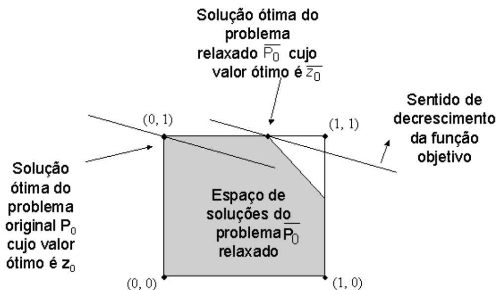
Fig. 3.1. - Espaço de soluções do problema P_0 .
