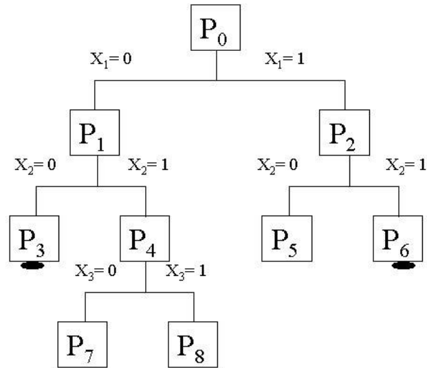
Figura 3.8 – Árvore B & B com os nós correspondentes a P_0 , P_1 e P_2 ; P_3 ; e P_4 ; P_5 e P_6 e P_7 e P_8 .
