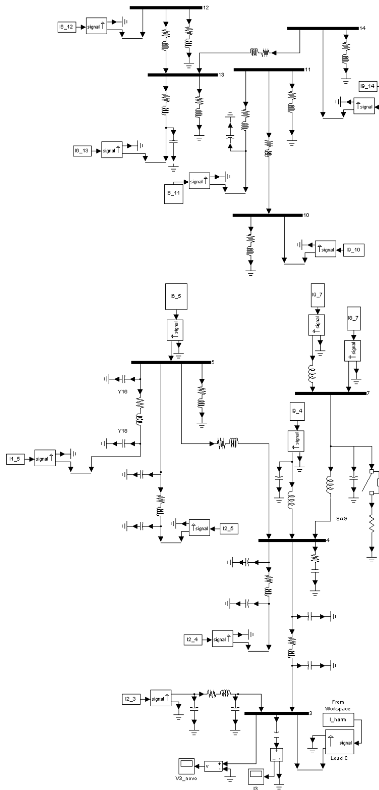
Figura 5.3 – Rede IEEE 14 barras reconstruída.
