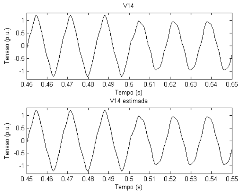
Figura 5.6 – Tensões: real e estimada na barra 14 com carga não-linear nas barras 3 e 7.
