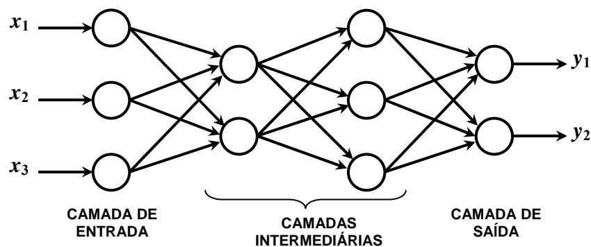
Figura 7 – Rede neural do tipo feedforward
