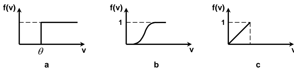
Figura 6 – Funções de ativação: (a) threshold ; (b) sigmoial; (c) linear.
