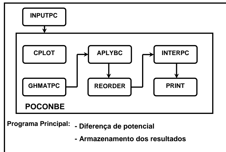
Figura 10 – Fluxograma do BEM para o potencial
