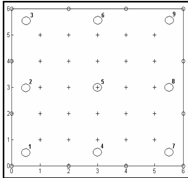
Figura 14 – Possíveis localizações dos furos na placa com 25 sensores
