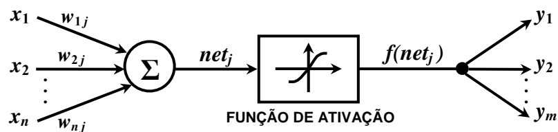
Figura 4 – Estrutura de um neurônio artificial (adaptado de Chong & Zak, 2001)
