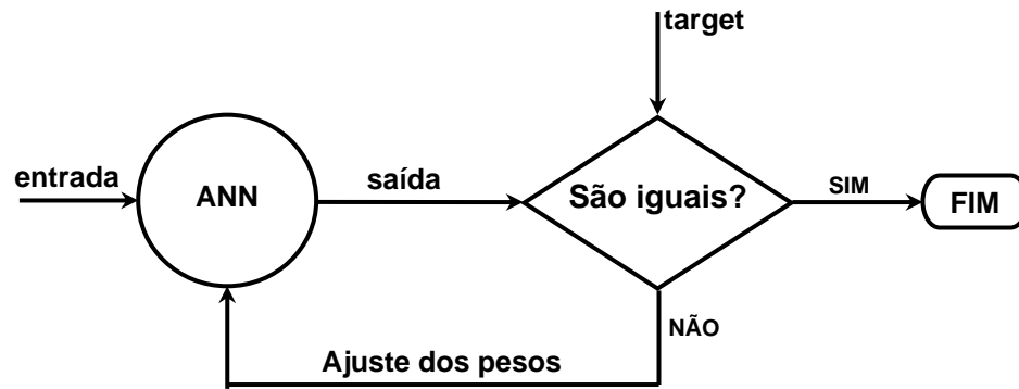
Figura 8 – Processo de treinamento de uma ANN (adaptado da Neural Network Toolbox do Matlab ® )
