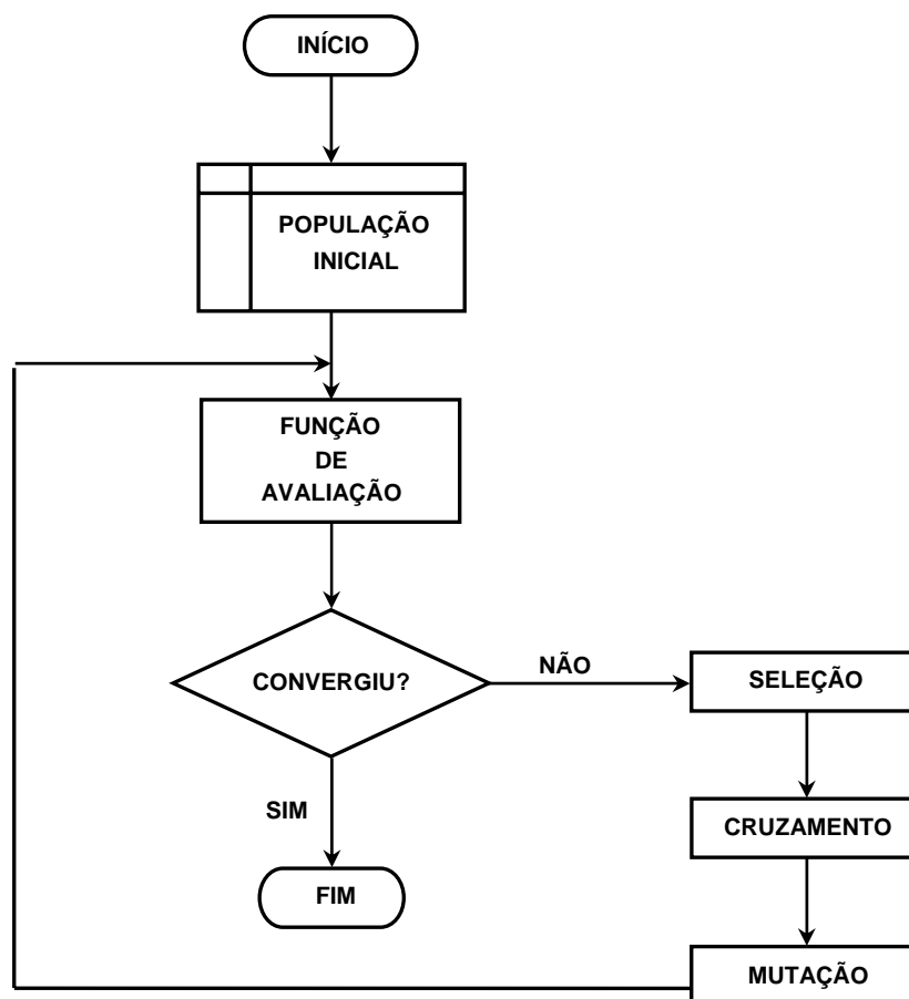
Figura 2 – Fluxograma do GA.
