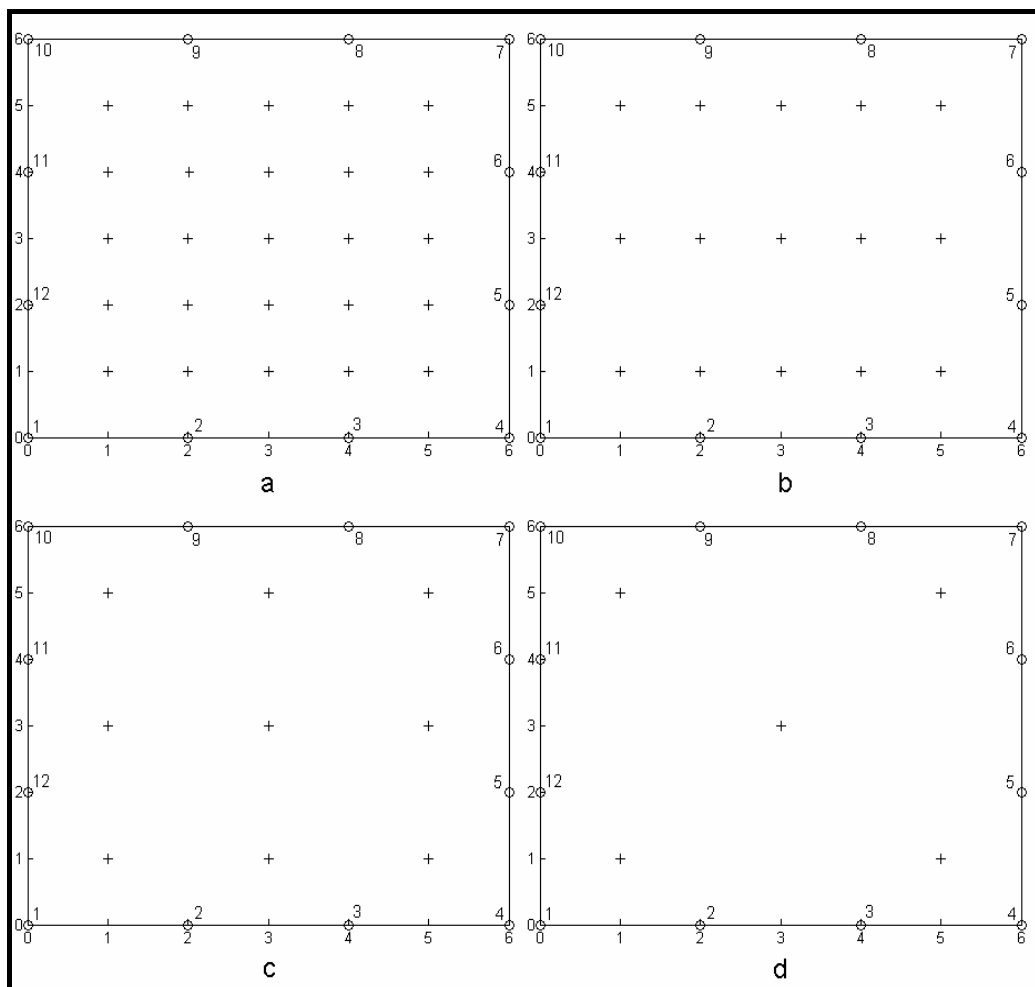
Figura 13 – Distribuição dos sensores para a ANN: (a) 25, (b) 15, (c) 9, (d) 5
