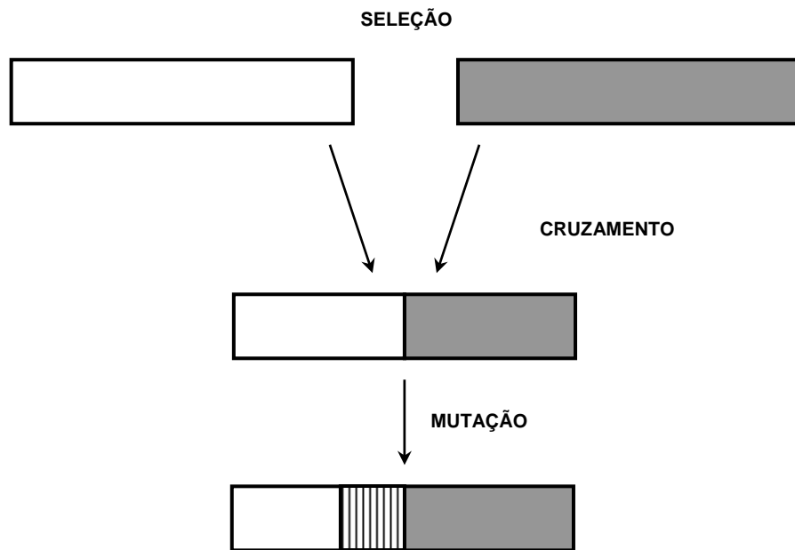
Figura 1 – Operadores genéticos.
