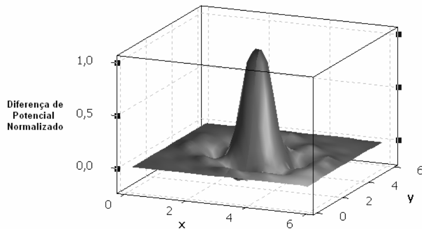
Figura 16 – Diferença de potencial normalizado para uma placa com furo central
