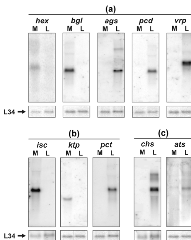
Figura 13. Análise por northern blot de genes super expressos em micélio e levedura de P. brasiliensis . RNA total de micélio (M) e levedura (L) foram analisados em gel desnaturante e transferidos para membranas de nylon, as quais foram hibridadas com sondas marcadas radioativamente dos seguintes genes específicos: a) Organização celular: hex -proteína peroxissomal hexagonal, bgl - 1,3 \beta -glucosidase, ags - \alpha -1,3-glucana sintase, cda - quitina deacetilase e vrp - verprolin. b) Transporte de íons: isc - iron-sulfur cluster, ktp - cation transporter de cation, pct - provável P-type cation. c) Metabolismo de enxofre: chs - coline sulfatase e ats - ATP sulfurilase. A proteína 60S ribossomal L34 constitutiva foi usada como controle de quantidade de RNA total aplicado em cada amostra.
