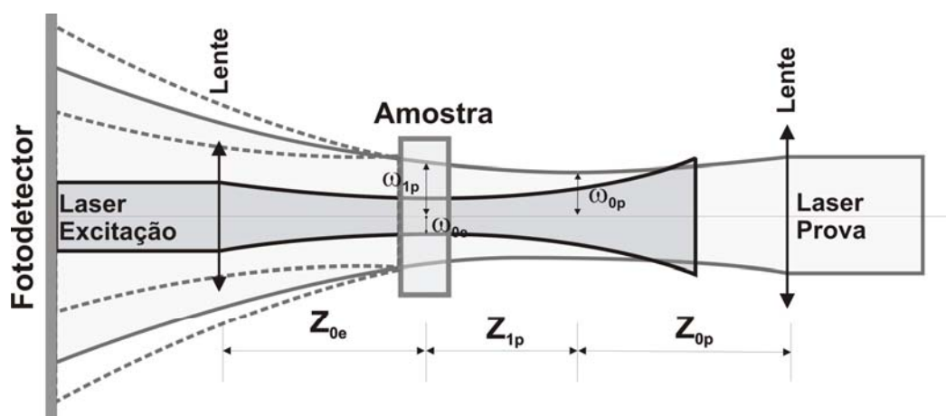
Figura B.1 – Esquema da configuração descasada para a lente térmica.
