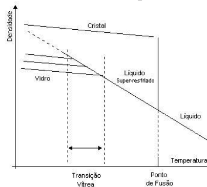
Figura 2.4 – Diagrama de fase, mostrando a variação da densidade com a temperatura.
