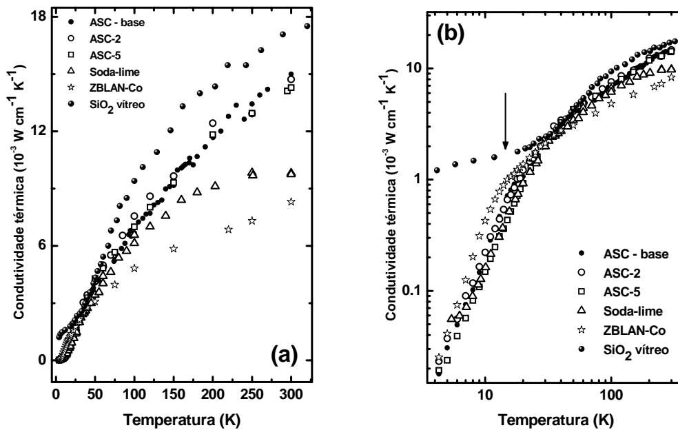
Figura 5.6 – (a) Condutividade térmica \kappa(T) como função da temperatura para os vidros ASC, soda-lime e ZBLAN e (b) \kappa(T) em função da temperatura, na escala logarítmica*. Os dados do vidro \text{SiO}_2 são mostrados apenas para comparação [6].
