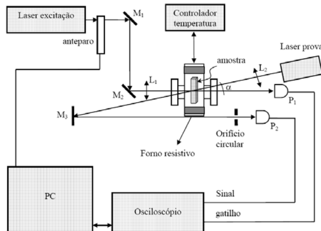
Figura 6.1 – Arranjo experimental da lente térmica. Os feixes de excitação e prova são gerados por um laser de Ar + (λ = 514 nm) e um laser de He-Ne (λ = 632,8 nm) respectivamente. M i , L i e P i são espelhos, lentes e fotodiodos, respectivamente. O aquecimento da amostra é feito por um forno resistivo e controlado por um controlador Lake-Shore 340.
