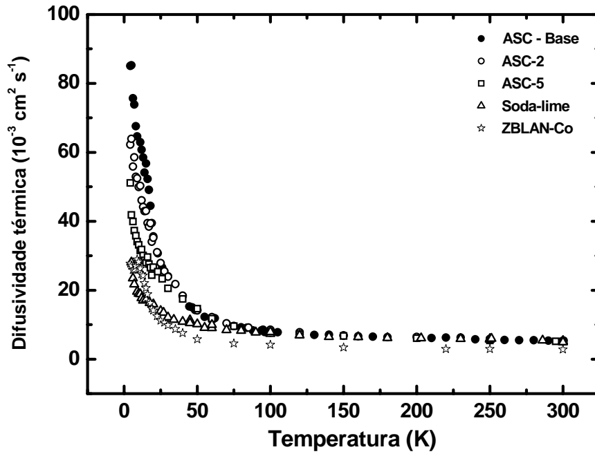
Figura 5.3 – Difusividade térmica ( D ) em função da temperatura para os vidros ASC, soda-lime e ZBLAN.
