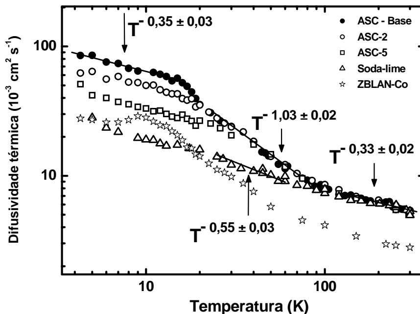
Figura 5.4 – Difusividade térmica ( D ) em função da temperatura para os vidros ASC, soda-lime e ZBLAN, na escala logarítmica.
