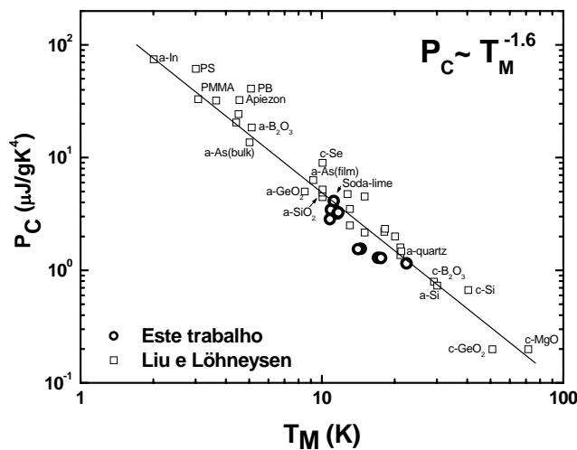
Figura 4.5 – Correlação entre o máximo na curva c_p/T^3 ( P_C ) e a temperatura em que o máximo ocorre ( T_M ) para os vidros analisados neste trabalho e os analisados em Ref. [36].
