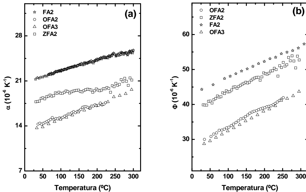
Figura 6.10 – Dependência com a temperatura do coeficiente de expansão térmica linear (a) e do coeficiente térmico da polarizabilidade eletrônica (b).
