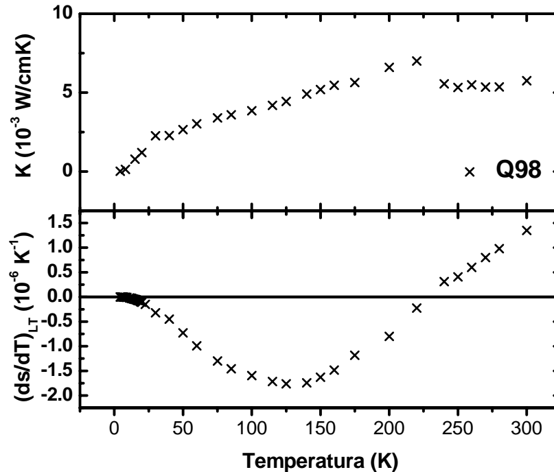
Figura 5.12 – Condutividade térmica (a) e (ds/dT)_{LT} (b) como função da temperatura para o vidro fosfato Q98 dopado com 2% em peso de Nd_2O_3 .
