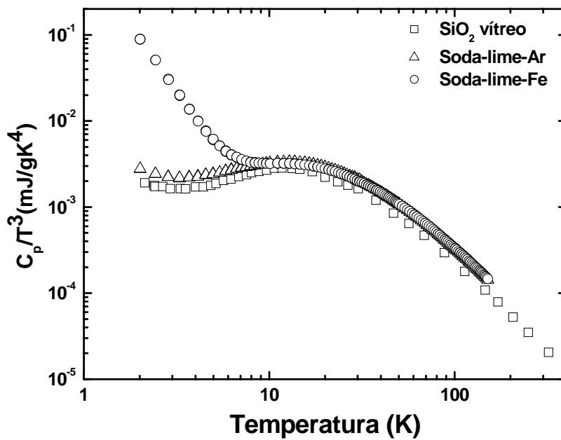
Figura 4.2 – Calor específico dos vidros soda-lime e \text{SiO}_2 [6] na representação c_p/T^3 , na escala logarítmica, em função da temperatura.
