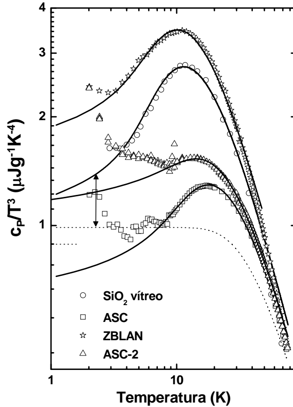
Figura 4.7 – Calor específico dos vidros ASC (dopados e não dopados), ZBLAN e \text{SiO}_2 [6] em função da temperatura, na representação c_p/T^3 , na escala logarítmica. A linha contínua representa a predição teórica para o calor específico. A linha pontilhada representa o calor específico calculado fazendo b = 0 . O pontilhado curto indica o calor específico calculado a partir dos dados das medidas elásticas [126].
