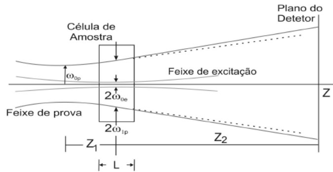
Figura 2.7 – Esquema da posição geométrica dos feixes em um experimento de LT em modo descasado.
