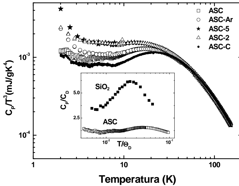
Figura 4.1 – Calor específico dos vidros aluminosilicato de cálcio (ASC) e do ASC cristalino na representação c_p/T^3 , na escala logarítmica, em função da temperatura. O detalhe na figura mostra o c_p dos vidros ASC e \text{SiO}_2 escalados pelos parâmetros de Debye de [6], para o \text{SiO}_2 , e da amostra de ASC cristalino para o ASC vítreo.
