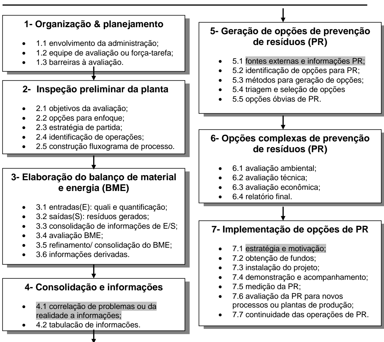
Figura 4.6 Metodologia para implementação de programa de prevenção de resíduos na fonte e economia de água e energia: Fundação Vanzolini, USP
