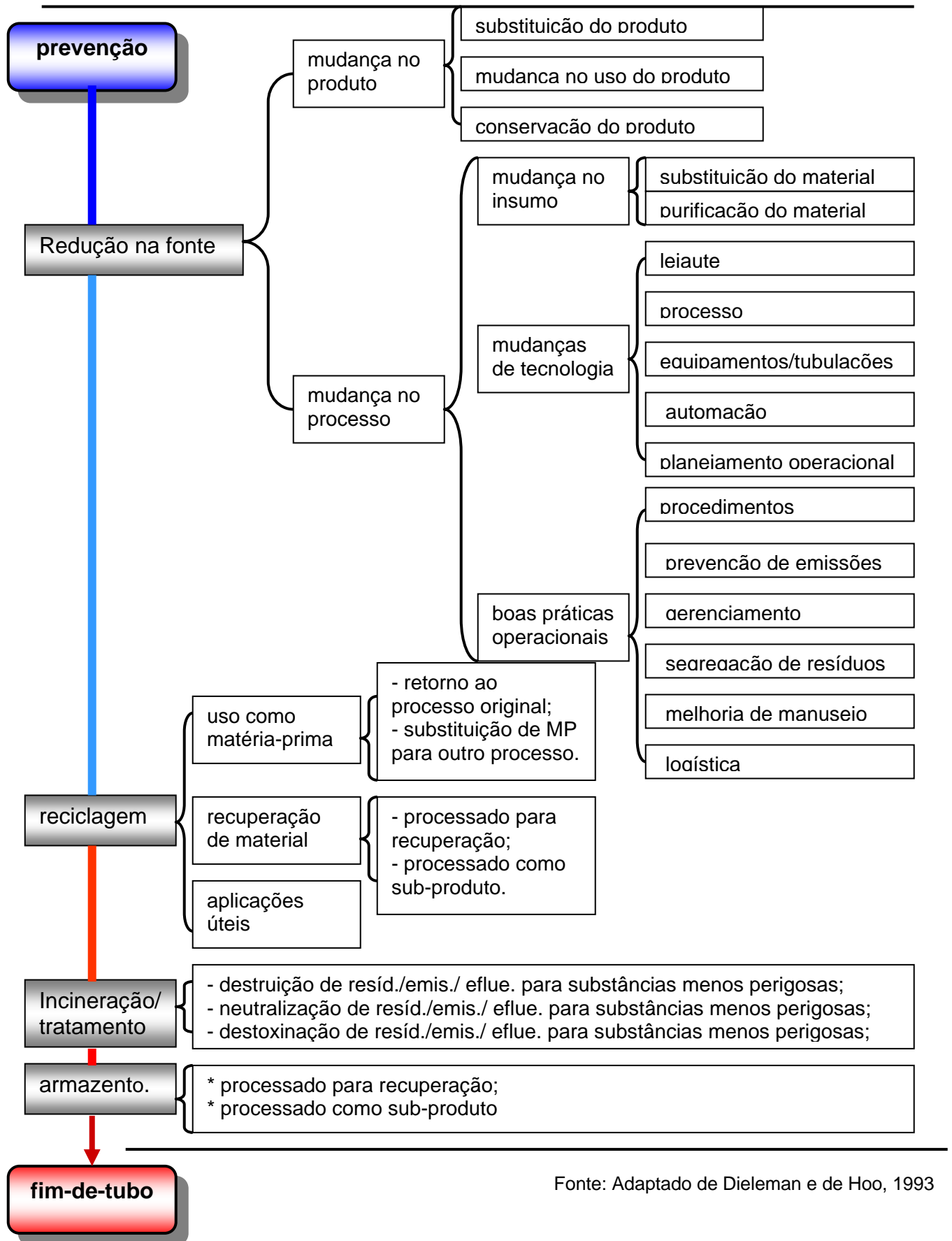
Figura 4.16 Da prevenção ao fim-de-tubo: identificando operações
