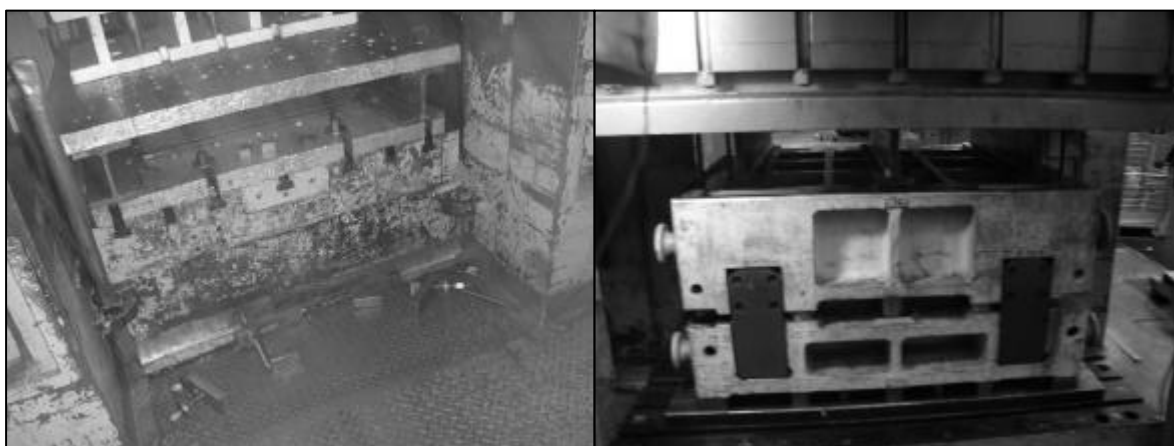
Figura 4.16 – Componentes do setup e regulagem de martelo.
