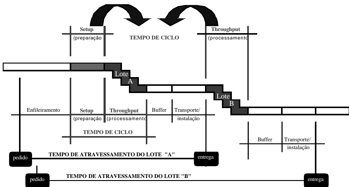
Figura 2.2 – Componentes do Tempo de Ciclo. Fonte: (SANTOS, 1999)
