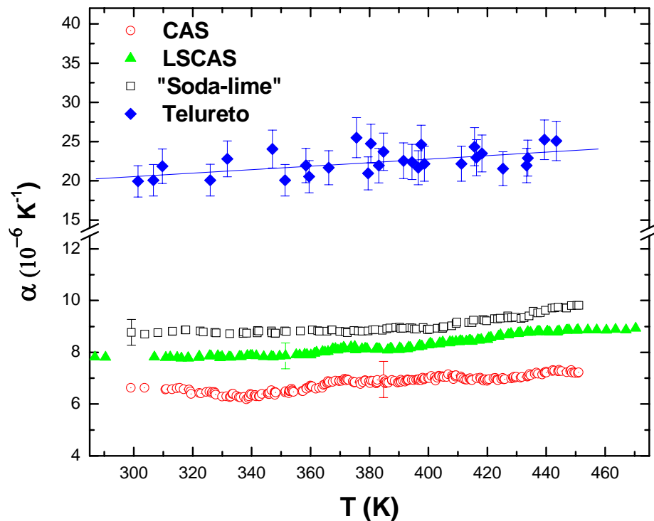
Figura 6.2 – Coeficiente de expansão térmica linear em função da temperatura para os vidros telureto, “soda-lime”, LSCAS e CAS. Linha contínua: ajuste linear.
