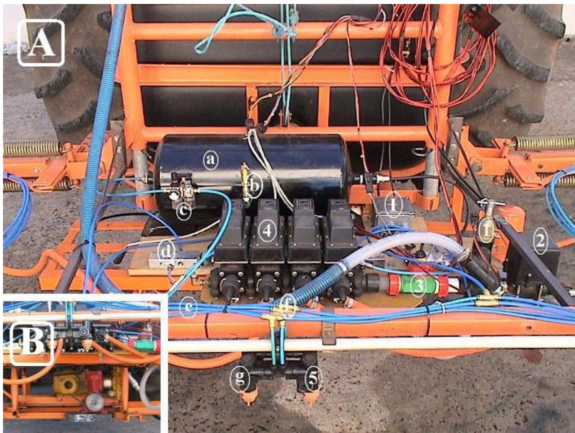
Figura 14. [A] Composição final do protótipo com seus principais componentes. Sistema hidráulico: (1) válvula de alívio; (2) válvula reguladora na linha de retorno; (3) fluxômetro de turbina; (4) válvula de seção sem retorno regulável; (5) bicos (Vario Select). Sistema pneumático: (a) reservatório 40 L; (b) válvula de alívio; (c) manômetro regulável e filtro; (d) válvula solenóide ou atuadores; (e) mangueiras pneumáticas de 1/4'; (f) T de distribuição; (g) bico comutador Vario Select; (I) placa controladora da comutação. [B] destaque do posicionamento do compressor no protótipo.
