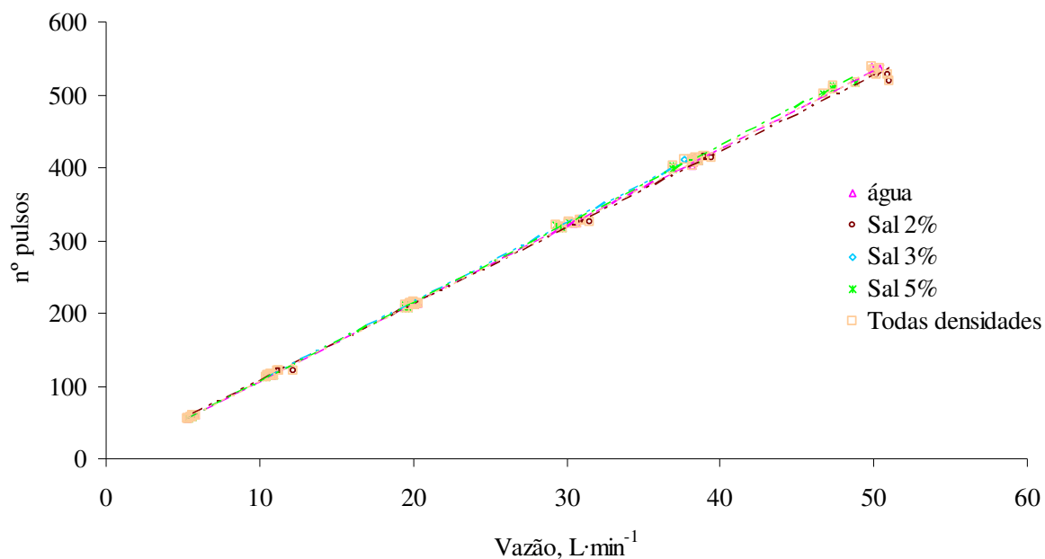
Figura 23. Regressão dos valores dos n^{\circ} de pulsos emitidos pelo fluxômetro de turbina em função da vazão nas diferentes densidades.
