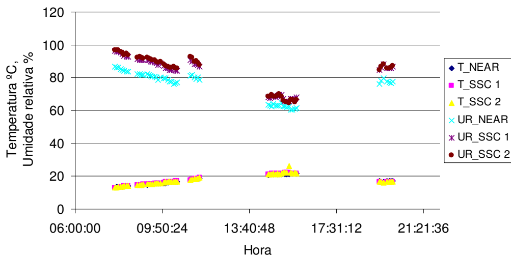
Figura 29. Temperatura e umidade relativa do ar para os sensores SSCs e termômetro referência durante o período das 06h30 às 20h30.
