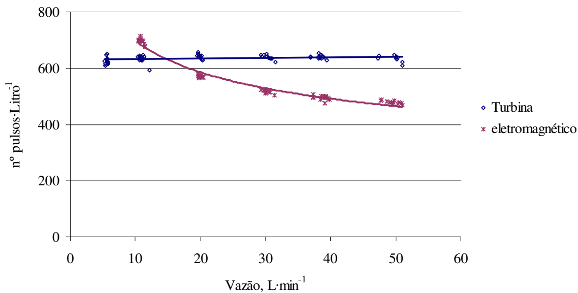
Figura 25. Valor de número de pulsos.Litro -1 em função da vazão em L.min -1 imposta ao sistema, para cada um dos fluxômetros, para todos os dados levantados.
