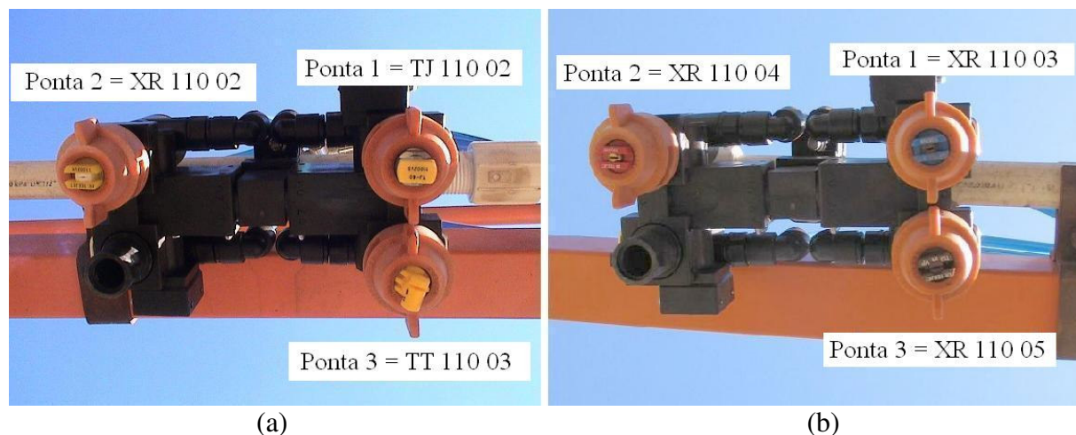
Figura 11. Disposição das pontas no bico conforme sua posição (a) para variação dos fatores climáticos e (b) para aplicação a taxa variada (VRT).
