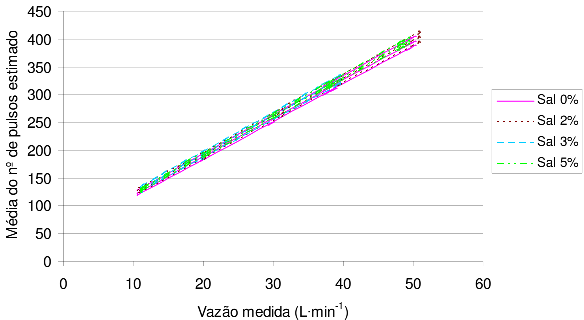
Figura 21. Valores máximos e mínimos de desvios da curva de regressão, da vazão em função do pulso, para as 4 concentrações de soluções salinas estudadas para o fluxômetro eletromagnético.
