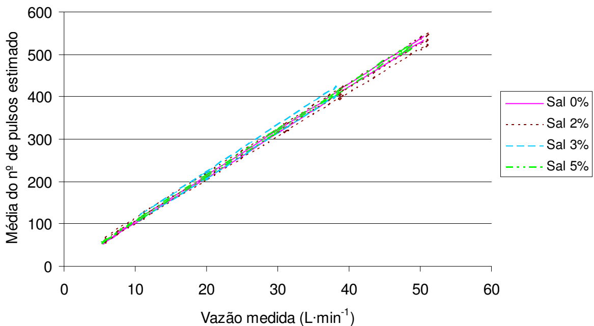
Figura 22. Valores máximos e mínimos de desvios da curva de regressão, da vazão em função do pulso, para as 4 concentrações de soluções salinas estudadas para o fluxômetro de turbina.
