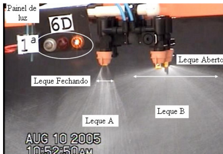
Figura 19. Momento da Comutação entre as pontas.
