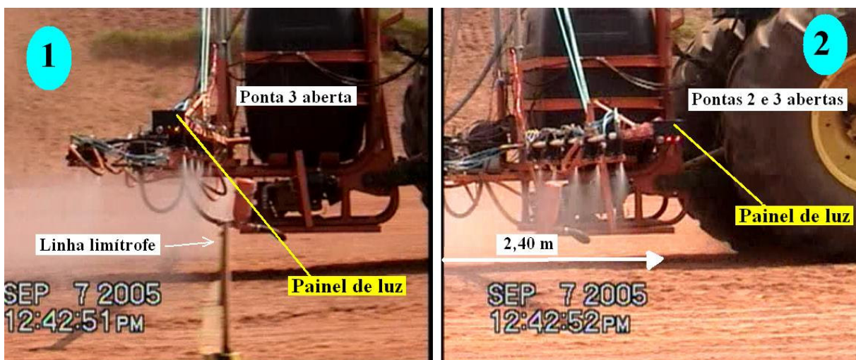
Figura 32. Instantes que o GPS passava pela estaca do alinhamento limítrofe (1) e; momento real da mudança de taxa aplicada (2).
