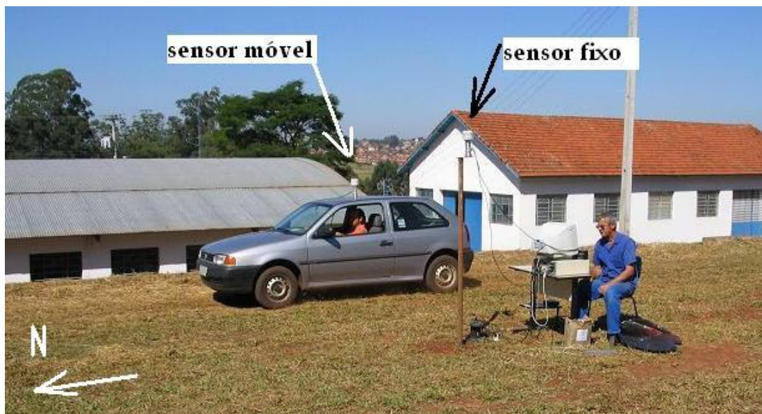
Figura 8. Ensaio do SSC em Condição Dinâmica.
