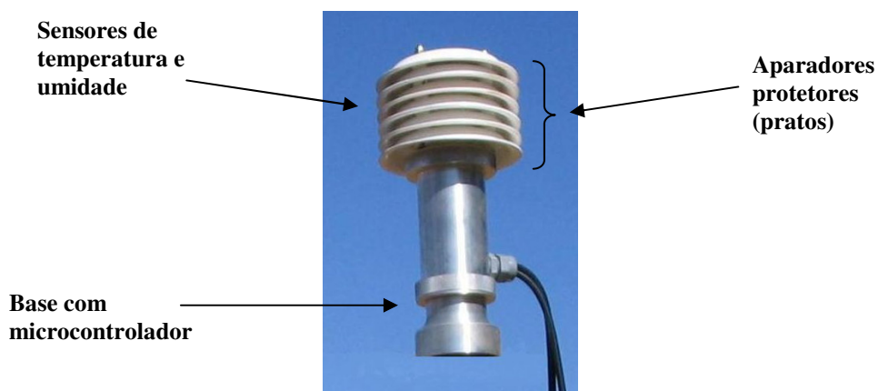
Figura 6. Abrigo dos sensores climáticos (SSC).
