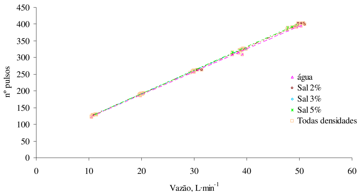
Figura 24. Regressão dos valores dos nº de pulsos emitidos pelo fluxômetro eletromagnético em função da vazão nas diferentes densidades.
