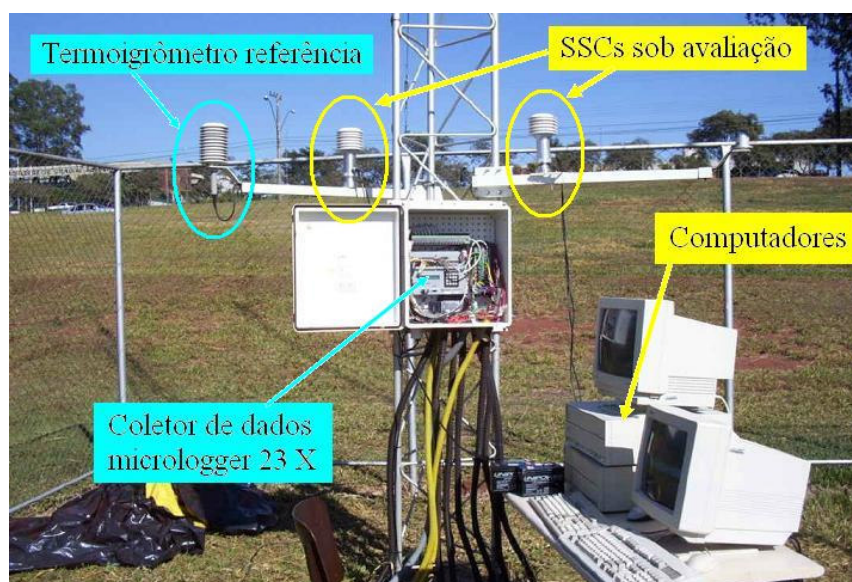
Figura 26. Ensaio estático dos SSCs, conectados a computadores e o termoiçrômetro referência, conectado ao coletor de dados Micrologger 23X.
