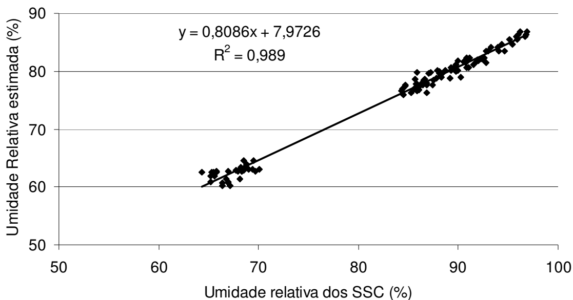
Figura 27. Equação de regressão para ajuste da umidade relativa do ar lida pelo SSC em função dos valores do termômetro referência.
