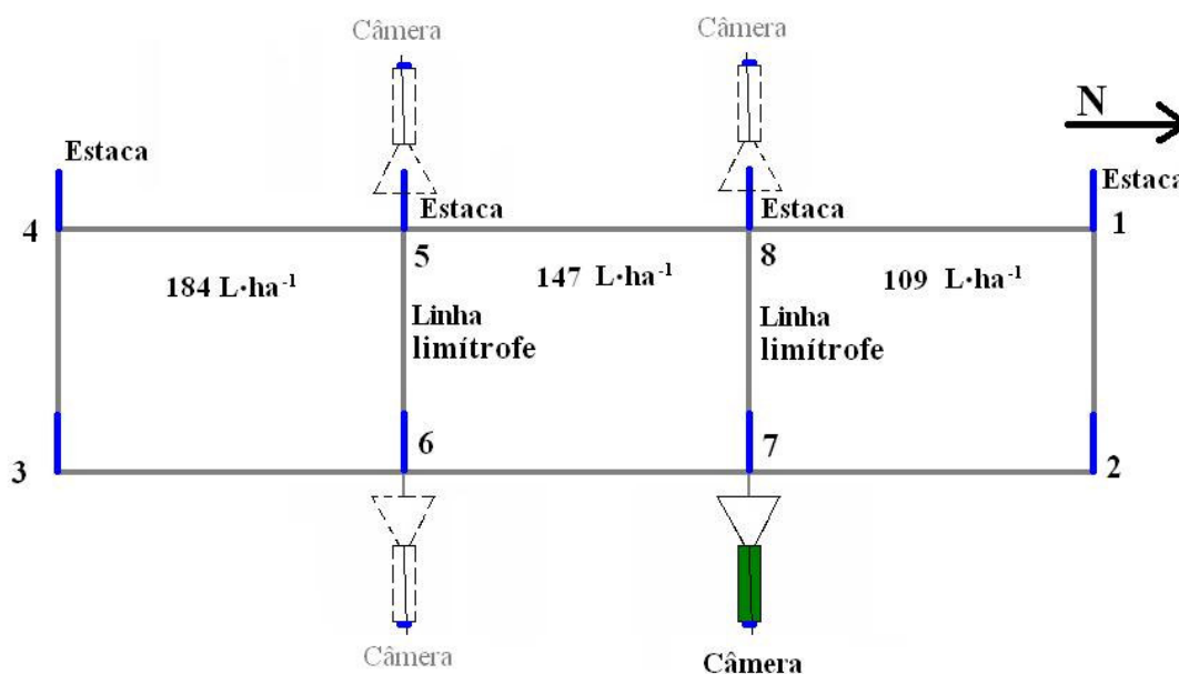
Figura 20. Posicionamento da câmera na estaca 7 e demonstração dos outros 3 pontos onde foi instalada a câmera, em alinhamento com as estacas que estão no alinhamento de divisa entre as subáreas de diferentes taxas de aplicação.
