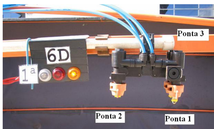
Figura 17. Painel de luz para mostrar o momento exato de acionamento das válvulas solenóides para comparação com os acionamentos das pontas do bico. Este exemplo é referente à primeira repetição do bico seis da barra direita do pulverizador.
