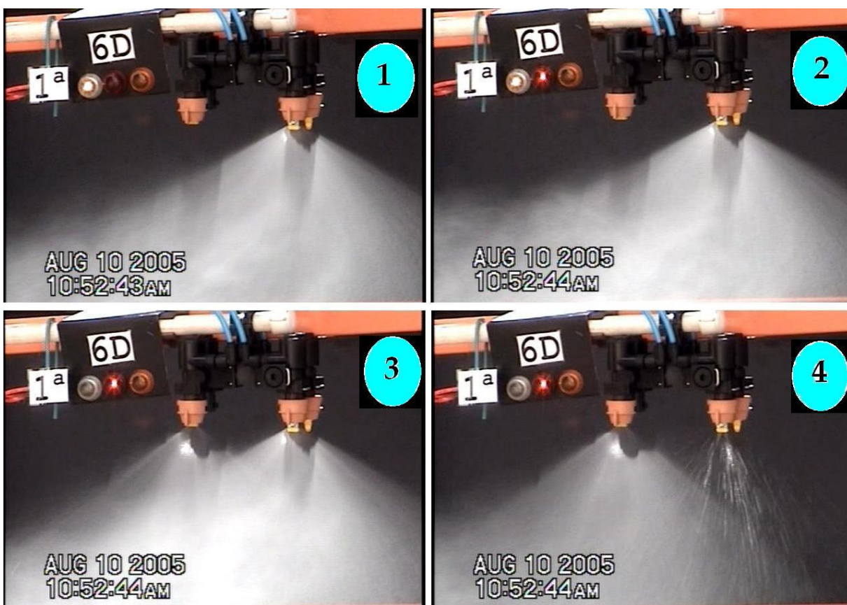
Figura 30. Seqüência da operação de comutação de pontas.
