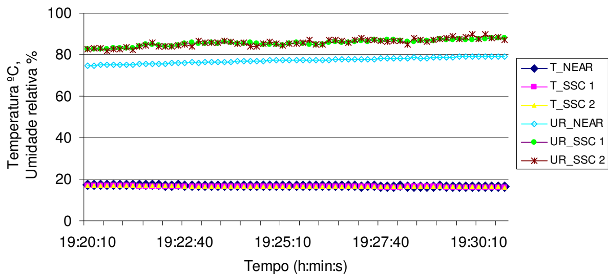
Figura 28. Temperatura e umidade relativa do ar para os sensores SSCs e termômetro referência durante o intervalo de tempo de 10 minutos.
