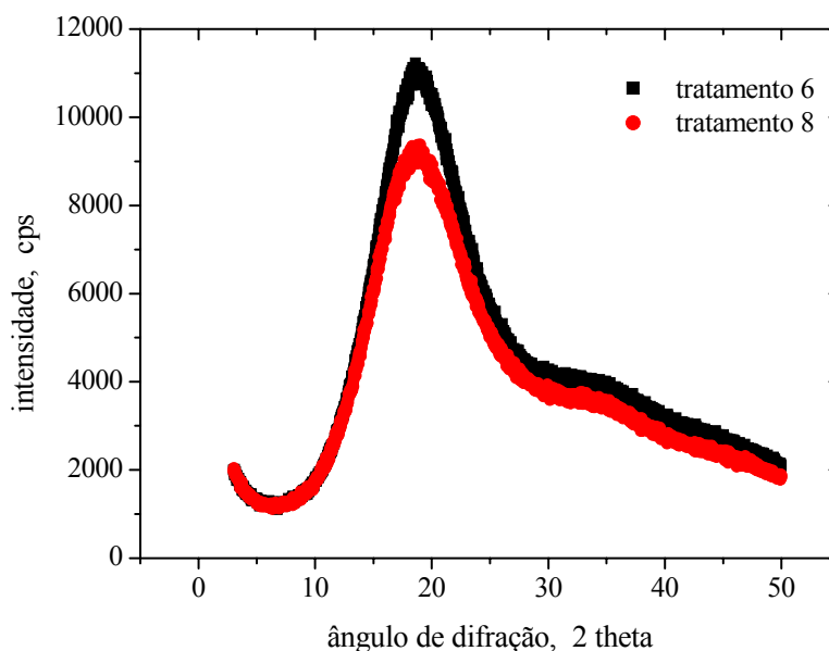
Figura 39. Difractogramas de raios-X das maltodextrinas de batata-doce dos tratamentos 6 e 8.
