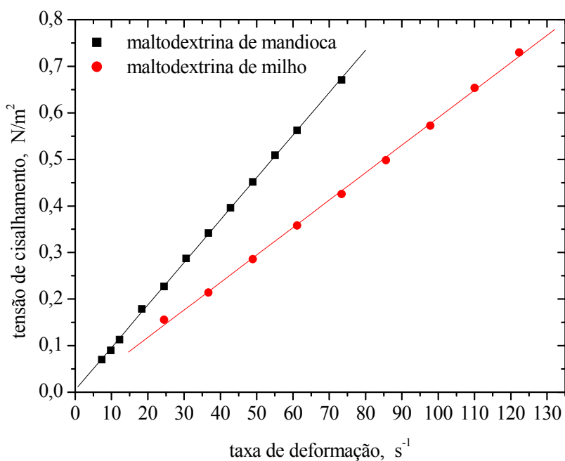
Figura 29. Tensão de cisalhamento em função da taxa de deformação para soluções de maltodextrinas comerciais de mandioca e milho a 20% a 25°C.
