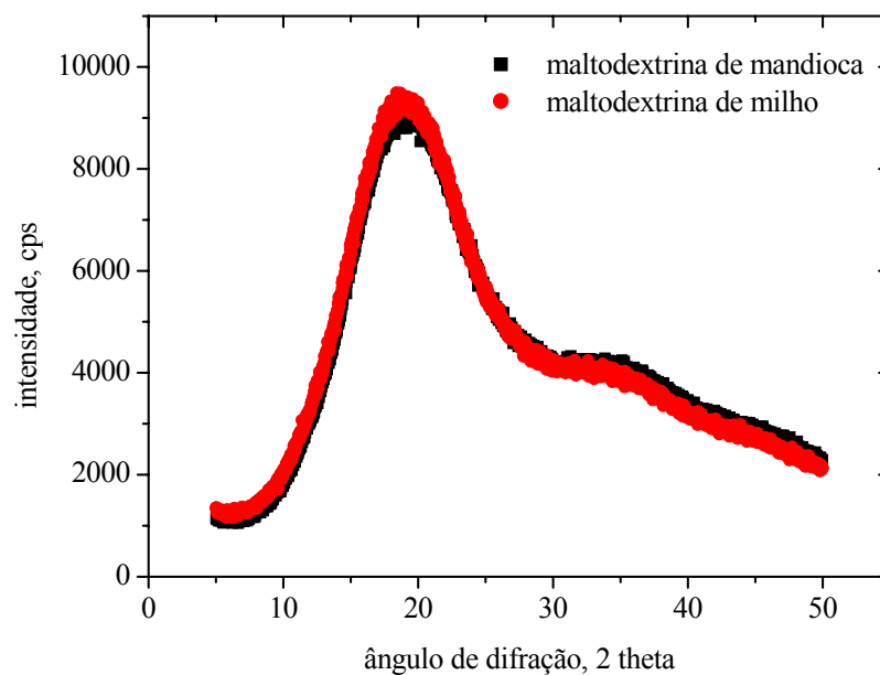
Figura 40. Diffractogramas de raios-X das maltodextrinas comerciais de mandioca e milho.
