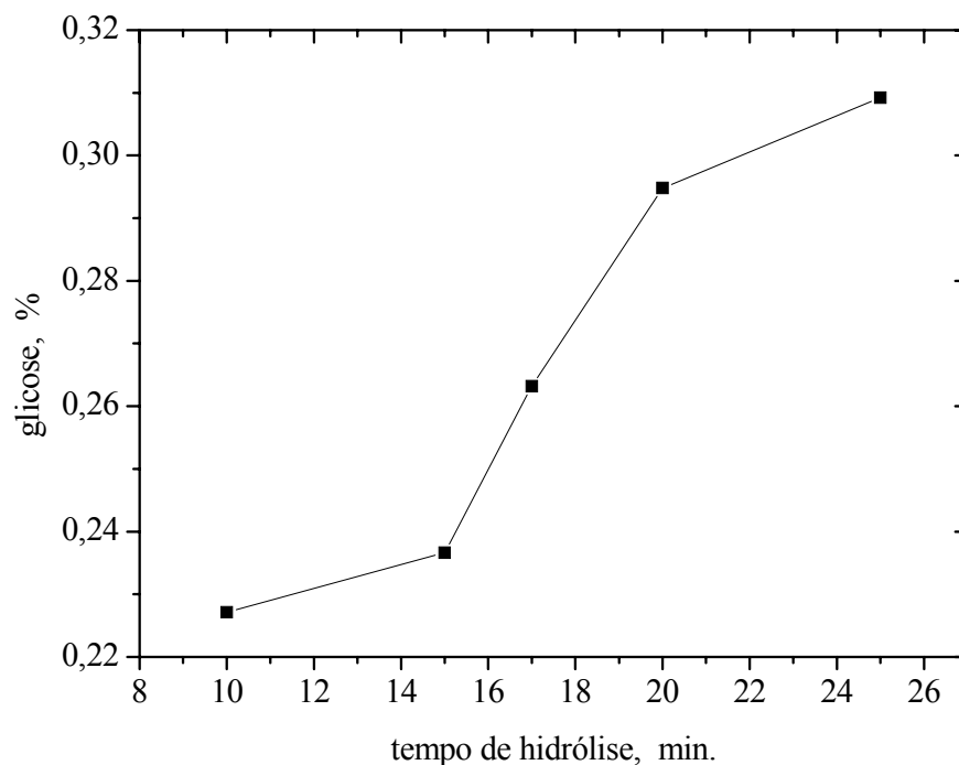
Figura 20. Efeito do tempo de hidrólise na porcentagem de glicose das maltodextrinas de mandioca, mantendo a agitação no ponto central (35rpm).
