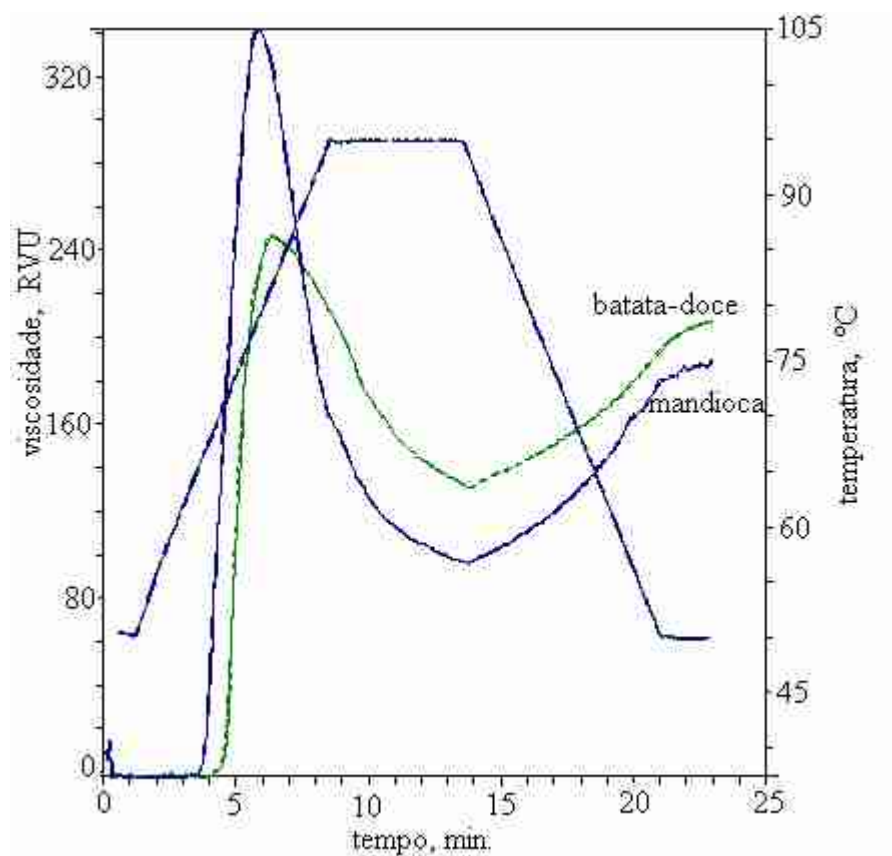
Figura 18. Curva viscoamilográfica de amidos de mandioca e batata-doce.
