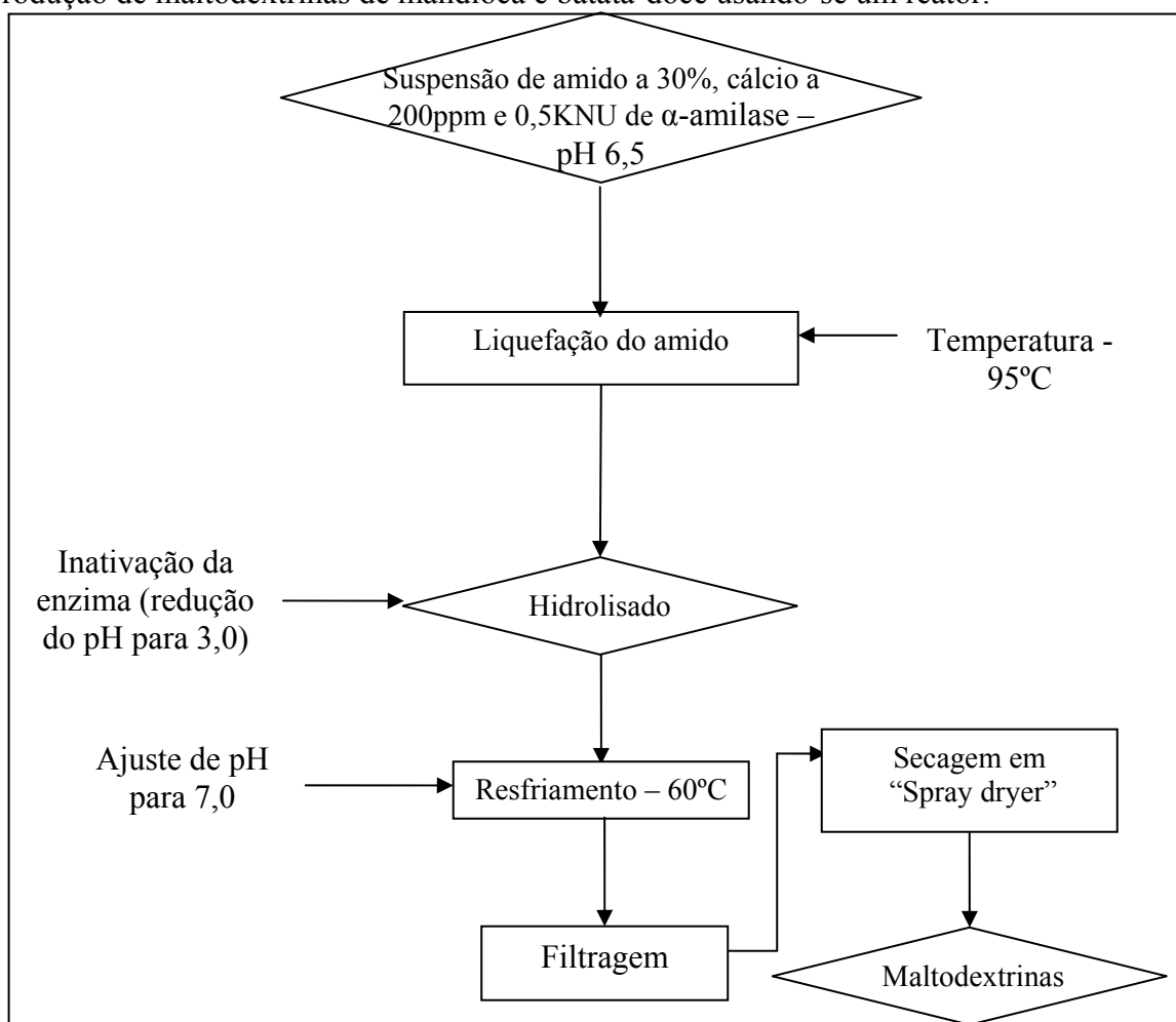
Figura 12. Fluxograma da produção de maltodextrinas de mandioca e batata-doce.
