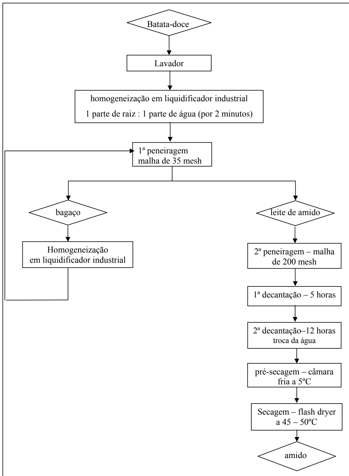
Figura 10. Fluxograma do processo de obtenção do amido de batata-doce.
