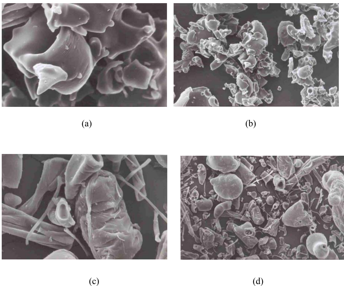
Figura 37. Micrografias de maltodextrinas comerciais secas em “spray dryer” por atomização observadas ao microscópio eletrônico de varredura (MEV). (a) maltodextrina de mandioca, aumento de 1000 X, (b) maltodextrina de mandioca, aumento de 200 X, (c) maltodextrina de milho, aumento de 1000 X, (d) maltodextrina de milho, aumento de 200 X.
