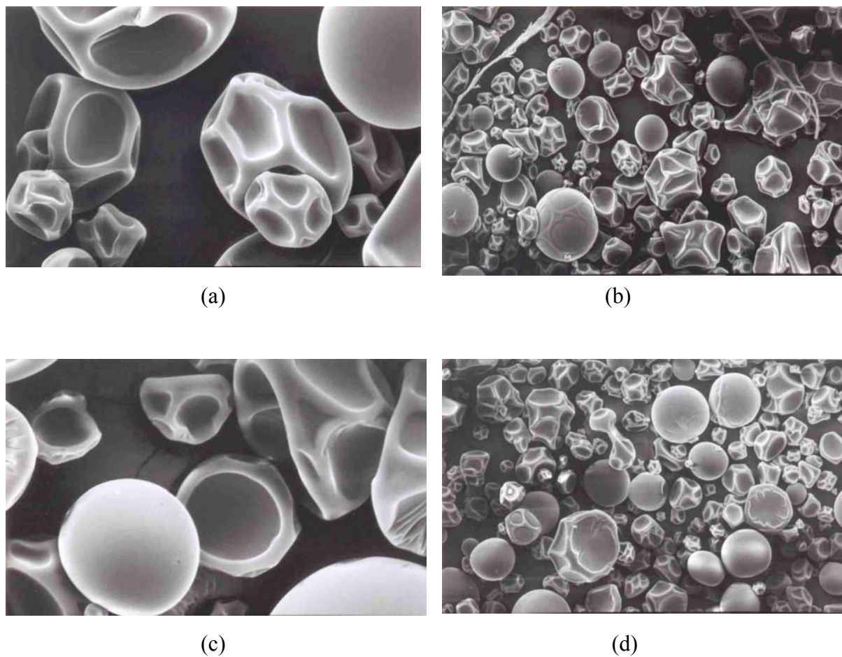
Figura 35. Micrografias de maltodextrinas de mandioca secas em “spray dryer” por pulverização observadas ao microscópio eletrônico de varredura (MEV). (a) tratamento 6, aumento de 1000 X, (b) tratamento 6, aumento de 200 X, (c) tratamento 8, aumento de 1000 X, (d) tratamento 8, aumento de 200 X.
