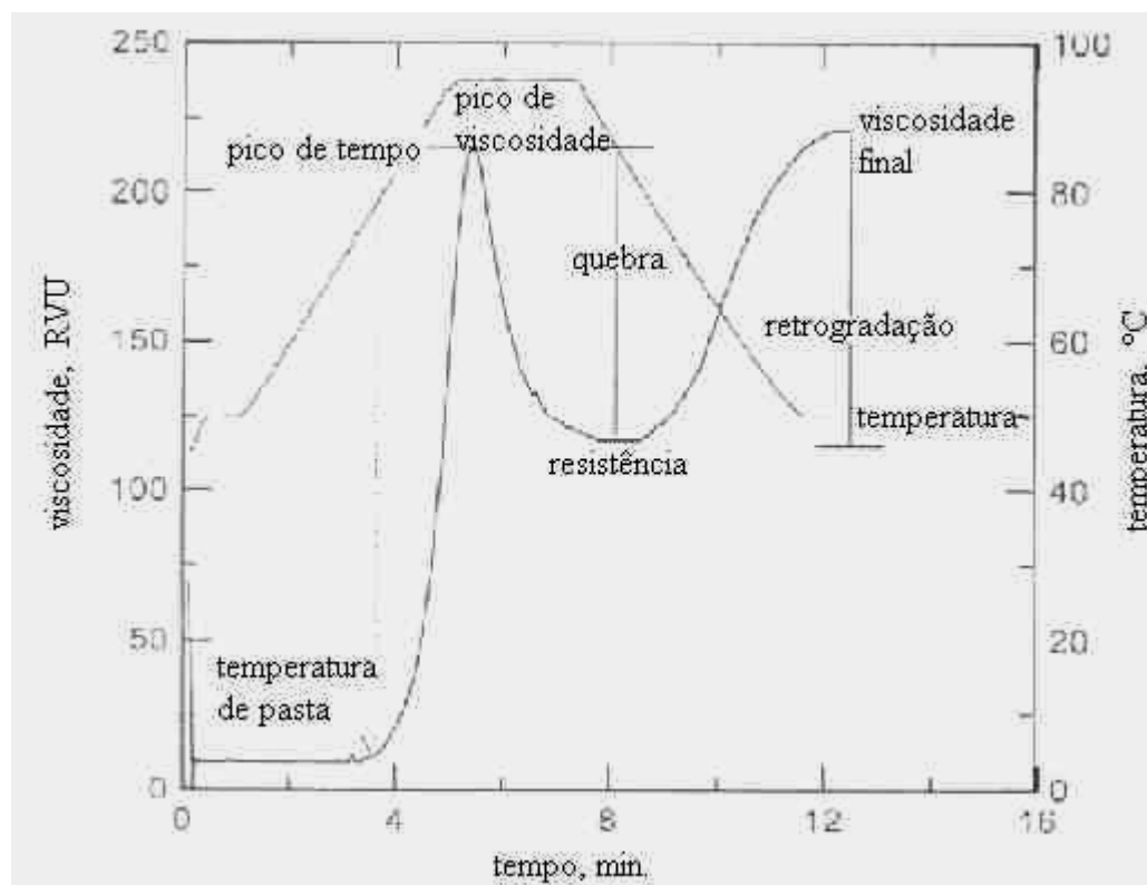
Figura 11. Parâmetros avaliados na curva amilográfica de amido.
