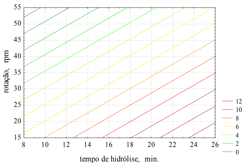
Figura 32. Gráfico da curva de contorno para a viscosidade da maltodextrina de mandioca a concentração de 20% em função do tempo de hidrólise e da agitação.
