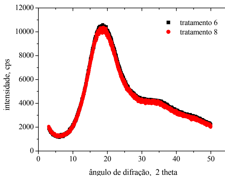
Figura 38. Difratogramas de raios-X das maltodextrinas de mandioca dos tratamentos 6 e 8.
