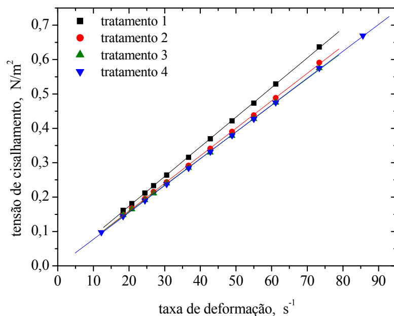
Figura 28. Tensão de cisalhamento em função da taxa de deformação para solução de maltodextrina de batata-doce a 30% a 25°C.
