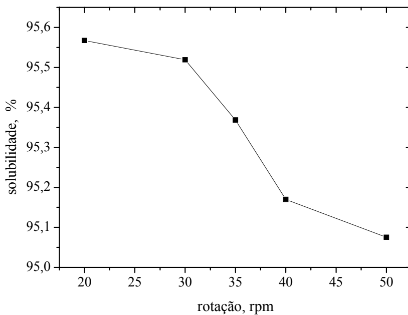
Figura 22. Efeito da agitação na solubilidade em água das maltodextrinas de mandioca, mantendo o tempo de hidrólise no ponto central (17 min.).
