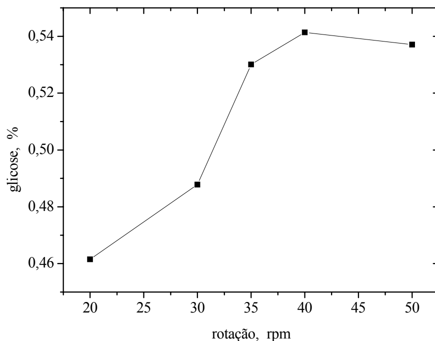
Figura 21. Efeito da agitação na porcentagem de glicose das maltodextrinas de batata-doce, mantendo o tempo de hidrólise no ponto central (17 min.).
