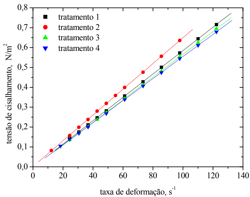
Figura 25. Tensão de cisalhamento em função da taxa de deformação para solução de maltodextrina de mandioca a 20% a 25°C.
