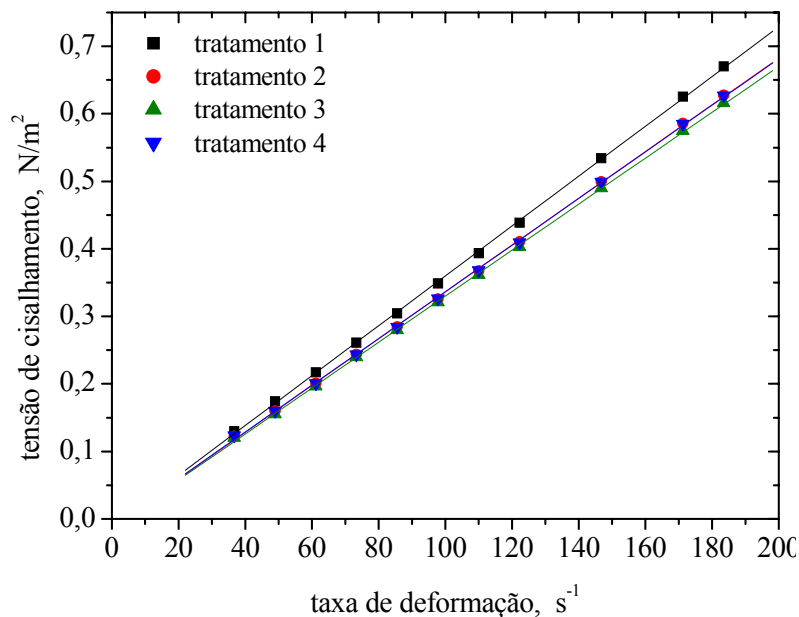
Figura 27. Tensão de cisalhamento em função da taxa de deformação para solução de maltodextrina de batata-doce a 20% a 25°C.
