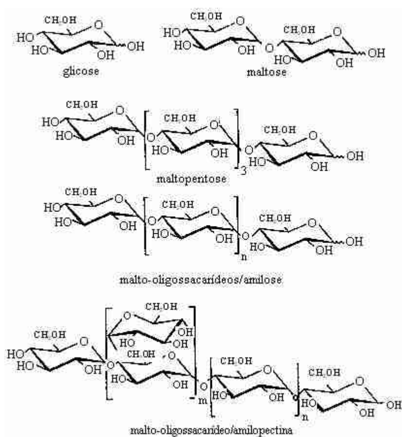
Figura 8. Principais componentes estruturais da maltodextrina. Fonte: Kennedy; Knill e Taylor (1995).
