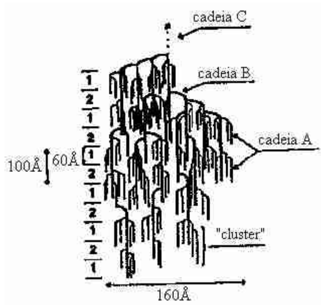
Figura 5. Modelo de cluster proposto para amilopectina. Fonte: French (1984).
