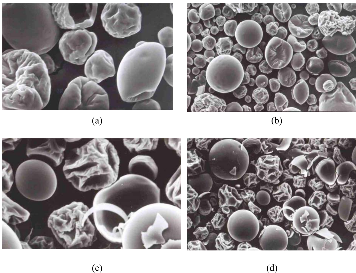
Figura 36. Micrografias de maltodextrinas de batata-doce secas em “spray dryer” por pulverização observadas ao microscópio eletrônico de varredura (MEV). (a) tratamento 6, aumento de 1000 X, (b) tratamento 6, aumento de 200 X, (c) tratamento 8, aumento de 1000 X, (d) tratamento 8, aumento de 200 X.
