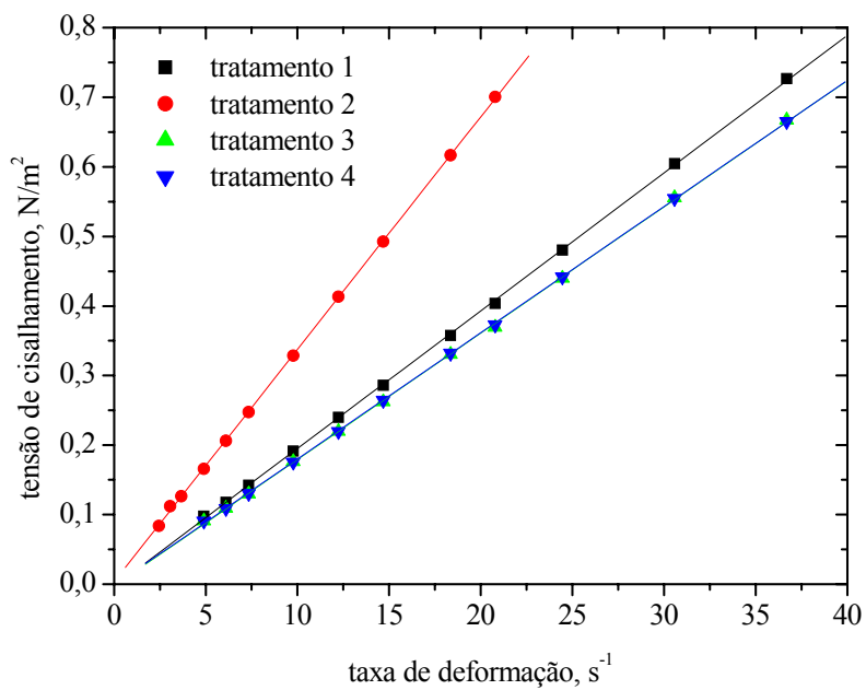
Figura 26. Tensão de cisalhamento em função da taxa de deformação para solução de maltodextrina de mandioca a 30% a 25°C.
