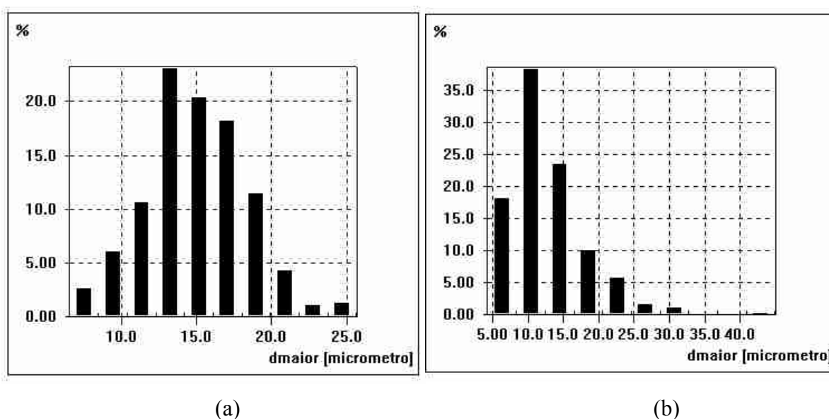
Figura 16. Distribuição dos grânulos de amidos de mandioca (a) e batata-doce (b).
