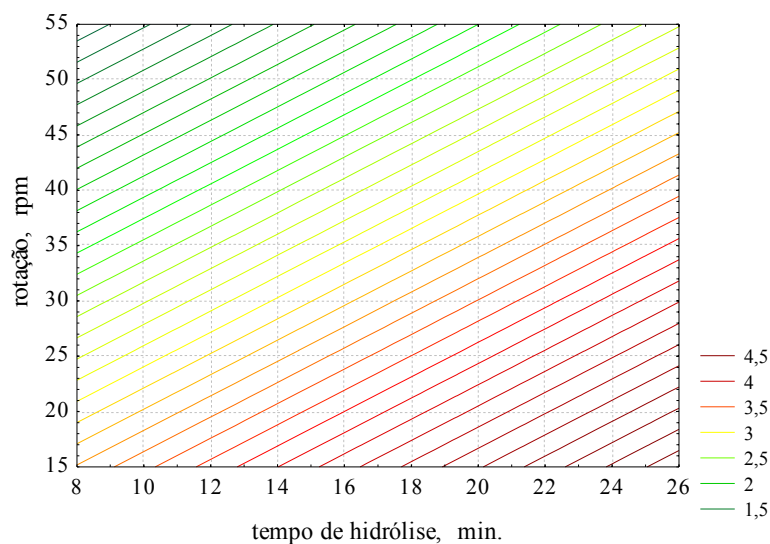
Figura 34. Gráfico da curva de contorno para a viscosidade da solução de maltodextrina de batata-doce a 20% em função do tempo de hidrólise e da agitação.
