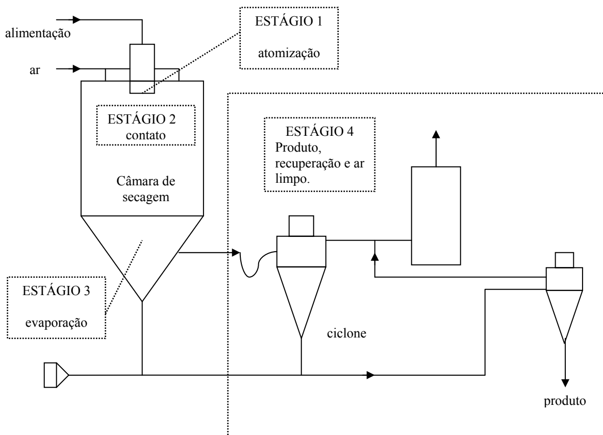
Figura 9. Esquema de funcionamento do “spray dryer”. Fonte: Masters (1979).
