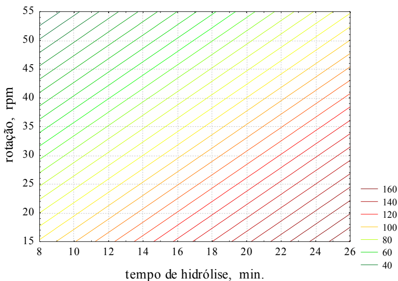
Figura 24. Gráfico da curva de contorno para a solubilidade das maltodextrinas de batata-doce para as variáveis de tempo de hidrólise e agitação.
