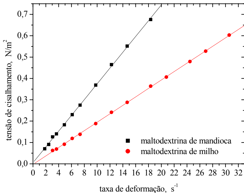
Figura 30. Tensão de cisalhamento em função da taxa de deformação para soluções de maltodextrinas comerciais de mandioca e milho a 30% a 25°C.
