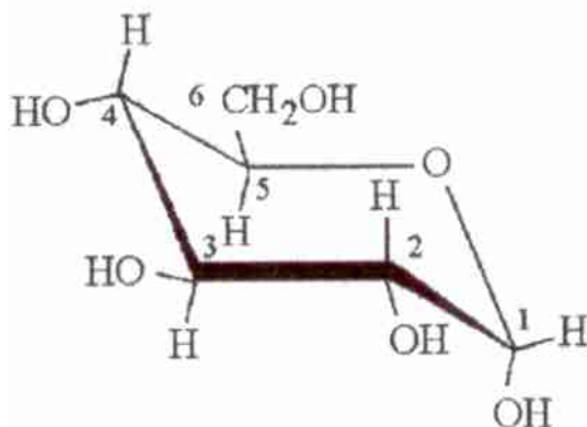
Figura 2. Molécula de glicose. Fonte: Swinkels (1985).
