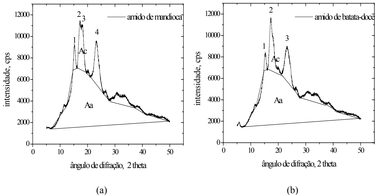
Figura 17. Difractogramas de raios-X de grânulos de amidos de mandioca (a) e batata-doce (b).
