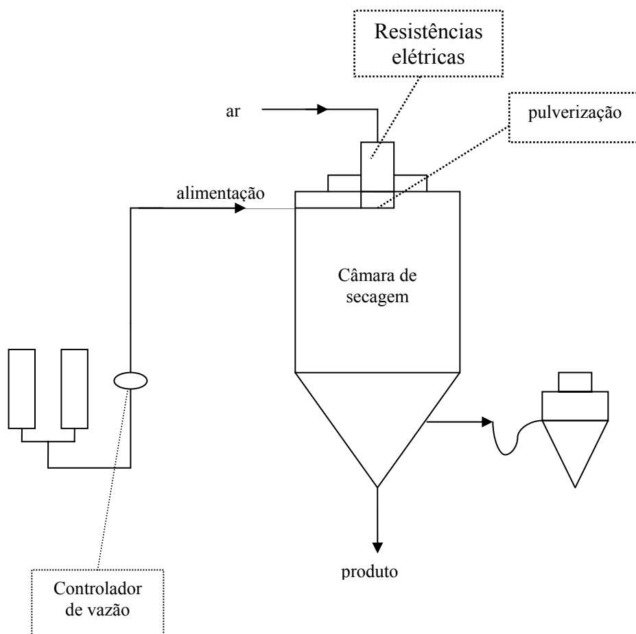
Figura 14. Esquema de funcionamento do “spray dryer” utilizado na secagem das maltodextrinas.
