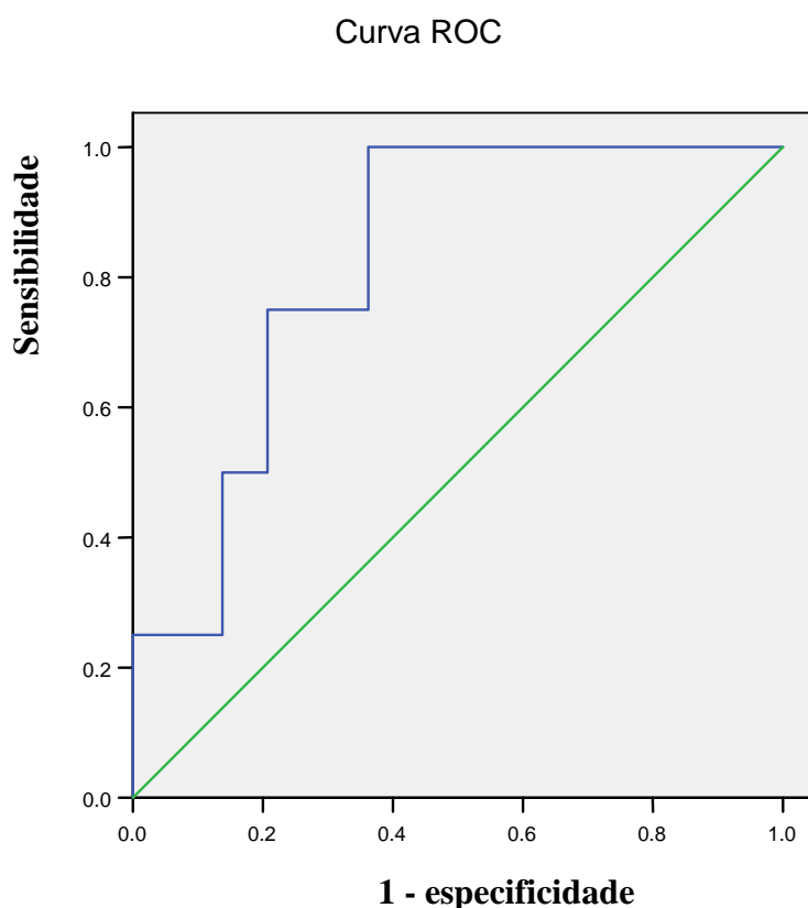
Gráfico 4: Curva ROC da concentração sérica pré-operatória do rs-FNT I com respeito a previsão de resposta desfavorável no pós-operatório de revascularização do miocárdio e operações valvares.
