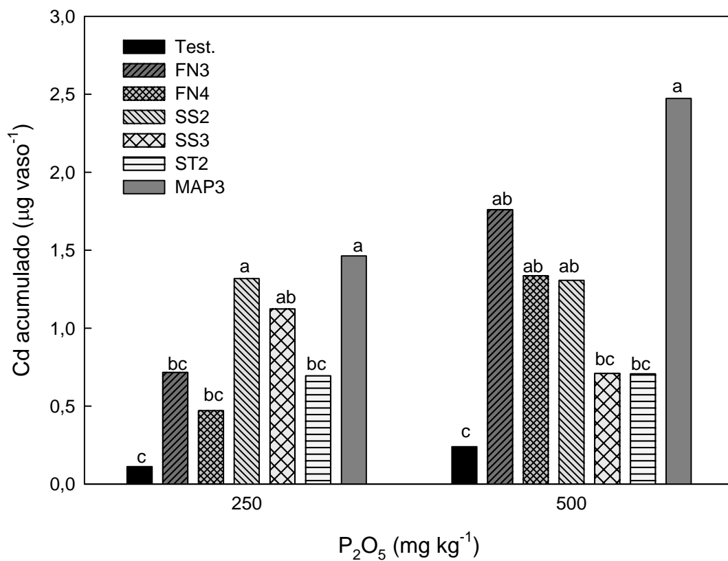
Figura 10. Conteúdo de Cd acumulado pelas raízes da aveia preta com adição de fertilizantes comerciais. Médias seguidas por mesma letra na dose não diferem pelo teste de Tukey ao nível de 5% de probabilidade.
