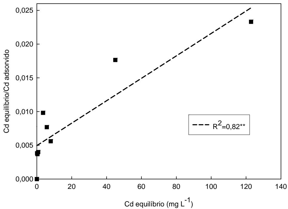
Figura 16. Ajuste dos dados experimentais do Argissolo Vermelho distrófico pela equação linearizada de Langmuir.
