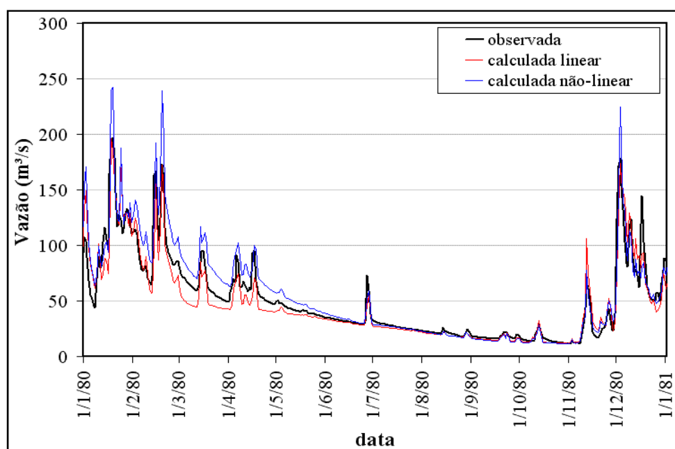
Figura 6.13: Hidrogramas observado e calculados com reservatório linear e não-linear de janeiro de 1980 a janeiro de 1981.
