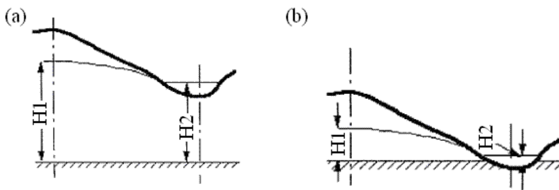
Figura 4.3: Seção esquemática do aquífero-rio: (a) pequena variação no escoamento com a profundidade H ; (b) variação significativa na profundidade de escoamento. (fonte: Chapman, 1999).
