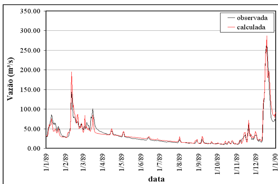
Figura 6.15: Hidrogramas de vazões diárias calculado e observado no rio Paranaíba de janeiro de 1989 a janeiro de 1990.
