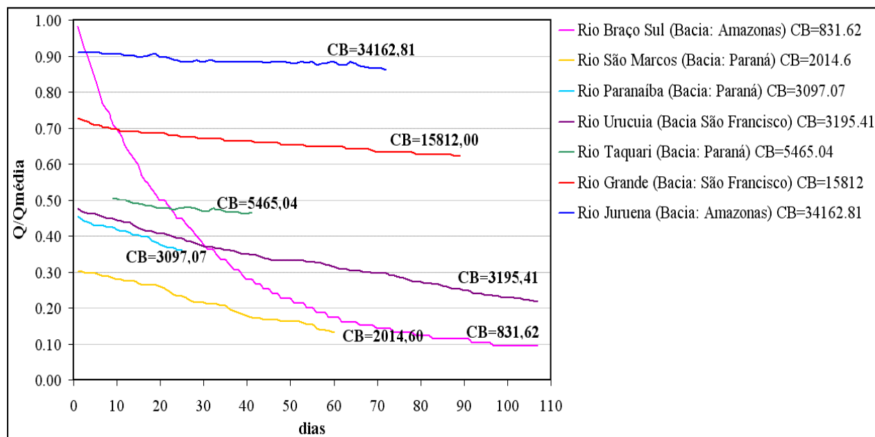
Figura 5.6: Valores do parâmetro CB (em horas) para recessões de diferentes rios brasileiros.
