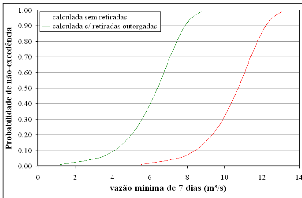
Figura 6.20: Curvas de frequência de vazões mínimas de 7 dias calculadas no rio Paranaíba no período de aplicação (01/01/1988 – 31/12/2005) sem e com as retiradas outorgadas na bacia.
