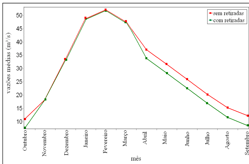
Figura 6.24: Vazões médias mensais calculados sem e com retiradas de 25% da Q_{7,10} e 3,5% da Q_{recarga} na bacia do Alto Rio Paranaíba (abril à outubro).
