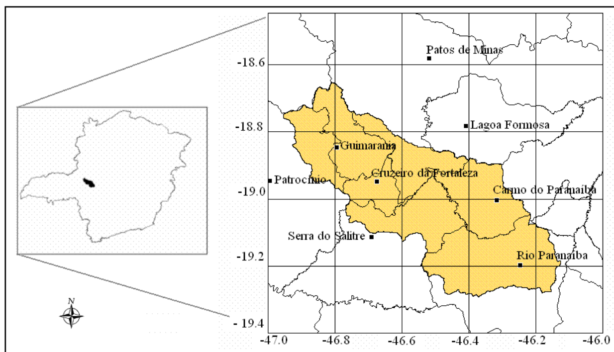
Figura 6.1: Localização da bacia em estudo.
