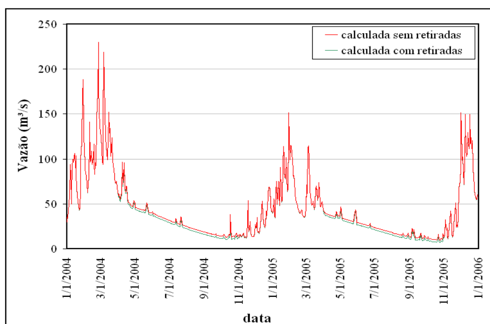
Figura 6.23: Hidrogramas calculados sem e com retiradas de 25% da Q_{7,10} e 3,5% da Q_{\text{recarga}} na bacia do Alto Rio Paranaíba (abril à outubro).
