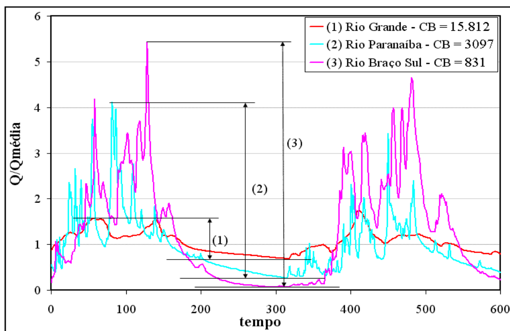
Figura 5.7: Hidrogramas dos rios Grande, Paranaíba e Braço Sul.
