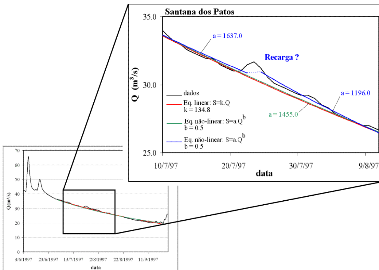
Figura 4.4: Ajuste de recessão com reservatório linear e não-linear no rio Paranaíba.
