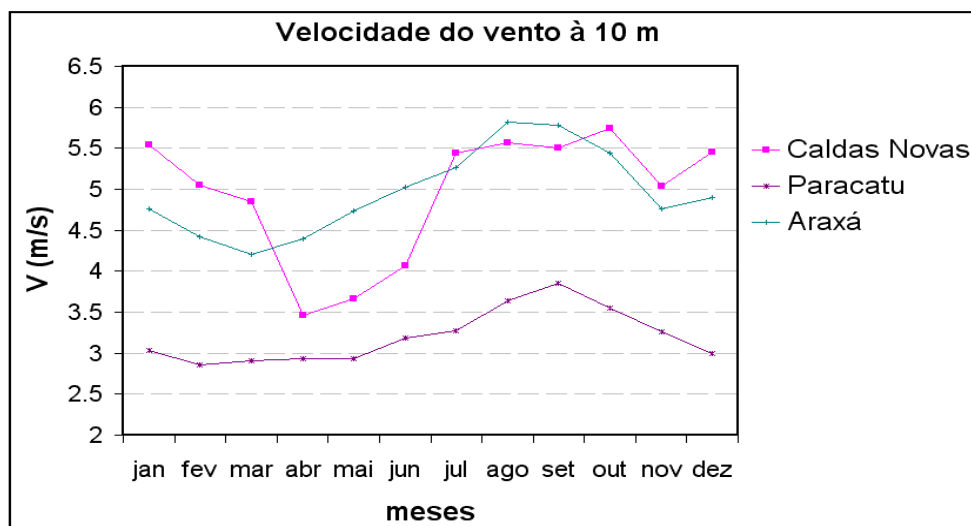
Figura E.4: Médias mensais dos ventos à 10 m nos postos climatológicos.
