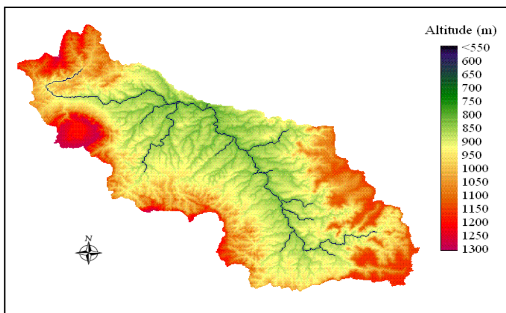
Figura 6.2: Relevo da bacia do Alto Rio Paranaíba.
