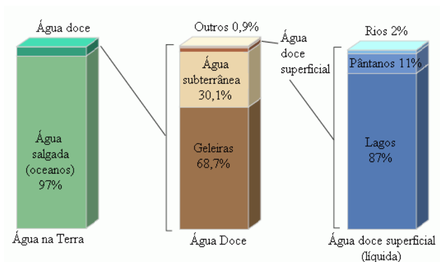
Figura 2.1: Distribuição global de água (fonte: adaptado de Estados Unidos, 2006).
