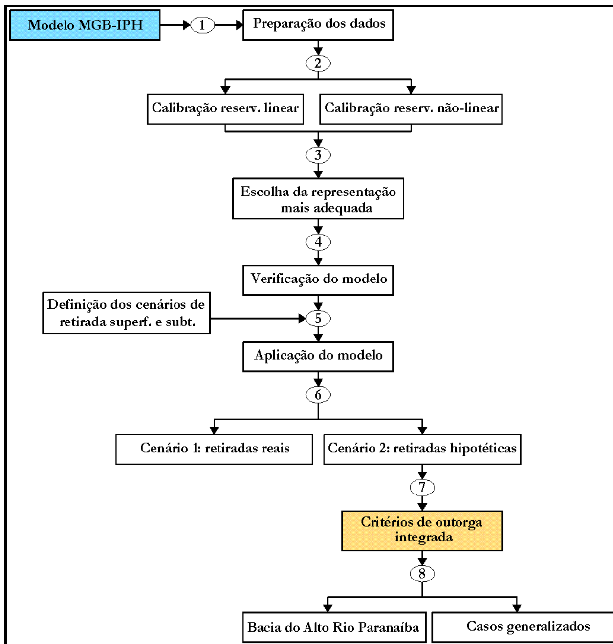
Figura 5.1: Fluxograma metodológico.
