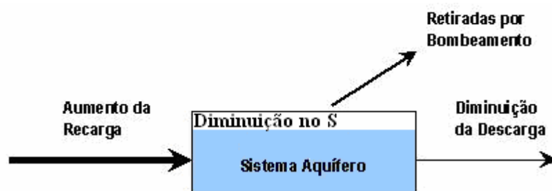
Figura 2.5: Balanço no aquífero em situação de desequilíbrio (adaptado de Alley et al. , 1999).
