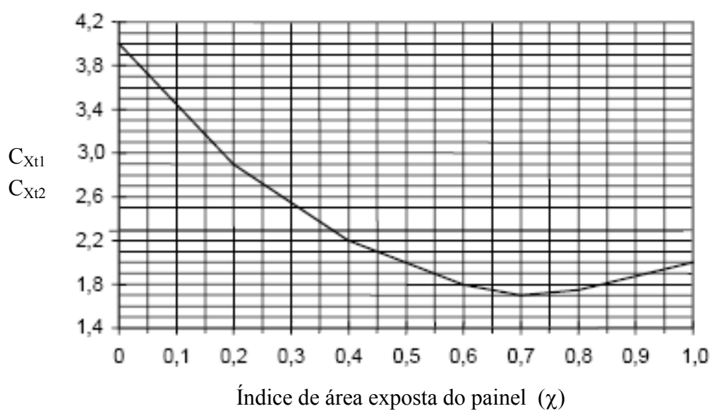
Figura A.7: Coeficientes de arrasto C_{Xt1} e C_{Xt2} para torres treliçadas formadas por barras com superfícies planas.
