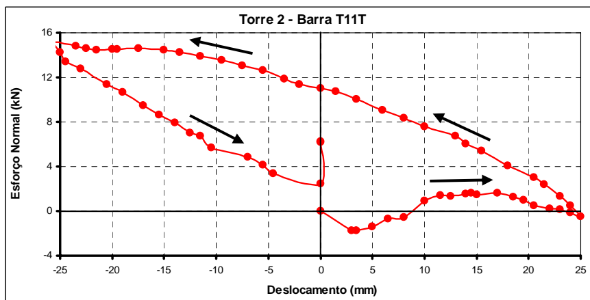
Figura 6.19: Esforço normal (kN) na barra T11T da torre “2” para deslocamentos impostos na base.
