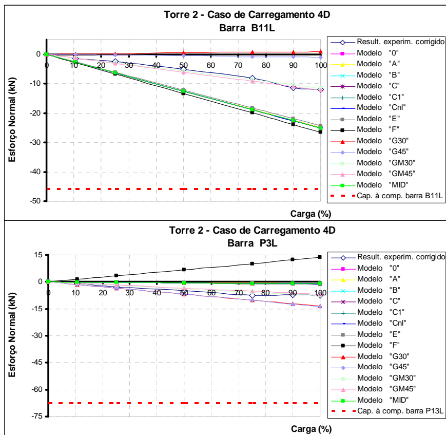
Figura 7.15: Esforço normal nas barras B11L e P3L da torre “2” para o caso de carregamento “4D”.
