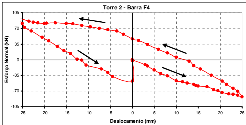
Figura 6.18: Esforço normal (kN) na barra F4 da torre “2” para deslocamentos impostos na base.
