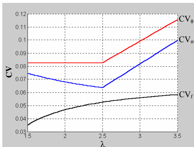
Figura 3.1: Incerteza total ( CV_\phi ), de modelo ( CV_m ) e física ( CV_f ) na resistência a compressão de placas de aço ensaiadas em laboratório.
