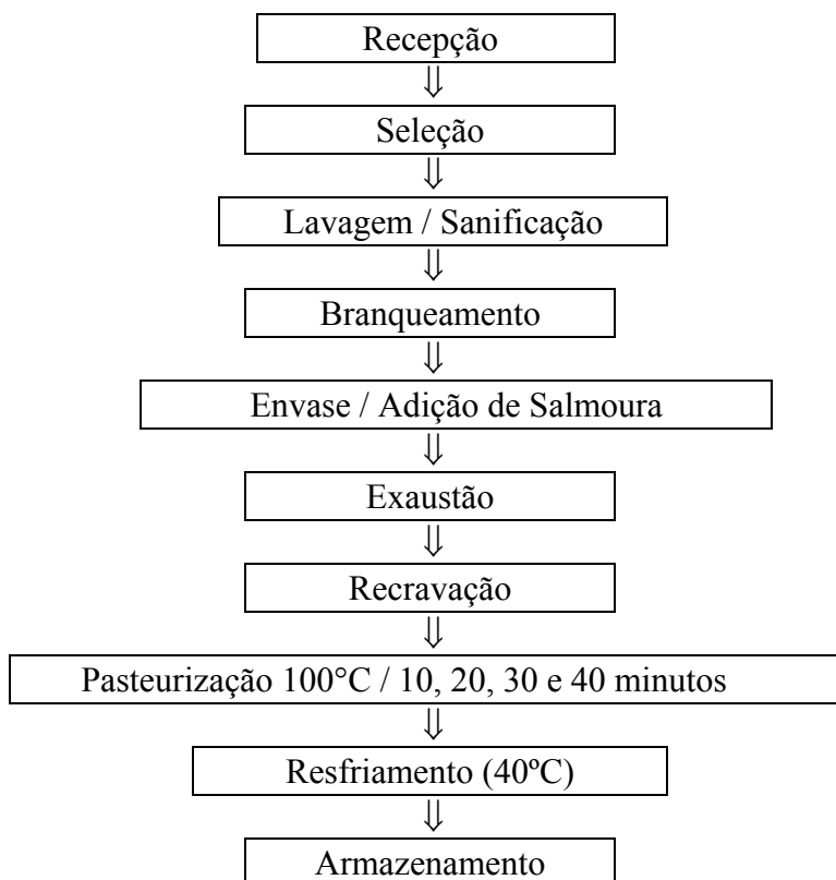
Figura 3.1 Fluxograma geral do processamento da pimenta em conserva
