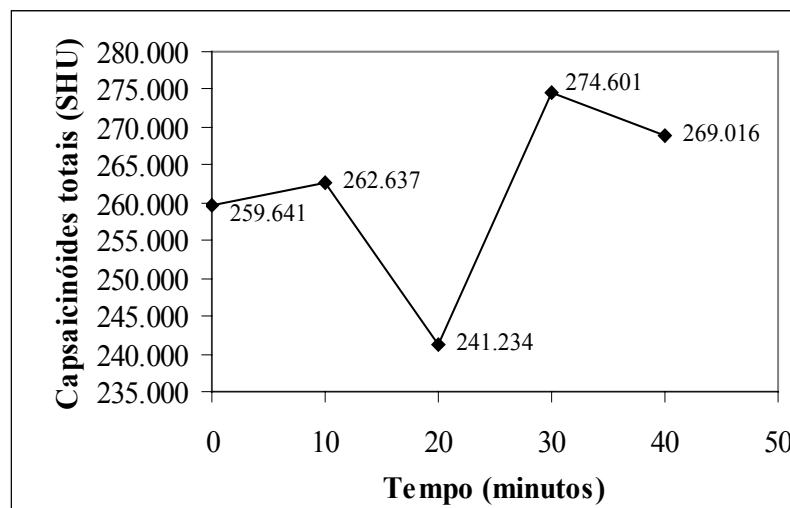
Figura 4.15 Determinação dos Capsaicinóides totais (SHU) do cultivar CNPH 0280 a 100°C por 0, 10, 20, 30 e 40 minutos
