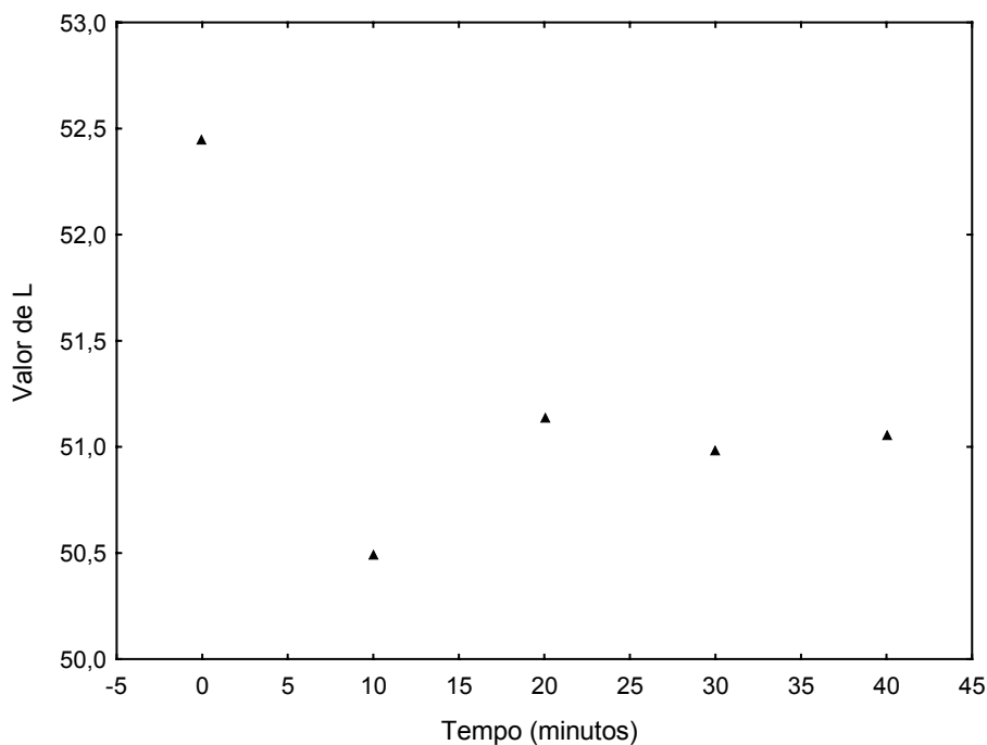
Figura 4.6 - Degradação térmica da Luminosidade do cultivar CNPH 0280 a 100°C por 0, 10, 20, 30 e 40 minutos
