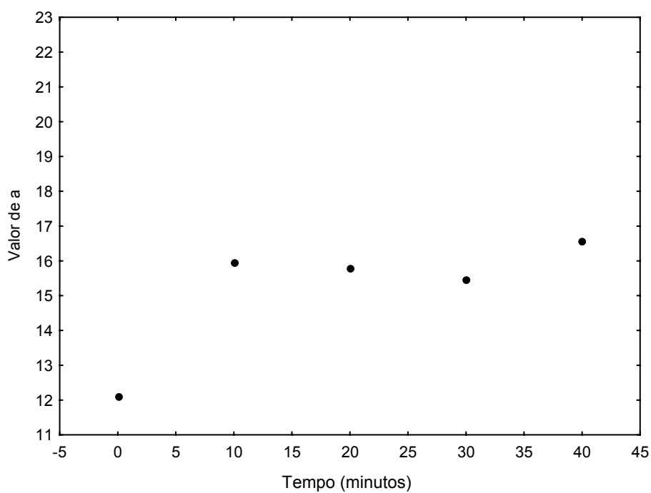
Figura 4.9 - Degradação térmica do valor de a do cultivar CNPH 0280 a 100°C por 0, 10, 20, 30 e 40 minutos
