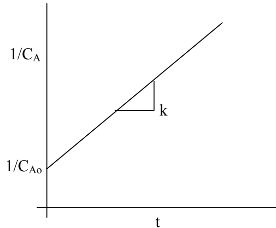
Figura 2.3 Modelo de reação de segunda ordem
