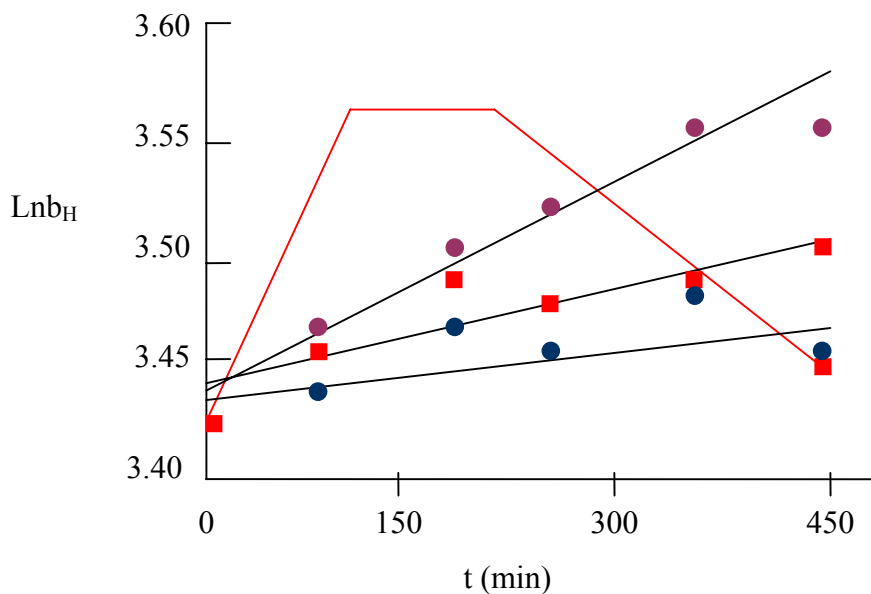
Figura 2.1 Modelo de reação de primeira ordem
