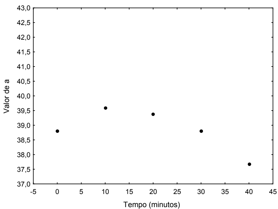
Figura 4.8 - Degradação térmica do valor de a do cultivar CNPH 0053 a 100°C por 0, 10, 20, 30 e 40 minutos
