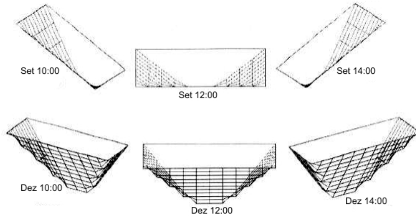
Fig. 54. Avaliação do SCE em Set. e Dez. Tempo crítico para o Sul às 12:00, ao E 10:00 e O às 14:00h. Fonte: Capeluto, 2003
