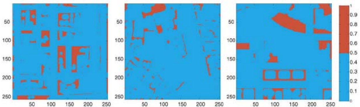
Fig. 72. Zonas não-passivas (mais de 6 m para dentro das fachadas). Fonte: Steemers et al., 2005
