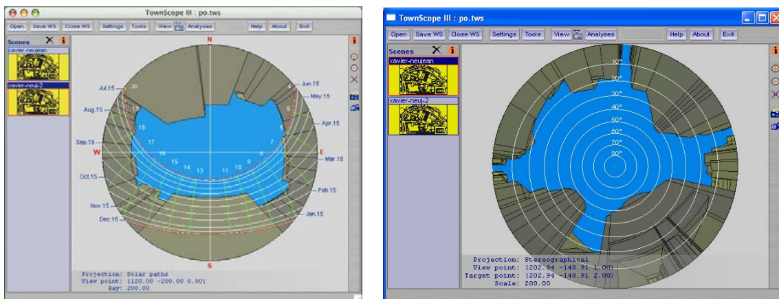
Fig. 62 e 63. Janelas da trajetória solar e vista estereográfica dos ângulos de elevação. Fonte: Townscope III
