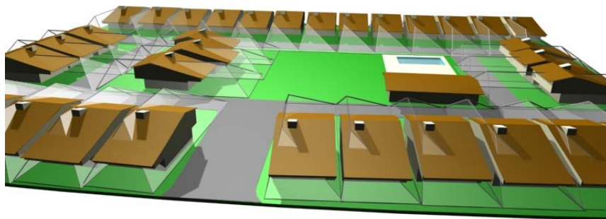
Fig. 111. Vista em 3d. 21 de junho. 15:00 h.
