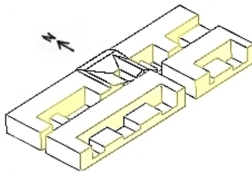
Fig. 3. Desenho de Walter Graham publicado por KNOWLES (1974). Planta isométrica de um bloco de Olynthus mostra que os volumes construídos tomam vantagens da orientação sul. Adaptação: Daniel B. Perez, 2006.
