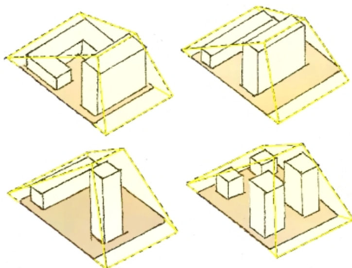
Fig. 73. Opções de diferentes tipologias dentro do volume definido pelo envelope solar. Fonte: Casablanca et al., 2001.
