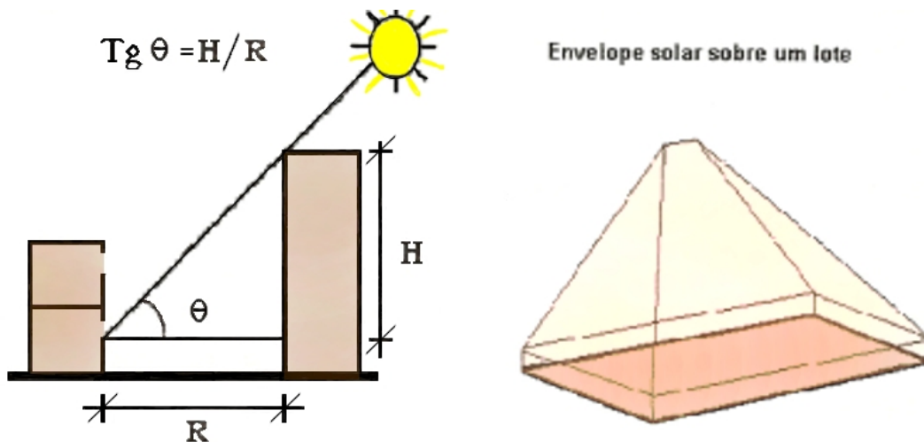
Fig. 33. Construção do envelope solar. Ângulos de obstrução. Fonte: Assis, 2000, adaptado por Daniel B. Pérez, 2006.
