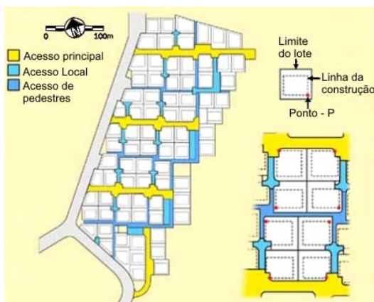
Fig. 60. Plano de Neve-Zin. Fonte: Pearlmutter, 2000
