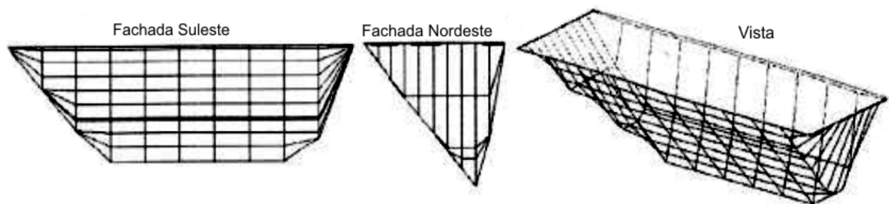
Fig. 56. SCE obtido para uma edificação inclinada a 30° do Norte. De maio a dezembro entre 10:00 e 14:00 h. Data crítica para a fachada norte: Junho 14:00 h e para a fachada sul: Setembro 10:00 h. Fonte: Capeluto, 2003.
