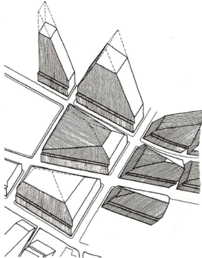
Fig. 37. Envelopes Solares. Fonte: Brown & Dekay (2004)
