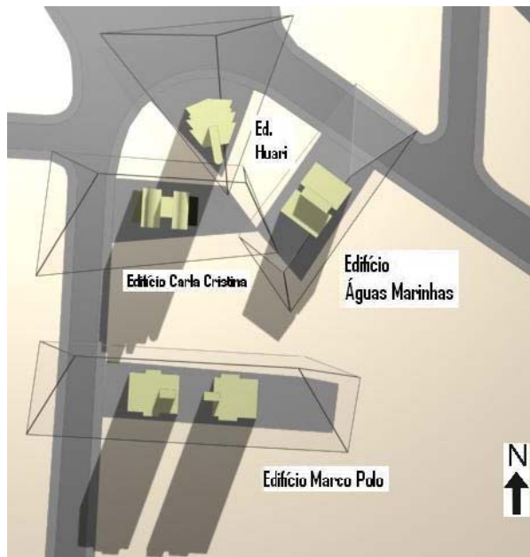
Fig 118. Implantação. Envelopes e sombras. 21 junho, 11:00 h
