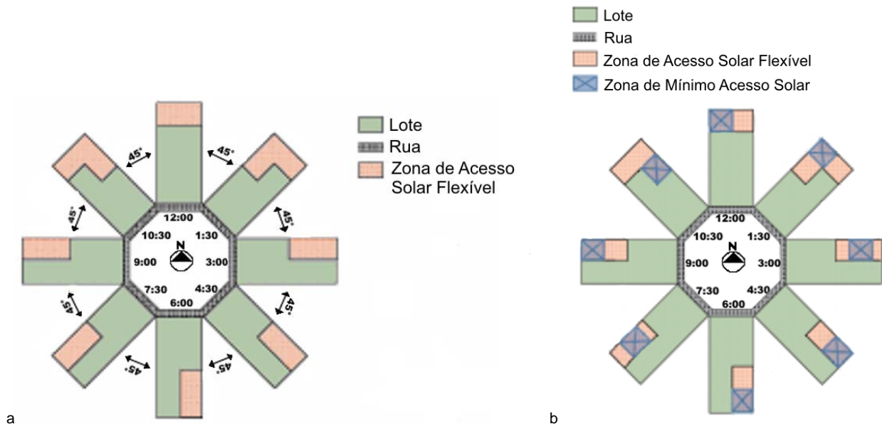
Fig. 30. Lotes com a Zona Flexível de Acesso Solar e com a Zona Mínima de Acesso Solar. Fonte: Seda, 1998
