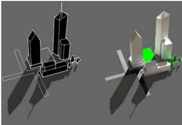
Fig. 91. Imagem computadorizada 3D das projeções de sombras pelo Ecotec e Radiance. Fonte: Square One. Fig. 92. Imagem criada de uma janela solar. Ecotec. Fonte: Square One.
