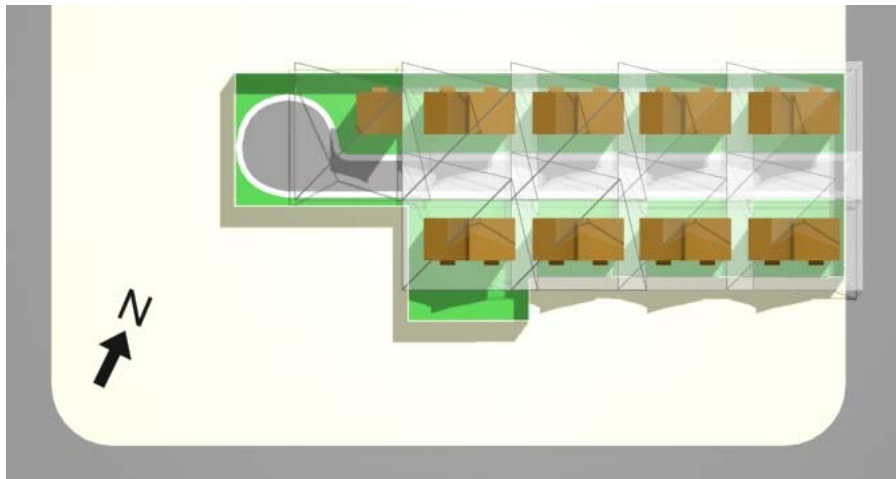
Fig. 100. Implantação das casas, suas sombras e envelopes solares. 21 de junho, 10:00 h.
