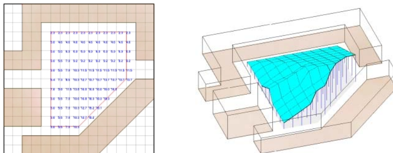
Fig. 43. SER - Envelope de Direito Solar, Fonte: Shaviv e Capeluto, 2001. Adaptado por Daniel B. Pérez, 2006.
