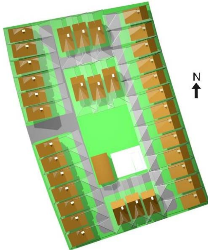
Fig. 110. Implantação das edificações, suas sombras e envelopes solares. 21 de junho. 15:00 h.
