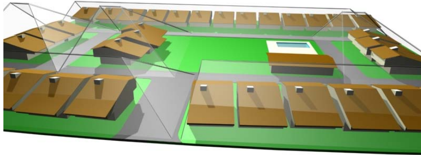
Fig. 115. Vista em 3d. 21 de junho. 9:00 h. Envelopes solares para agrupamento de residências.
