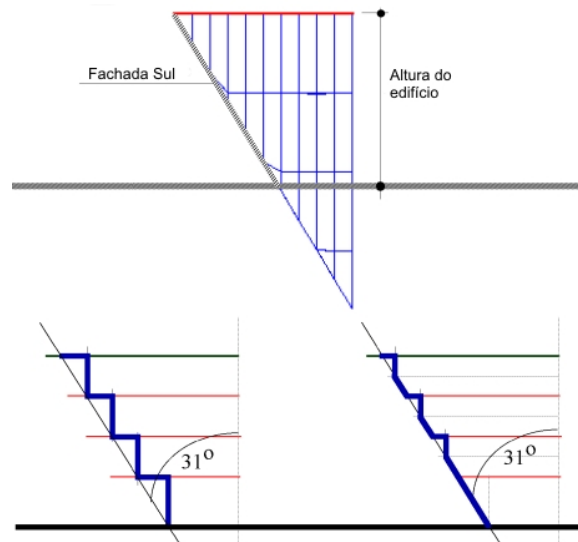
Fig. 55. Duas propostas para a fachada sul. Protegendo todo o vão, e a metade do vão à direita. Fonte: Capeluto, 2003.
