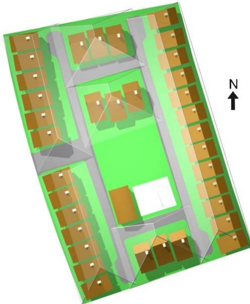
Fig. 116. Implantação das edificações, suas sombras e envelopes solares para agrupamento de residências. 21 de junho. 15:00 h
