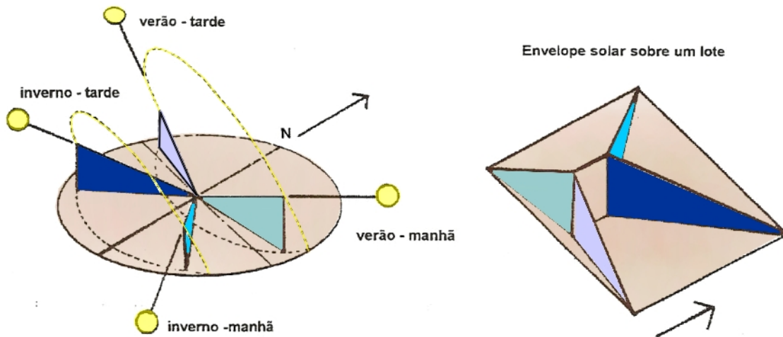
Fig. 34. Construção do envelope solar. Ângulos de altura solar. Fonte: Assis, 2000, adaptado por Daniel B. Pérez, 2006.
