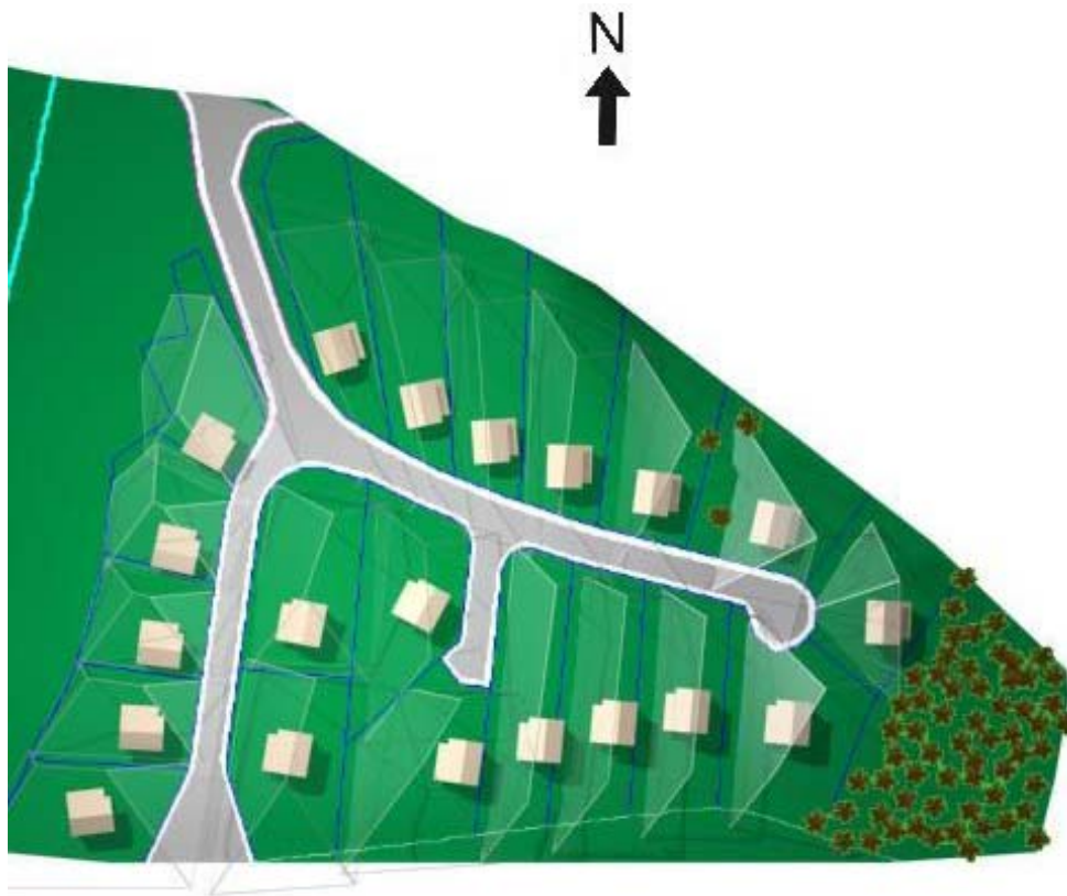
Fig. 98. Implantação geral com as casas, suas sombras e envelopes solares. 21 de junho. 15:00 h.
