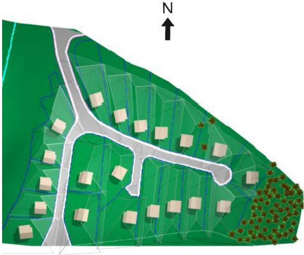
Fig. 95. Implantação geral com as casas, suas sombras e envelopes solares. 21 de junho. 9:00 h.
