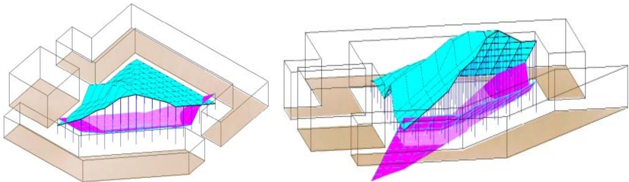
Fig. 45. Volume solar. Fonte Shaviv e Capeluto, 2001. Adaptado por D. Pérez, 2006
