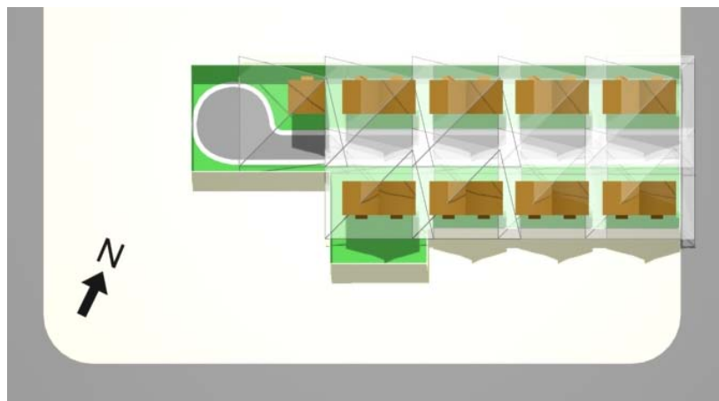
Fig. 102. Implantação das casas, suas sombras e envelopes solares. 21 de junho, 14:00 h
