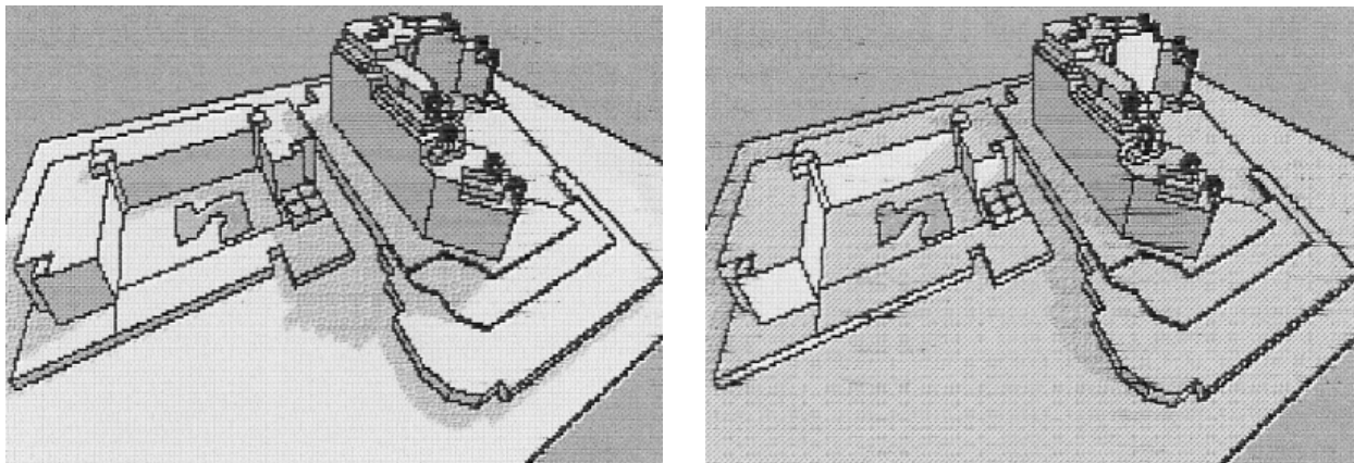
Fig. 51. Avaliação visual e qualitativa de áreas insoladas e sombreadas. A implantação do novo edifício não afeta a piscina e o pátio do edifício existente, nesse horário. Dezembro 11:00 e 15:00 h. Fonte: Shaviv e Yezioro, 1999
