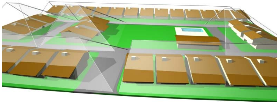
Fig. 117. Vista em 3d. 21 de junho. 15:00 h. Envelopes solares para agrupamento de residências.
