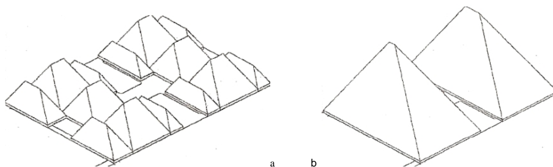
Fig. 76. a) configuração de envelopes solares resultantes do parcelamento do meio da quadra; b) configuração de envelopes solares resultante de um parcelamento com apenas dois grandes lotes. Fonte: Pereira e Nome Silva, 1997
