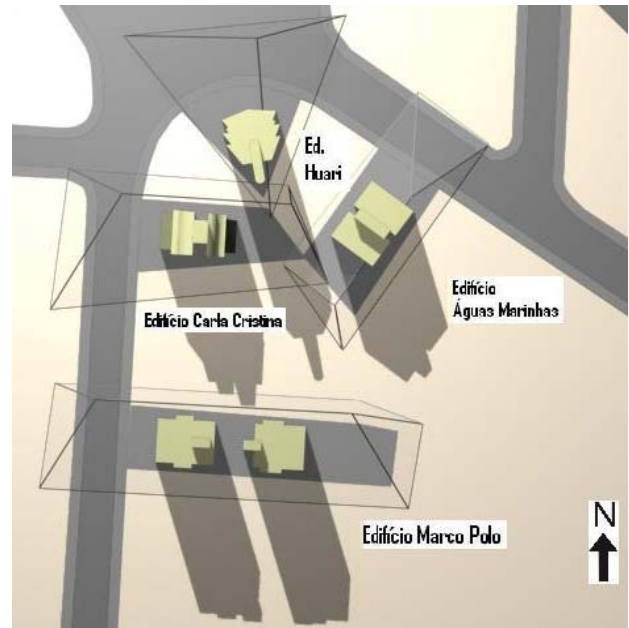
Fig. 119. Implantação. Envelopes e sombras. 21 junho 13:00 h
