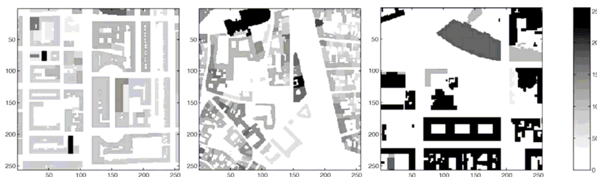
Fig. 70. DEMs de áreas centrais de Londres, Toulouse e Berlin. Alturas representadas em escalas com 256 níveis em cinza.
