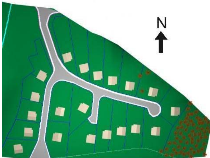
Fig. 84. Implantação Geral.
