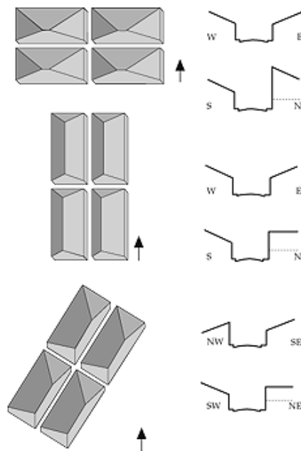
Fig. 41. Volume do envelope varia com a orientação da rua. Fonte: Knowles, 1981.
