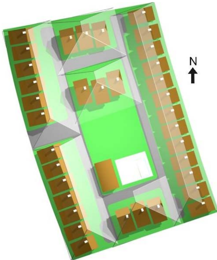
Fig. 114. Implantação das edificações, suas sombras e envelopes solares para agrupamento de residências. 21 de junho. 9:00 h.
