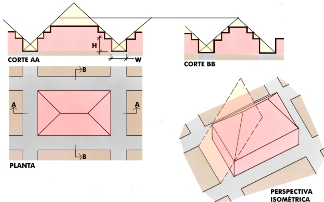
Fig. 42. Envelope de iluminação. Fonte Brown e Dekay, 2004. Adaptado por Daniel B. Pérez, 2006
