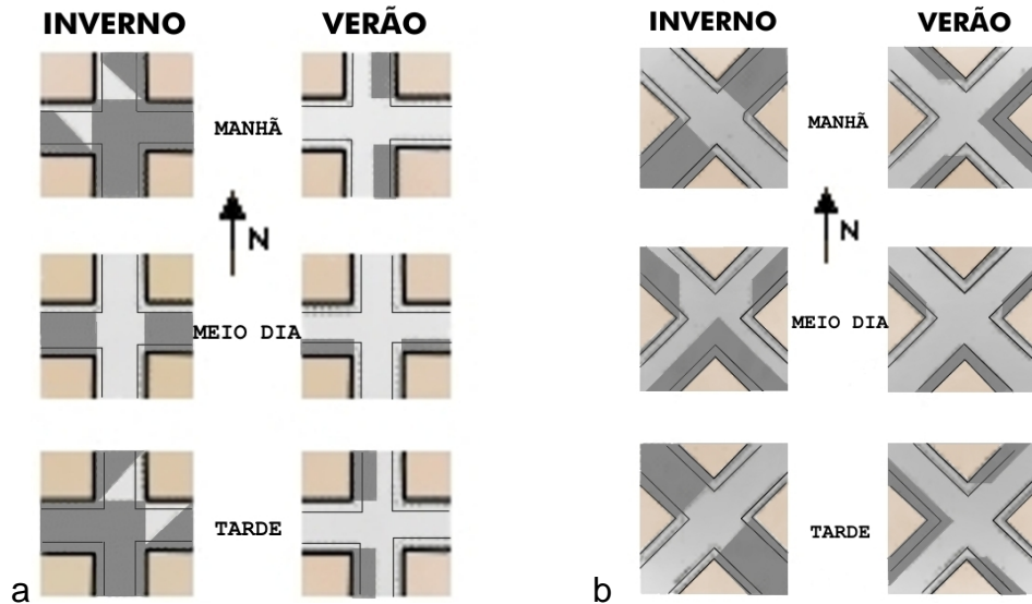
Fig. 40. a) Sombras no cruzamento de ruas orientação norte-sul e b) Sombras no cruzamento de ruas orientadas a 45° do norte Fonte: Knowles (1981) adaptado por Daniel B. Pérez, 2006.
