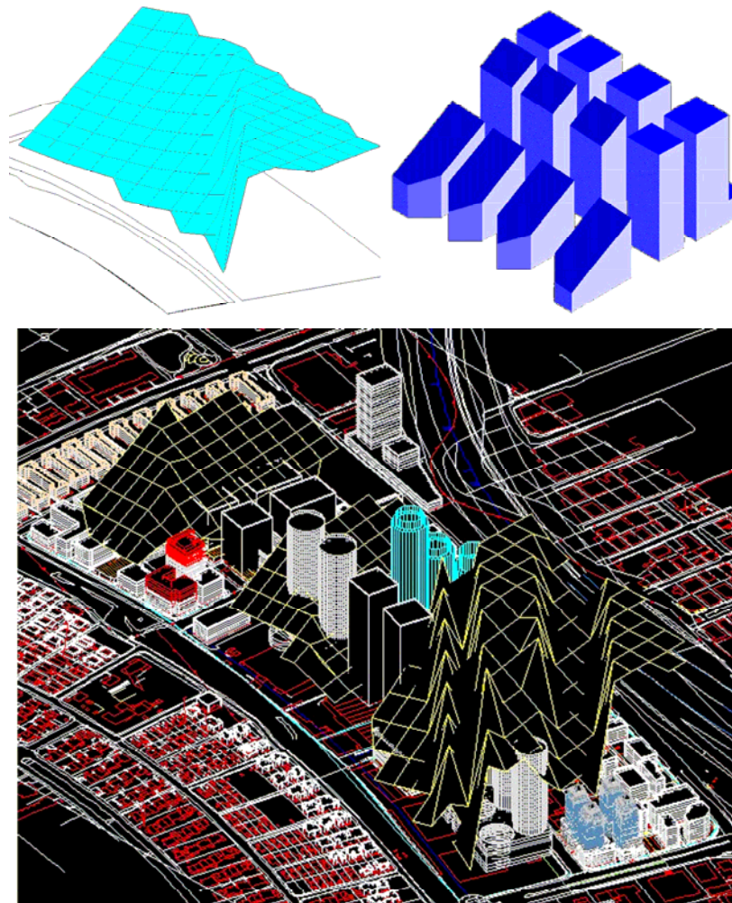
Fig. 58. O envelope solar aceito para garantir os direitos ao sol. Fonte: Yezioro et al, 2001.
