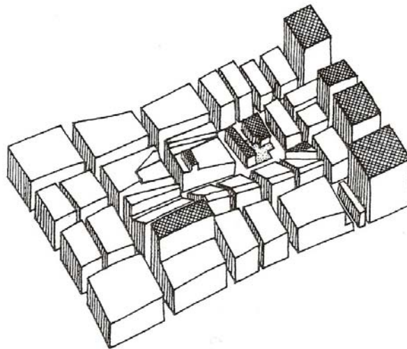
Fig. 38. Variante do envelope solar usado para desenvolver controles de altura em torno do play-ground chinês em São Francisco, Califórnia. Fonte: Brown & Dekay (2004).
