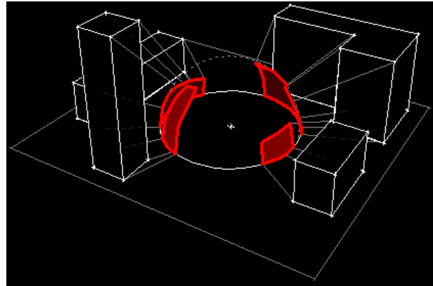
Fig. 91. Imagem computadorizada 3D das projeções de sombras pelo Ecotec e Radiance. Fonte: Square One. Fig. 92. Imagem criada de uma janela solar. Ecotec. Fonte: Square One.
