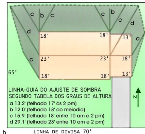
Fig. 26. a) Casa para ser analisada e b) Análise simples de sombras para uma casa. Fonte: Solar Access Guide or Solar Shadow Analysis, 2000. www.ci.boulder.co.us/buildingservices . Acesso em: 07/abr/2007. Adaptação: Daniel B. Pérez, 2006
