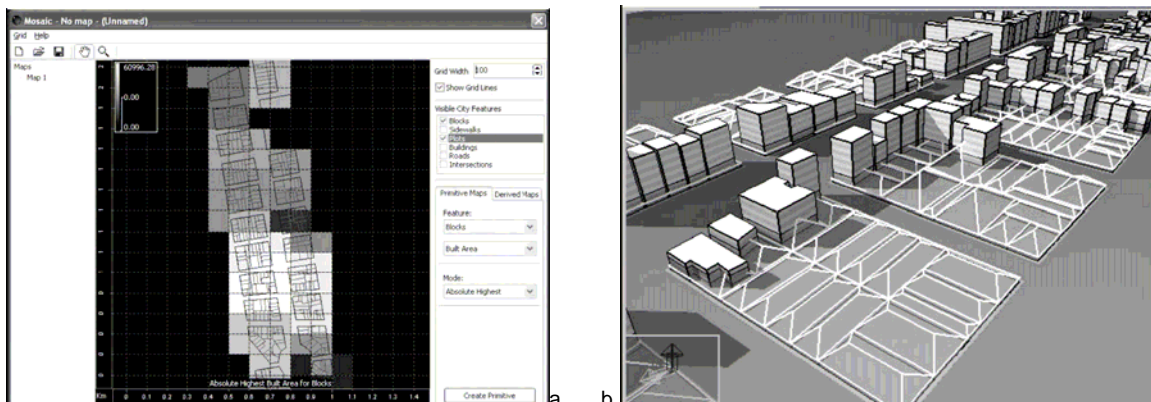
Fig. 79 a) Modelo de avaliação do Cityzoom; b) Vista em 3d com envelopes solares superpostos. Fonte: Grazziotin et al. 2004
