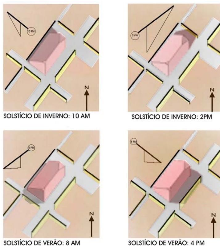
Fig. 32. Horários de corte. Fonte: Kensek & Knowles, 1995, adaptado por Daniel B. Pérez, 2006.
