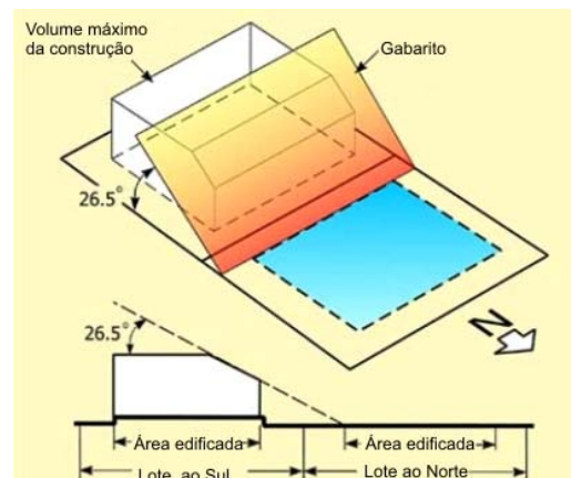
Fig. 61. Plano inclinado. Fonte: Pearlmutter, 2000
