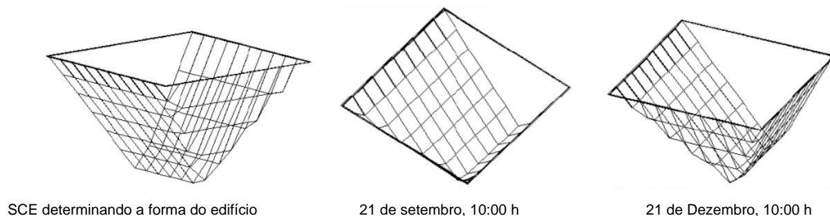
Fig. 52. SCE gera auto-sombreamento de maio a set. das 10:00 às 14:00 h. Avaliação visual do sol às 10:00 h, em 21 de set., a cobertura sombreada as paredes e, em dezembro, às 10:00 h, a fachada sul exposta ao sol. Fonte: Capeluto, 2003.
