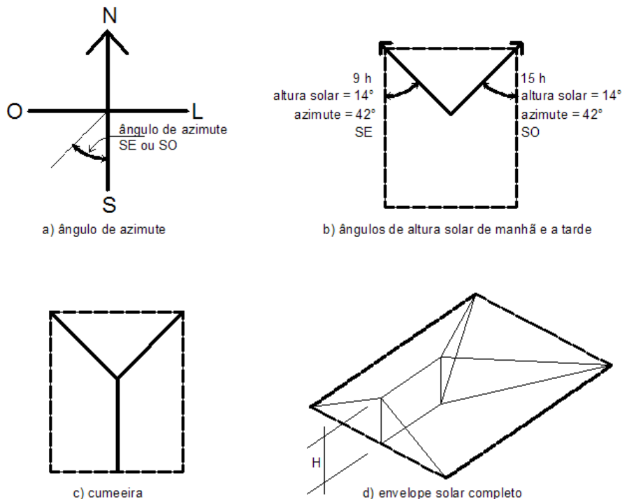
Fig. 35. Construção do envelope solar. Fonte: Brown & Dekay, 2004. Adaptado por D. Pérez, 2007
