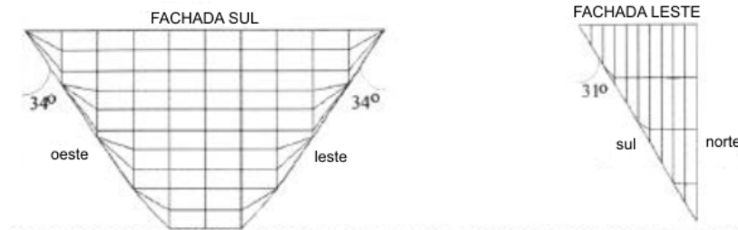
Fig. 53. Fachada sul e fachada leste. Fonte: Capeluto, 2003
