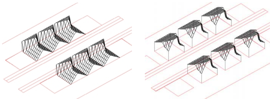
Fig. 48. Acesso solar para todas as fachadas. Fonte: Shaviv e Capeluto, 2001
