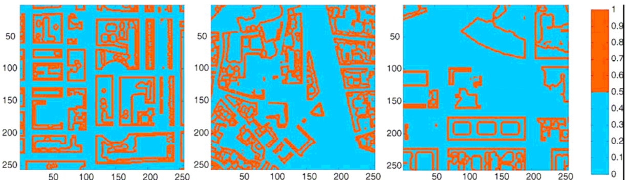
Fig. 71. Zonas passivas (6 m para dentro das fachadas) para Londres, Toulouse e Berlin. Fonte: Steemers et al., 2005
