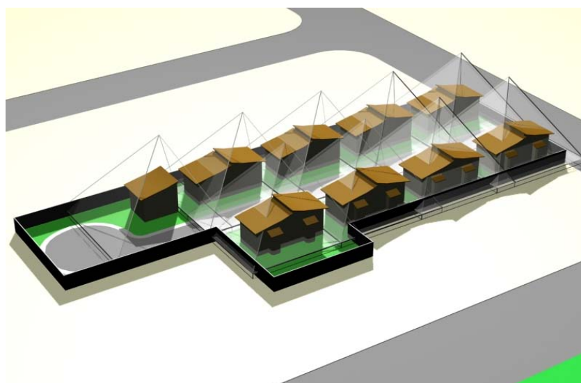
Fig. 101 Vista em 3d. 21 de junho, 10:00 h.
