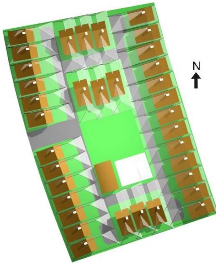
Fig. 106. Implantação das edificações, suas sombras e envelopes solares. 21 de junho. 9:00 h.
