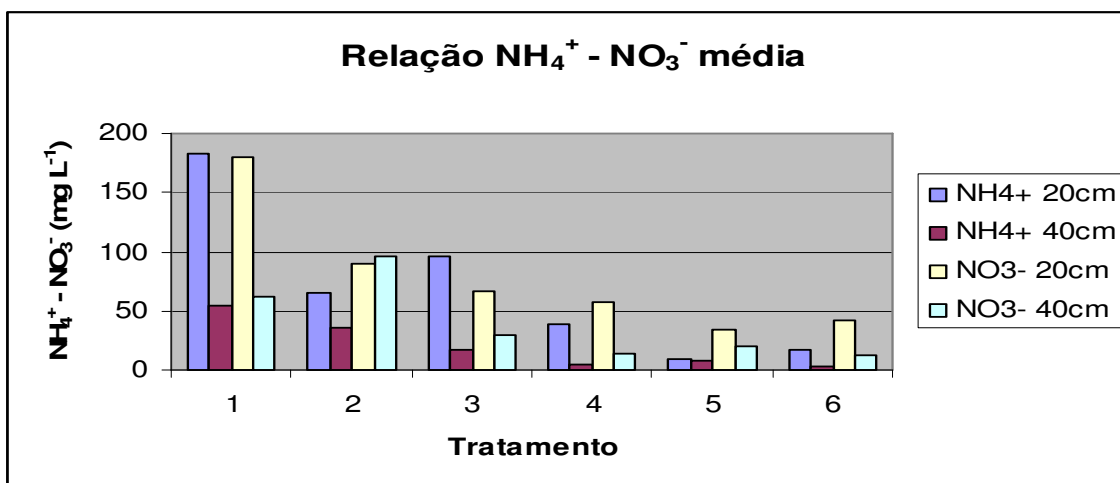
Figura 19. Comparação entre os teores de amônio ( \text{NH}_4^+ ) e nitrato ( \text{NO}_3^- ) na solução do solo, de acordo com os tratamentos e com as profundidades de extração da solução.
