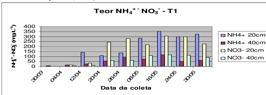
Figura 13. Teores de amônio ( \text{NH}_4^+ ) e nitrato ( \text{NO}_3^- ) na solução do solo, nas profundidades de 20 e 40cm do tratamento 1 (100% N mineral) no decorrer do experimento.
