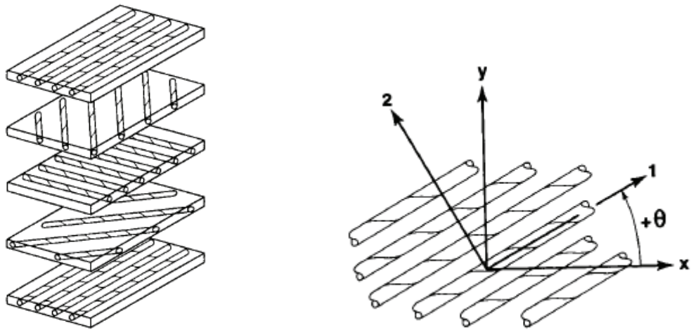
Figura 2.2: Lâminas formando o laminado e ângulo entre eixo principal do material 1-2 e sistema x-y do laminado (Jones,1999).
