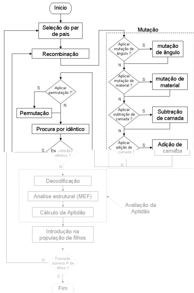
Figura 3.2: Fluxograma da geração da população de filhos
