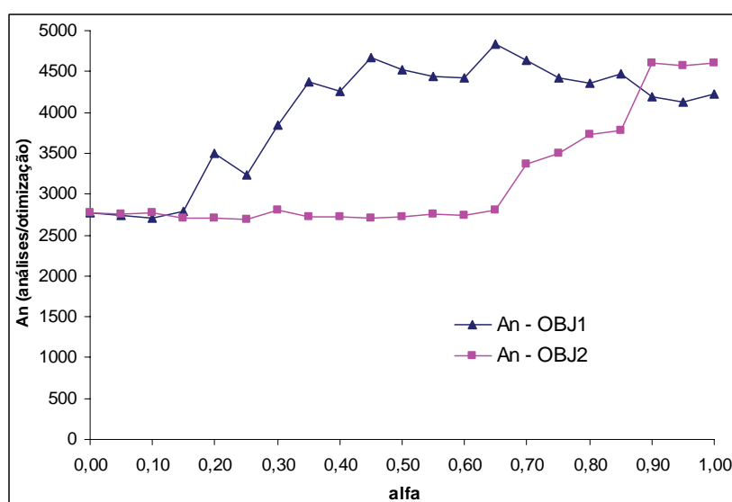
Figura 4.25: Número médio de análises requeridas nas otimizações para cada valor de
