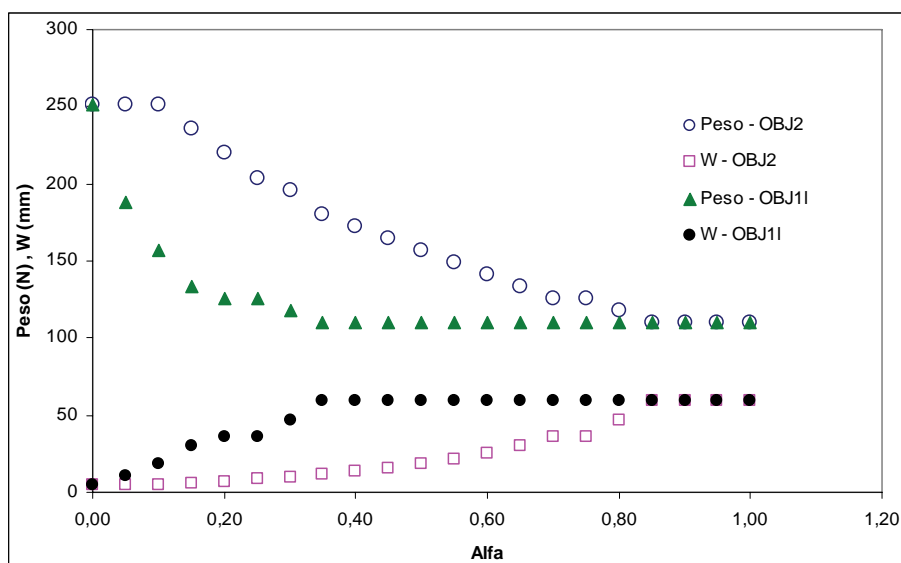
Figura 4.24: Evolução de peso e de deslocamento máximo das soluções ótimas obtidas para consecutivos valores de
