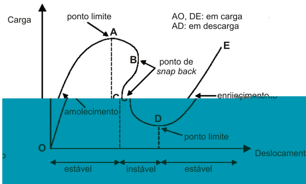
Figura 2.9: Características de um sistema não-linear (Yang e Shieh, 1990).
