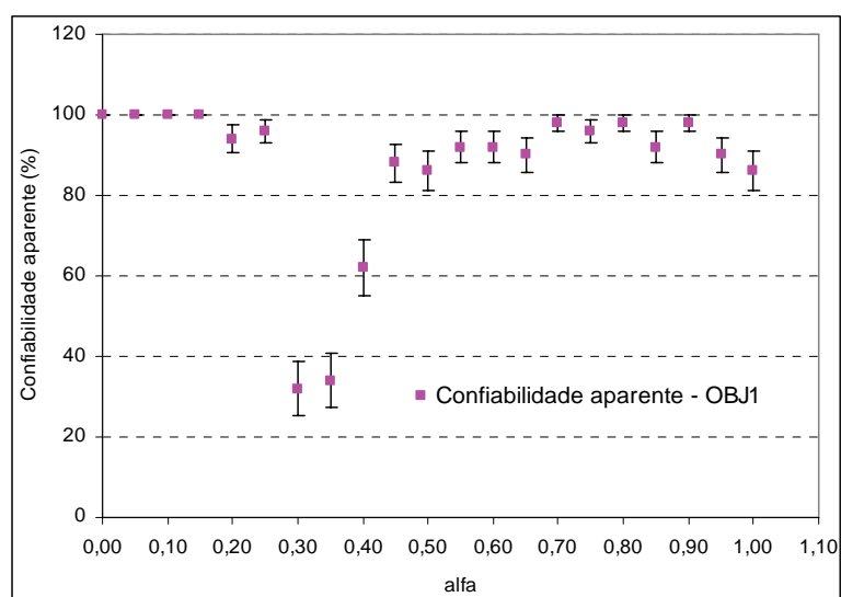
Figura 4.26: Confiabilidade aparente para OBJ1
