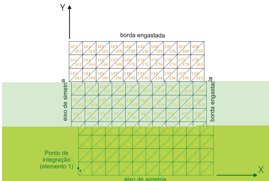
Figura 4.17: Malha de elementos finitos e indicação do ponto de integração onde são comparadas as tensões calculadas
