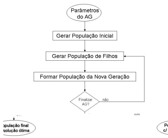
Figura 3.1: Fluxograma básico do AG
