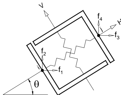
Figura 3.7.1.3- Elemento de ligação, forças nodais.
