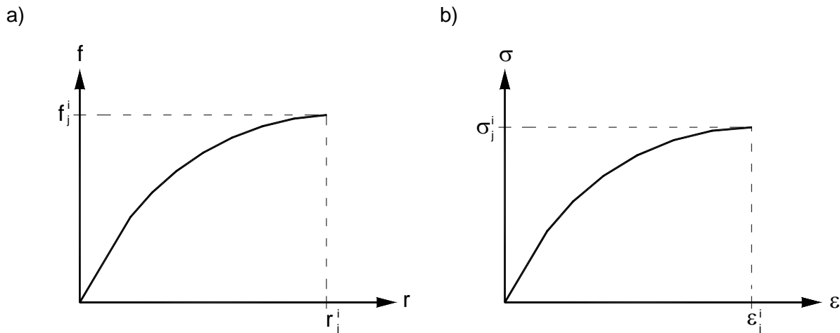
Figura 3.3.1- a) Curva carregamento-deslocamento ( f \times r ); b) Curva tensão-deformação ( \sigma \times \varepsilon ).
