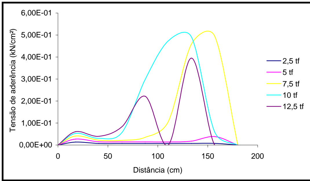
Figura 6.2.16- Gráfico: distribuição da tensão de aderência entre o aço e o concreto – ANLEC 2007 (a).
