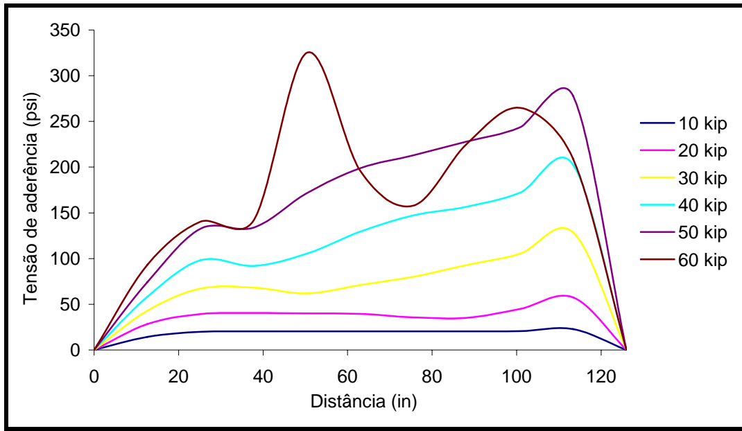
Figura 6.2.3- Gráfico: distribuição da tensão de aderência entre o aço e o concreto – ANLEC 2007 (a).
