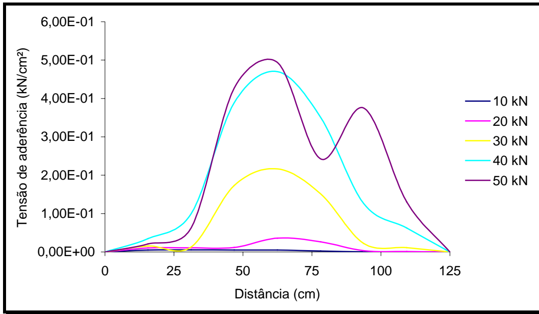
Figura 6.2.25- Gráfico: distribuição da tensão de aderência entre o aço e o concreto – ANLEC 2007 (a).
