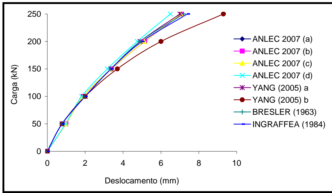
Figura 6.2.20- Gráfico: carga x deslocamento vertical no centro do vão.
