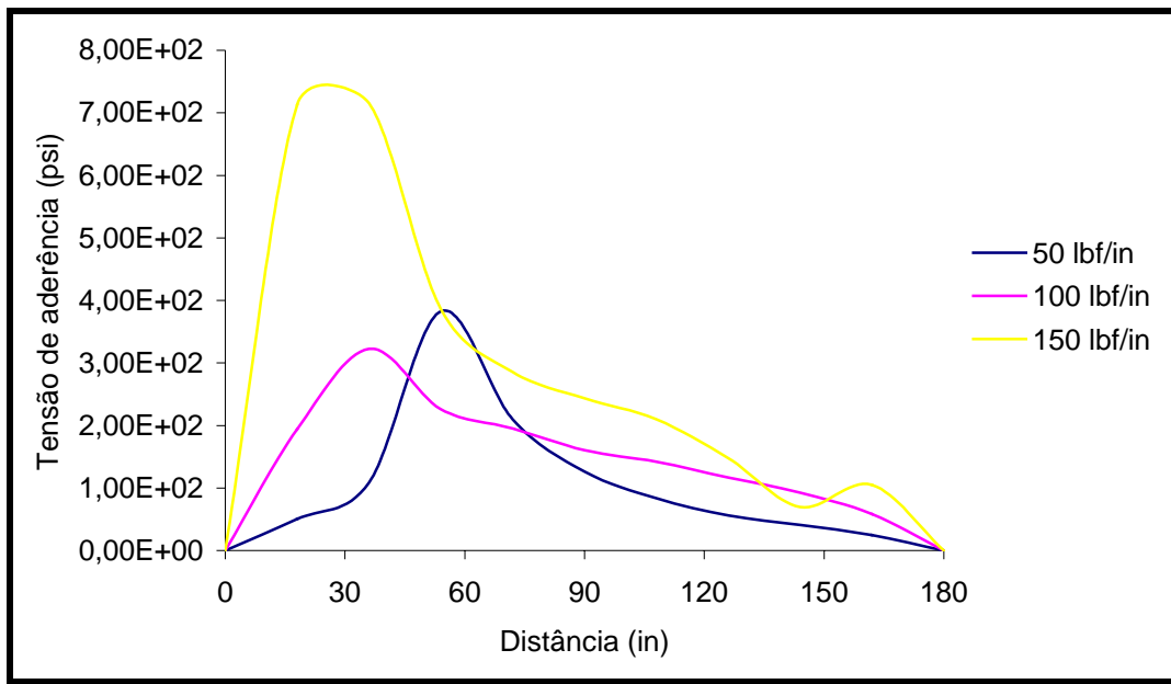
Figura 6.2.34- Gráfico: distribuição da tensão de aderência entre o aço e o concreto – ANLEC 2007 (a).
