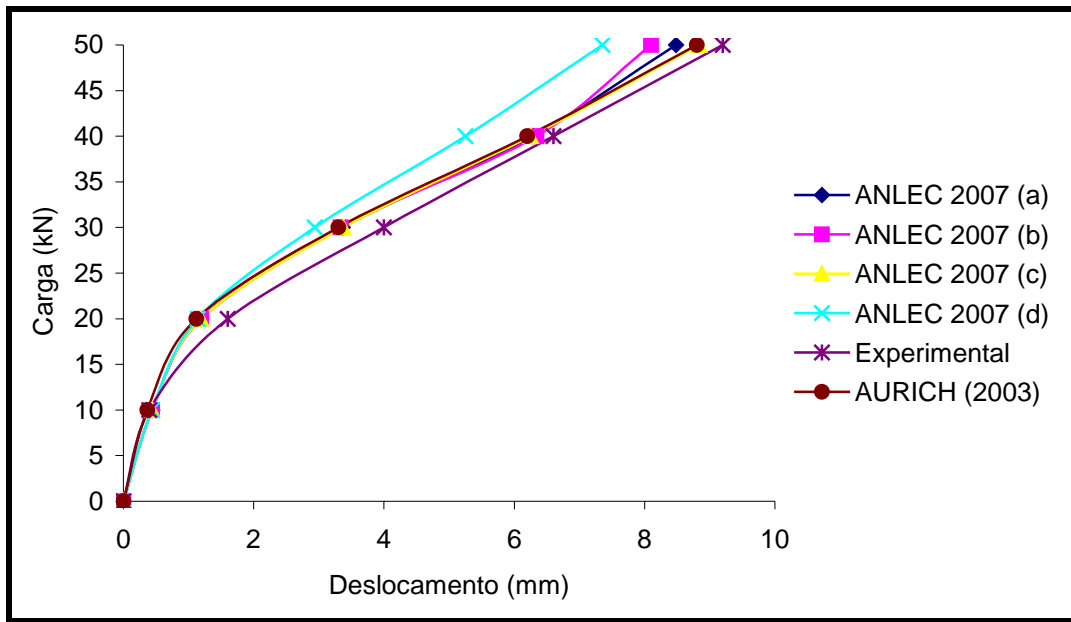
Figura 6.2.24- Gráfico: carga x deslocamento vertical no centro do vão.
