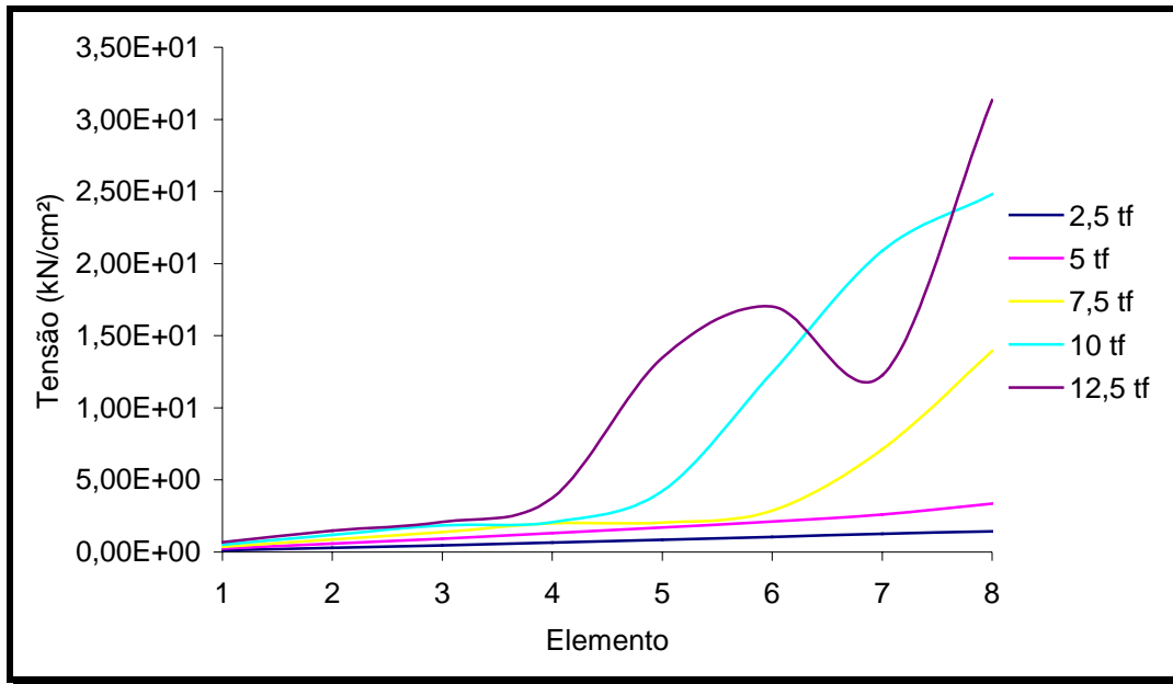
Figura 6.2.17- Gráfico: distribuição da tensão no centro dos elementos da barra de aço – ANLEC 2007 (a) .
