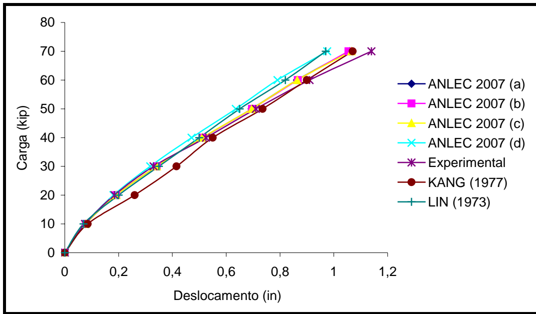
Figura 6.2.2- Gráfico: carga x deslocamento vertical no centro do vão.
