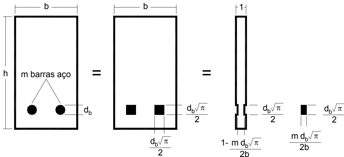
Figura 4.2.3- Transformação da viga tridimensional para o modelo numérico plano.
