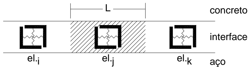
Figura 3.7.1.6- Área de influência dos elementos de ligação.
