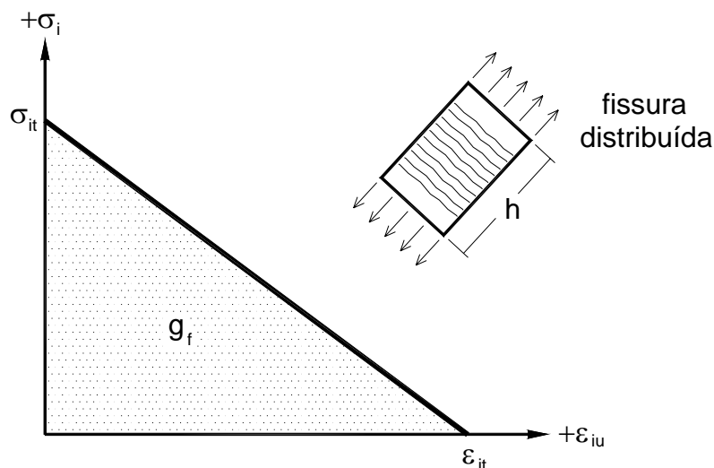
Figura 3.4.5.3- Curva tensão-deformação para o elemento com fissuras distribuídas.
