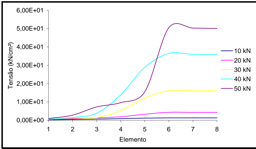
Figura 6.2.26- Gráfico: distribuição da tensão no centro dos elementos da barra de aço – ANLEC 2007 (a) .
