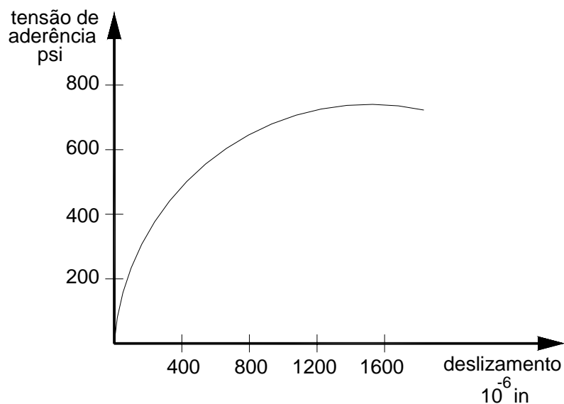
Figura 3.6.2- Curva tensão de aderência x deslizamento (fonte: MIRZA, 1979 ).
