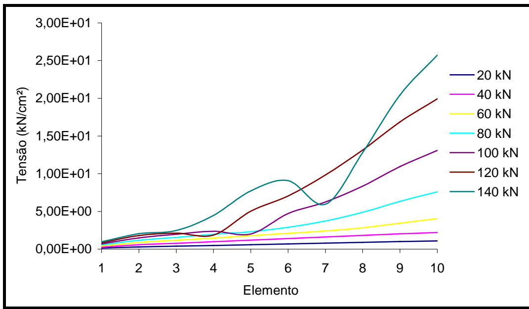
Figura 6.2.9- Gráfico: distribuição da tensão no centro dos elementos da barra de aço (aderência perfeita).
