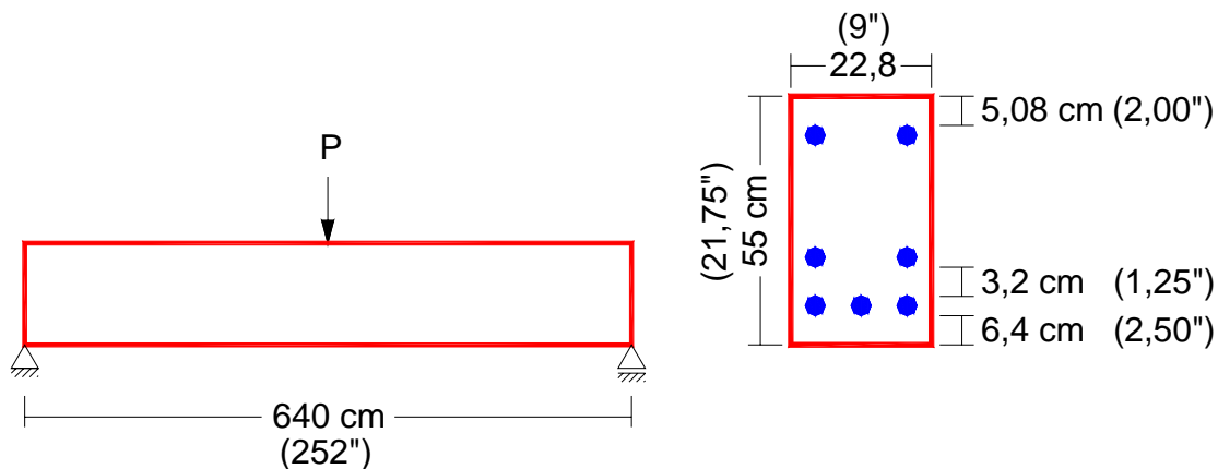
Figura 6.2.1- Conformação geométrica da viga simétrica.
