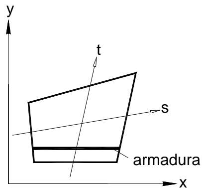
Figura 3.5.1.2- Representação embutida da armadura.
