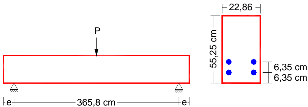
Figura 6.2.10- Conformação geométrica da viga simétrica.
