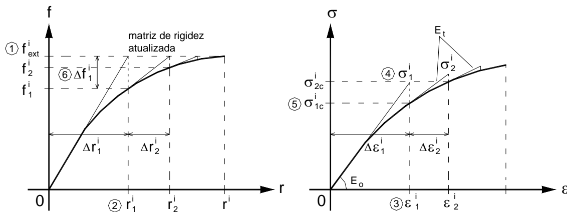
Figura 3.3.4- Método da rigidez tangente para análise não-linear.
