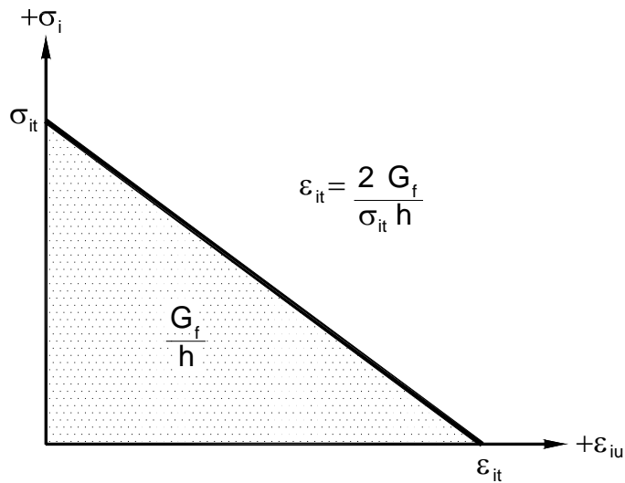
Figura 3.4.5.5- Curva tensão-deformação em função da energia de fratura.
