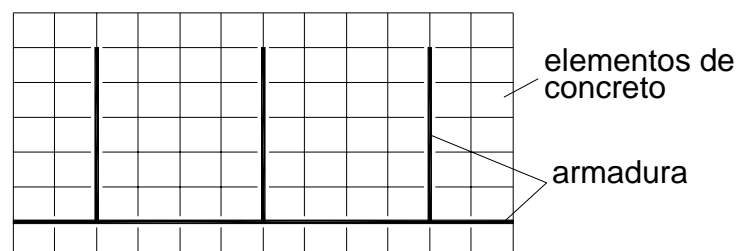
Figura 3.5.1.3- Representação discreta da armadura.
