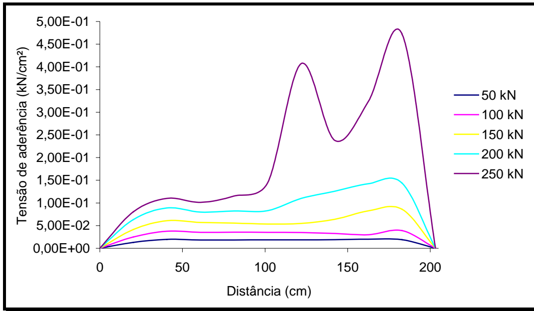
Figura 6.2.12- Gráfico: distribuição da tensão de aderência entre o aço e o concreto – ANLEC 2007 (a).
