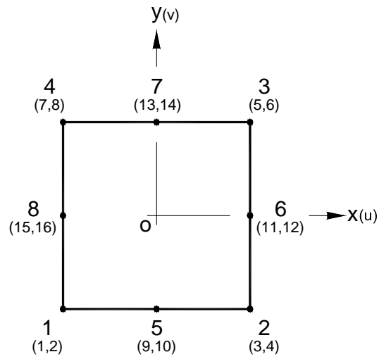
Figura 3.2.2.1- Elemento finito retangular ( LSR ).
