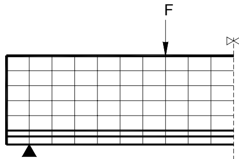
Figura 4.2.2- Consideração da simetria da viga.
