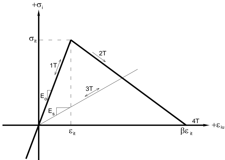
Figura 3.4.4.2- Condições de descarregamento e recarregamento para diferentes estados do concreto tracionado.
