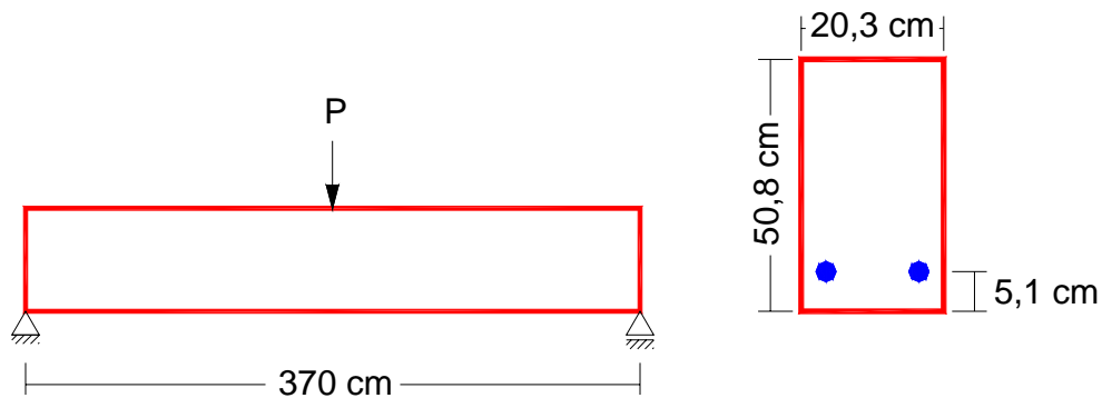
Figura 6.2.5- Conformação geométrica da viga simétrica.
