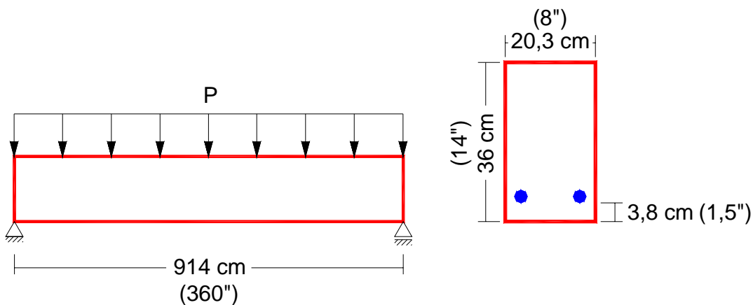
Figura 6.2.32- Conformação geométrica da viga simétrica.
