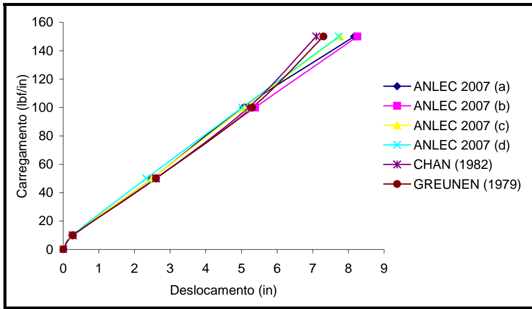
Figura 6.2.33- Gráfico: carga x deslocamento vertical no centro do vão.
