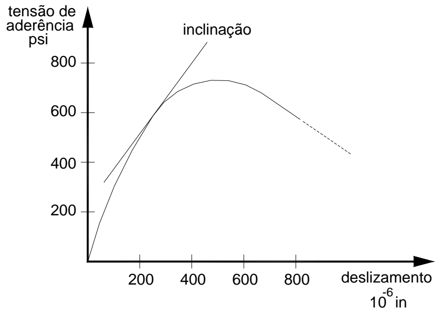
Figura 3.7.1.4- Inclinação da curva tensão de aderência x deslizamento.
