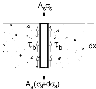
Figura 1.3.2- Obtenção da tensão de aderência pelo equilíbrio de forças.
