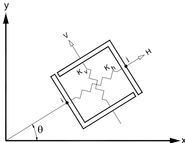
Figura 3.7.1.1- Elemento de ligação (fonte: NGO, 1967 ).
