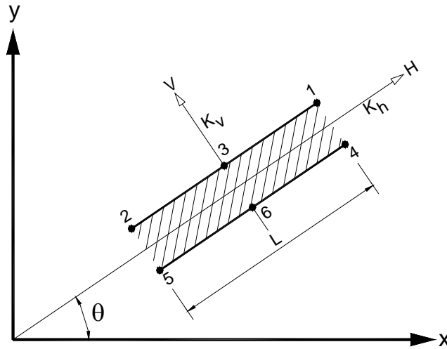
Figura 3.7.2.1- Elemento de Interface.
