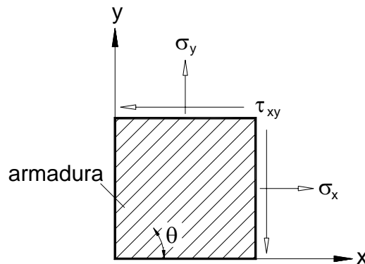
Figura 3.5.1.1- Representação distribuída da armadura.
