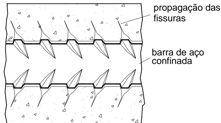
Figura 2.2.5- Propagação do cone formado por fissuras ao redor da barra de aço.
