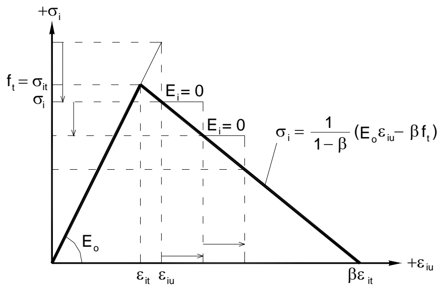
Figura 3.4.3.5- Curva tensão x deformação uniaxial equivalente para o concreto tracionado acima da máxima resistência à tração.
