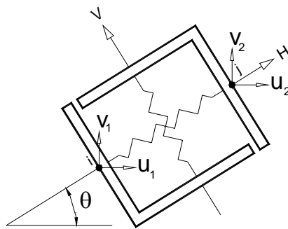
Figura 3.7.1.2- Elemento de ligação, deslocamentos nodais.
