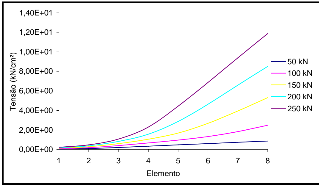
Figura 6.2.22- Gráfico: distribuição da tensão no centro dos elementos da barra de aço – ANLEC 2007 (a) .
