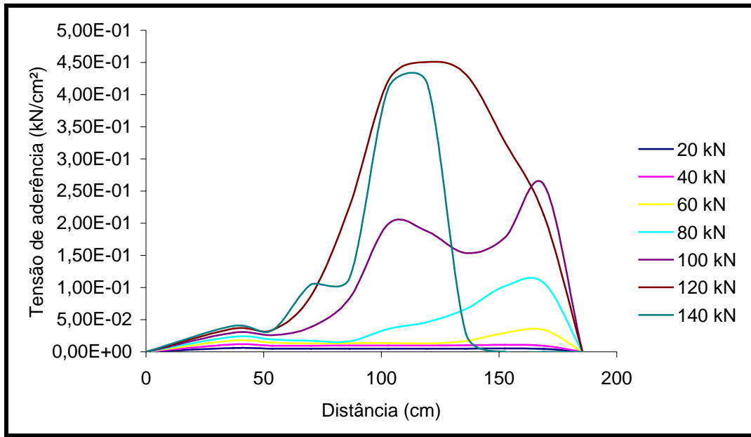
Figura 6.2.7- Gráfico: distribuição da tensão de aderência entre o aço e o concreto – ANLEC 2007 (a).
