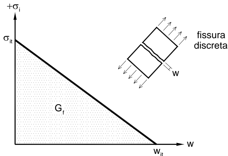
Figura 3.4.5.4- Curva tensão-abertura da fissura.
