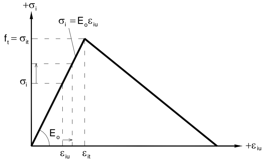
Figura 3.4.3.4- Curva tensão x deformação uniaxial equivalente para o concreto tracionado abaixo da máxima resistência à tração.
