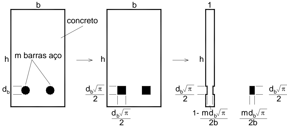
Figura 3.7.1.8- Seção modificada (unitária) de um elemento de concreto armado.
