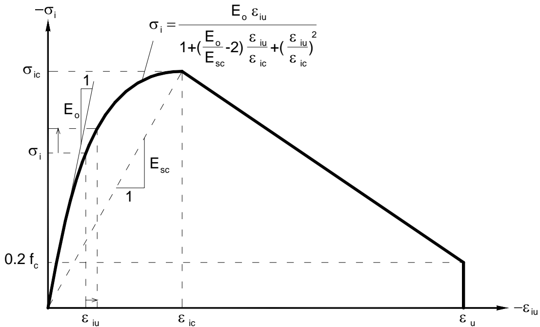
Figura 3.4.3.1- Curva tensão-deformação uniaxial equivalente para o concreto comprimido abaixo da máxima resistência à compressão (fonte: DARWIN, 1974 ).
