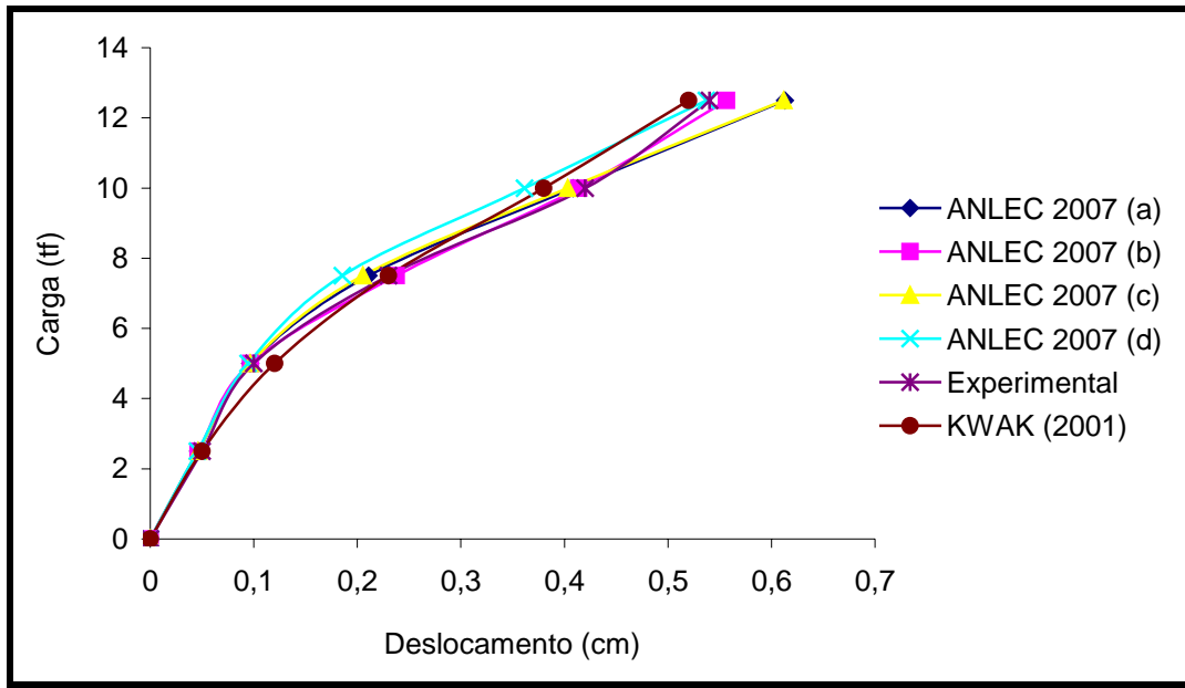
Figura 6.2.15- Gráfico: carga x deslocamento vertical no centro do vão.
