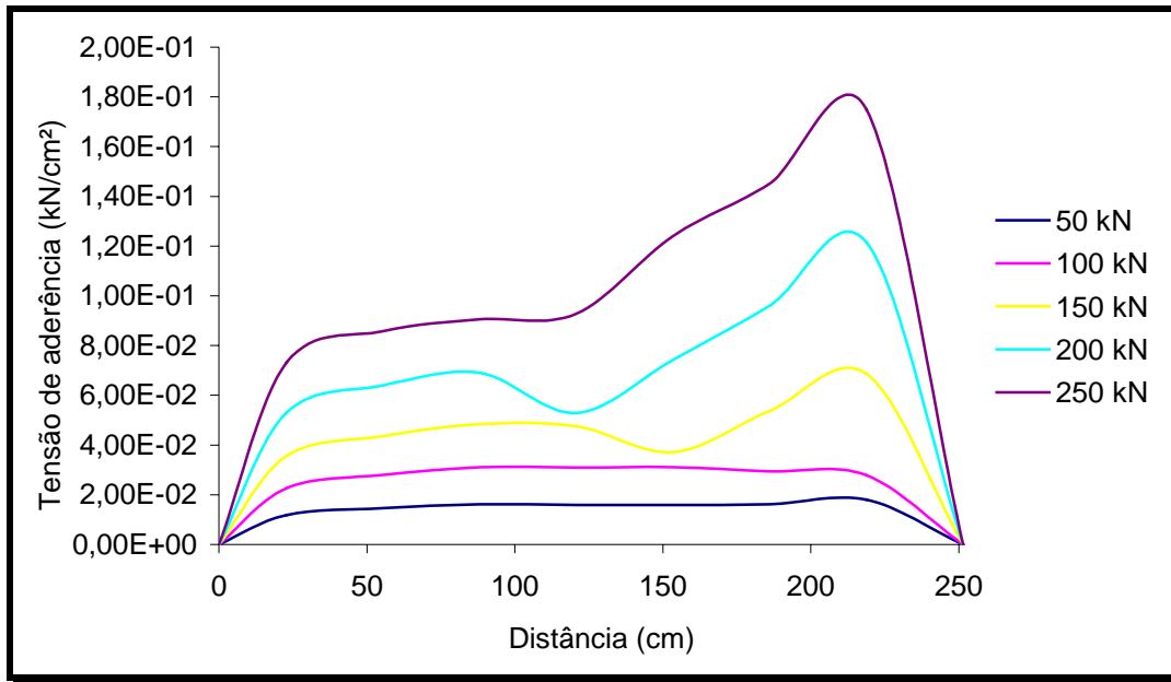
Figura 6.2.21- Gráfico: distribuição da tensão de aderência entre o aço e o concreto – ANLEC 2007 (a).
