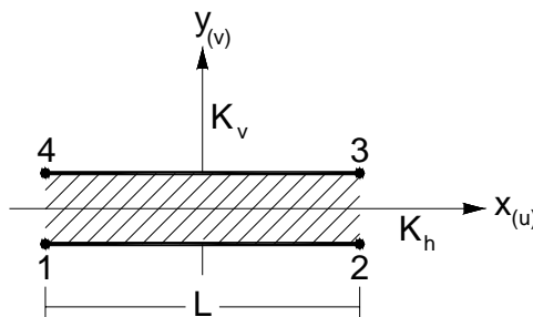
Figura 3.7.2.2- Elemento de Interface linear.
