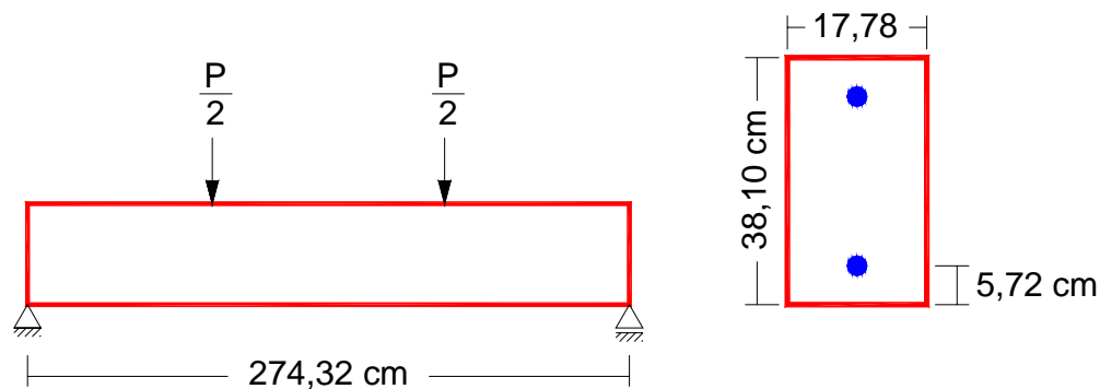
Figura 6.2.27- Conformação geométrica da viga simétrica.
