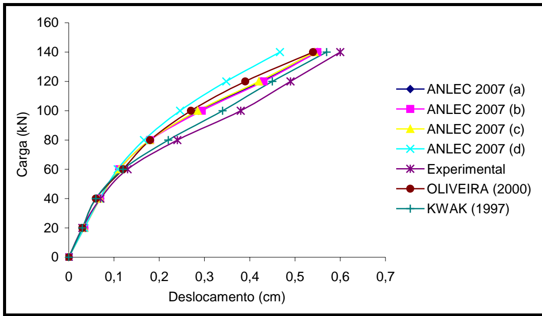
Figura 6.2.6- Gráfico: carga x deslocamento vertical no centro do vão.
