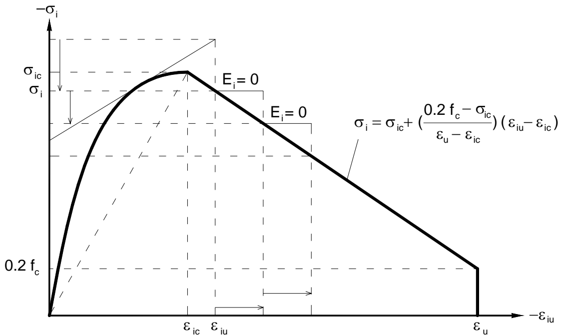
Figura 3.4.3.2- Curva tensão-deformação uniaxial equivalente para o concreto comprimido acima da máxima resistência à compressão (fonte: DARWIN, 1974 ).
