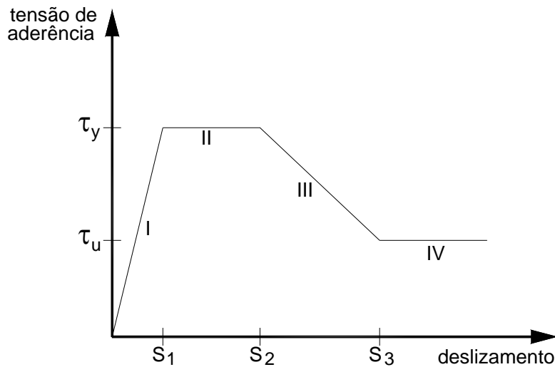
Figura 2.2.4- Relação local da tensão de aderência x deslizamento (fonte: YANKELEVSKY, 1985 ).
