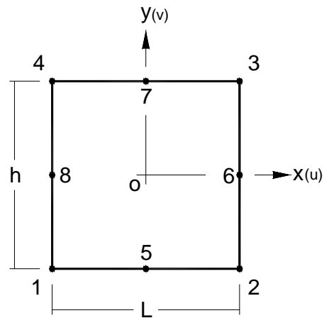
Figura 3.2.2.2- Dimensões dos elementos finitos.
