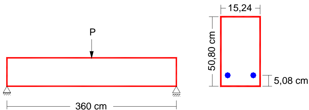
Figura 6.2.14- Conformação geométrica da viga simétrica.
