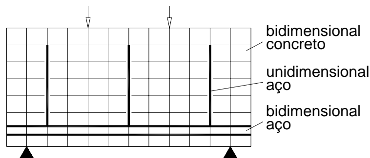
Figura 3.5.1.4- Elementos de representação da armadura.
