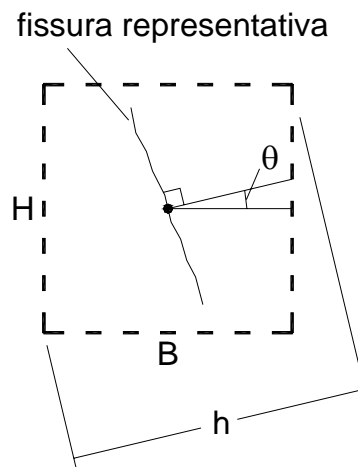
Figura 3.4.5.7- Definição de Comprimento equivalente em função do ângulo de propagação da fissura.
