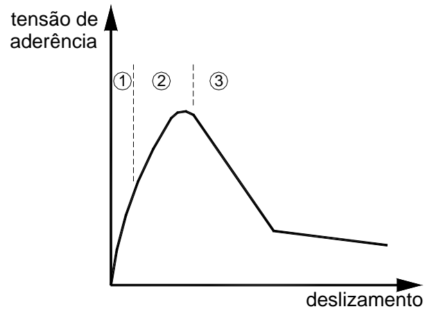
Figura 2.2.6- Estágios decorrentes da propagação das fissuras.
