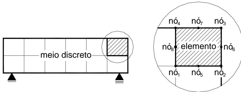
Figura 3.2.1.2- Meio discreto, divisão em elementos finitos (malha).
