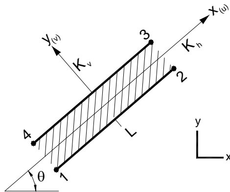
Figura 3.7.2.3- Elemento de Interface linear no sistema de coordenada global.
