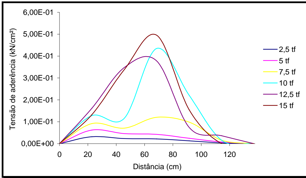
Figura 6.2.29- Gráfico: distribuição da tensão de aderência entre o aço e o concreto – ANLEC 2007 (a).
