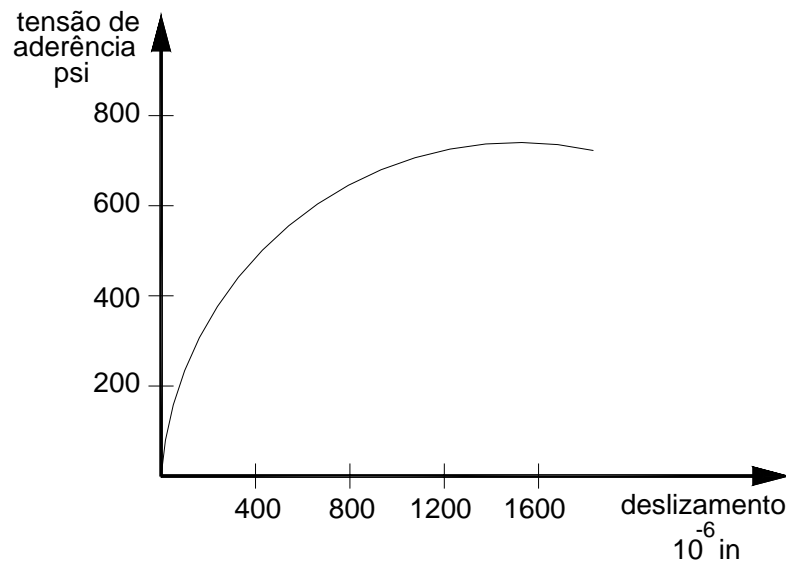
Figura 2.2.3- Curva tensão de aderência x deslizamento (fonte: MIRZA, 1979 ).
