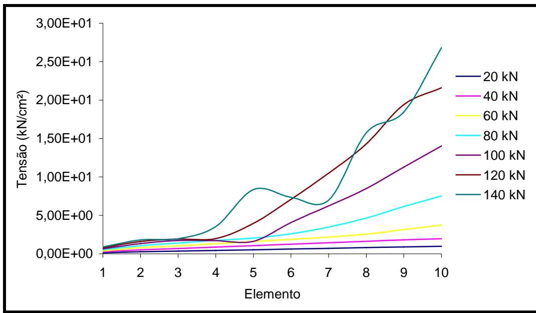
Figura 6.2.8- Gráfico: distribuição da tensão no centro dos elementos da barra de aço – ANLEC 2007 (a) .
