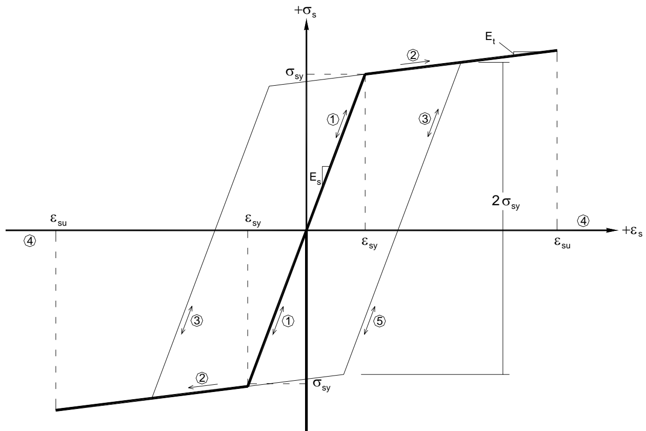
Figura 3.5.2.1- Comportamento do elemento de aço na compressão e na tração.
