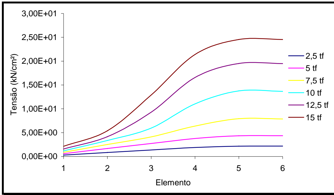
Figura 6.2.31- Gráfico: distribuição da tensão no centro dos elementos da barra de aço (aderência perfeita).
