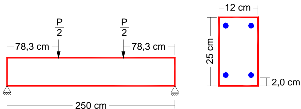
Figura 6.2.23- Conformação geométrica da viga simétrica.
