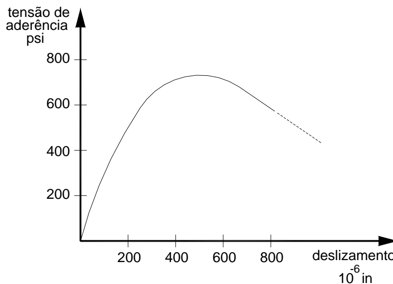
Figura 3.6.1- Curva tensão de aderência x deslizamento (fonte: NILSON, 1968 ).
