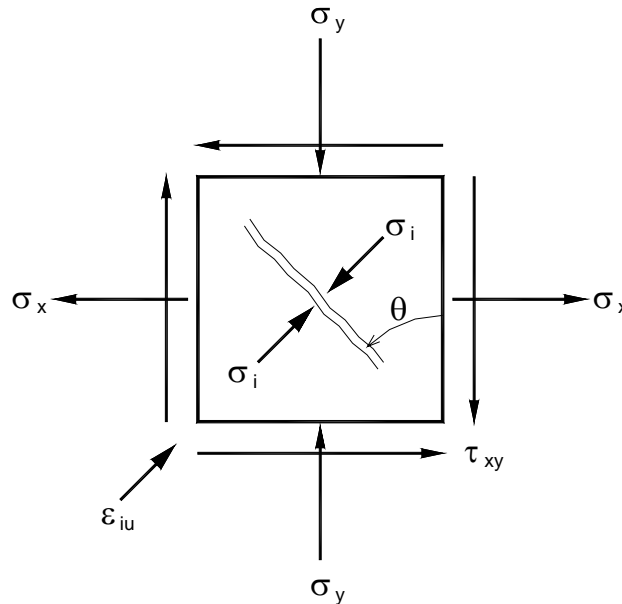
Figura 3.4.3.3- Ângulo entre o sistema de coordenada local e o sistema de coordenada global para o concreto comprimido.
