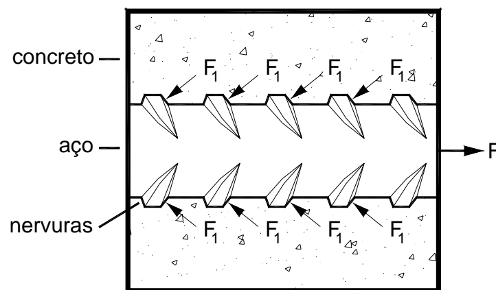
Figura 1.3.1- Interação mecânica entre as nervuras da barra de aço e o concreto ao redor.
