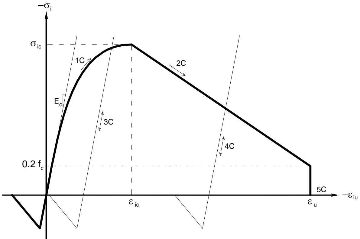
Figura 3.4.4.1- Condições de descarregamento e recarregamento para diferentes estados do concreto comprimido (fonte: GREUNEN, 1979 ).
