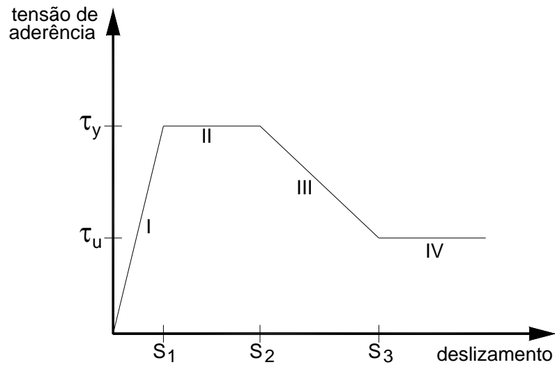
Figura 3.6.3- Curva tensão de aderência x deslizamento (fonte: YANKOLEVSKY, 1985 ).
