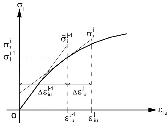
Figura 3.4.2.1- Curva tensão-deformação uniaxial equivalente.
