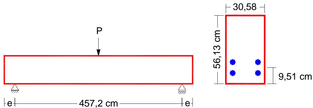
Figura 6.2.19- Conformação geométrica da viga simétrica.
