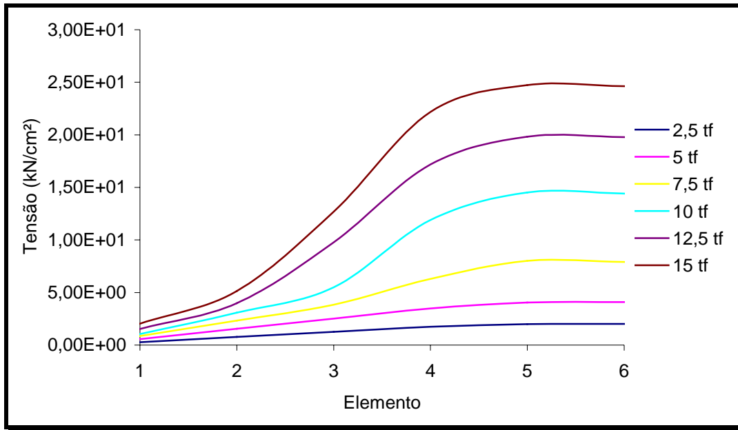
Figura 6.2.30- Gráfico: distribuição da tensão no centro dos elementos da barra de aço – ANLEC 2007 (a) .
