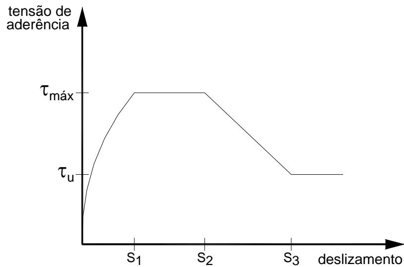
Figura 3.6.4- Curva tensão de aderência x deslizamento (fonte: CEB, 1990 ).
