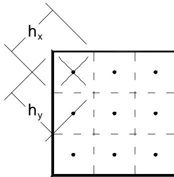
Figura 3.4.5.6- Comprimento equivalente de cada ponto de integração do elemento finito.
