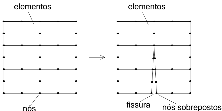
Figura 3.4.5.1- Esquema do modelo de fissuração discreta.
