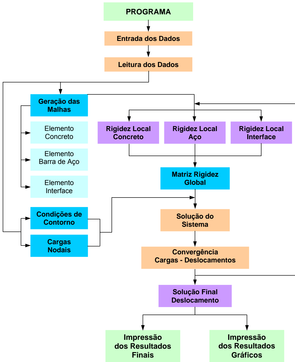
Figura 4.4.1- Fluxograma do programa.
