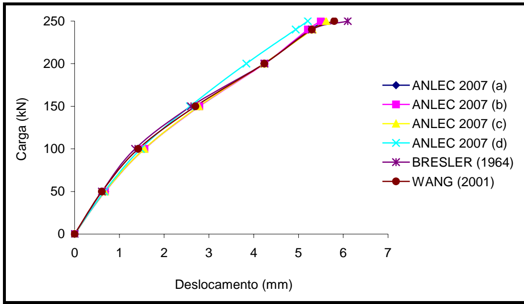
Figura 6.2.11- Gráfico: carga x deslocamento vertical no centro do vão.
