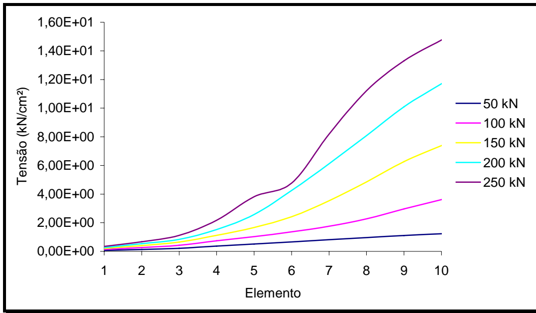
Figura 6.2.13- Gráfico: distribuição da tensão no centro dos elementos da barra de aço – ANLEC 2007 (a) .
