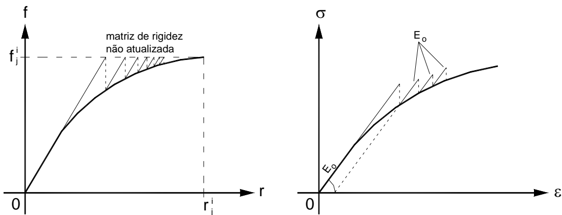
Figura 3.3.2- Método da rigidez inicial para análise não-linear.
