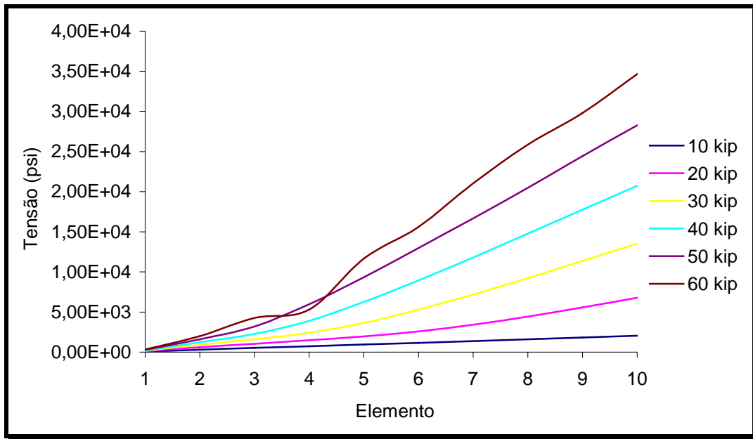
Figura 6.2.4- Gráfico: distribuição da tensão no centro dos elementos da barra de aço – ANLEC 2007 (a) .
