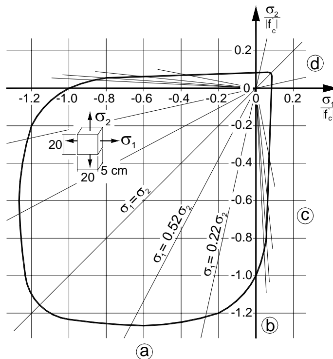
Figura 3.4.6.1- Curva envoltória da resistência biaxial do concreto (KUPFER, 1969).
