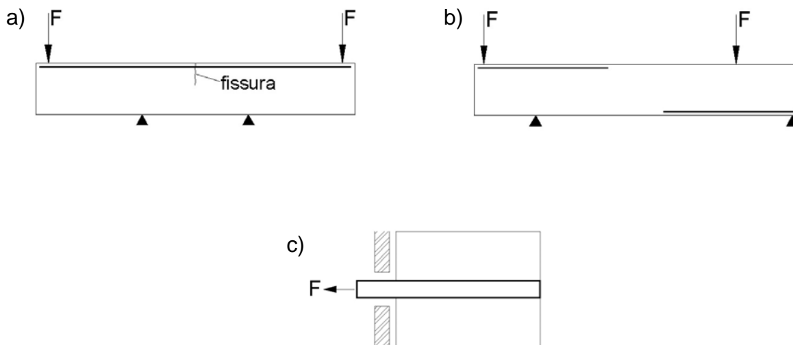
Figura 2.2.1- Representação dos ensaios analisados por PERRY (1966) .
