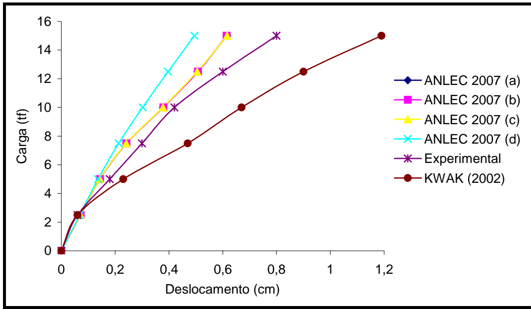
Figura 6.2.28- Gráfico: carga x deslocamento vertical no centro do vão.
