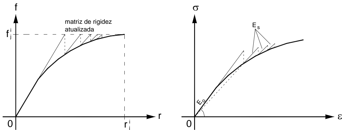
Figura 3.3.3- Método da rigidez secante para análise não-linear.
