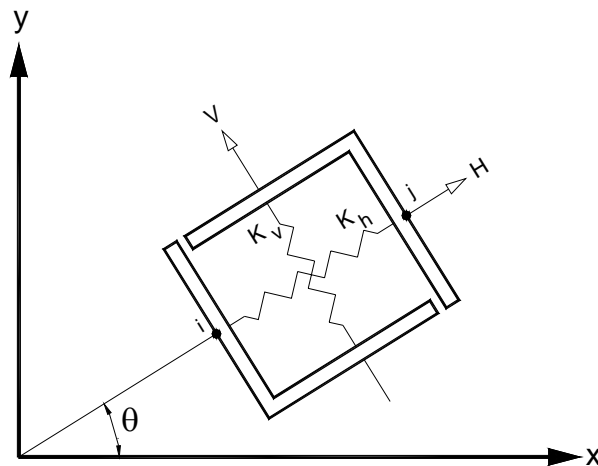
Figura 2.2.2- Elemento de ligação (fonte: NGO, 1967 ).
