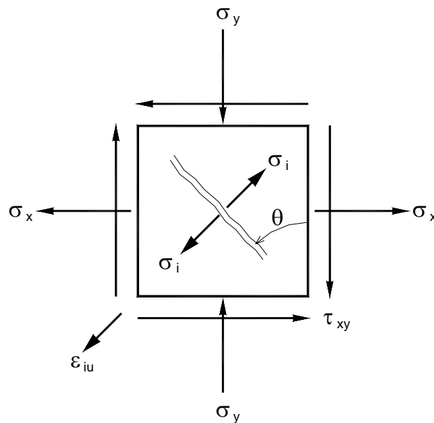
Figura 3.4.3.6- Ângulo entre o sistema de coordenada local e o sistema de coordenada global para o concreto tracionado.
