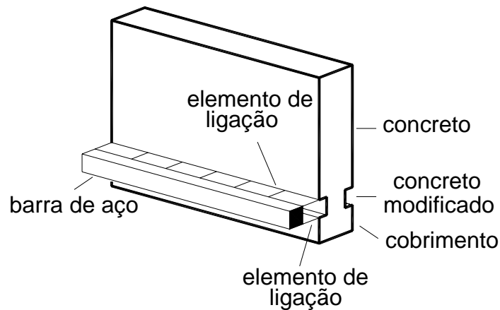
Figura 3.7.1.7- Elemento de ligação: topo e base das barras de aço.
