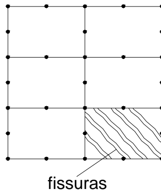
Figura 3.4.5.2- Esquema do modelo de fissuração distribuída.
