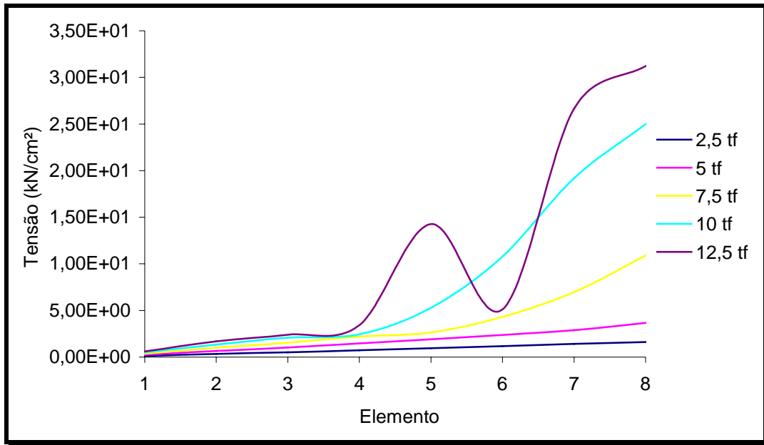
Figura 6.2.18- Gráfico: distribuição da tensão no centro dos elementos da barra de aço (aderência perfeita).
