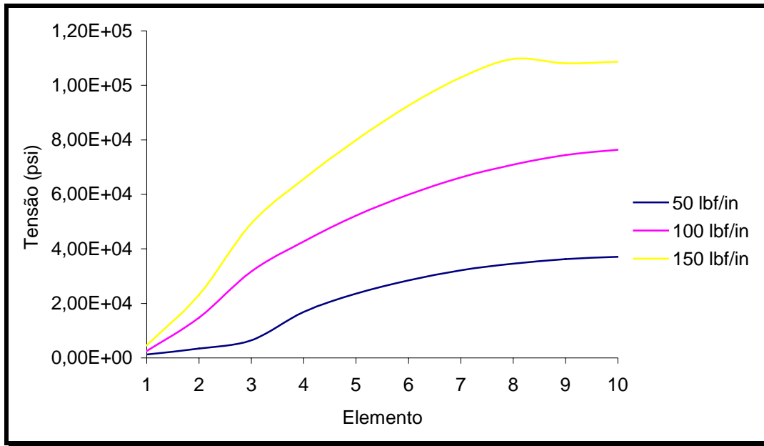
Figura 6.2.35- Gráfico: distribuição da tensão no centro dos elementos da barra de aço – ANLEC 2007 (a) .
