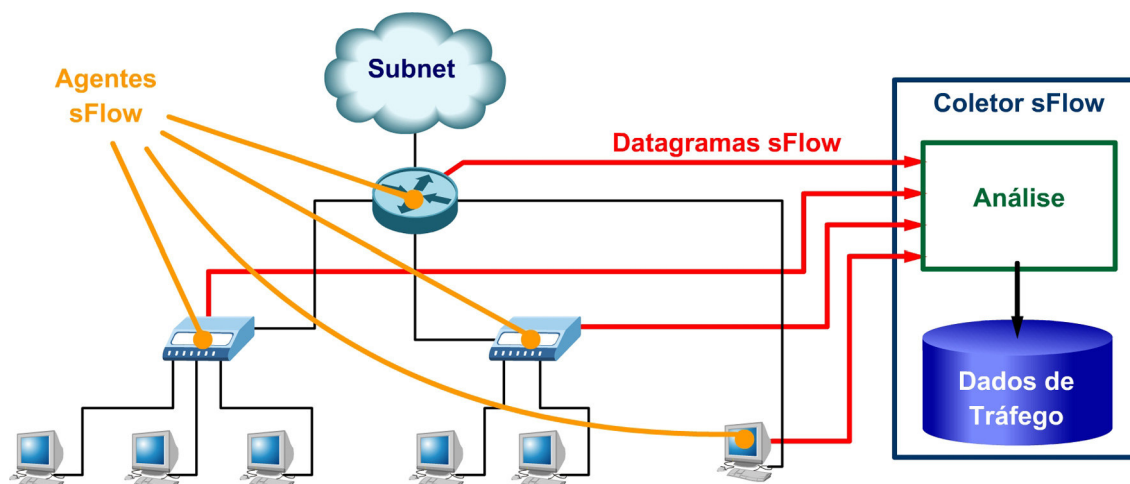
Figura 5 Arquitetura sFlow.
