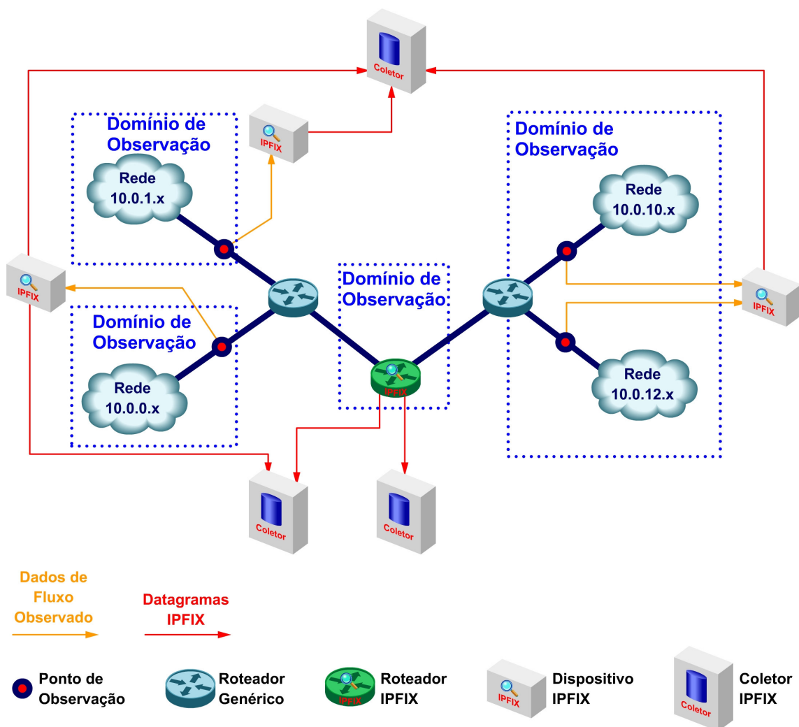
Figura 6 Arquitetura IPFIX.
