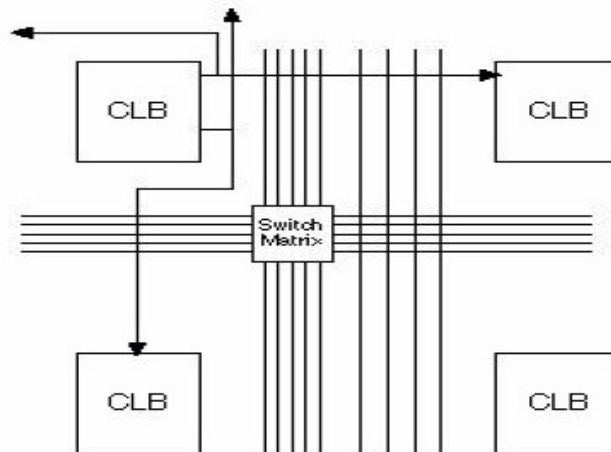
Figura 2.3 – Interconexão programável de um FPGA (TOROK, 2001).
