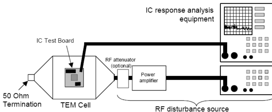
Figura 5.12 – TEM-Cell (IEC, 2004).
