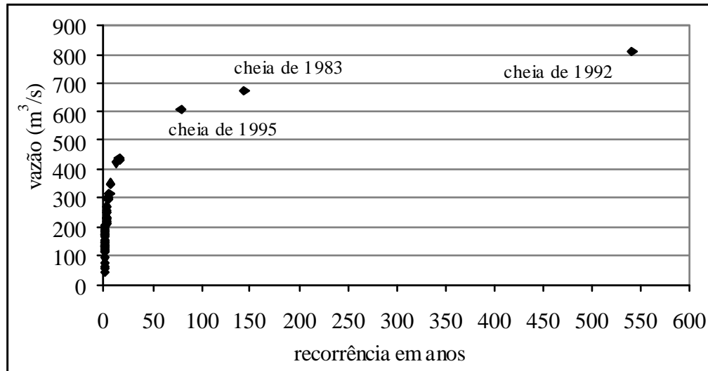
Gráfico 26 - Recorrência das vazões máximas anuais – seção Rio dos Patos
