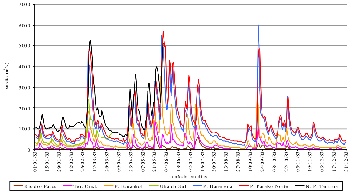
Gráfico 28 - Cheia Tipo A – ano de 1983
