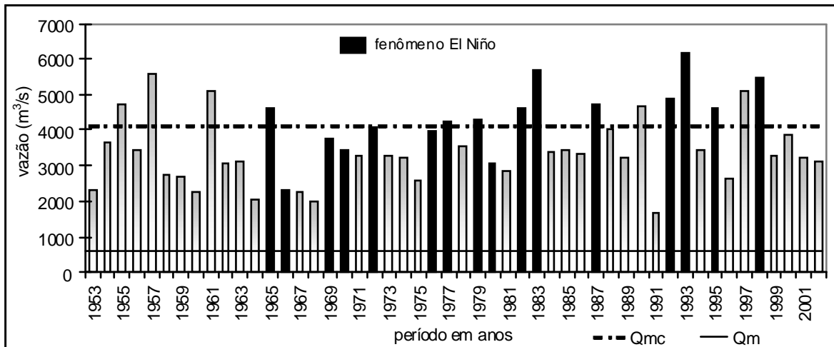
Gráfico 24 - Vazões máximas anuais, seção Porto Paraíso do Norte – período 1953 - 2003
