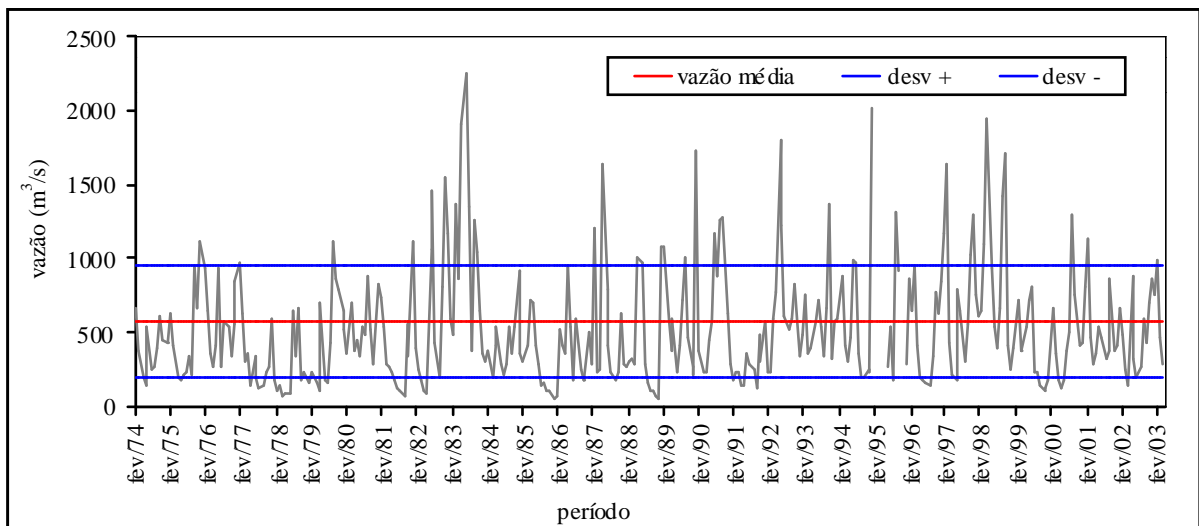
Gráfico 50 - Vazão média mensal – estação Porto Bananeira
