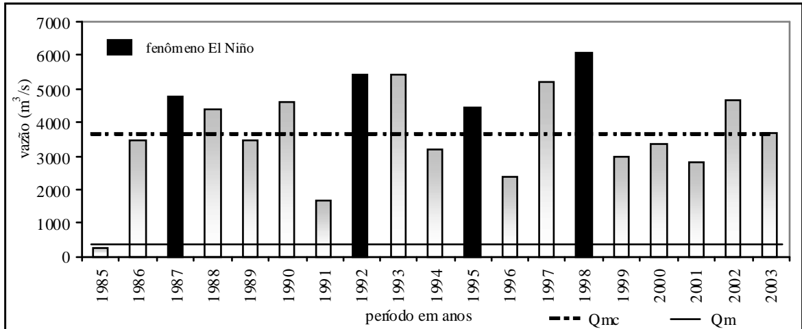
Gráfico 22 - Vazões máximas anuais, seção Vila Rica – período 1985 - 2003
