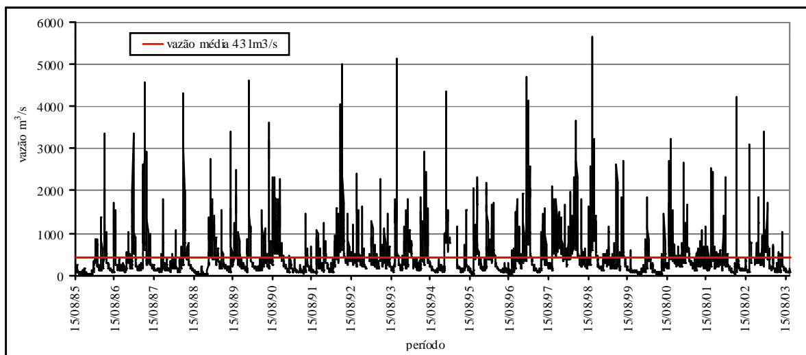
Gráfico 5 – Vazão média diária do rio Ivaí na estação Vila Rica, no segmento médio – 15/8/1985 – 30/9/2003
