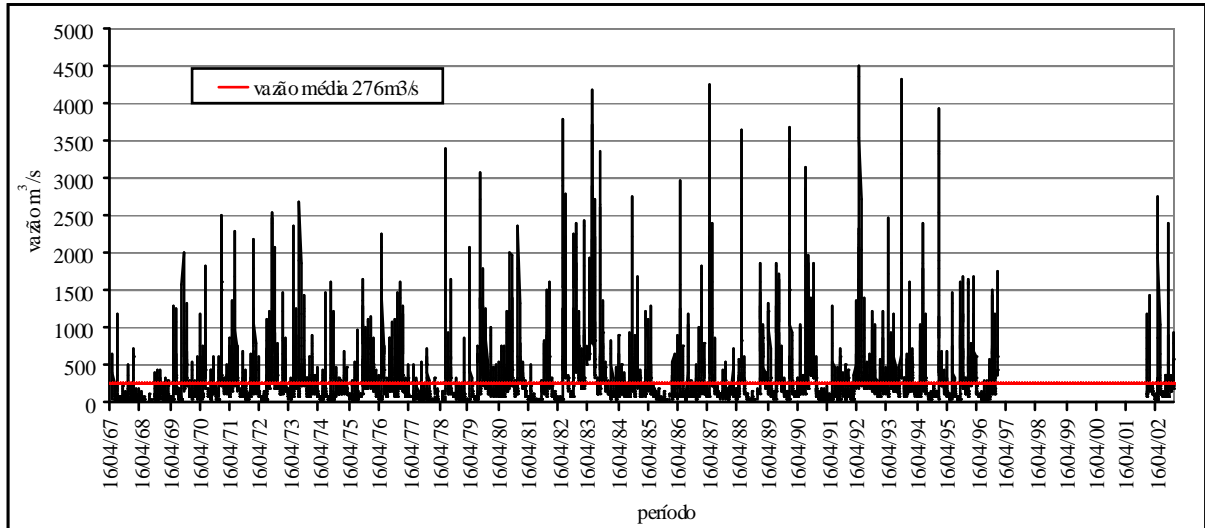
Gráfico 4 – Vazão média diária do rio Ivaí na estação Ubá do Sul, segmento superior – período 16/4/1967 – 30/11/2002
