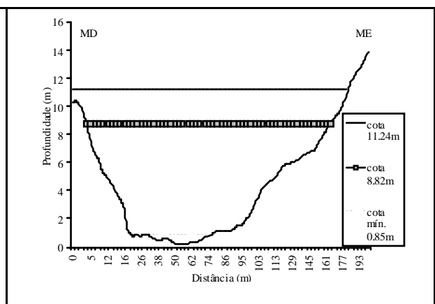
Figura 5 - Perfil transversal - seção Tereza Cristina
