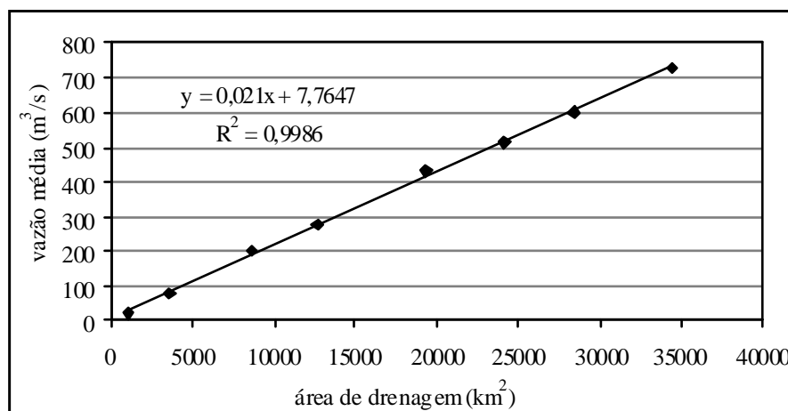
Gráfico 9 – Correlação vazões médias vs área de drenagem
