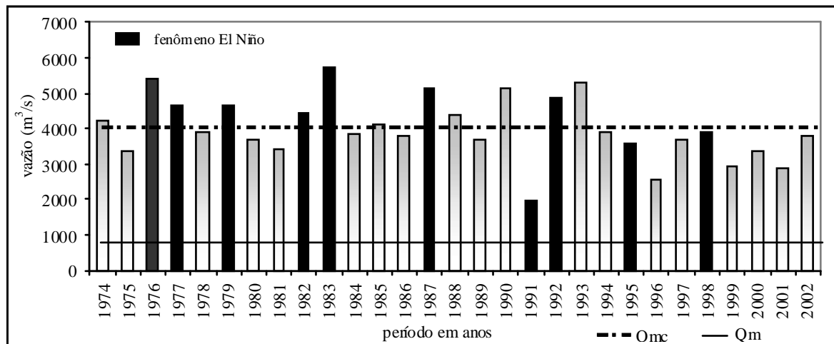
Gráfico 25 - Vazões máximas anuais, seção Novo Porto Taquara – período 1974 - 2002
