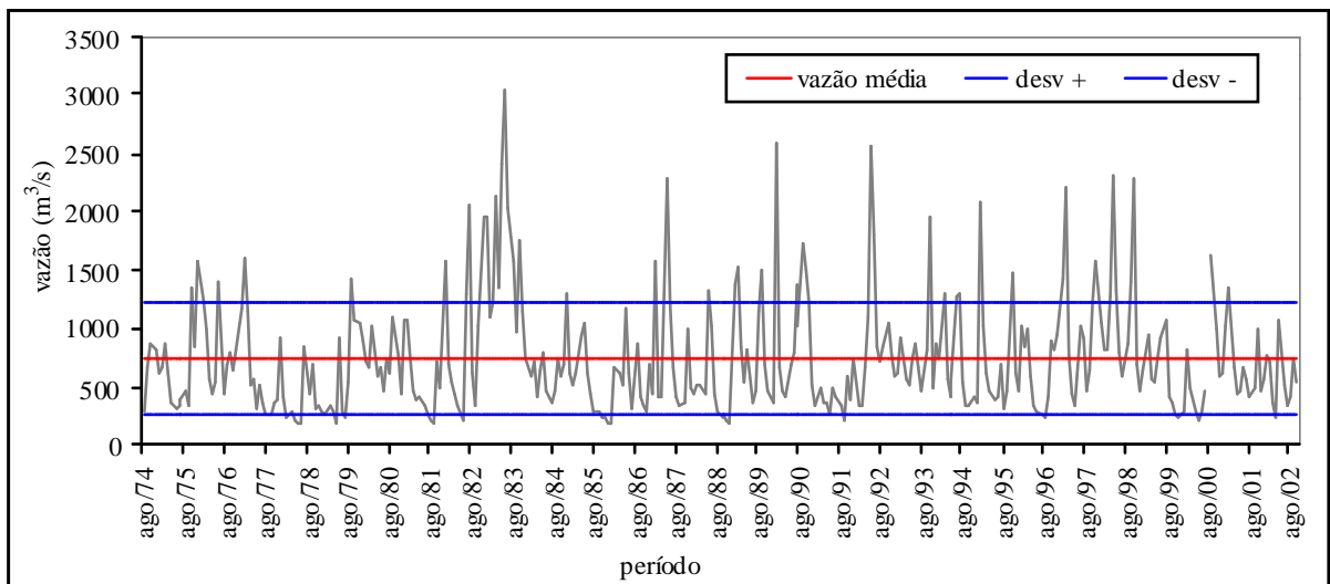
Gráfico 52 - Vazão média mensal do rio Ivaí – estação Novo Porto Taquara
