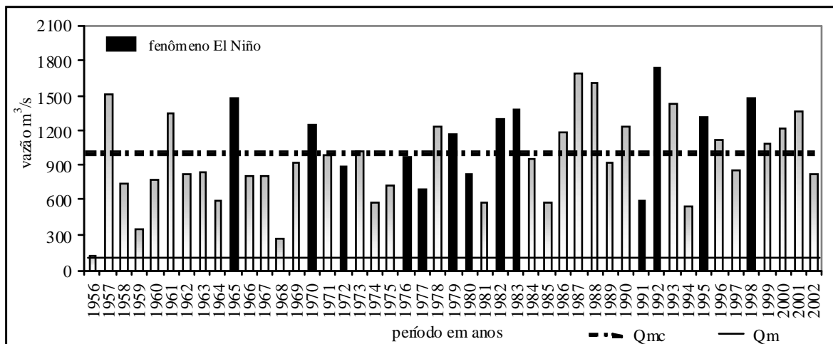
Gráfico 19 - Vazões máximas anuais, seção Tereza Cristina – período 1956 - 2002
