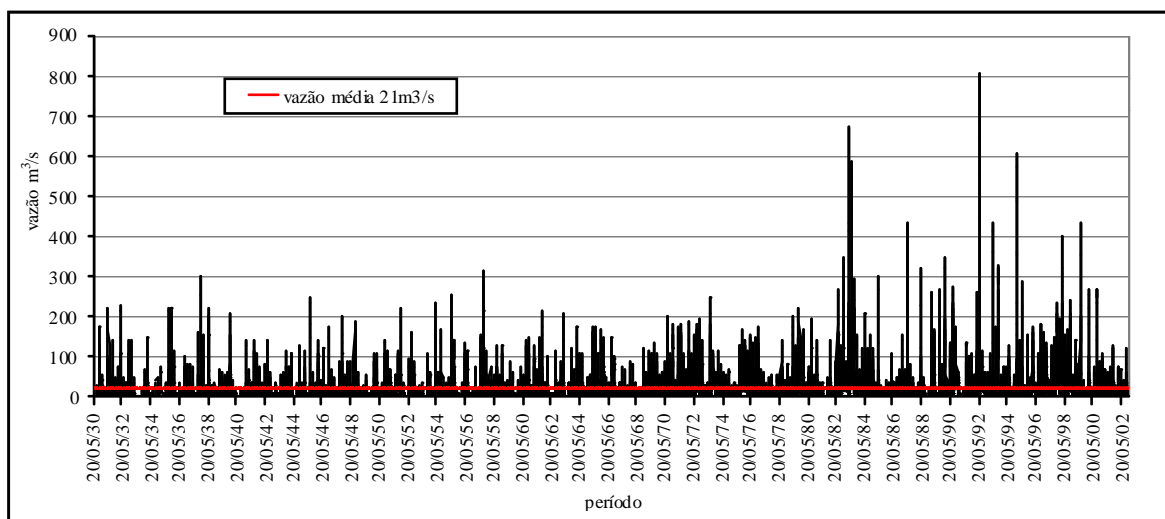
Gráfico 1 – Vazão média diária do rio dos Patos na estação Rio dos Patos, segmento superior – período 20/5/1930 – 30/9/2002
