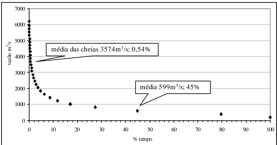
Gráfico 16 - Curva de duração do fluxo – seção Porto Paraíso do Norte
