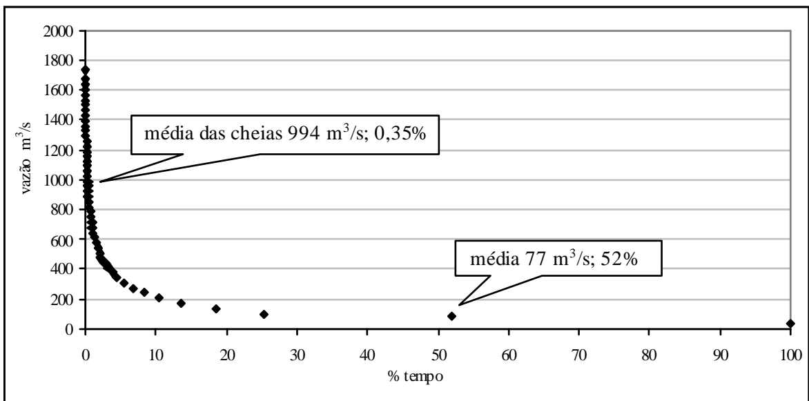
Gráfico 11 - Curva de duração do fluxo – seção Tereza Cristina
