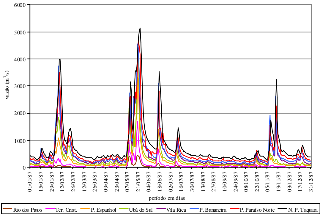
Gráfico 30 - Cheia Tipo B – ano de 1987
