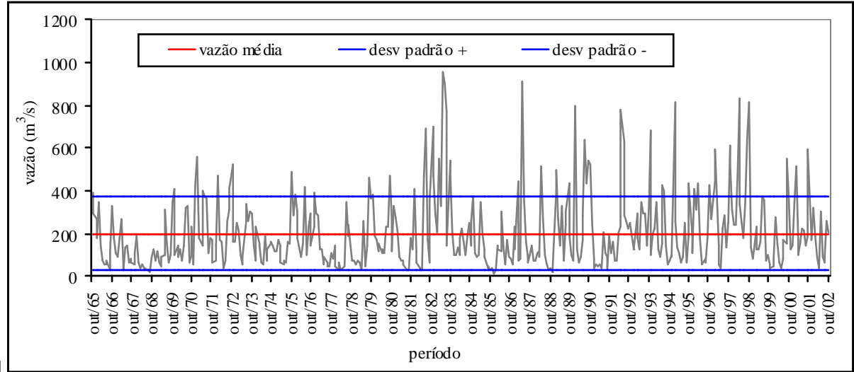
Gráfico 47 - Vazão média mensal – estação Porto Espanhol
