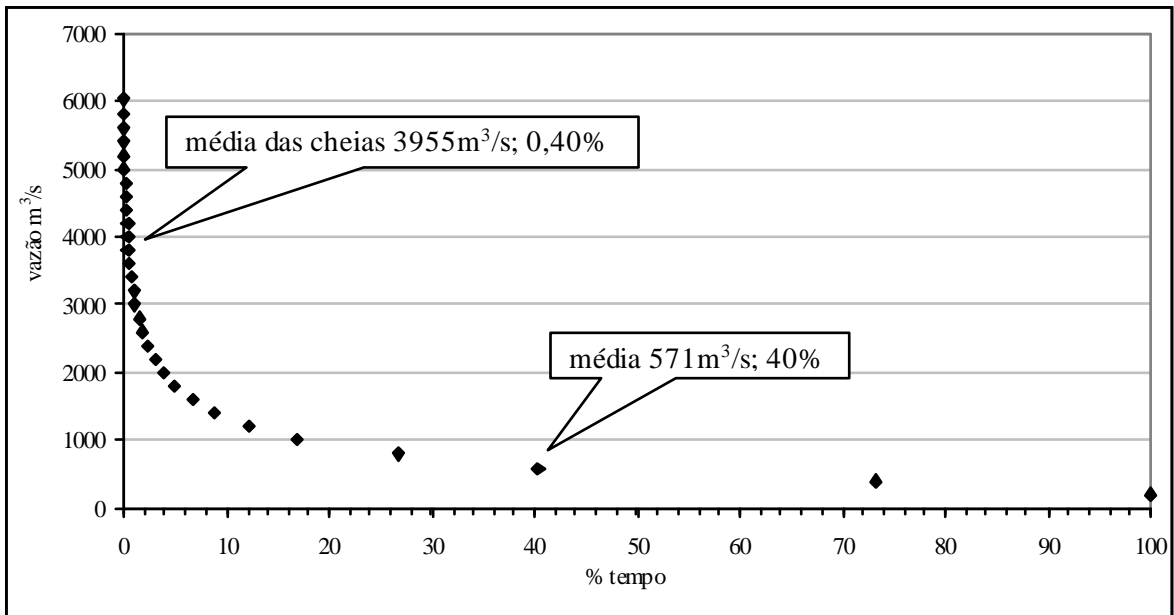
Gráfico 15 - Curva de duração do fluxo – seção Porto Bananeira
