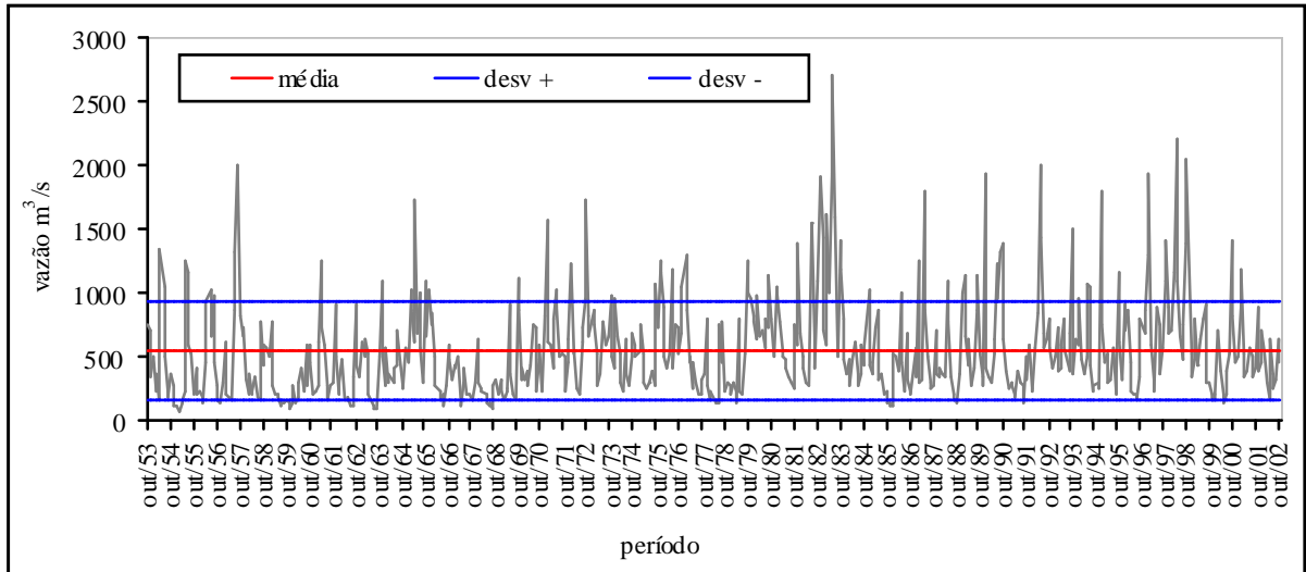
Gráfico 51 - Vazão média mensal do rio Ivaí – estação Porto Paraíso do Norte
