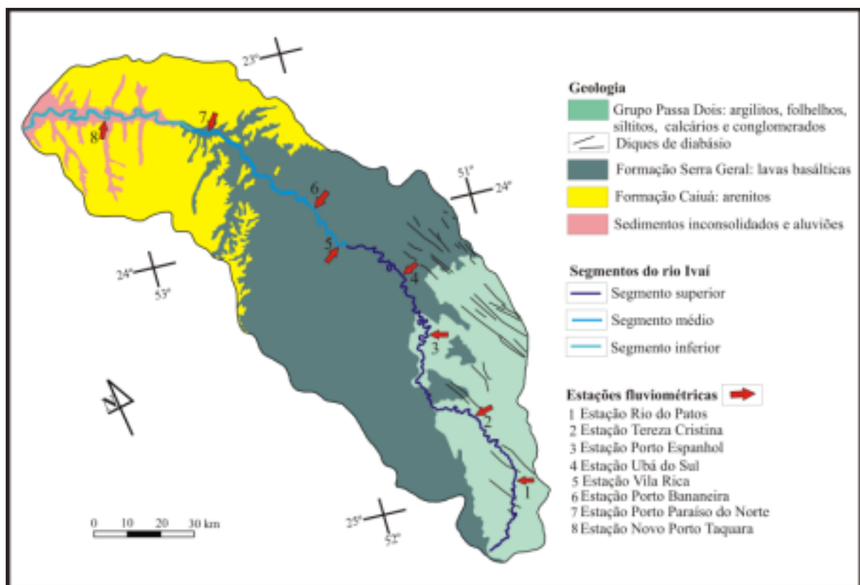
Figura 2 - Unidades geológicas da bacia hidrográfica do rio Ivaí Fonte: PARANÁ (1998); MINEROPAR (2000)
