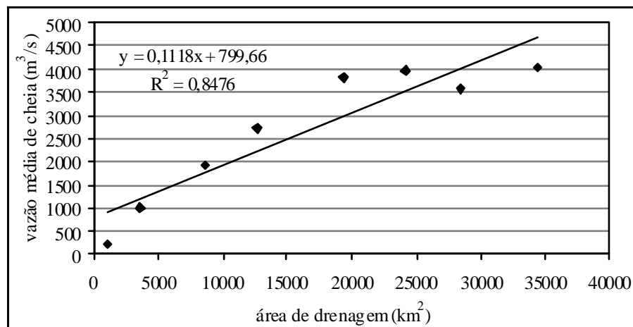
Gráfico 36 - Correlação área de drenagem vs vazão média das cheias anuais
