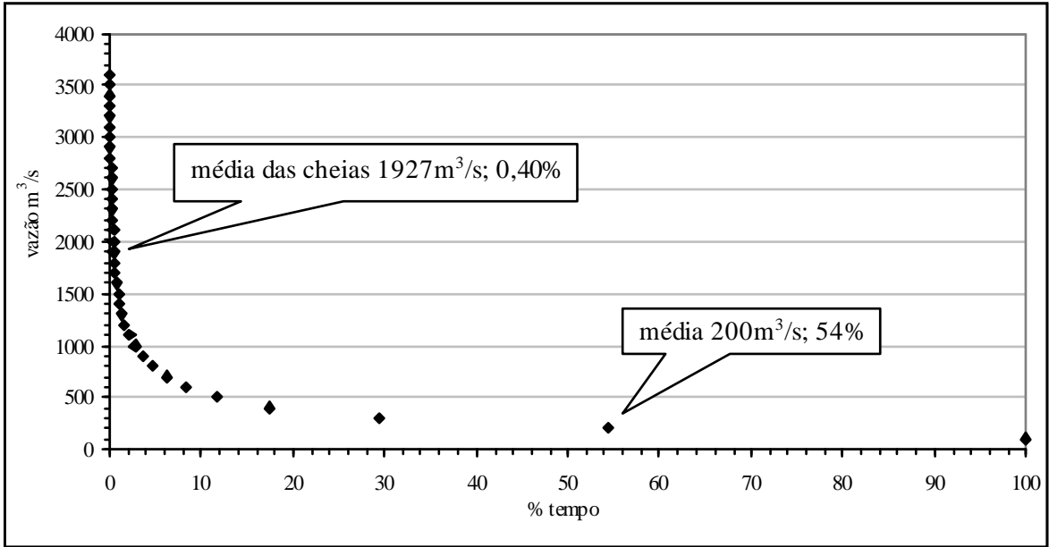
Gráfico 12 - Curva de duração do fluxo – seção Porto Espanhol
