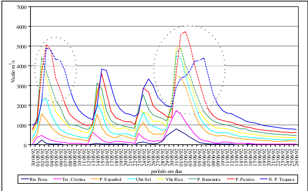
Gráfico 35 - Onda da cheia de mai/jun de 1992, com um pico máximo de cheia para a estação Porto Paraíso do Norte ao invés de Novo Porto Taquara que por sua vez, configura um amortecimento de pico da cheia
