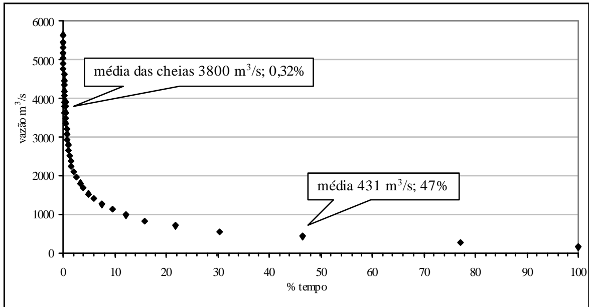
Gráfico 14 - Curva de duração do fluxo – seção Vila Rica
