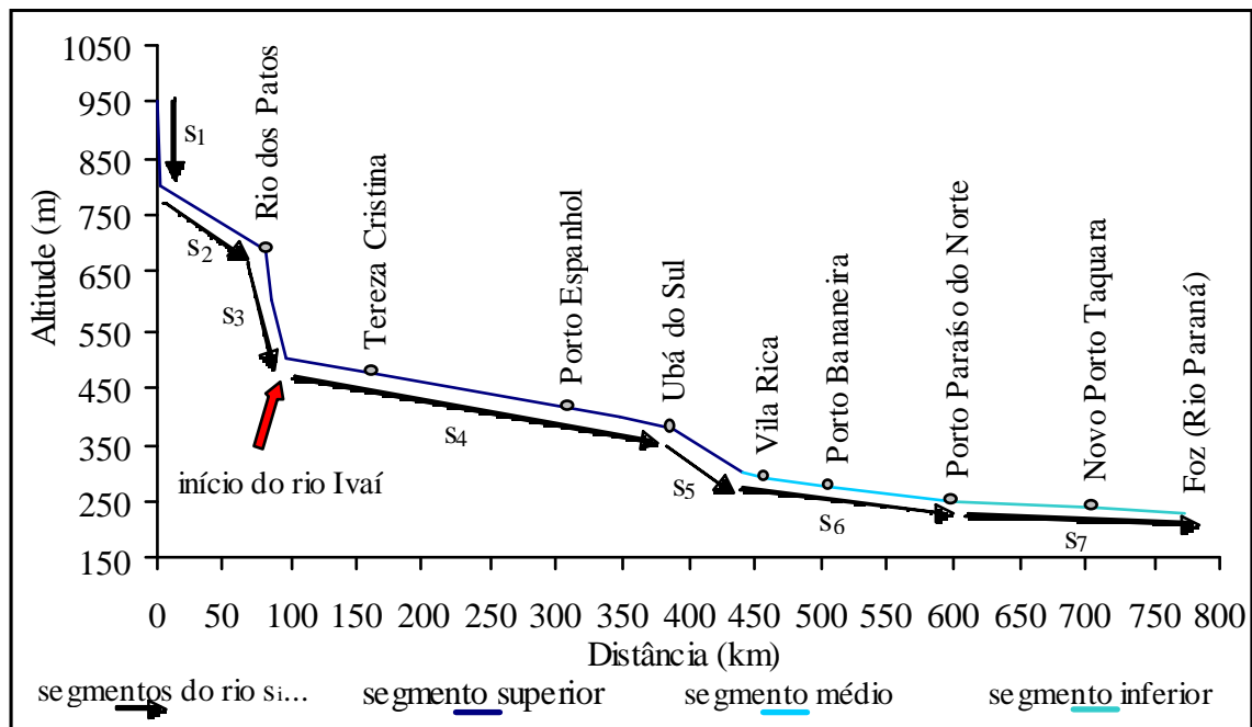
Figura 3 - Perfil longitudinal do rio Ivaí
