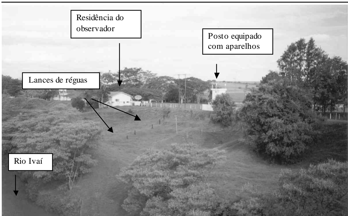
Foto 2 – Estação fluviométrica de Porto Paraíso do Norte – segmento médio
