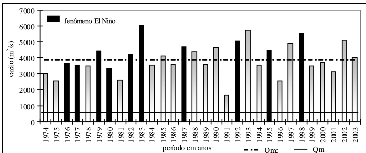
Gráfico 23 - Vazões máximas anuais, seção Porto Bananeira – período 1974 - 2003
