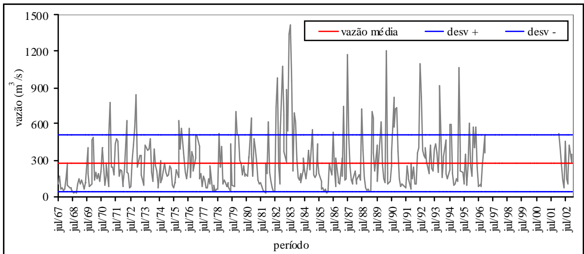
Gráfico 48 - Vazão média mensal – estação Ubá do Sul
