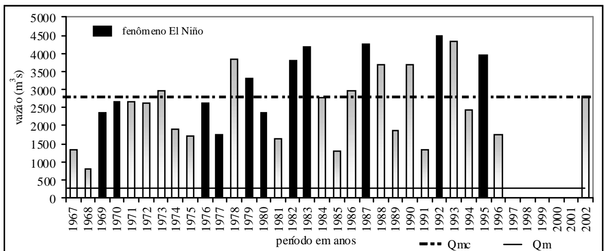
Gráfico 21 - Vazões máximas anuais, seção Ubá do Sul – período 1967 - 2002
