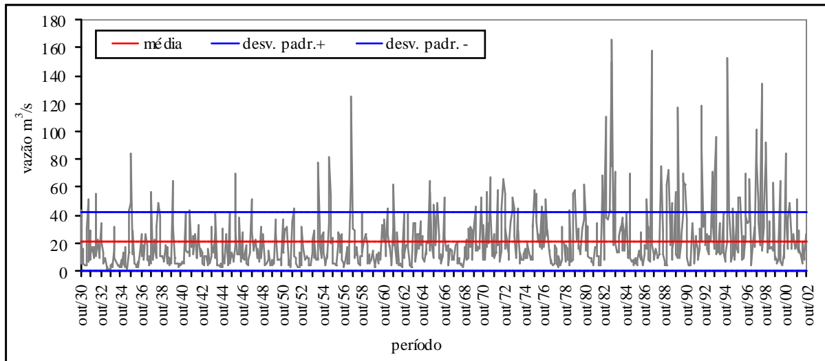
Gráfico 45 - Vazão média mensal – estação Rio dos Patos
