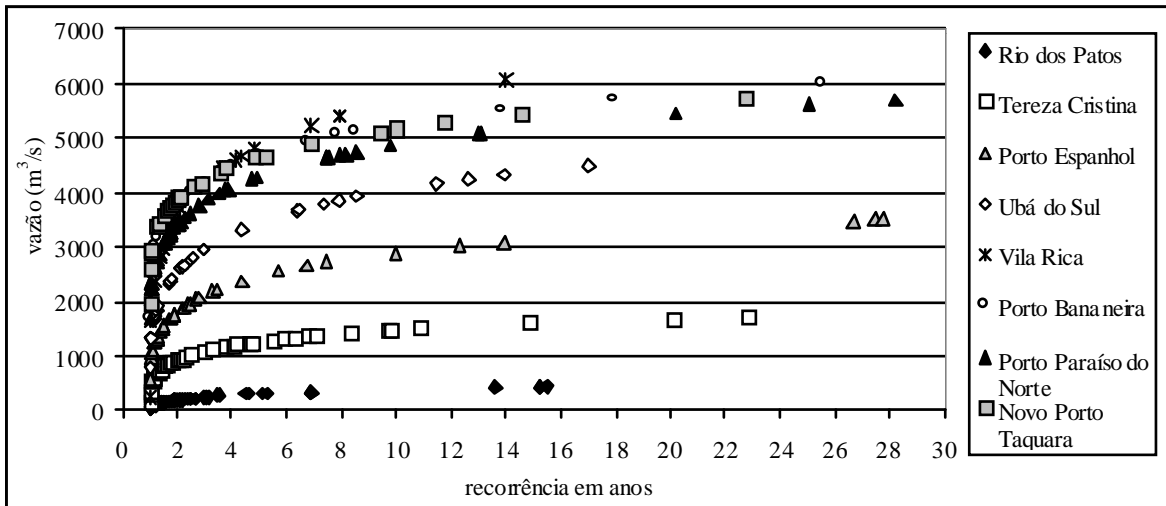
Gráfico 27 - Recorrência das vazões máximas anuais para as seções do rio Ivaí
