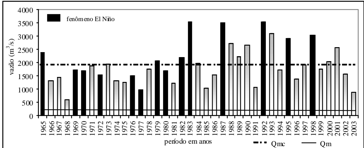
Gráfico 20 - Vazões máximas anuais, seção Porto Espanhol – período 1965 - 2003
