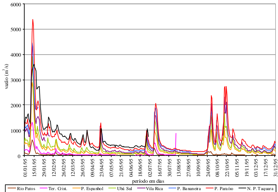
Gráfico 34 - Cheia Tipo C – ano de 1995
