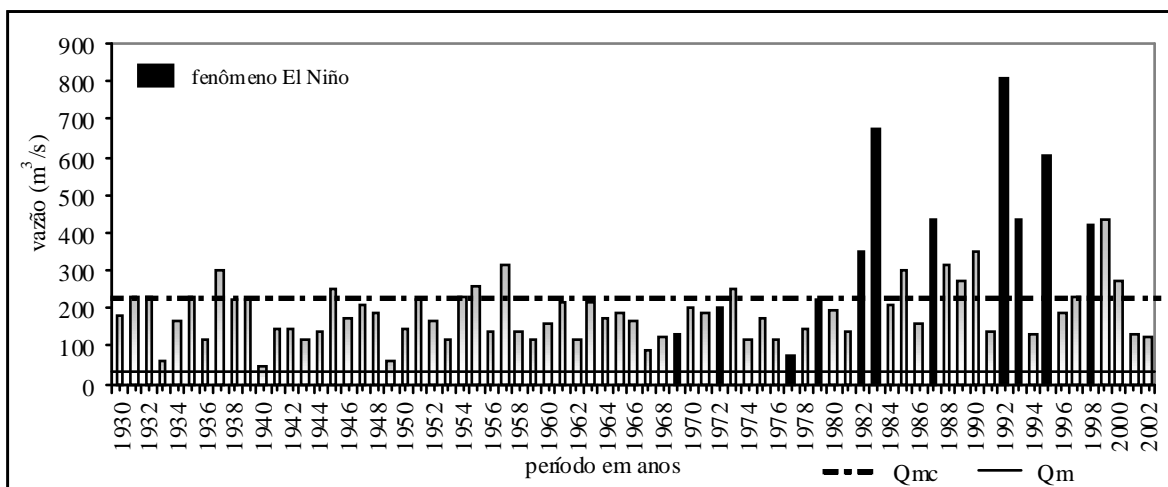
Gráfico 18 - Vazões máximas anuais, seção Rio dos Patos – período 1930 - 2002
