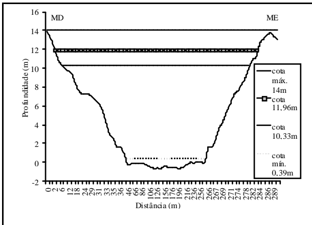
Figura 10 - Perfil transversal - seção Porto Paraíso do Norte Figura 11 - Perfil transversal - seção Novo Porto Taquara
