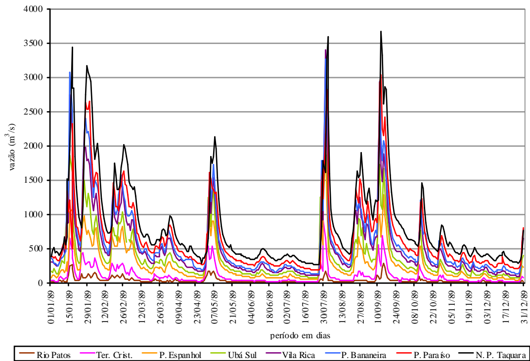
Gráfico 31 - Cheia Tipo B – ano de 1989
