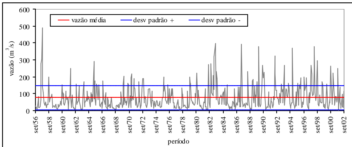
Gráfico 46 - Vazão média mensal – estação Tereza Cristina
