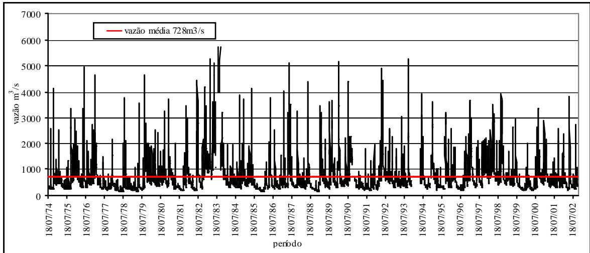
Gráfico 8 – Vazão média diária do rio Ivaí na estação de Novo Porto Taquara, segmento inferior – período 8/7/1974 – 31/10/2002
