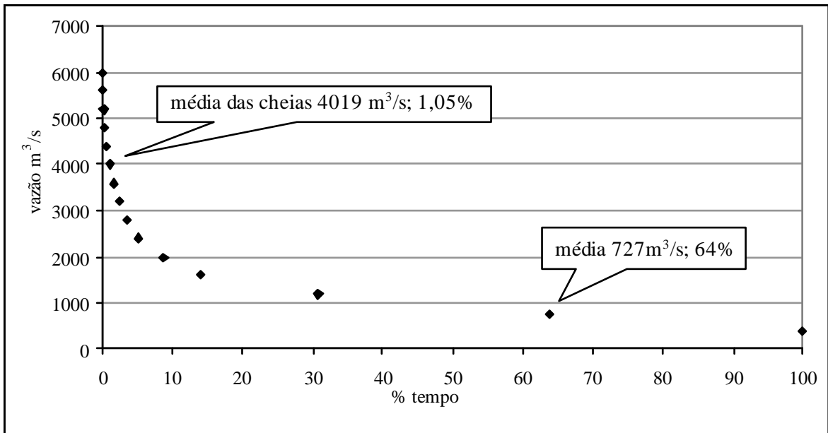
Gráfico 17 - Curva de duração do fluxo – seção Novo Porto Taquara
