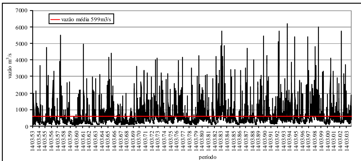
Gráfico 7 – Vazão média diária do rio Ivaí na estação de Porto Paraíso do Norte, segmento médio – período 14/3/1953 – 13/12/2003
