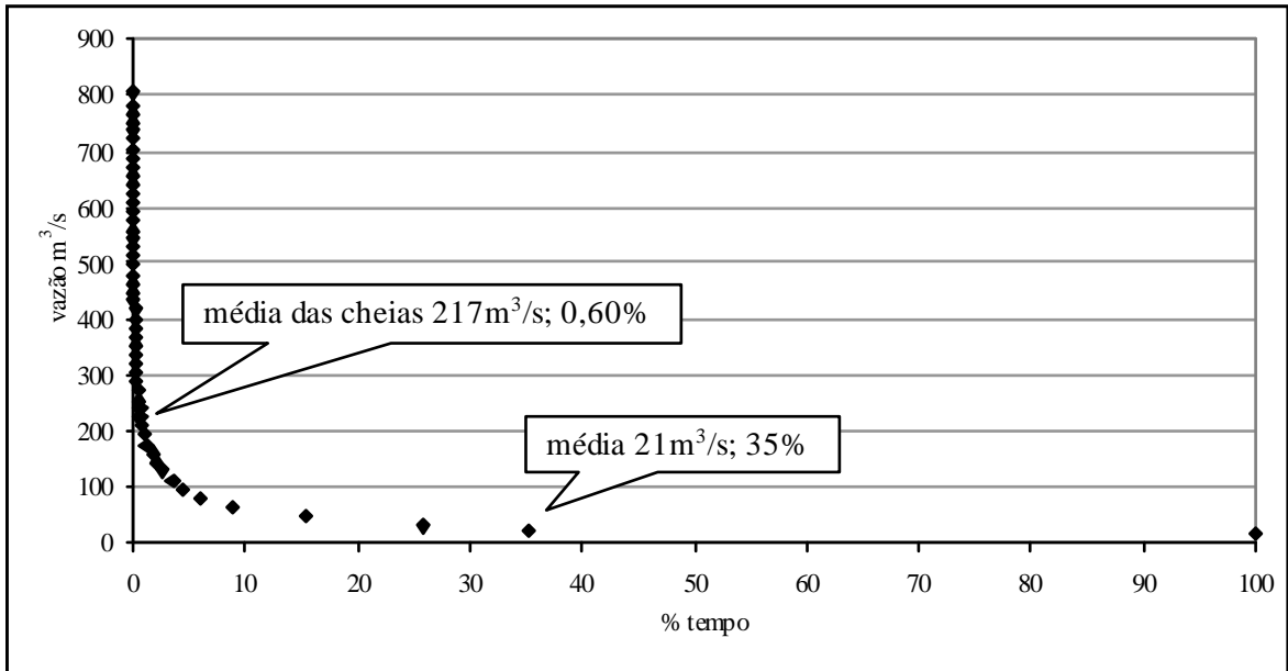
Gráfico 10 - Curva de duração do fluxo – seção Rio dos Patos
