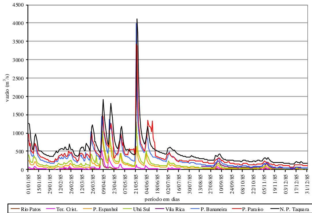
Gráfico 33 - Cheia Tipo C – ano de 1985
