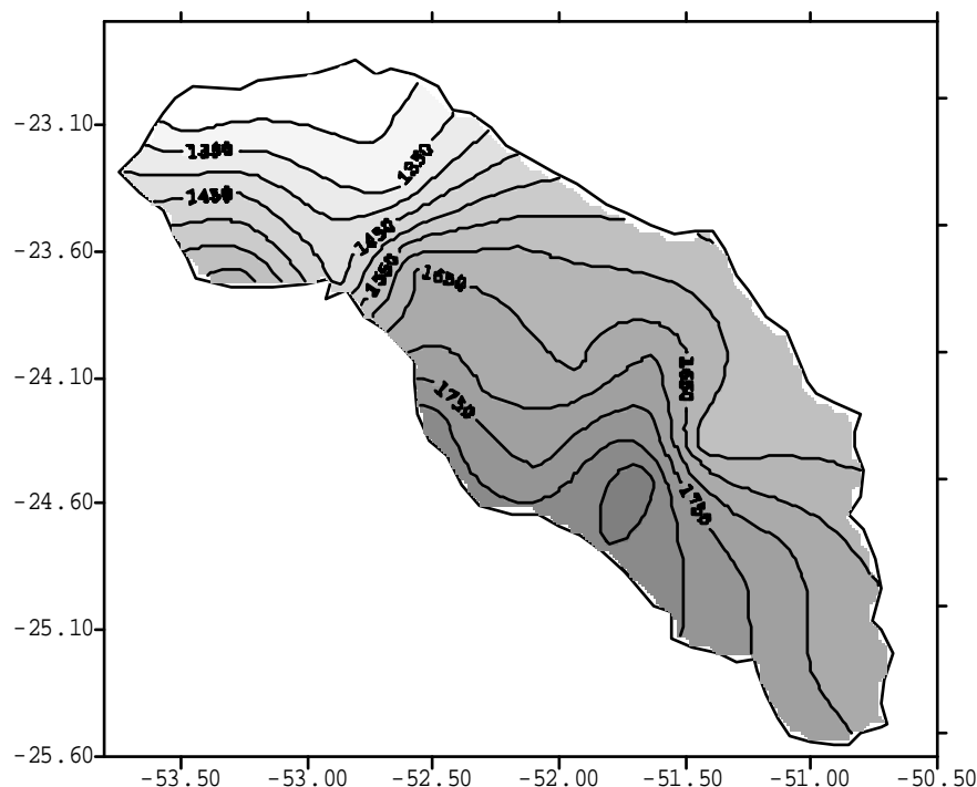
Figura 12 - Precipitação média na bacia hidrográfica do Ivaí Fonte: ANDRADE (2002)
