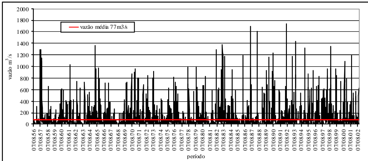
Gráfico 2 – Vazão média diária do rio Ivaí na estação Tereza Cristina, segmento superior – período 7/8/1956 – 30/9/2002
