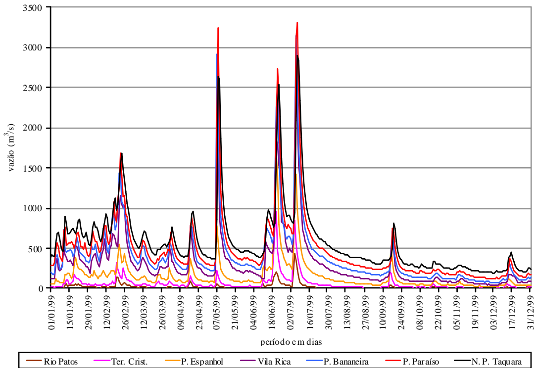
Gráfico 32 - Cheia Tipo B – ano de 1999
