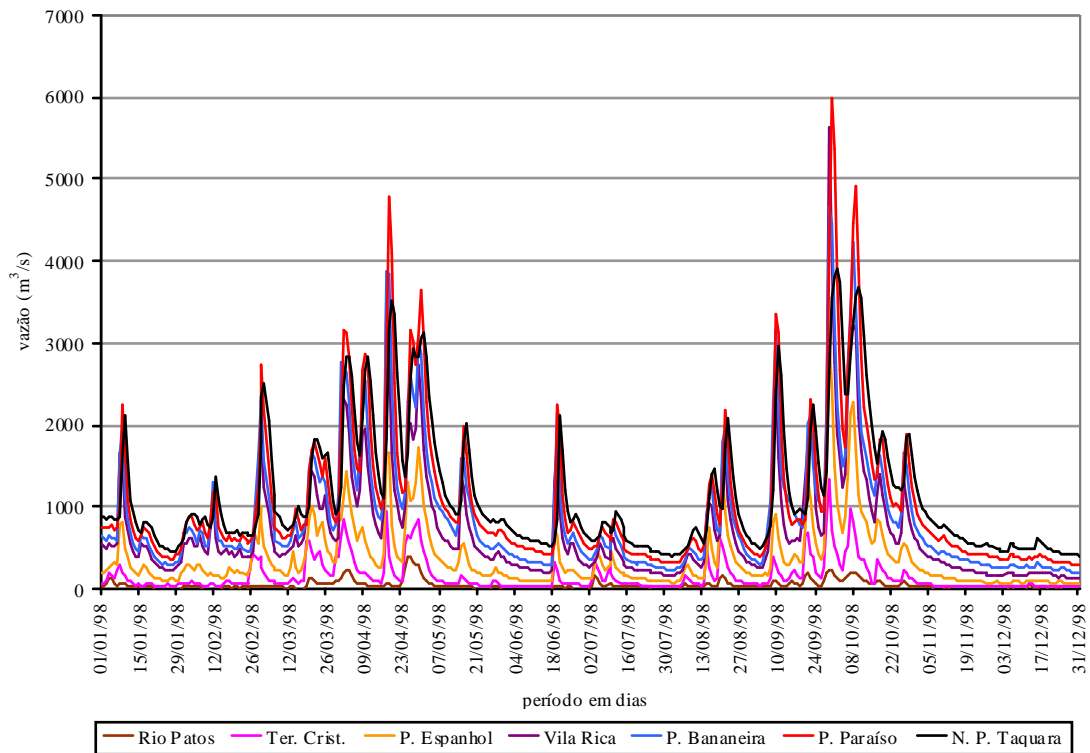
Gráfico 29 - Cheia Tipo A – ano de 1998
