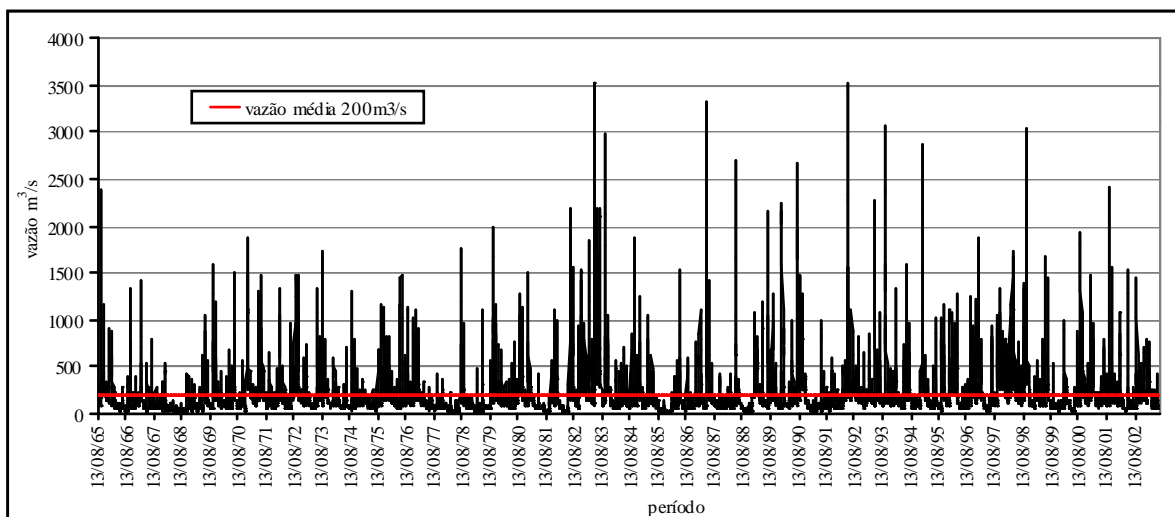
Gráfico 3 – Vazão média diária do rio Ivaí na estação Porto Espanhol, segmento superior – período 13/8/1965 – 30/6/2003
