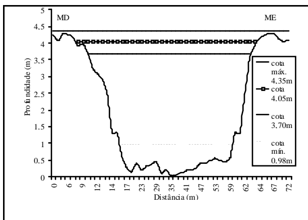
Figura 4 - Perfil transversal - seção Rio dos Patos
