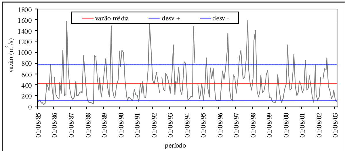
Gráfico 49 - Vazão média mensal – estação Vila Rica
