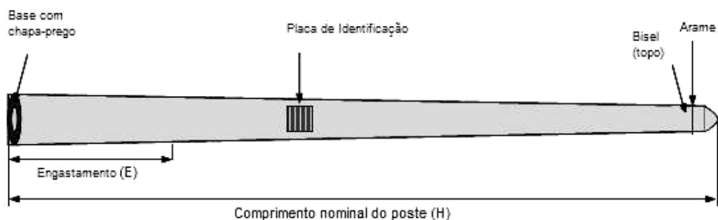
Figura 4 – Modelo de poste de madeira utilizado pela AES Sul (Adaptado de VIDOR, 2003).
