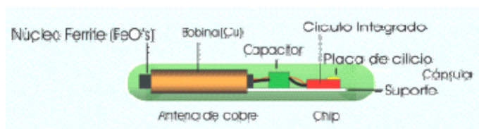
Figura 10 – Modelo de TAG RFID, construção interna (PINHEIRO, 2005).
