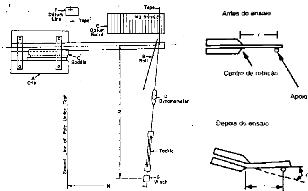
Figura 7 – Esquemático para ensaio de flexão em postes de madeira segundo a norma ASTM D1036 – Standard Test Methods of Static Tests of Wood Poles, 1990.
