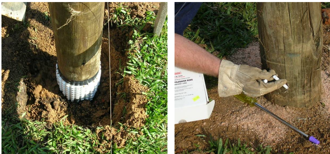
Figura 23 – Fotos dos preservativos sendo aplicados: A bandagem Bioguard (esquerda) e os bastonetes Polisaver (PRESCHEM, 2004).
