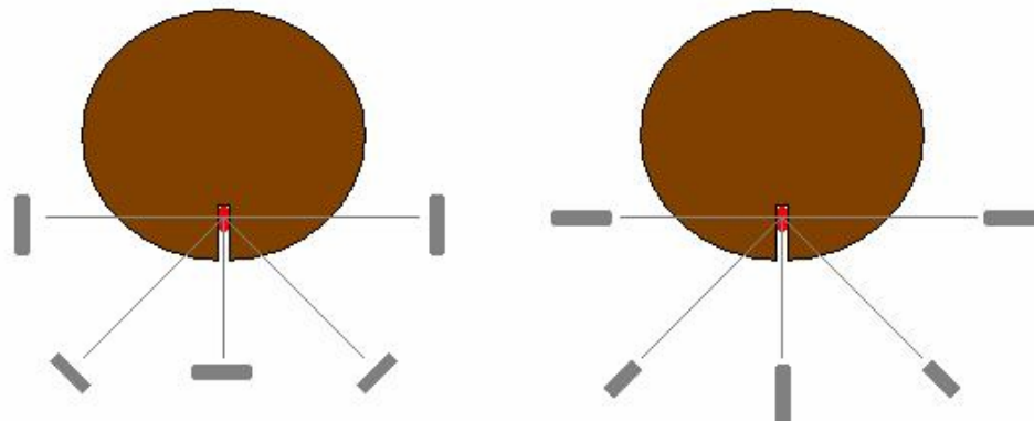
Figura 26 – Vista de corte horizontal, indicando o TAG (em vermelho), o poste (marrom), e a antena de leitura (em cinza). Esquema dos testes de leitura.
