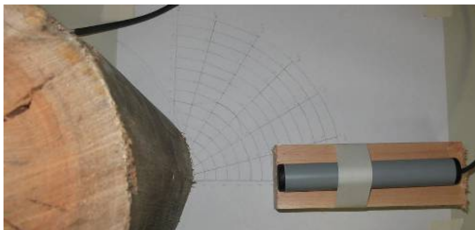
Figura 27 – Esquema de montagem do teste de bancada para determinar a área de leitura dos TAGs implantados na madeira. Escala para medição das distâncias máximas de leitura em diferentes ângulos.
