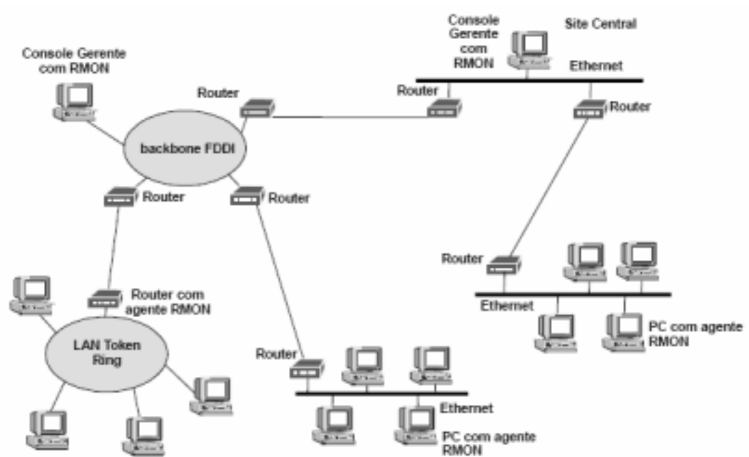
Figura C.5 – Estrutura de redes com gerenciamento RMON
