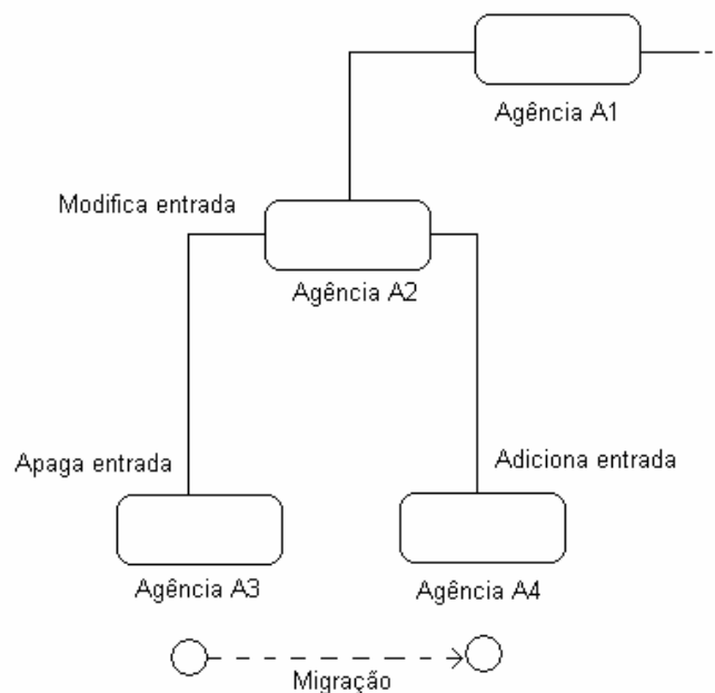
Figura 3.7 – Abordagem Hierárquica.
