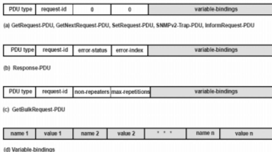
Figura C.3 – Estrutura das mensagens SNMPv2
