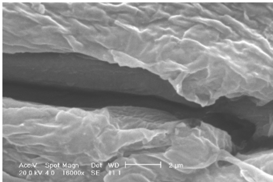
Figura 9: Fotografia de um UHMWPE, com um aumento de 16000X. Foto produzida no MEV da PUCRS.
