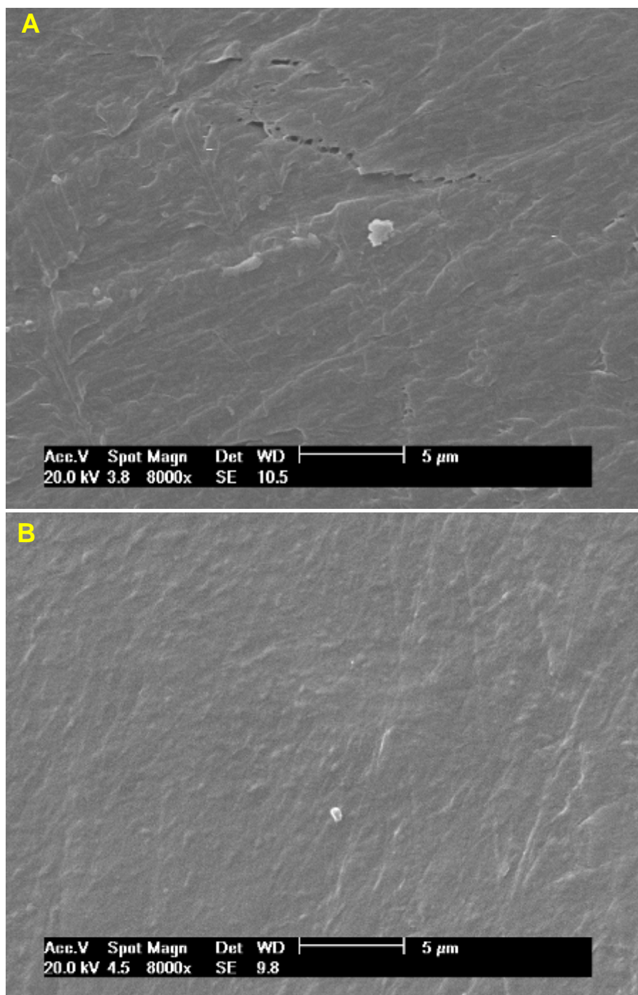
Figura 35: Micrografia das amostras AB01 (A) e AB03 (B) com magnificação de 8000 vezes.
