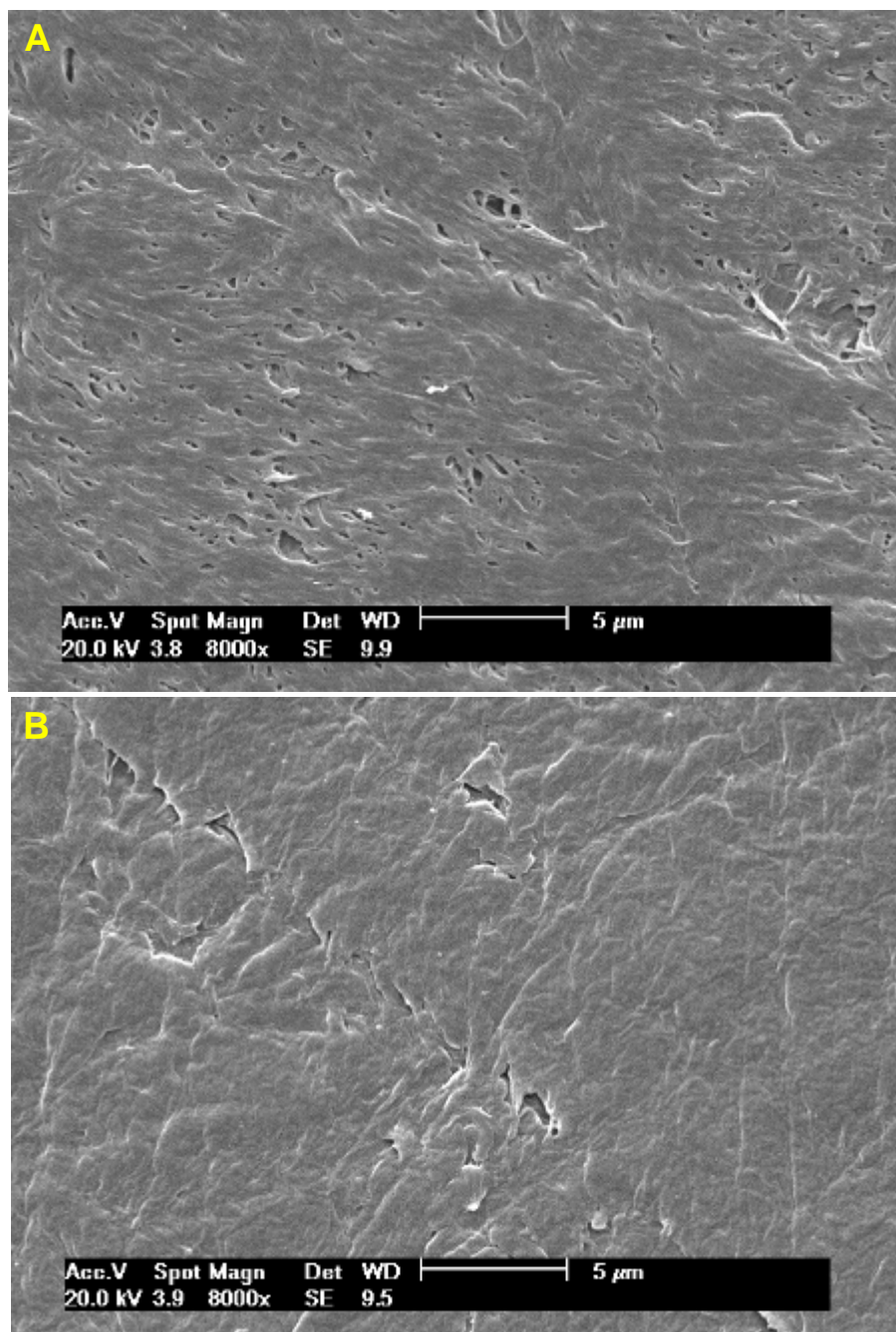
Figura 37: Micrografias das amostras AB05 (A) e AB06 (B) com magnificação de 8000 vezes.
