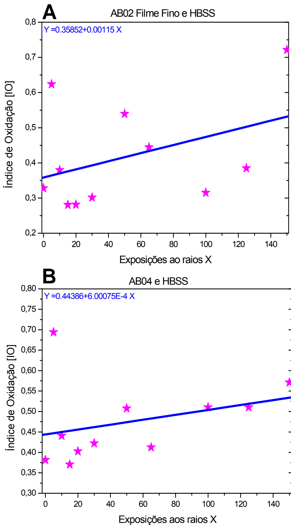
Figura 29: Índice de oxidação (IO) para as amostras irradiadas aos raios X diagnóstico e submersas em HBSS. Amostra AB02 (A) com filme fino e amostra AB04 (B) somente submersa.
