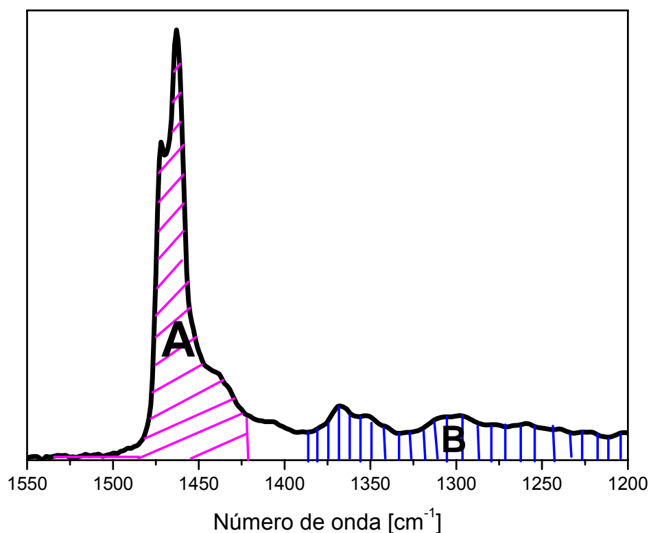
Figura 17: Áreas utilizadas para o cálculo de índice de oxidação para as amostras.
