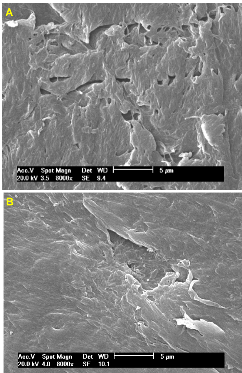
Figura 36: Micrografia das amostras AB02 (A) e AB04 (B) com magnificação de 8000 vezes.
