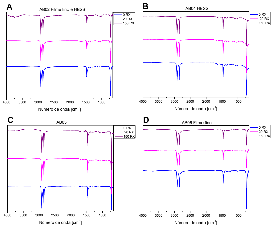
Figura 27: Espectro de FTIR-ATR das amostras de UHMWPE irradiadas nos raios X convencional. Amostra AB02 (A) tinha filme fino e foi submersa em HBSS, amostra AB04 (B) foi submersa em HBSS, amostra AB05 (C) não possuía filme fino e ficou em ar e a amostra AB06 (D) tinha filme fino e ficou em ambiente atmosférico.
