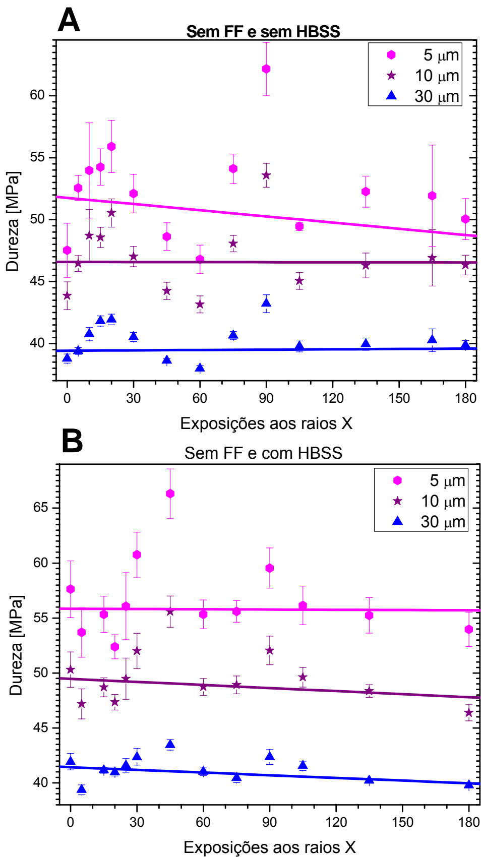
Figura 20: Dureza obtida pelo nano-indentador (do tipo Berkovich) para as amostras sem filme fino e no ar (A) e para as sem filme fino e na solução de Hank's (B).
