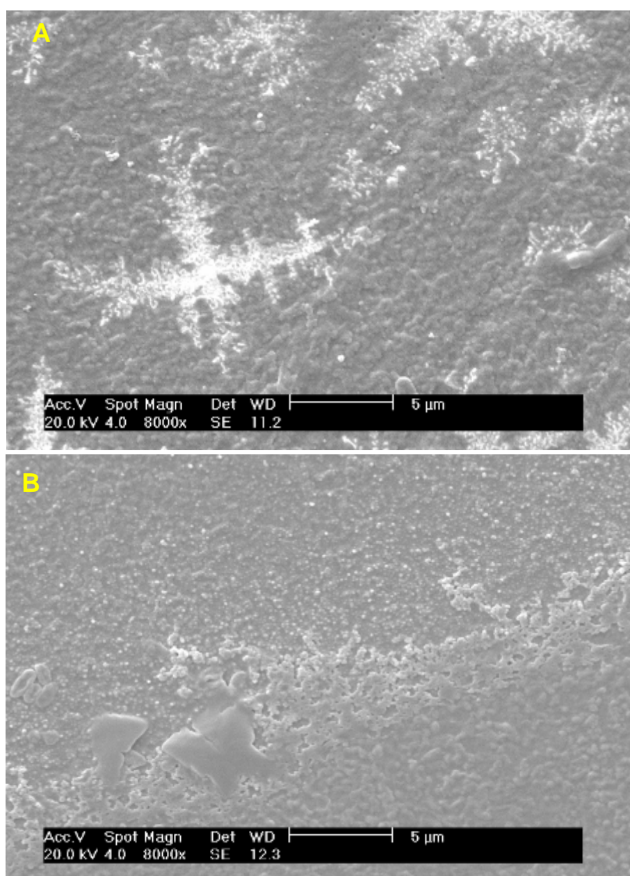
Figura 23: Micrografias das amostras A2 (A) e A18 (B) com magnificação de 8000 vezes.
