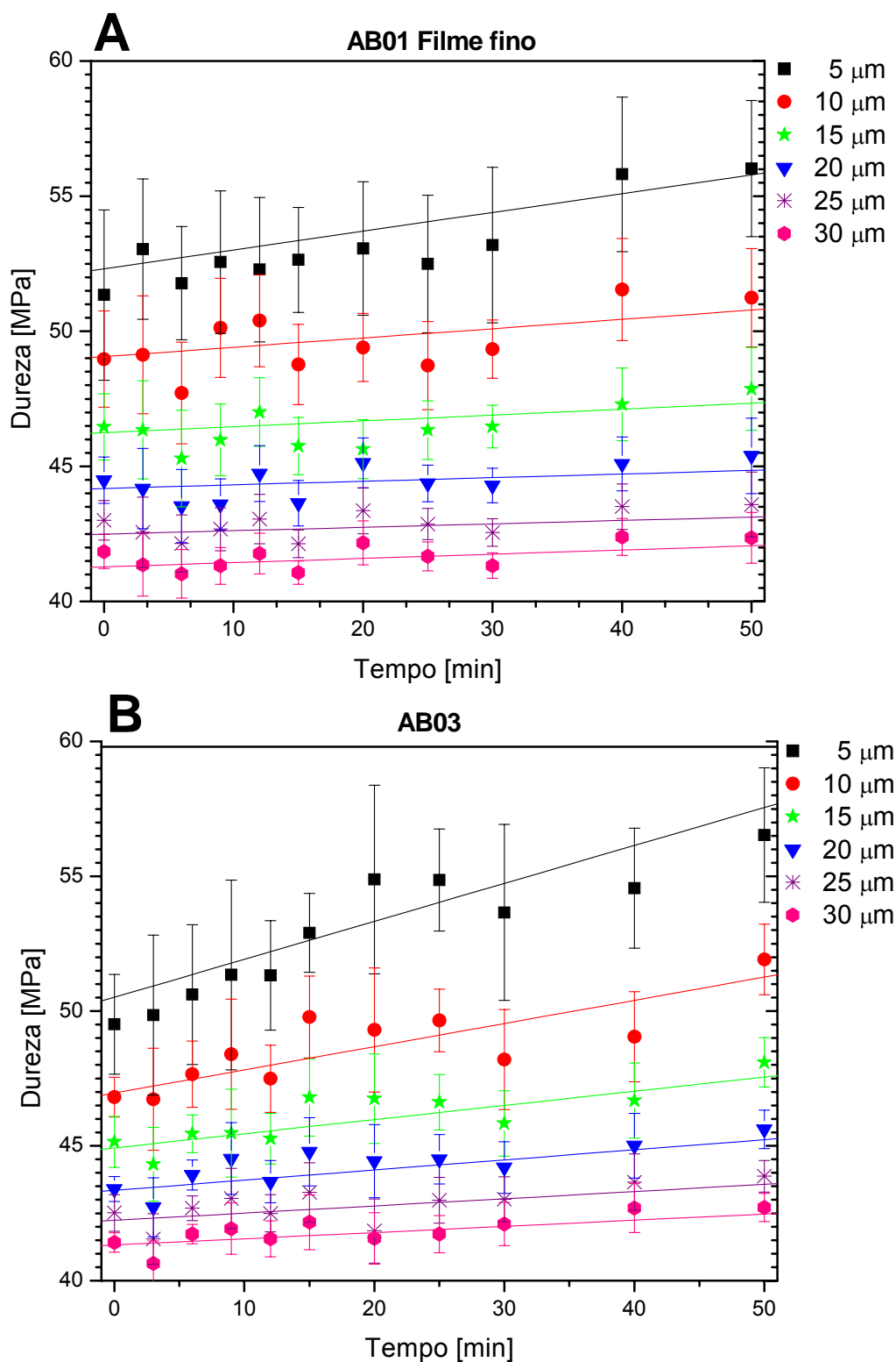
Figura 31: Dureza das amostras irradiadas em fluoroscopia (AB01 e AB03). Amostra AB01 (A) possuía filme fino de titânio e amostra AB03 (B) ao natural.
