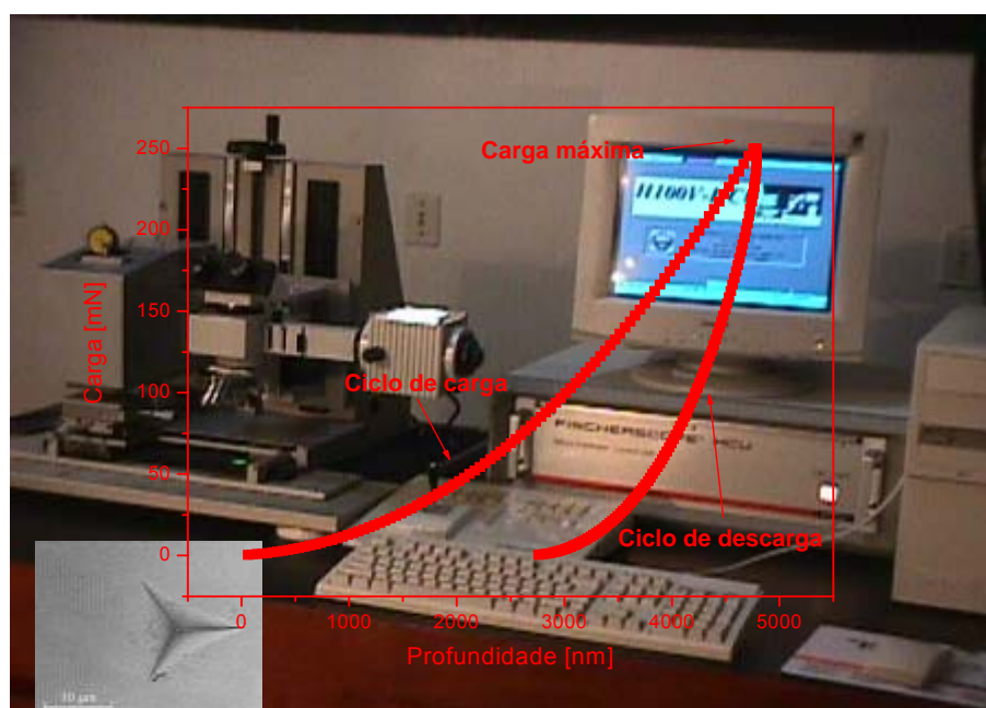
Figura 10: Ciclo carga-descarga de um equipamento de nanodureza.
