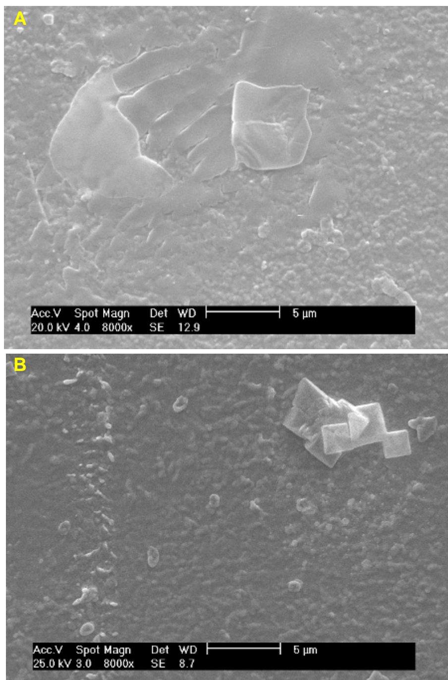
Figura 25: Micrografias das amostras A36 (A) e A52 (B) com magnificação de 8000 vezes.
