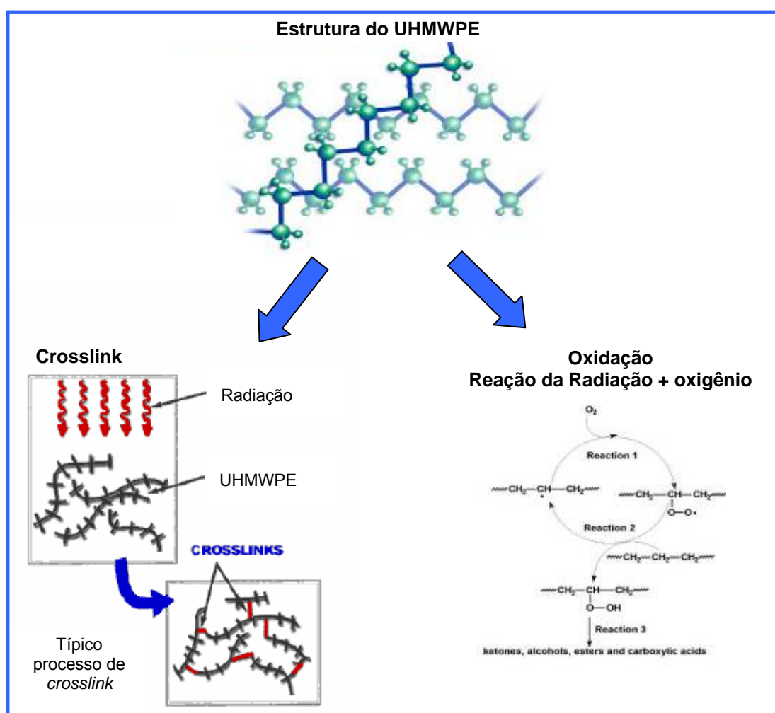
Figura 7: Esquema da oxidação e do crosslink do UHMWPE [19].
