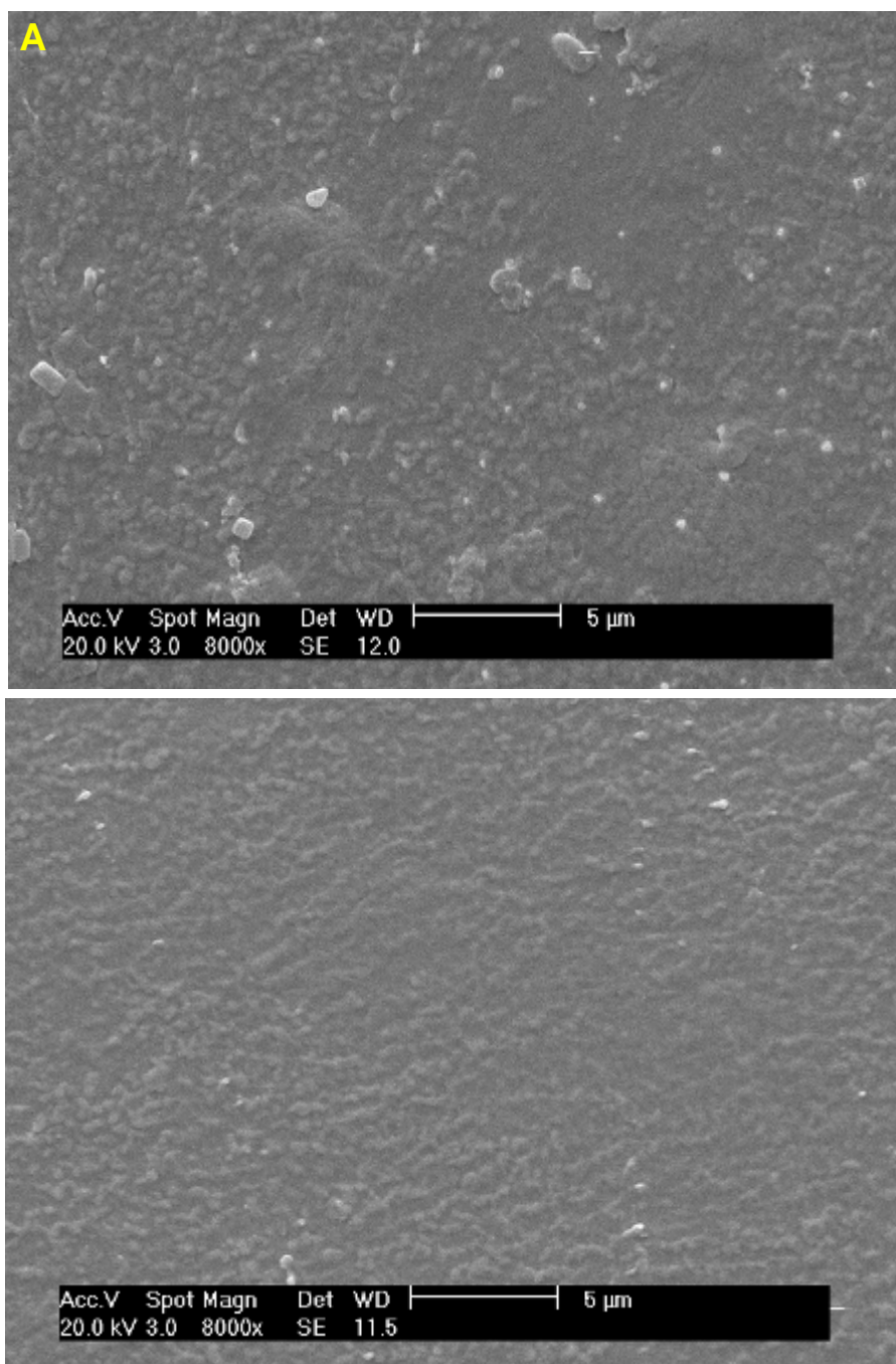
Figura 24: Micrografias das amostras A35 (A) e A68 (B) com magnificação de 8000 vezes.
