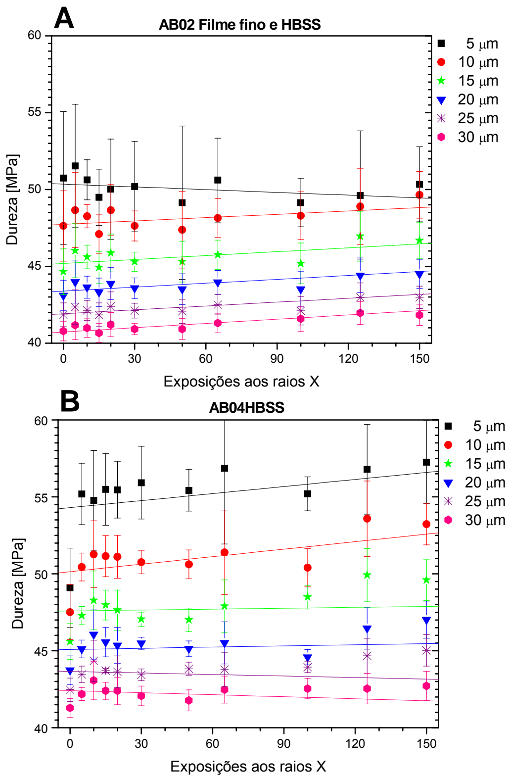
Figura 32: Dureza das amostras irradiadas no equipamento de raios X convencional. Amostra AB02 que tinha filme fino e estava em HBSS (A) e a amostra AB04 que estava submersa em HBSS (B).
