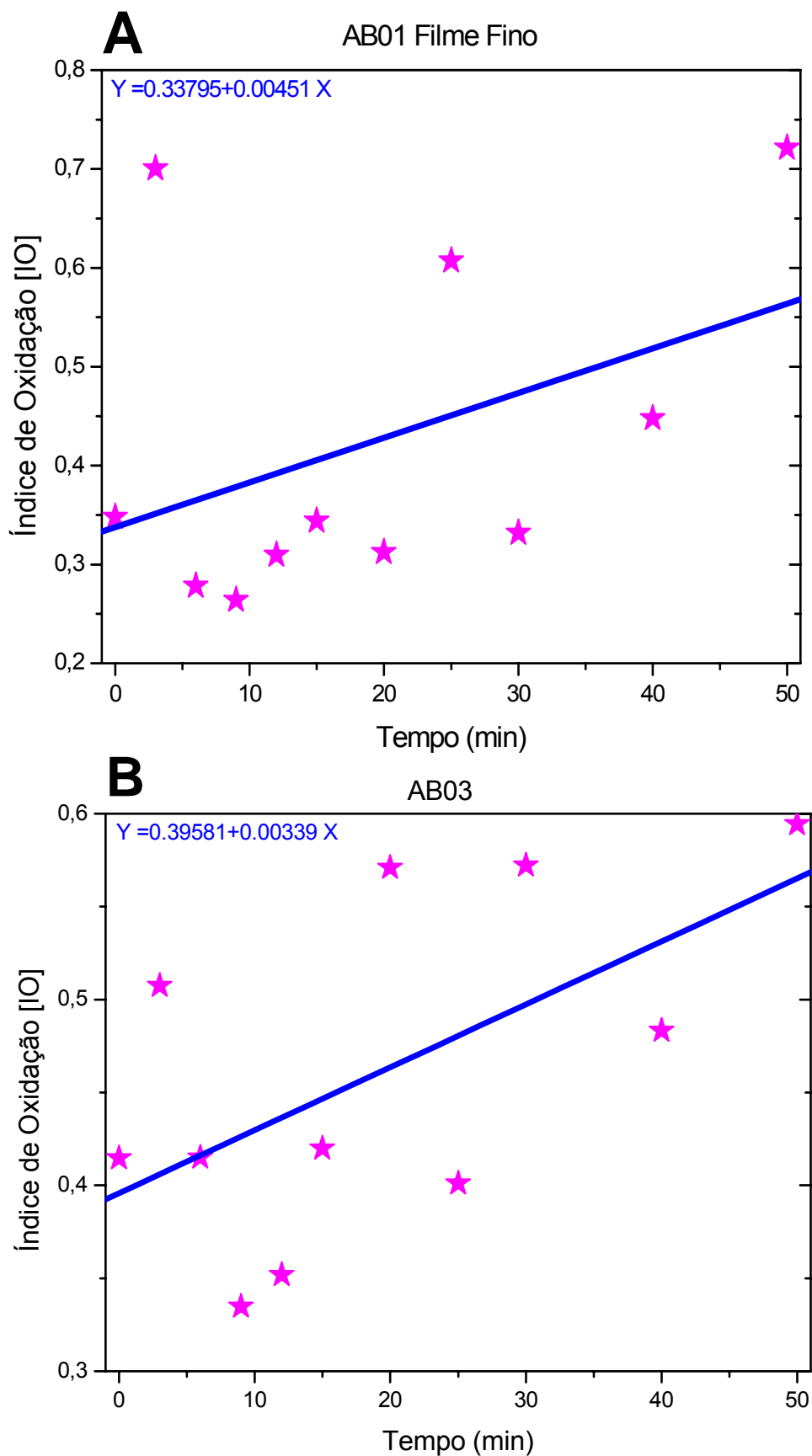
Figura 28: Índice de oxidação das amostras irradiadas na fluoroscopia. Amostra AB01 (A) que possuía filme fino e amostra AB03 (B) que estava ao natural.
