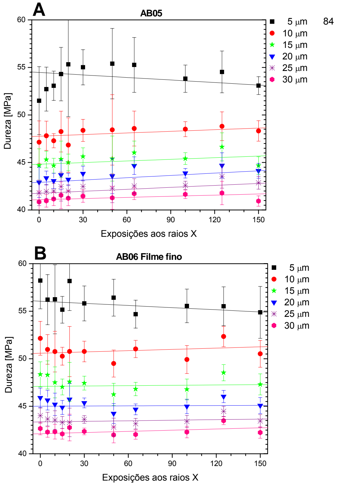
Figura 33: Dureza das amostras irradiadas no equipamento de raios X convencional. Amostra AB05 que estava em ar (A) e a amostra AB06 que tinha filme fino e foi exposta em ar (B).
