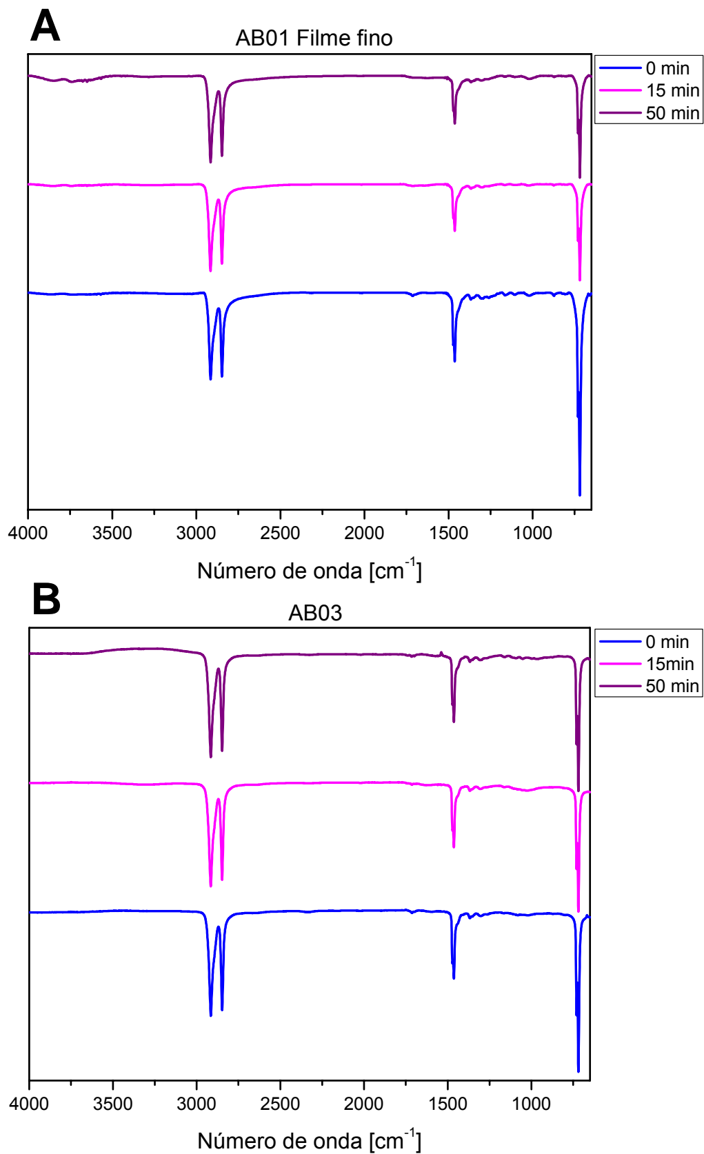
Figura 26: Espectro de FTIR-ATR das amostras de UHMWPE irradiadas na fluoroscopia. Amostra AB01 (A) que possuía filme fino de titânio e a amostra AB03 (B) que estava natural.
