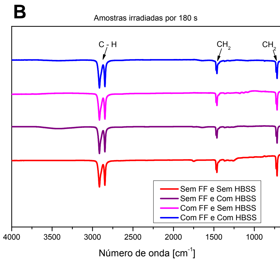
Figura 19: Espectros de FTIR com 75 exposições (A) e 180 exposições (B).
