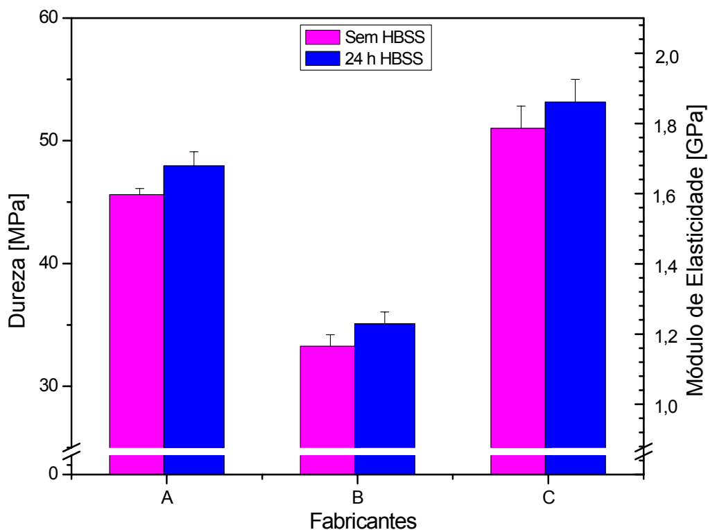
Figura 34: Teste de dureza e módulo de elasticidade realizado com amostras de UHMWPE de três diferentes fabricantes como recebidos e após 24 horas em HBSS.
