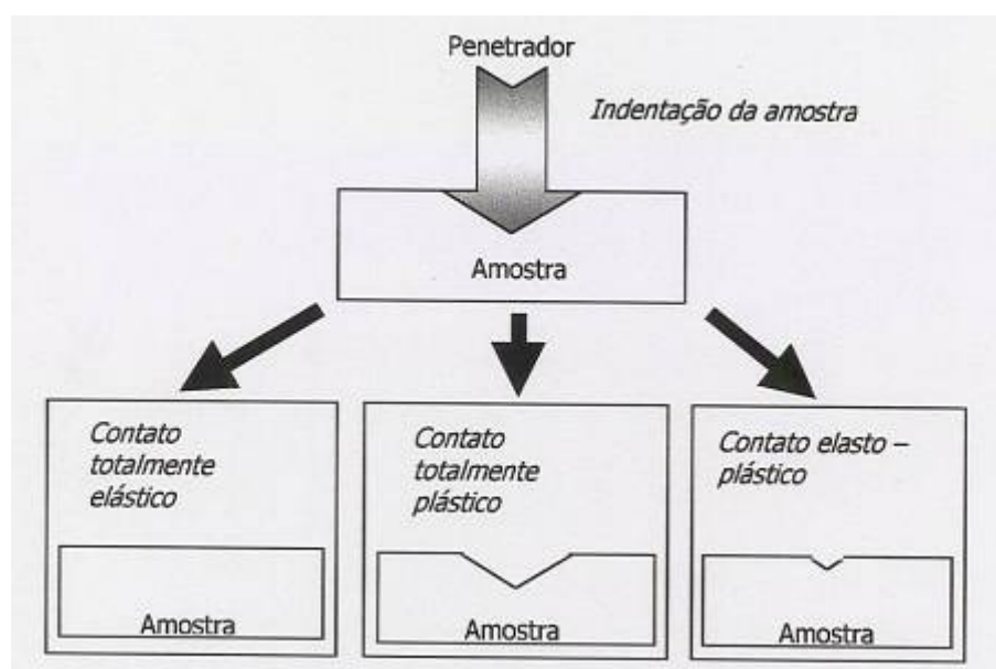
Figura 11: Representação esquemática dos possíveis contatos entre penetrador e amostra.
