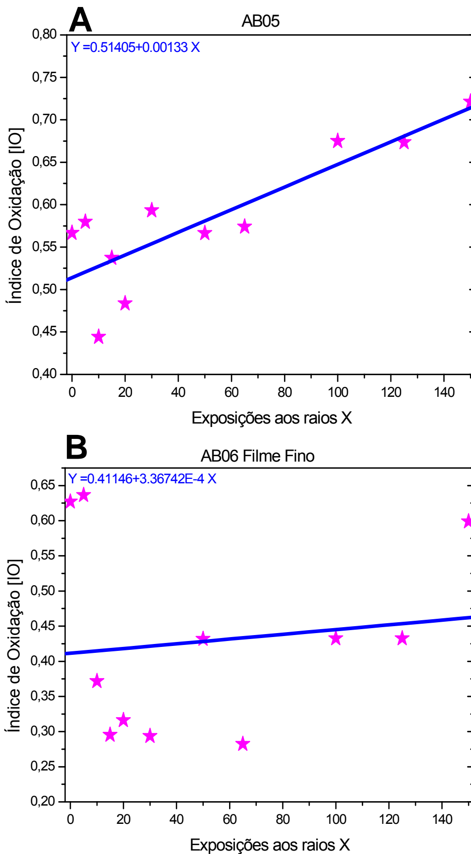
Figura 30: Índice de oxidação (IO) para as amostras irradiadas aos raios X diagnóstico e exposta em ambiente atmosférico. Amostra AB05 (A) ao natural e amostra AB06 (B) com filme fino.
