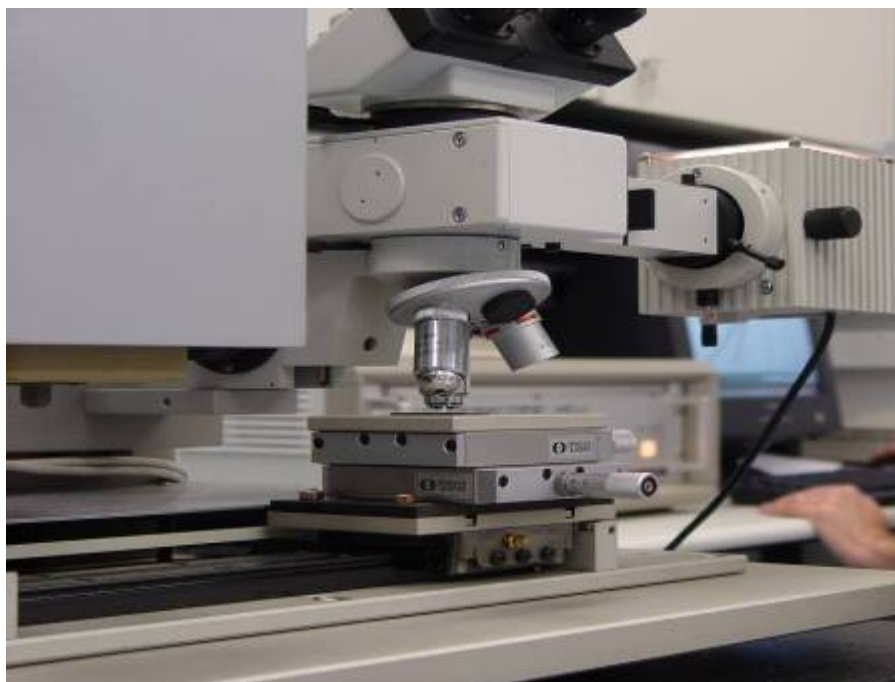
Figura 15: Equipamento utilizado para as análises de dureza.
