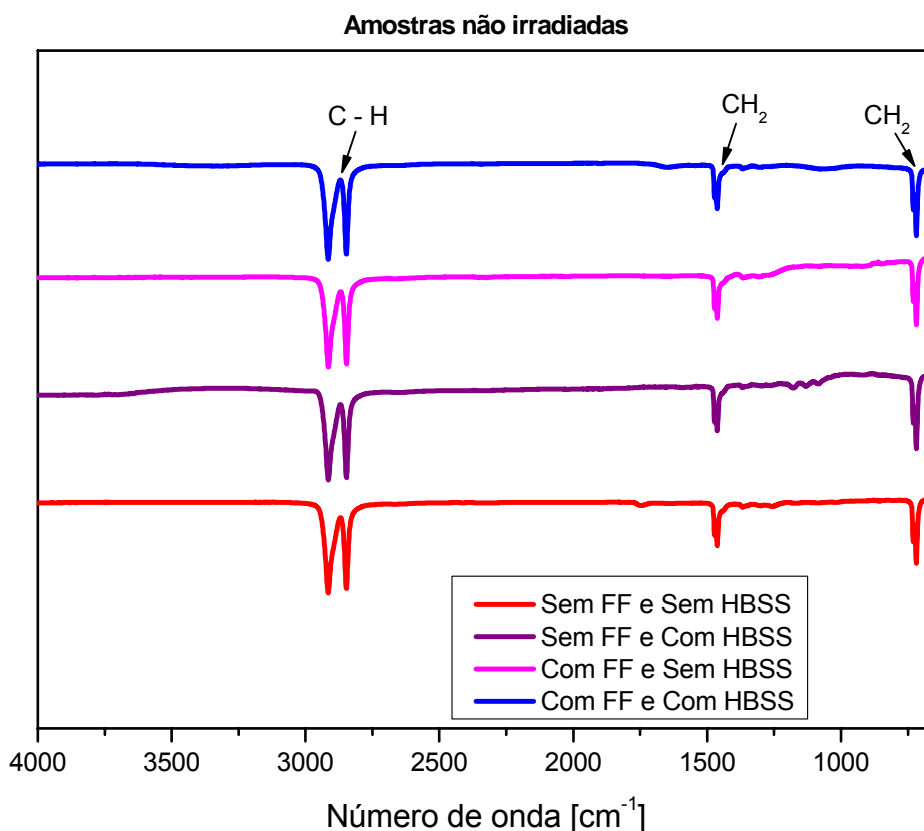
Figura 18: Espectro de FTIR em modo ATR das amostras padrões.
