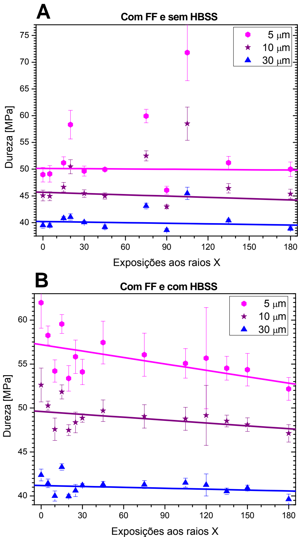
Figura 21: Dureza das amostras revestidas com filme fino de titânio obtidas pelo nano-indentador.
