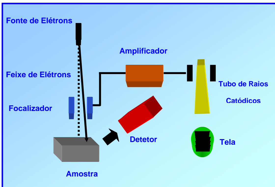
Figura 8: Esquema do Microscópio Eletrônico de Varredura (MEV).
