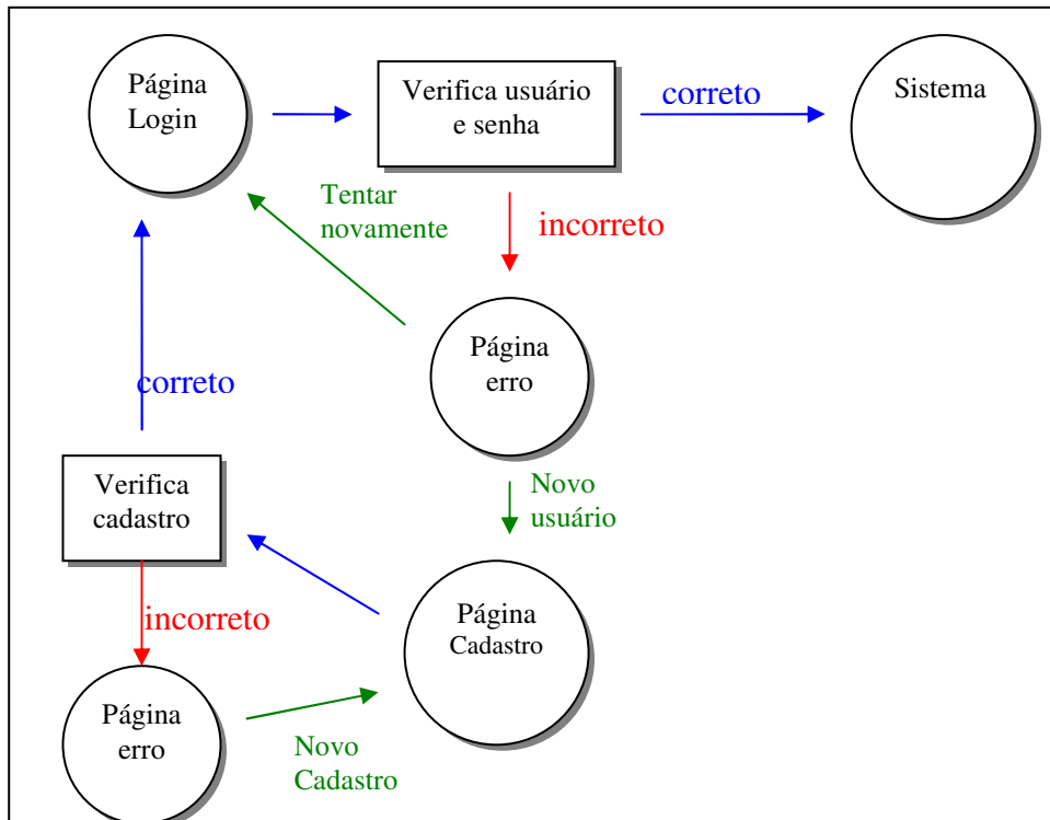
Figura 6 1 - Diagrama do Sistema de Cadastro e Login.
