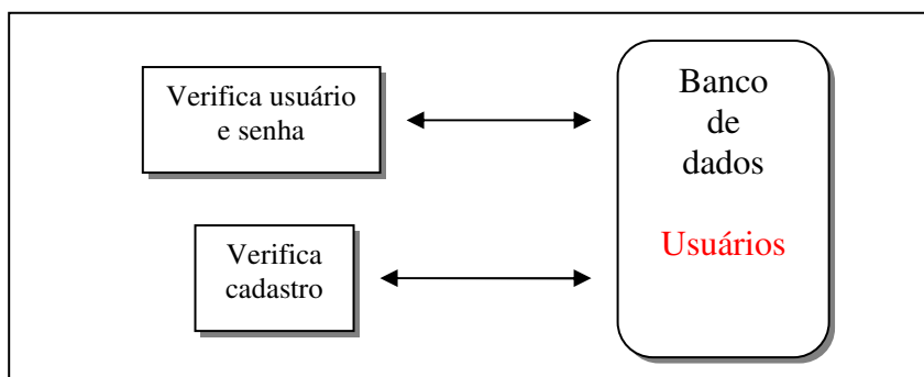
Figura 6 2 - Conexão do Sistema de Login com o banco de dados.
