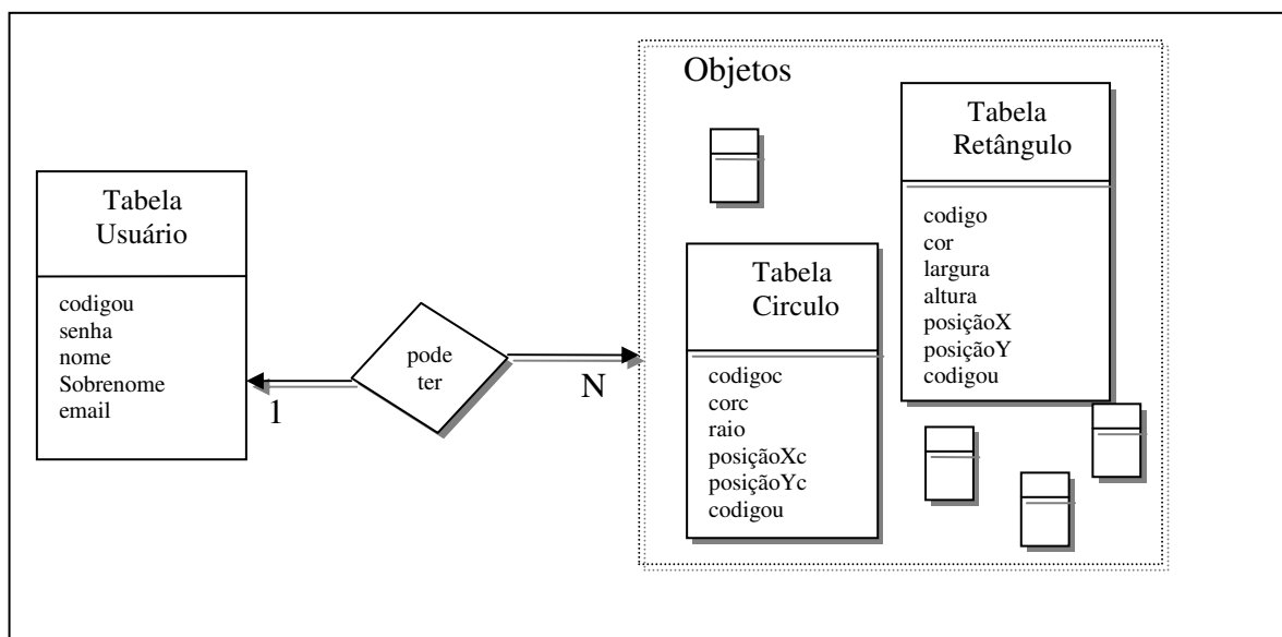
Figura 6 7 - Diagrama da relação entre as tabelas do banco de dados.
