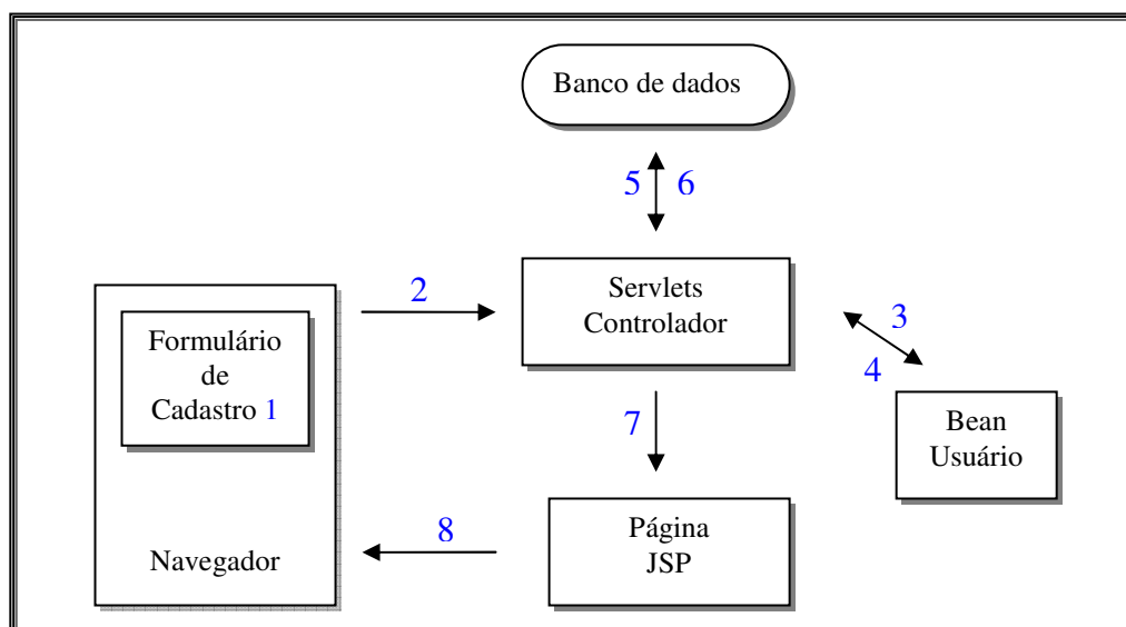
Figura 6 3 - Modelo para Cadastro de usuários
