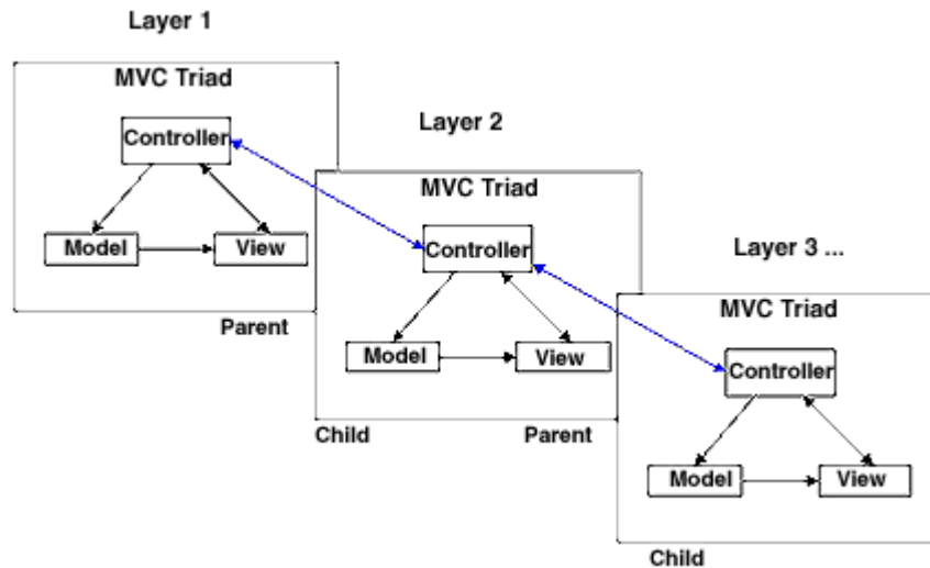
Figura 4 16 -Arquitetura da camada HMVC.
