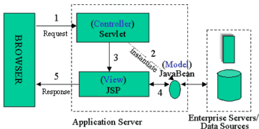
Figura 4 12 - Funcionamento do modelo MVC 2.
