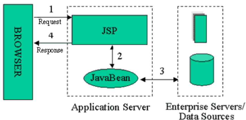
Figura 4 11- Funcionamento do modelo MVC 1.
