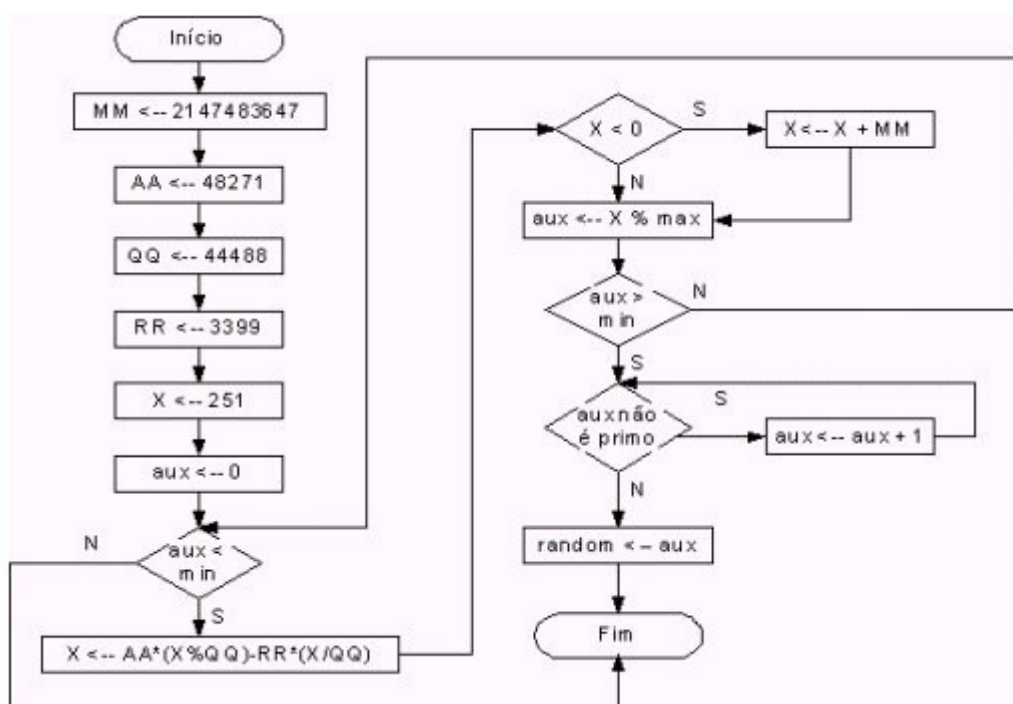
Figura 34 - Esquema do Gerador de N meros Aleatórios.
