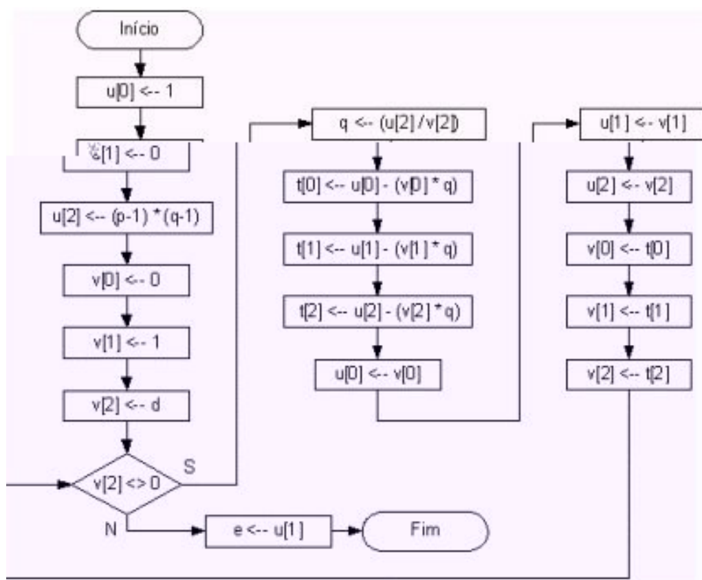
Figura 35 - Algoritmo de Euclides Estendido.
