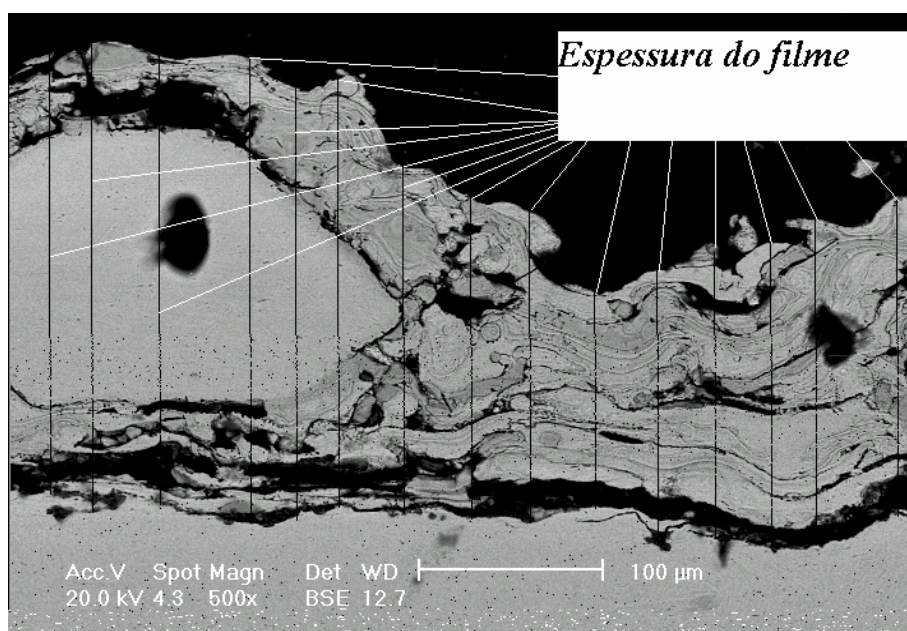
Figura 18: Procedimento utilizado para medir a espessura do revestimento. Magnificação 500 x em SEM
