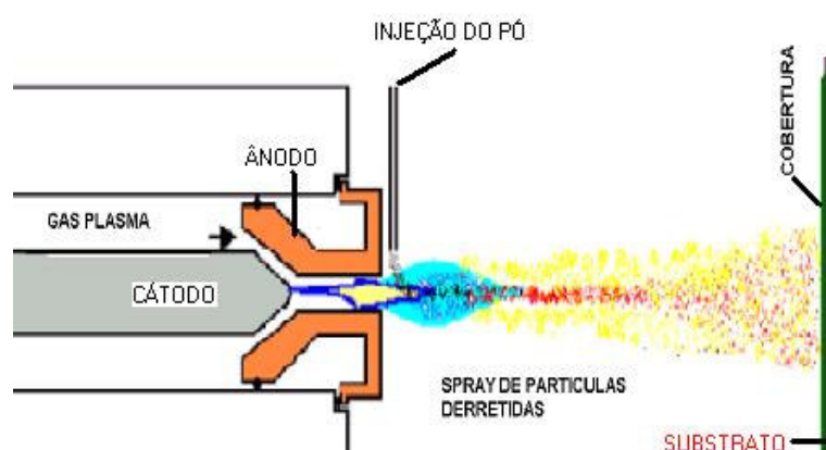
Figura 4: Processo de plasma spray (PS), cobertura de partículas fundidas sobre um substrato. Fonte: (33)
