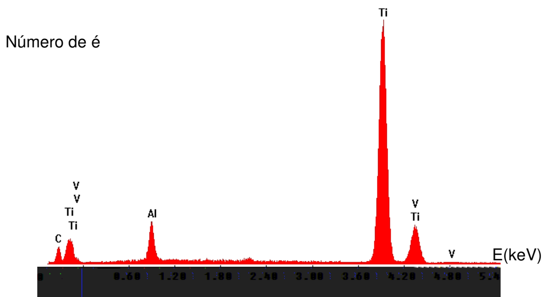
Figura 36: Detalhe do espectro de EDS obtido da região central da haste. A análise foi feita com energia de 20 keV.
