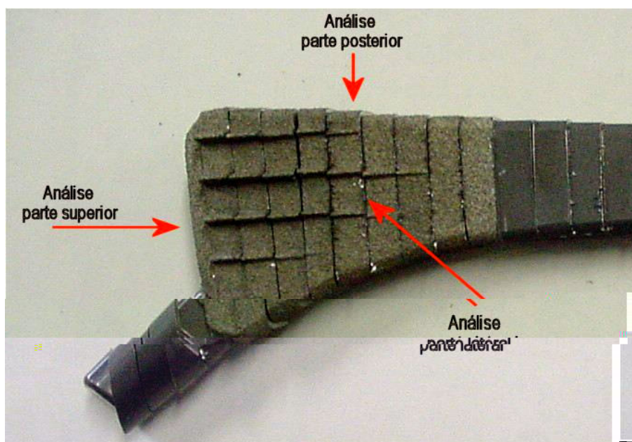
Figura 30: Fotografia da prótese não cimentada, após o corte. As setas indicam as posições das regiões de análise.
