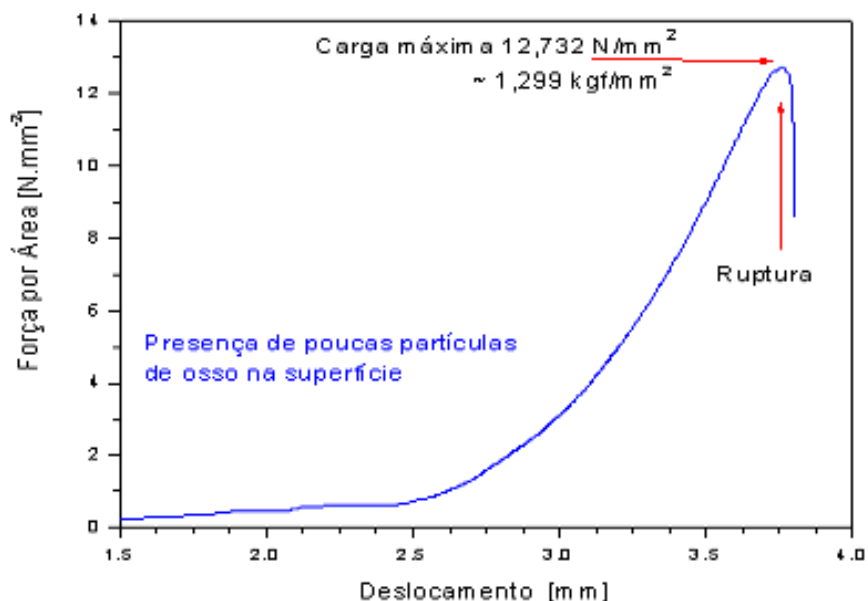
Figura 23: Comportamento adesivo do material poroso ao metal base.
