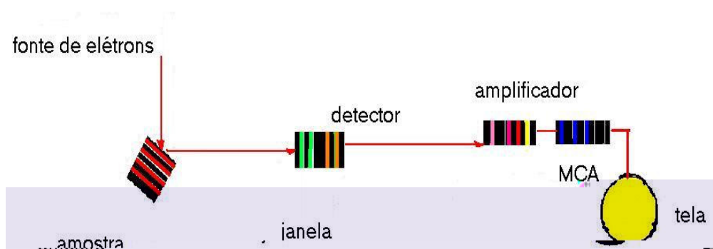
Figura 10: Esquema de funcionamento do EDS.
