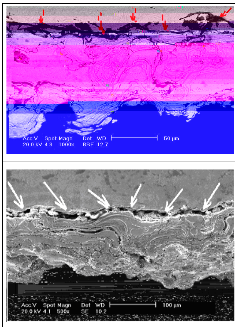
Figura 25: Amostras do grupo (c) com o revestimento sem fusão ao substrato. Magnificações de 1000 x e 500 x em SEM.
