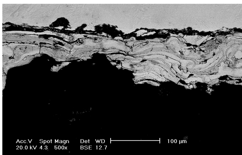
Figura 35: Micrografia da secção transversal do implante de quadril na região onde foi aplicado revestimento PS. Magnificação 500 x em SEM.
