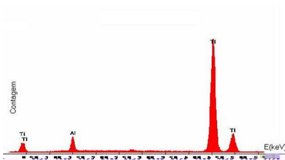
Figura 40: Espectro de EDS do revestimento, contagens em função da energia em n3 da figura 39.
