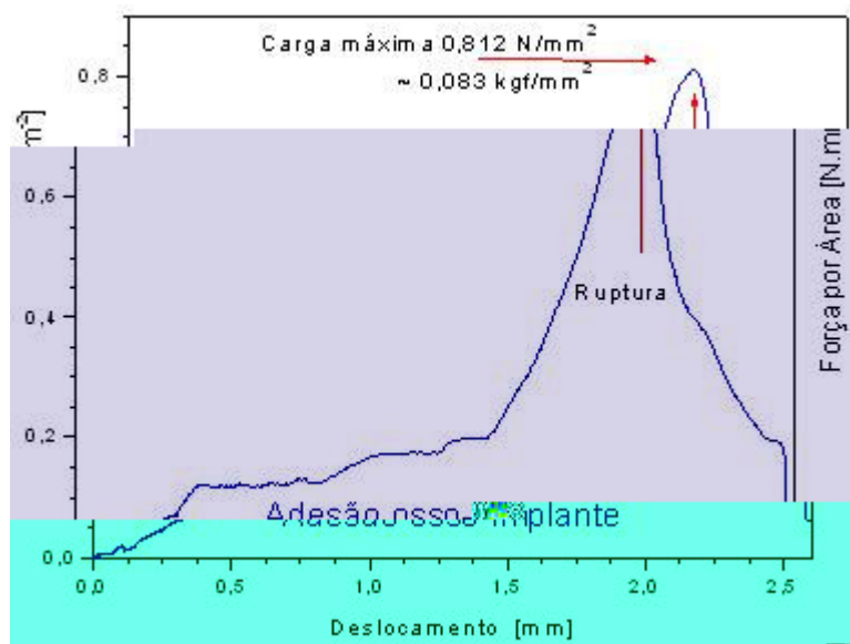
Figura 29: Adesão do osso ao implante, implantado por tempo indefinido.
