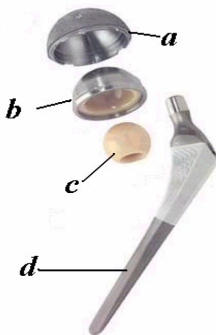
Figura 5: Prótese de quadril: (a) acetábulo, (b) componente cerâmico, (c) cabeça cerâmica (esfera), (d) haste (cimentada). Trident ®. Fonte: (42)
