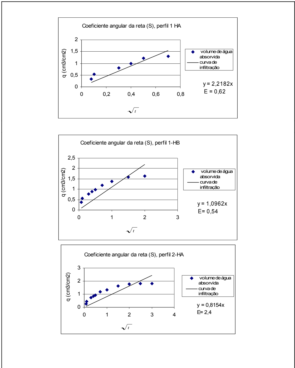
Figura 1- Gráficos de determinação dos coeficientes angulares para o cálculo de erodibilidade (E) dos horizontes A e B dos perfis de solo 1 e 2
