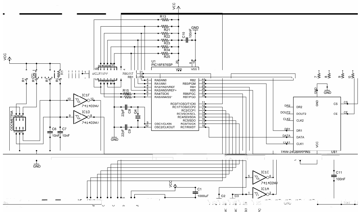
Figura 5.12 – Esquema elétrico da placa de controle do robô Cube 3
