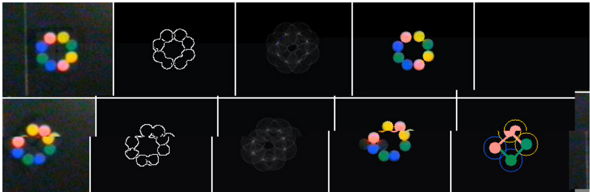
Figura 5.7 – Caso especial em que o sistema pode não detectar os robôs
