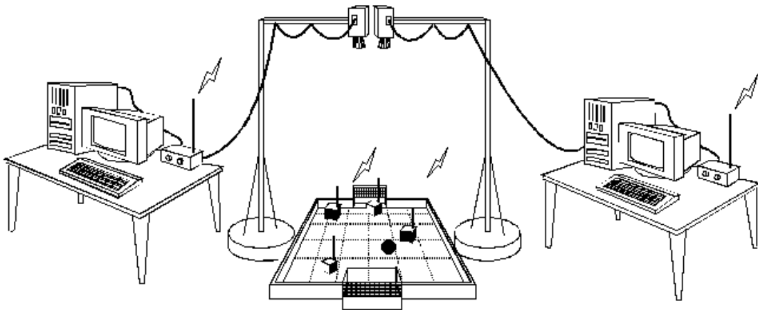
Figura 4.2 – Arquitetura proposta pela FIRA para a categoria Mrosot Le 'u e
