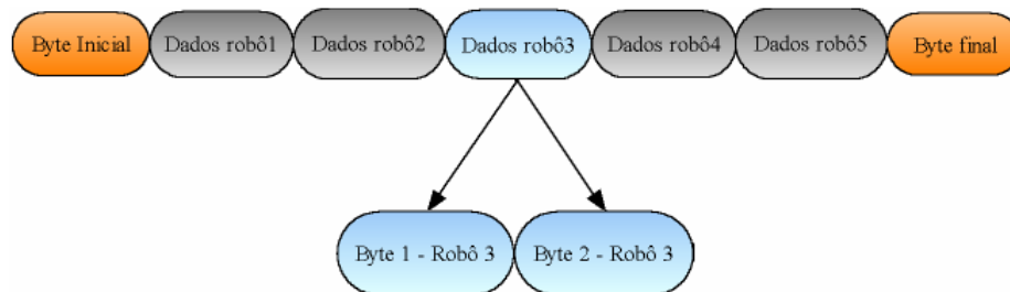
Figura 5.11 – Pacote de dados do protocolo proposto
