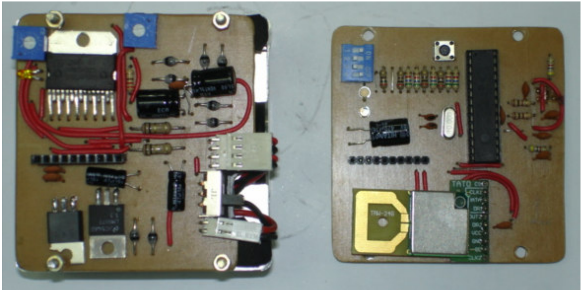
Figura 5.14 – Placas de potência (à esquerda) e controle (à direita) dos robôs Cube 3
