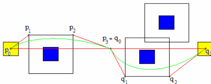
Figura 5.9 – Trajetória com descontinuidade entre as curvas de Bezier
