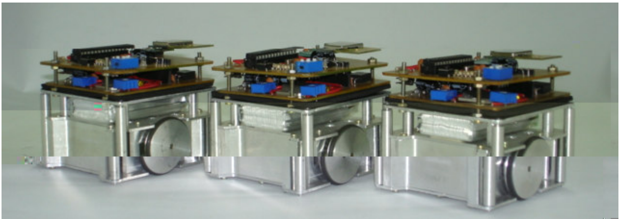
Figura 5.15 – Os robôs Cube 3
