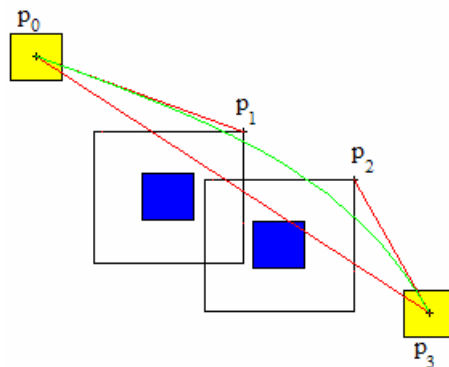
Figura 5.8 – Curva de Bezier de grau cúbico
