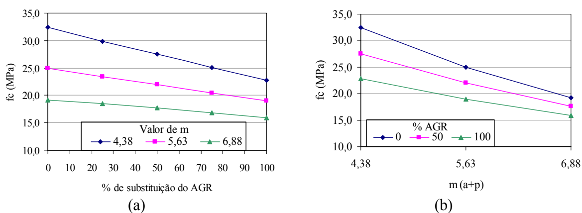
Figura 32: resistência à compressão em função da interação m \times AGR: (a) f_c em função de AGR, para os diferentes valores de m ; (b) f_c em função de m , para os diferentes teores de AGR
