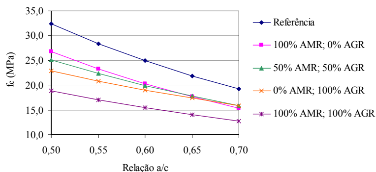
Figura 38: curvas de resistência à compressão em função da relação a/c
