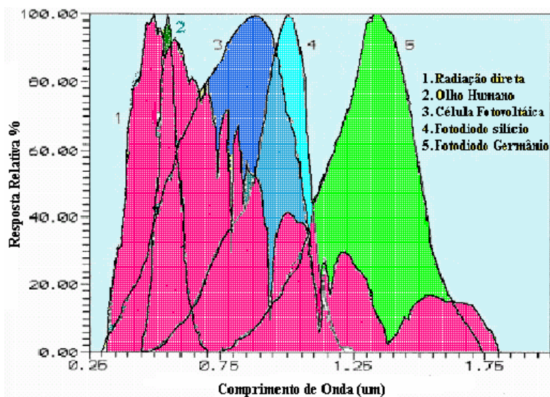
Figura 13 Espectro solar e faixas de detecção (adaptado de Rocha, 1992)
