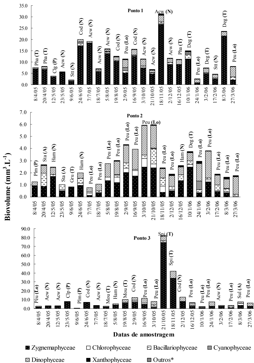
Figura 13. Biovolume acumulado (mm 3 .L -1 ) e espécies dominantes da comunidade fitoplancônica ( Pha = Phymatodocis alternans , Clg = Closterium cf. gracile , Acw = Actnotaeonium wollei , Stt = Staurodesmus triangularis , Cod = Cosmarium denticulatum , Peu = Peridinium umbonatum , Deg = Desmidium cf. graciliceps , Plm = Pleurotaenium minutum , Sta = Stauroneis sp, Ham = Haplotaenium minutum , Gru = Groenbladia undulata , Clp = Closterium cf. parvulum , Mou = Mougeotia sp., Spi = Spirogyra sp., Sul = Surirella linearis ) e os respectivos grupos funcionais (N, Lo, T, P, e A) em três pontos amostrais na Lagoa Bonita entre abril/2005 e março/2006. *Outros: Chrysophyceae e Cryptophyceae.
