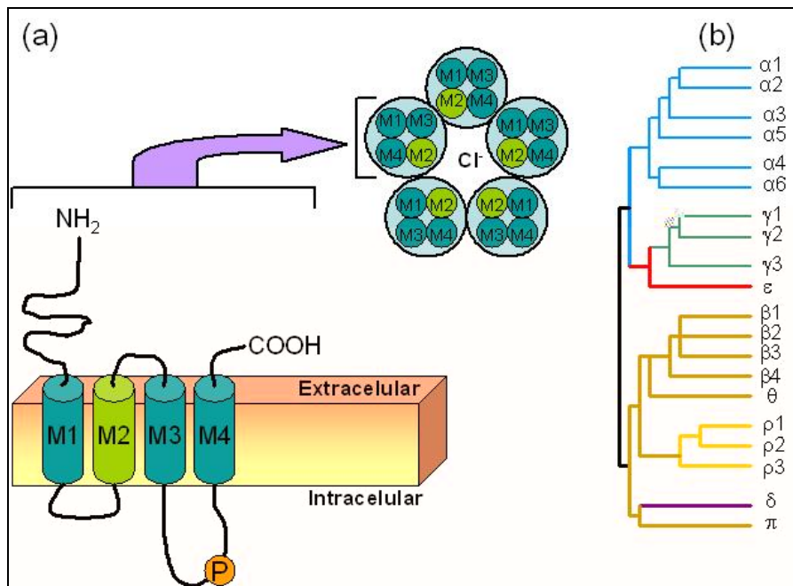
Figura 2 - Estrutura de cada subunidade que compõe o receptor GABA A , destacando-se os quatro domínios transmembrânicos (M 1 , M 2 , M 3 e M 4 ), a porção N e C-terminal extracelularmente e alça citoplasmática intracelularmente (a), e as diferentes subunidades do receptor GABA A clonadas e seqüenciadas até o momento (b). Fonte: Adaptado de Whiting et al., 1999.
