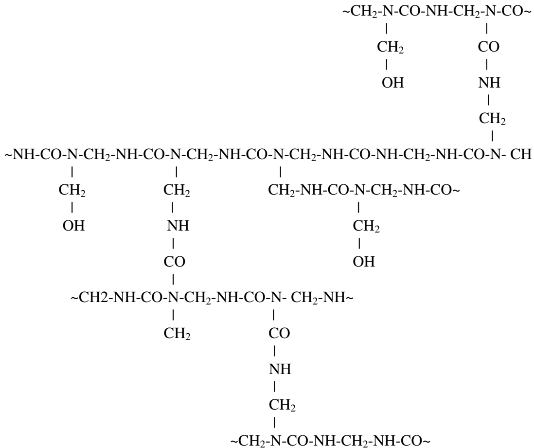
Figura 4.3 – Ligações cruzadas da resina uréia formaldeído.
