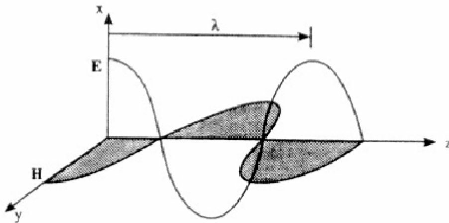
Figura 6.1 – Representação gráfica de um campo eletromagnético (Committee on Microwave Processing of Materials, 1994)
