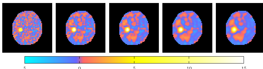
Figura 7.3: Mapas contendo uma área de atividade simulada com raio 10 mm e com sinal BOLD com amplitude de 0,9%, cujas séries temporais foram suavizadas com filtros de largura variável. Da esquerda para a direita, respectivamente: sem suavização, 1,5, 2,0, 2,5 e 3,0 voxels de largura.
