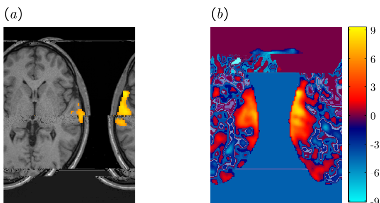
Figura 2.9: Resultado de um experimento de fMRI. Os mapas estatísticos podem ser limiarizados e apresentados sobrepostos à uma imagem estrutural de alta resolução (a), ou exibidos diretamente (b). A limiarização facilita a interpretação do resultado, mas despreza informações potencialmente relevantes.
