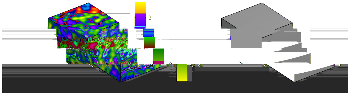
Figura 4.3: Um campo aleatório tipo Gaussiano tridimensional ( esquerda ). Neste exemplo, as variáveis aleatórias preenchem todo o espaço delimitado pelo campo, como pode-se observar sem o código de cores ( direita ).
