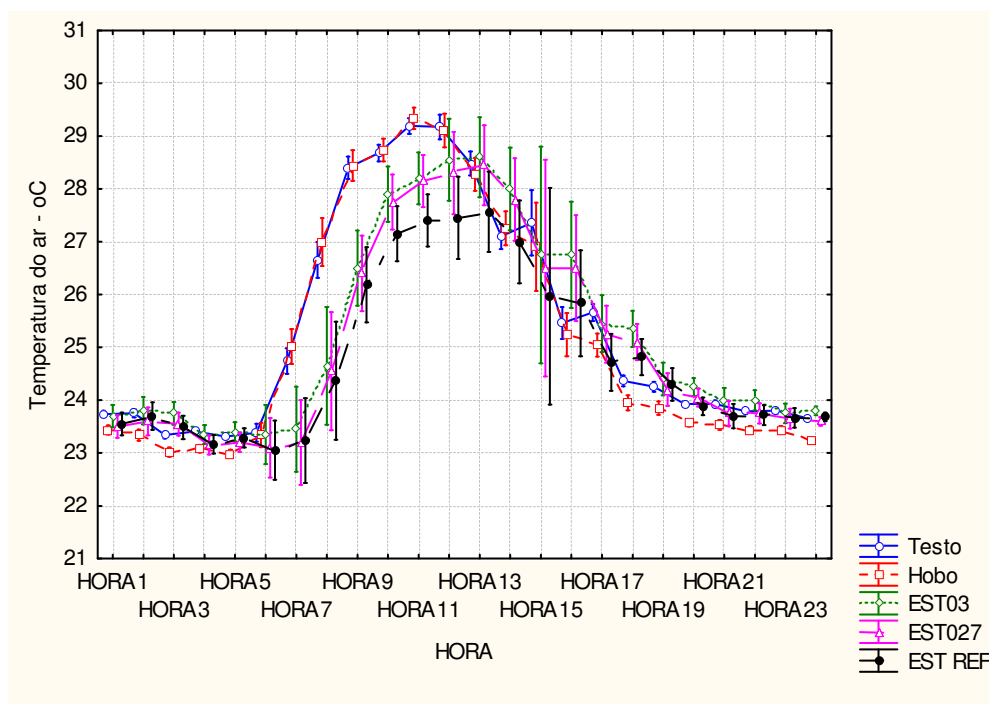
Figura 5.11 – Gráfico da temperatura do ar média por marca de equipamento no período de inverno
