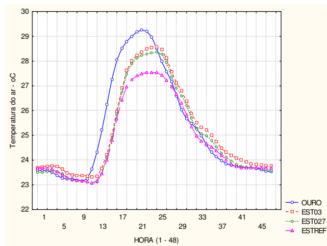
Figura 3 - Curvas de calibração para os equipamentos da marca estação Davis – verão
