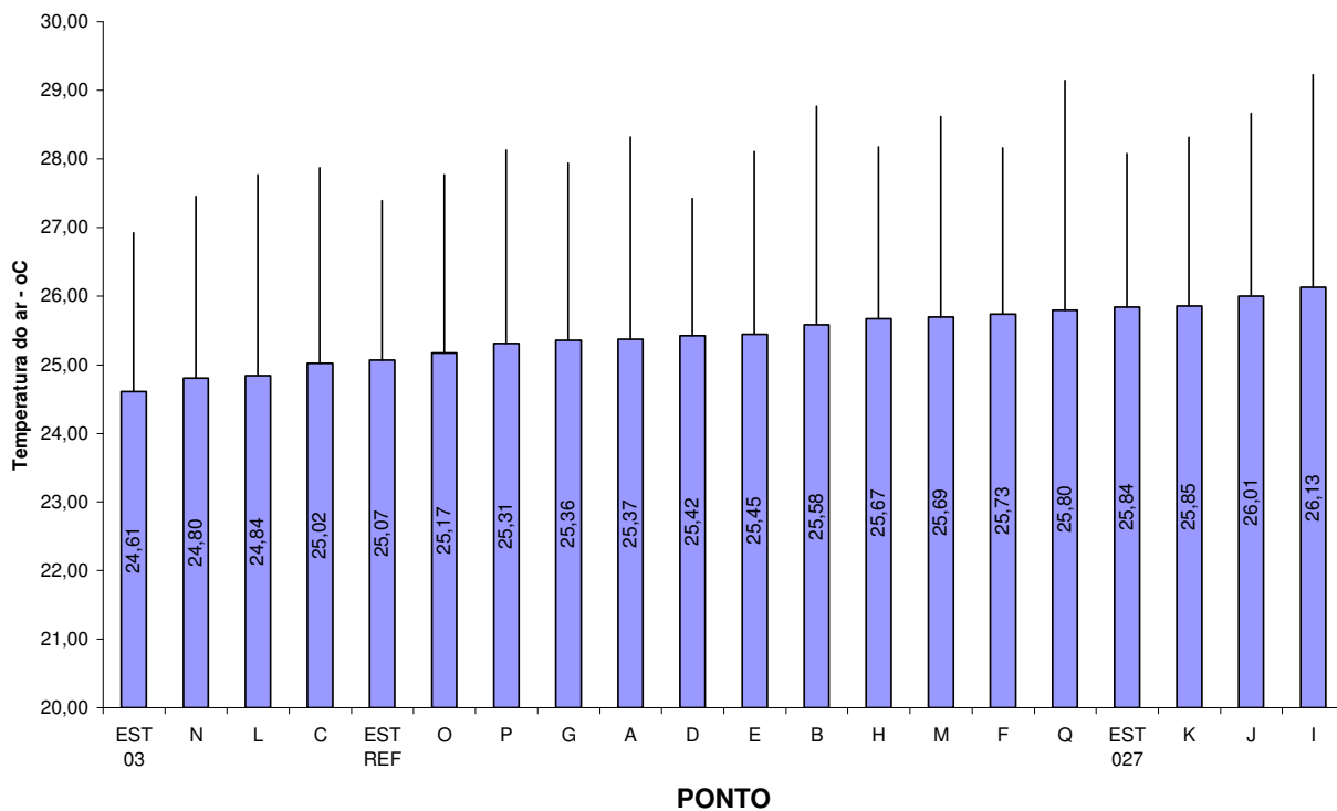
Figura 7.19 – Gráfico da Temperatura do ar média nos pontos de forma ordenada.
