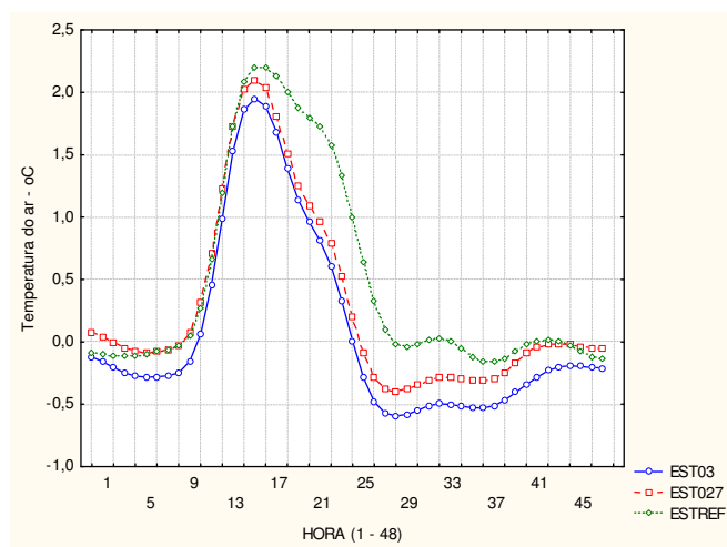
Figura 4 - Curvas de calibração para os equipamentos da marca estação Davis – inverno
