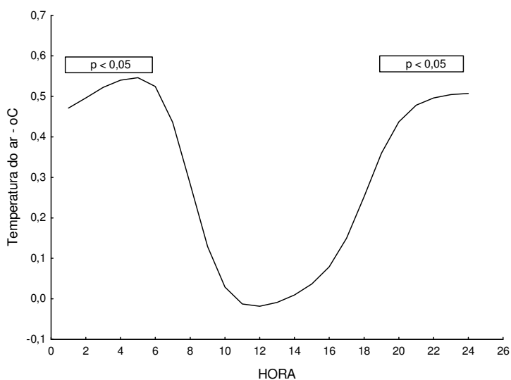
Figura 8.1 - Curva de correlação entre a temperatura do ar e o ICR – Verão
