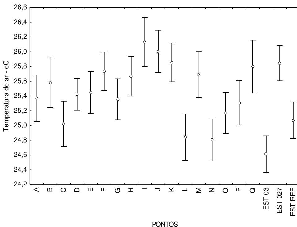
Figura 7.17 – Gráfico com comportamento médio da temperatura do ar para um intervalo de confiança de 95%, por ponto de coleta no período de inverno.
