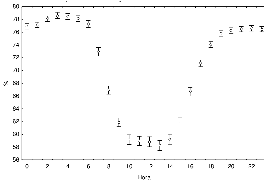
Figura 7.10 – Gráfico do comportamento médio da umidade relativa do ar
