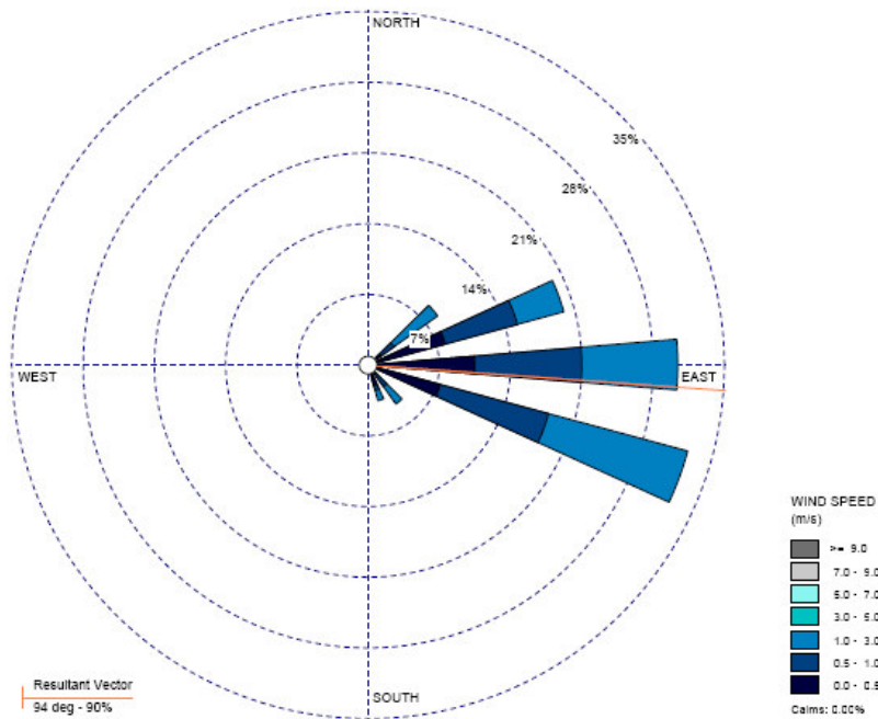
Figura 7.14 – Gráfico tipo rosa dos ventos para o ponto EST027
