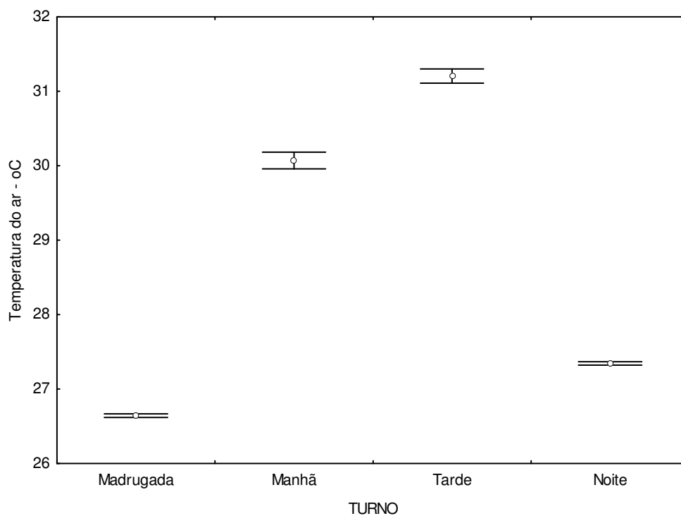
Figura 7.11 – Gráfico do comportamento médio da temperatura do ar por turno, com intervalo de confiança de 95%.
