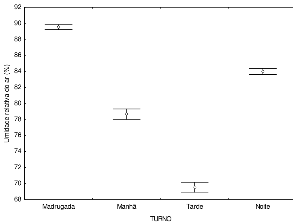
Figura 7.28 – Gráfico do comportamento médio da umidade relativa d ar por turno, com intervalo de confiança de 95%.
