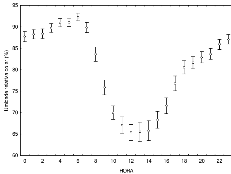
Figura 7.26 – Gráfico do comportamento médio da umidade relativa do ar, ao longo do dia
