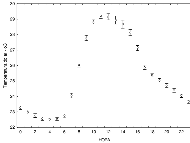
Figura 7.25 – Gráfico do comportamento médio da temperatura do ar, ao longo do dia
