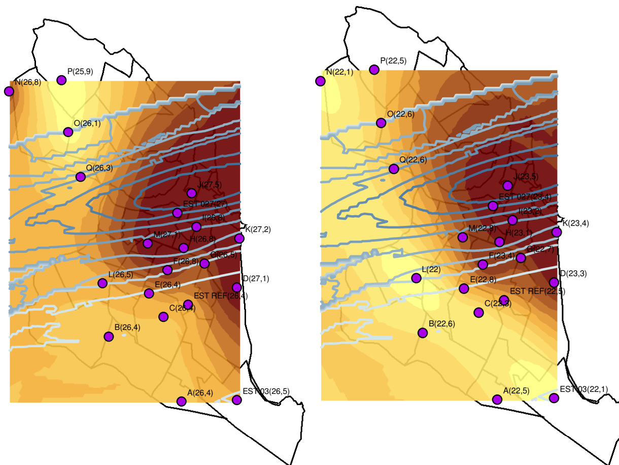
Figura 8.6 – Mapas resultantes da krigagem entre a temperatura média do ar no turno da madrugada e o índice calculado ICR para os 20 pontos de coleta – período de verão e inverno.
