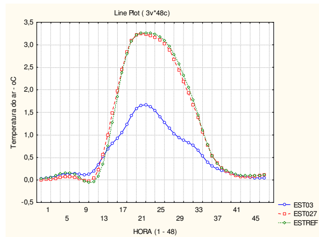
Figura 2 - Curvas de correção para o verão, por marca de instrumento
