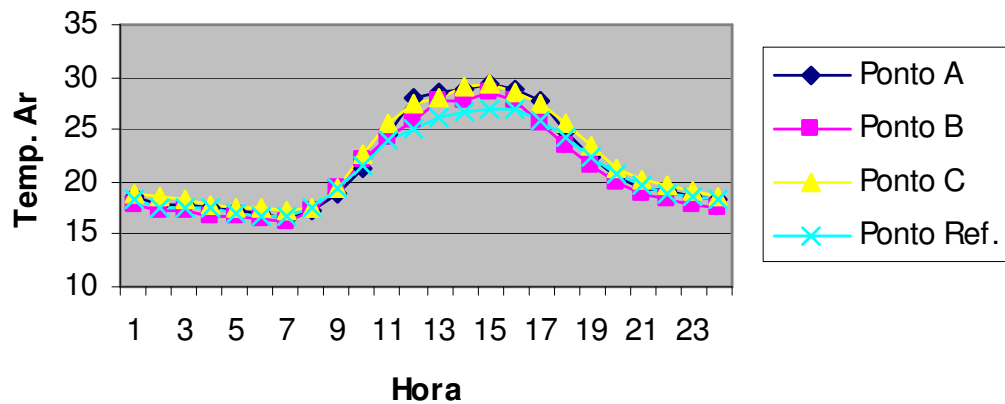
Figura 5.5 – Gráfico do comportamento médio diário da temperatura do ar para os 04 pontos medidos.
