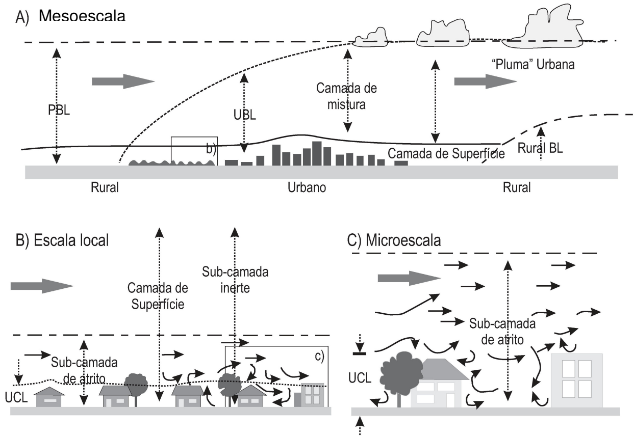
Figura 3.1 – Esquema das escalas climáticas
