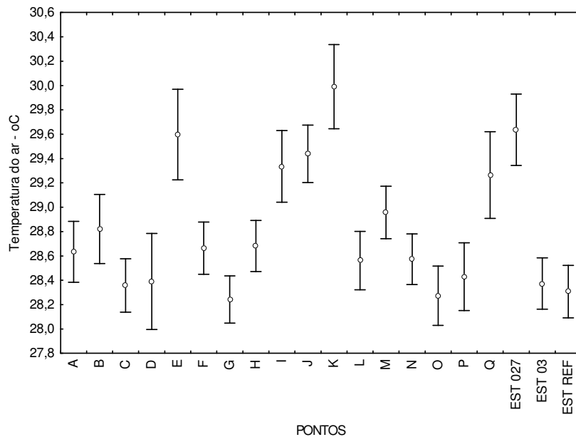
Figura 7.1 – Gráfico com comportamento médio da temperatura do ar para um intervalo de confiança de 95%, por ponto de coleta no período de verão.
