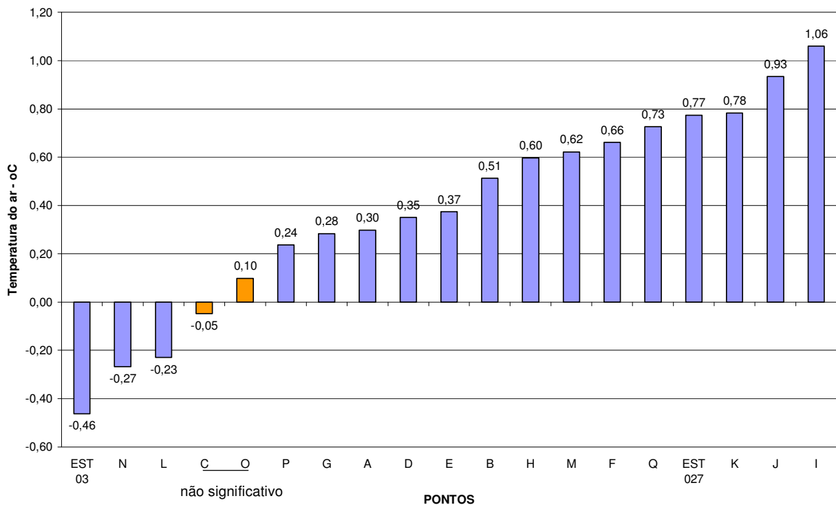
Figura 7.33 - gráfico com diferenciais de temperatura do ar dos pontos em relação ao ESTREF em ordem crescente para o período de inverno.
