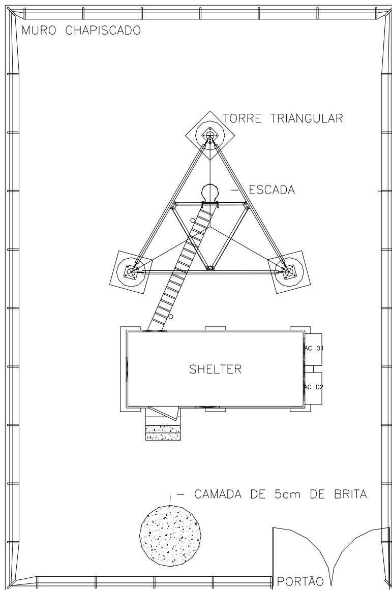
PLANTA BAIXA – SITE s/ESCALA
