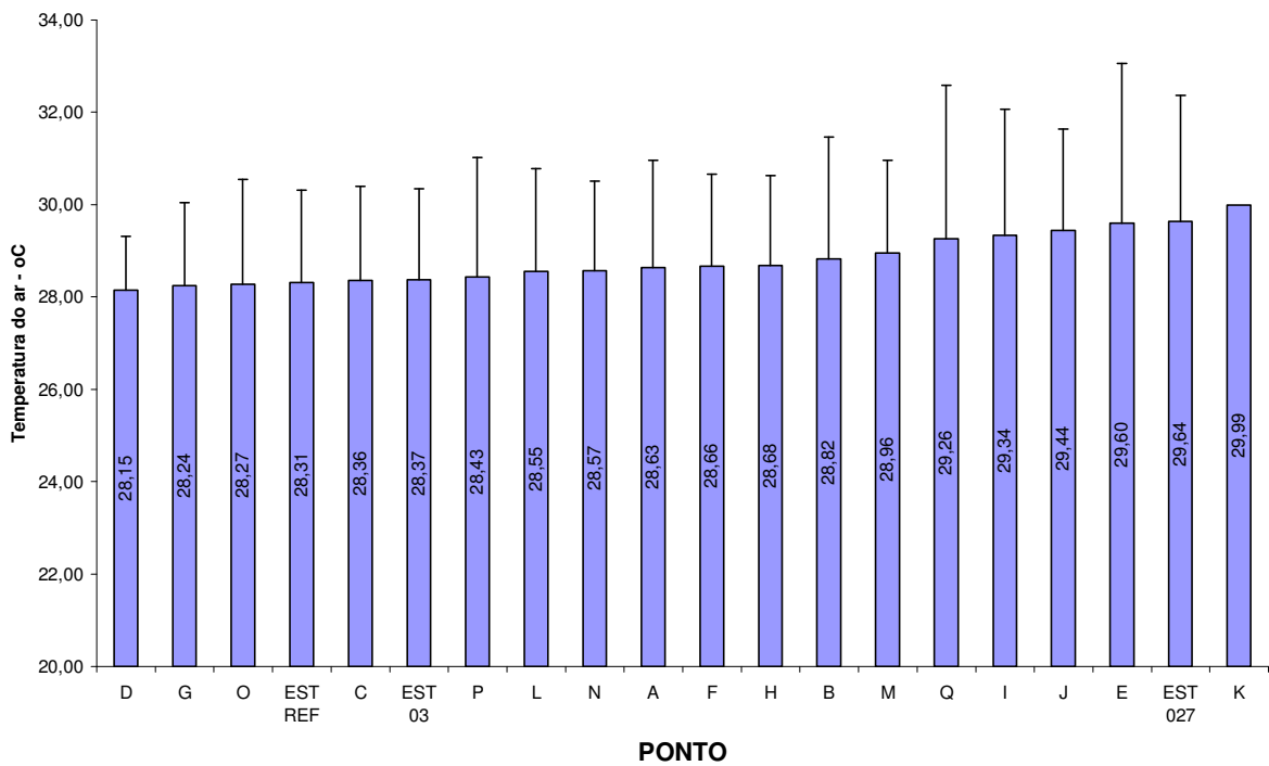
Figura 7.3 – Gráfico da Temperatura do ar média nos pontos de forma ordenada
