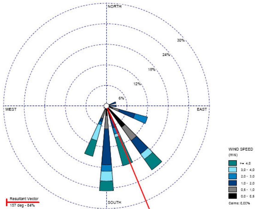
Figura 7.31 – Gráfico do tipo Rosa dos ventos para a média entre os pontos EST03 e EST027.
