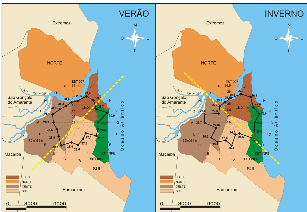
Figura 7.39 – Mapas estrela resultantes da análise de campo, com as médias gerais por ponto, por período.
