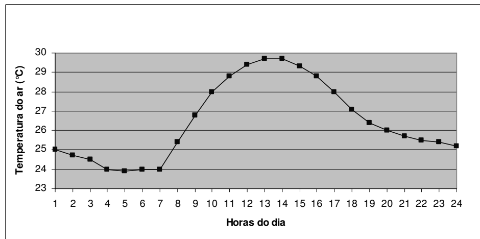
Figura 4.3 – Gráfico do comportamento do Dia Típico da temperatura do ar para Natal
