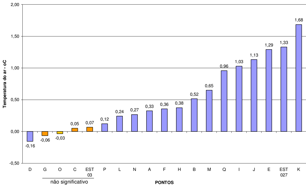
Figura 7.32 – Gráfico dos diferenciais de temperatura do ar dos pontos de coleta em relação ao ponto de referência em ordem crescente.
