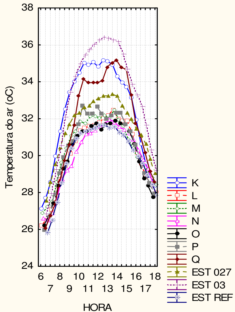
Figura 7.7 – Gráficos da temperatura do ar média no intervalo 6h-18h nos pontos de coleta
