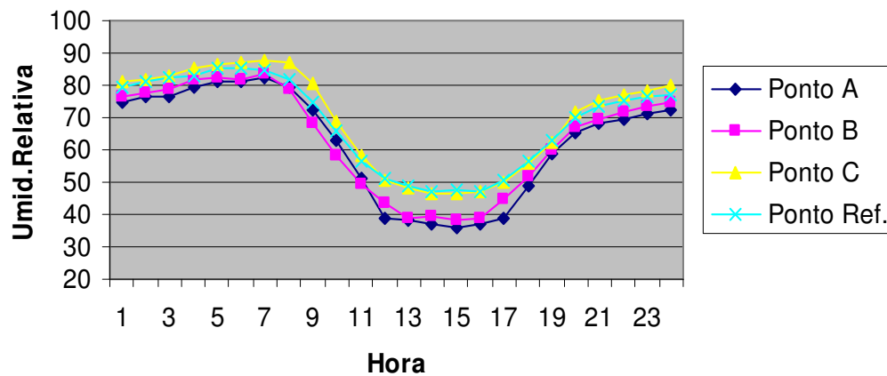
Figura 5.6 - Gráfico do comportamento médio diário da umidade relativa do ar para os 04 pontos medidos.
