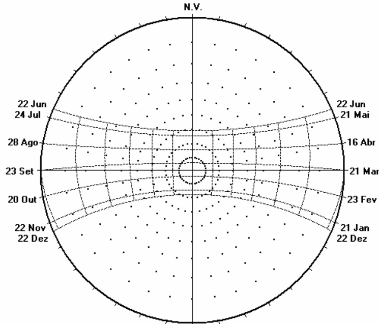
Projeção Estereográfica dos Percursos Aparentes do Sol - Latitude=-5,45
