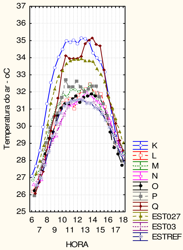
Figura 7.23 – Gráficos da Temperatura do ar horária nos pontos no intervalo 6h-18h
