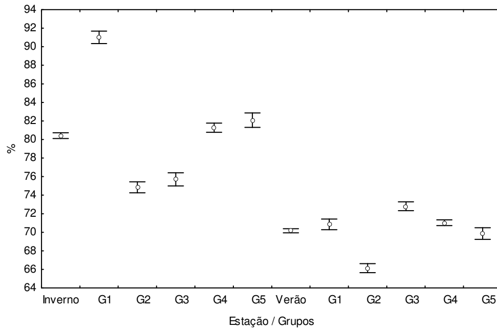
Figura 7.37 – Perfil médio de umidade relativa do ar e intervalos de confiança para grupos homogêneos de pontos nos períodos de verão e inverno
