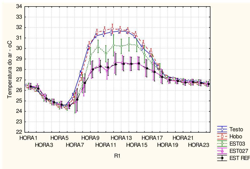
Figura 5.10 – Gráfico da temperatura média do ar horária por marca de equipamento no período de verão
