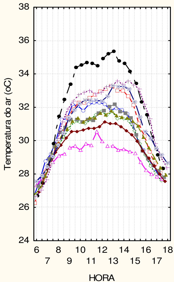
Figura 7.7 – Gráficos da temperatura do ar média no intervalo 6h-18h nos pontos de coleta
