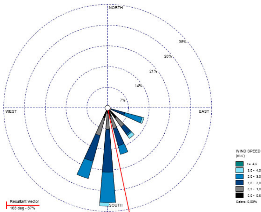
Figura 7.29 – Gráfico tipo Rosa dos ventos para o ponto EST03
