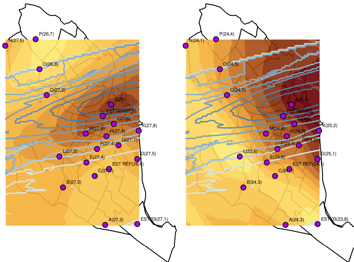
Figura 8.9 – Mapas resultantes da krigeagem entre a temperatura média do ar no turno da noite e o índice calculado ICR para os 20 pontos de coleta – período de verão e inverno.
