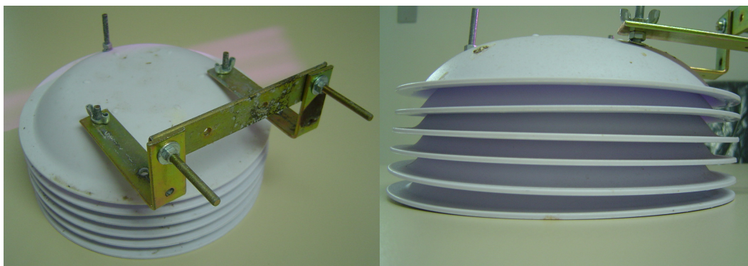
Figura 5.8 – Fotografias das Proteções levemente deformadas e com partes em ferro oxidadas, respectivamente.
