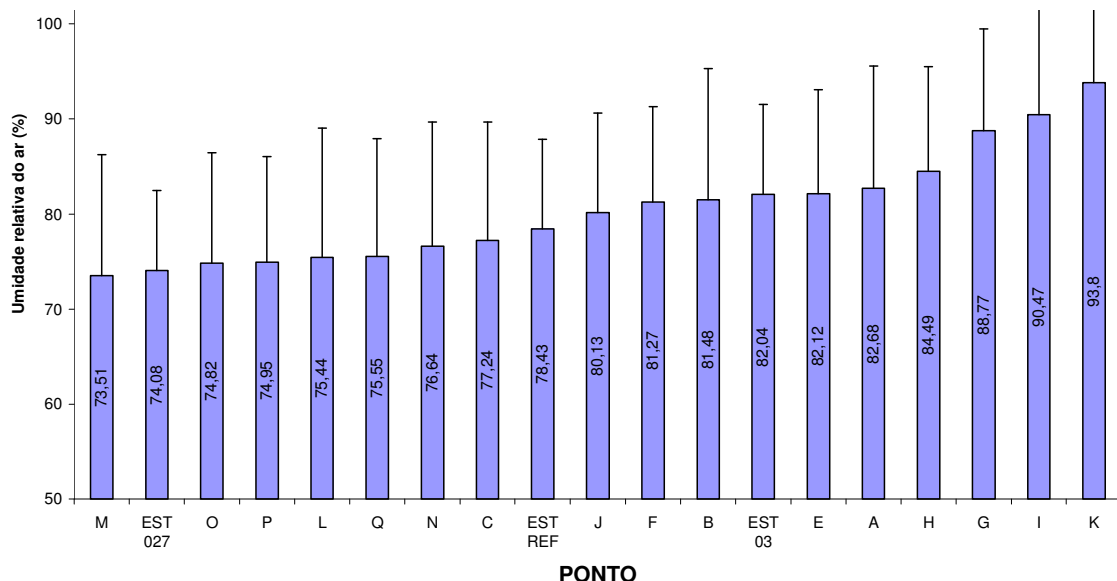
Figura 7.20 – Gráfico da Umidade relativa do ar média nos pontos de forma ordenada.
