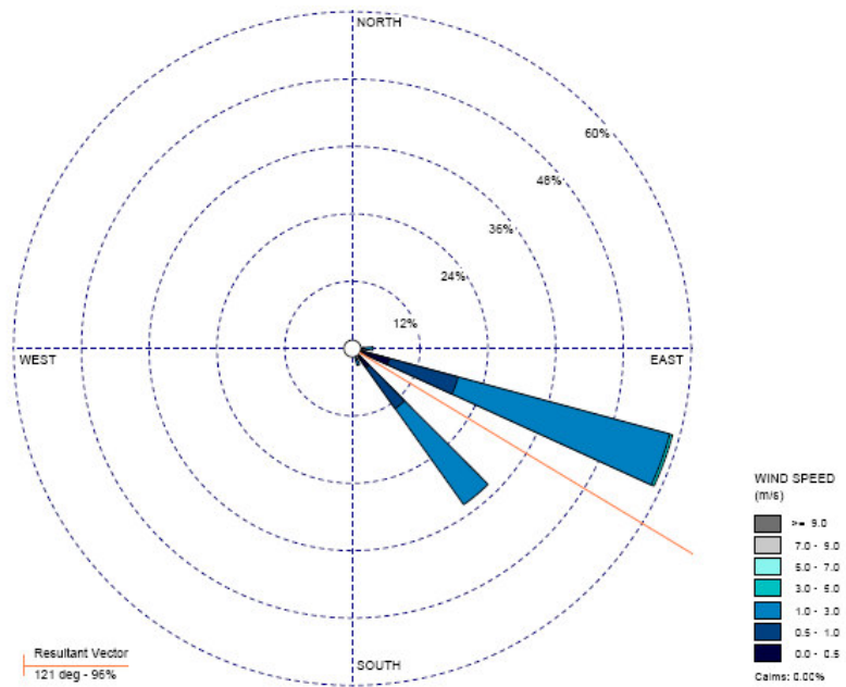
Figura 7.13 – Gráfico tipo rosa dos ventos para o ponto EST03
