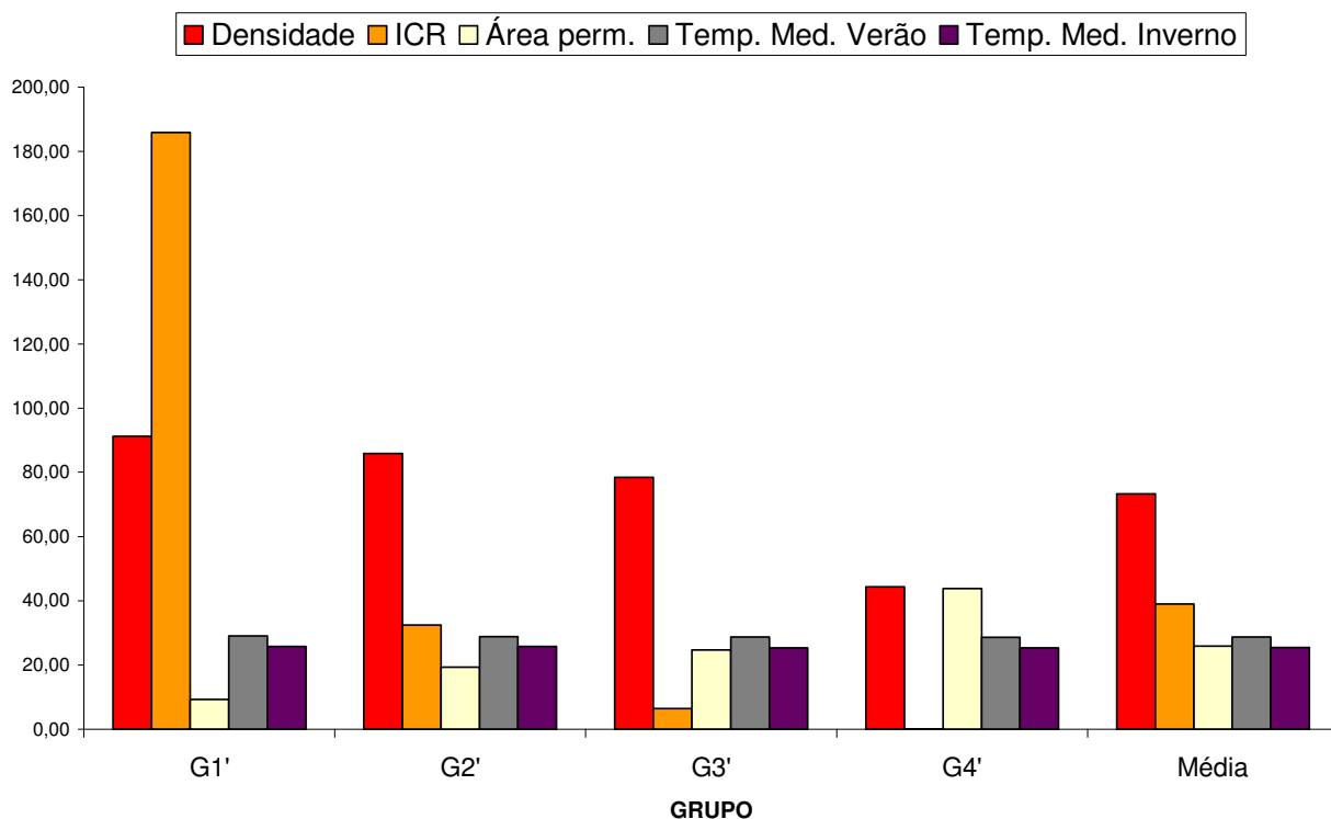
Figura 8.3 – Gráfico do agrupamento segundo os fatores densidade, ICR, área permeável e temperatura do ar média no verão e inverno.
