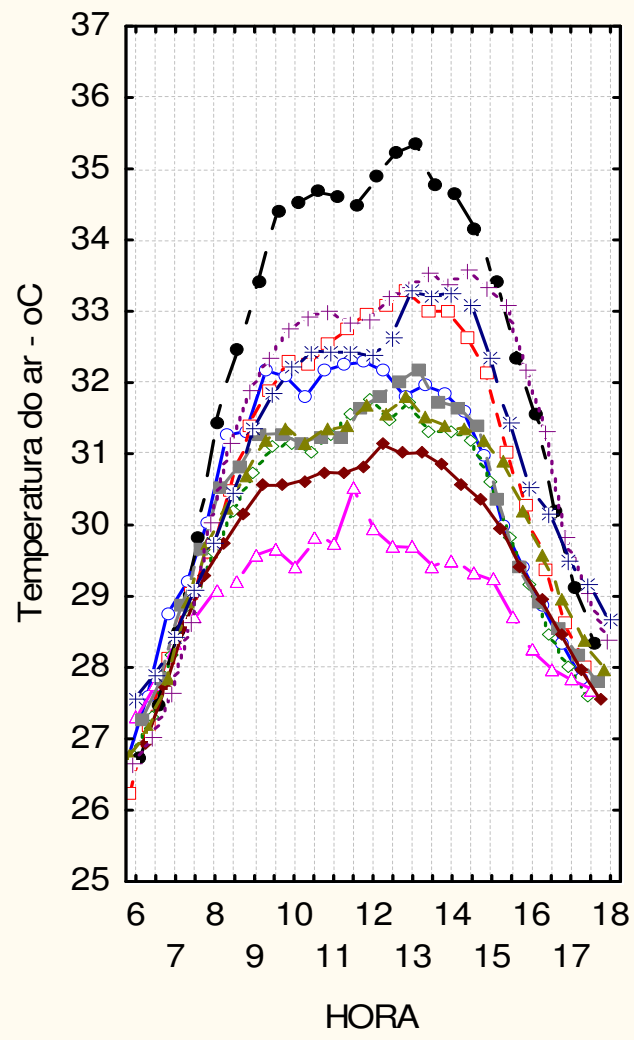
Figura 7.23 – Gráficos da Temperatura do ar horária nos pontos no intervalo 6h-18h
