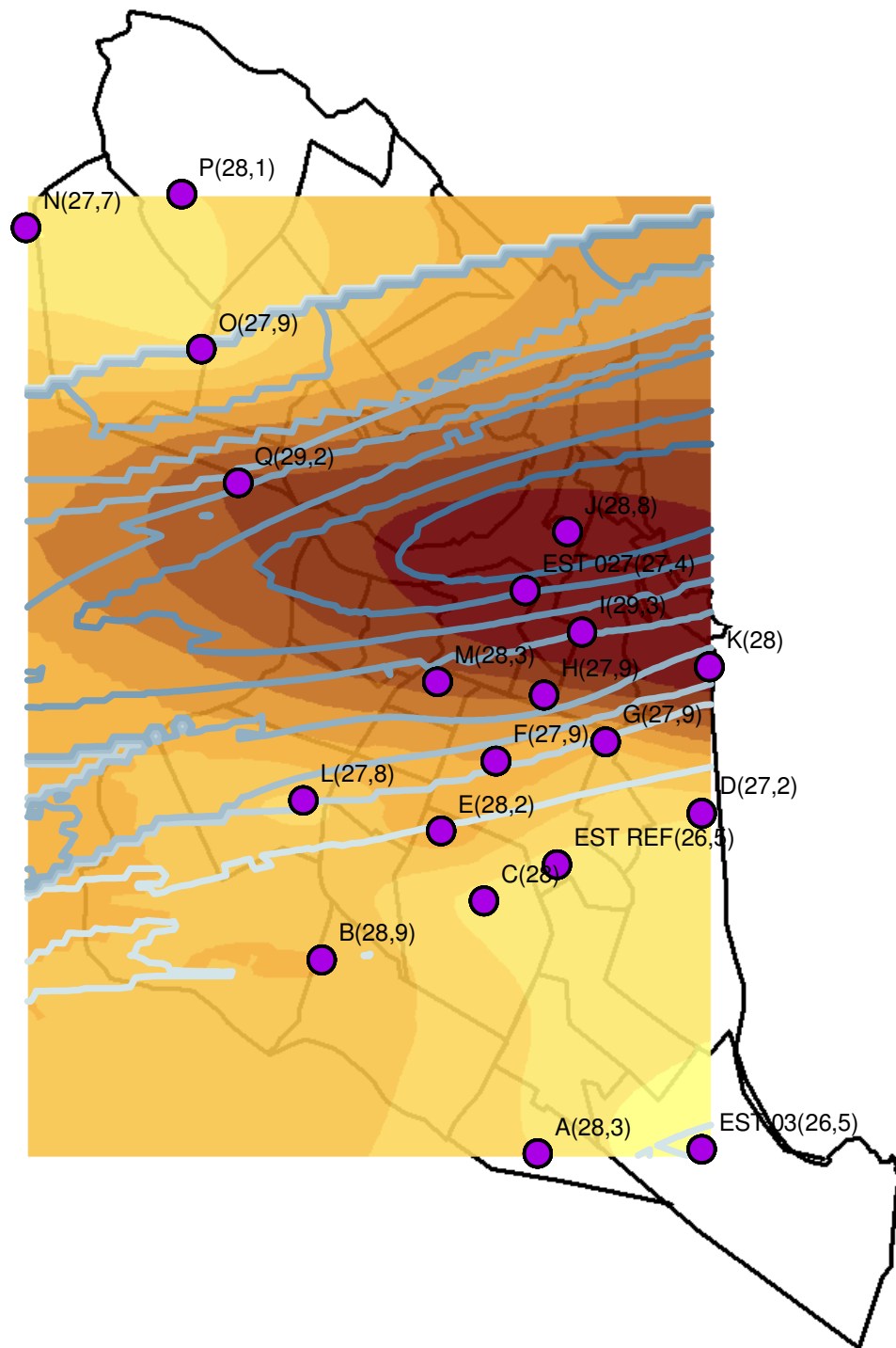
Figura 8.10 – Mapa resultante da krigeagem entre a temperatura média do ar em todos os turnos e períodos, e o índice calculado ICR para os 20 pontos de coleta.
