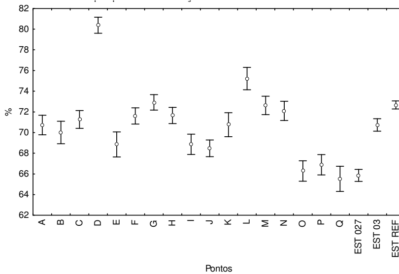
Figura 7.2 – Gráfico com comportamento médio da umidade relativa do ar para um intervalo de confiança de 95%, por ponto de coleta, no período de verão.
