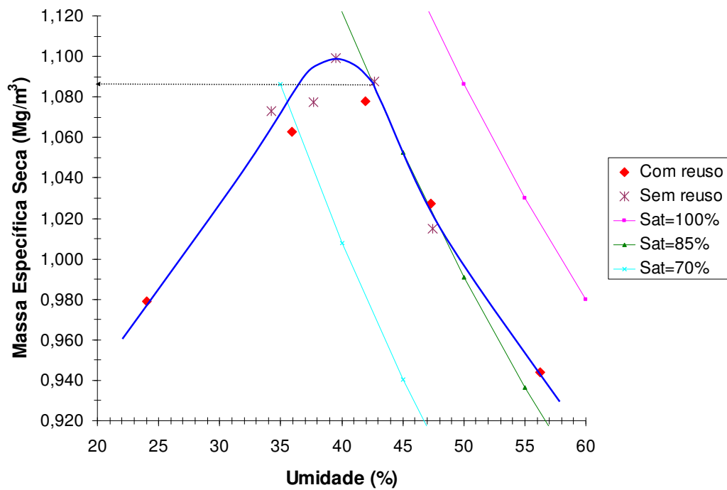
Curva Compactação Proctor Normal M2
