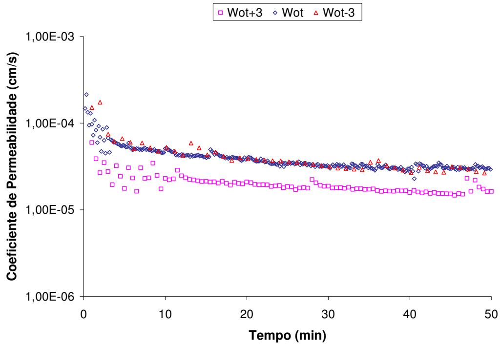
Figura 5.48-Coeficiente de permeabilidade versus tempo para corpos de prova da M3
