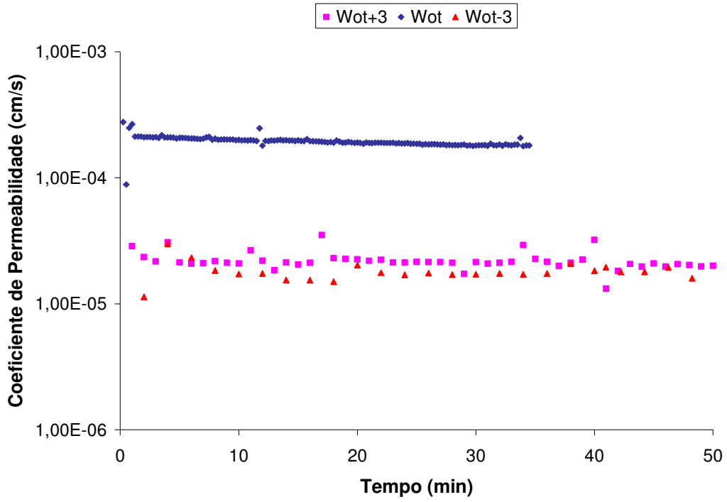
Figura 5.44-Coefficiente de permeabilidade versus tempo para corpos de prova da M3 moldados com pisoteamento.
