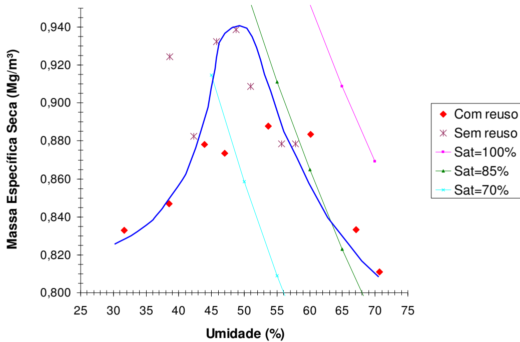
Curva Compactação Proctor Normal M3
