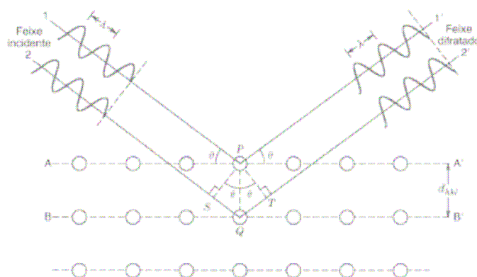
Figura 4.3. Difração de raios-X em planos atômicos.
