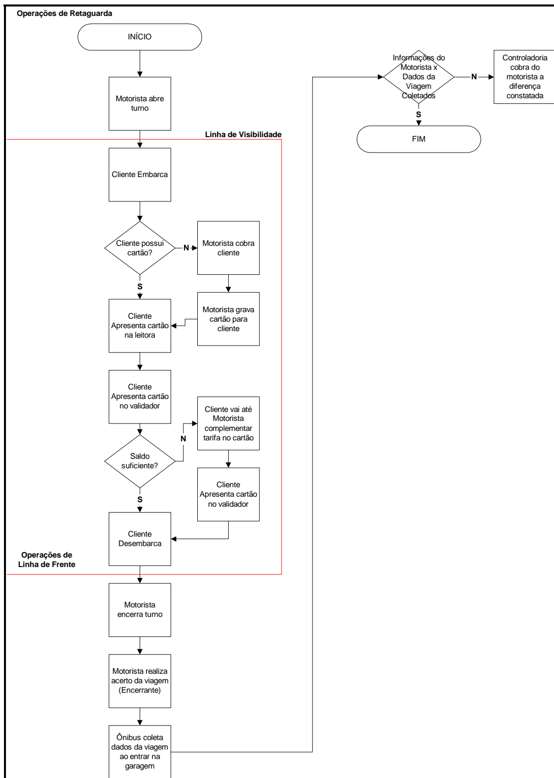
Figura 3.10 - Fluxograma da operação com bilhetagem eletrônica em linhas seccionadas
