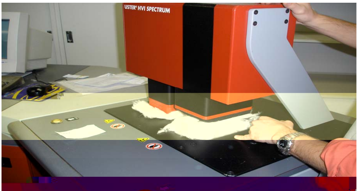
Figura 6. Classificação no aparelho HVI para se obter características tecnológicas de grau de cor e impurezas de fibras de algodão.
