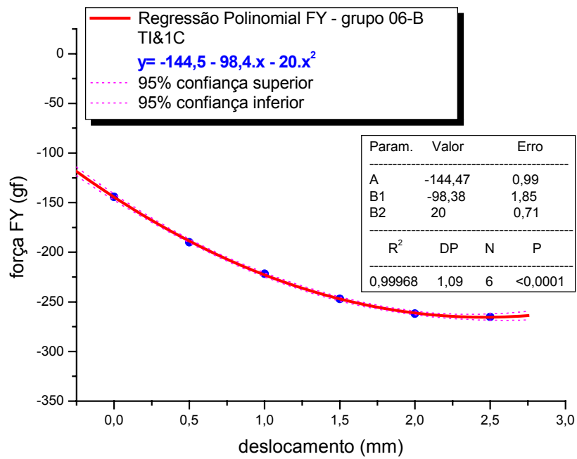
Figura 81 – Regressão Polinomial FY do grupo 06-B – TI&amp;1C
