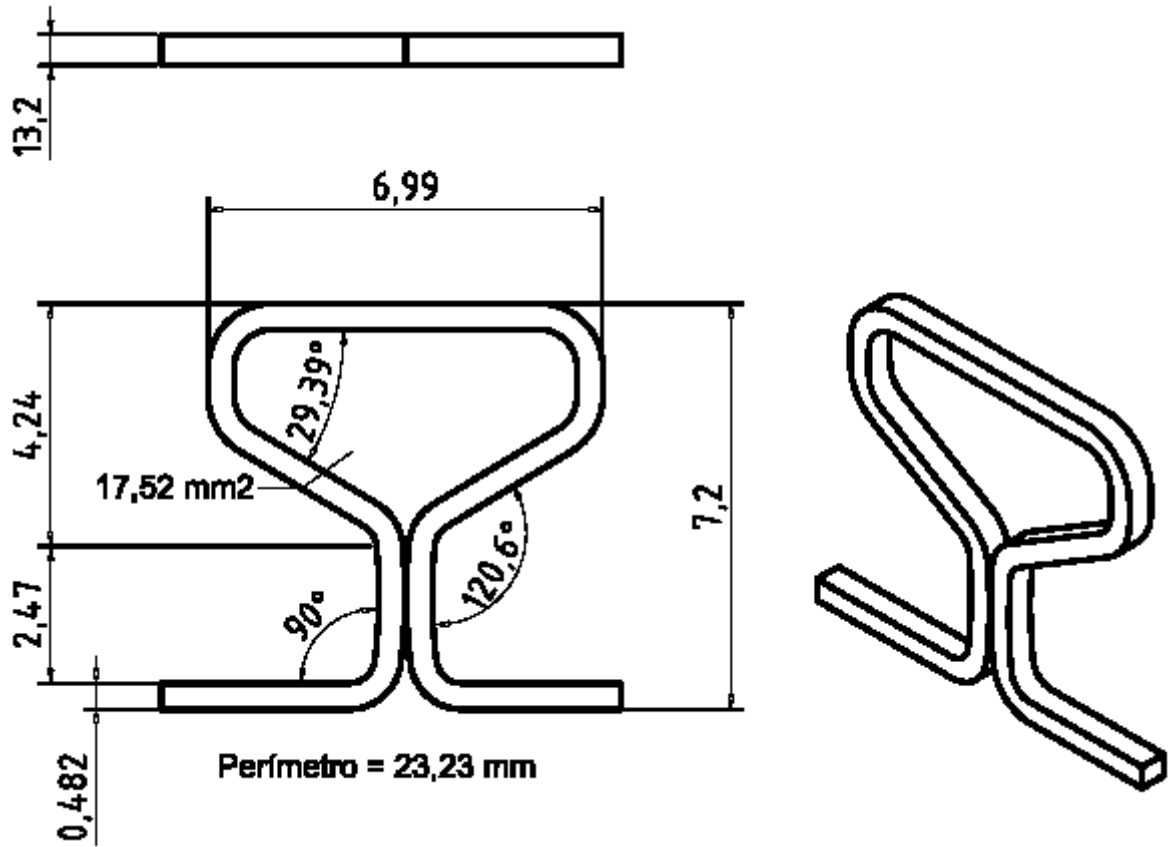
Figura 38 – Medidas lineares, angulares e de área das alças do grupo 06-A
