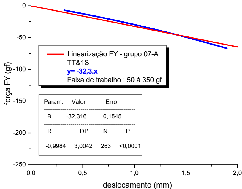
Figura 88 – Comportamento elástico em FY do grupo 07-A – TT&1S ( 50 \leq FX \leq 350 gf)
