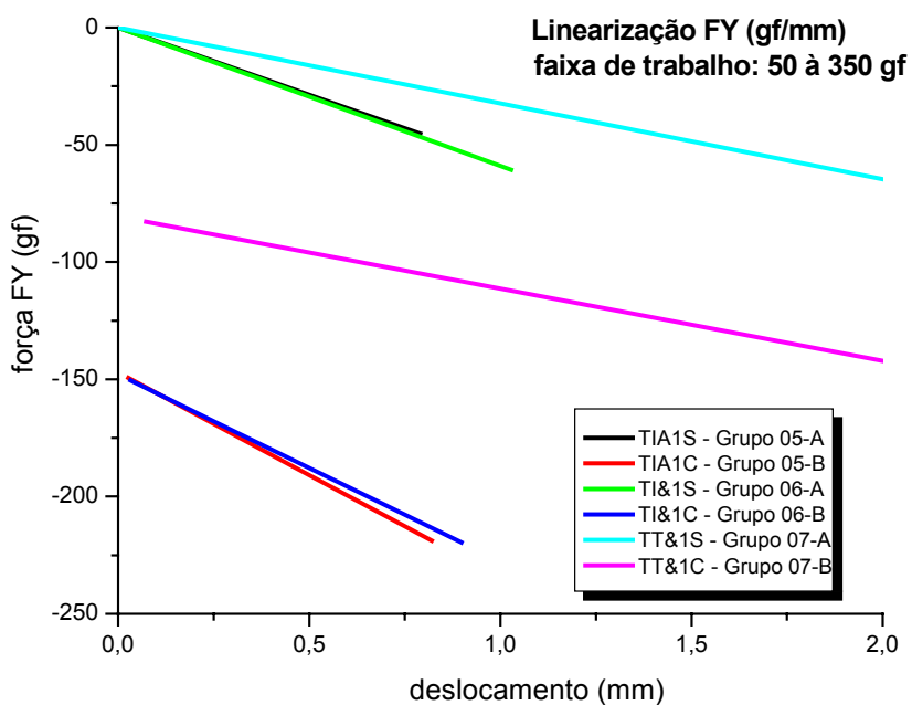
Figura 101 – Comportamento elástico para FY para os grupos 01 ao 07-B para a faixa de trabalho entre 50 e 350 gf em FX – Comparativo
