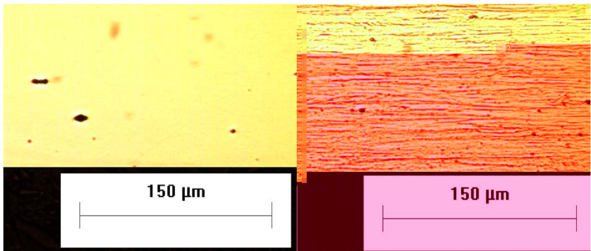
Figura 44 – (A) Imagem metalográfica sem ataque eletrolítico (200X) - grupo 03 (B) Imagem metalográfica com ataque eletrolítico (200X) - grupo 03
