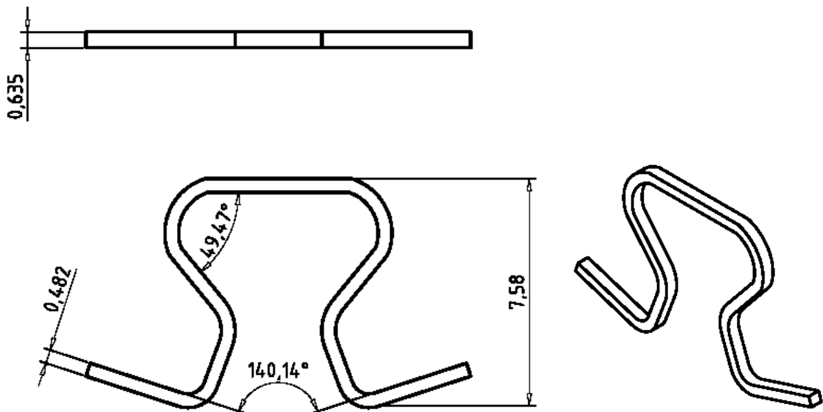
Figura 41 – Medidas lineares, angulares e de área das alças do grupo 07-B
