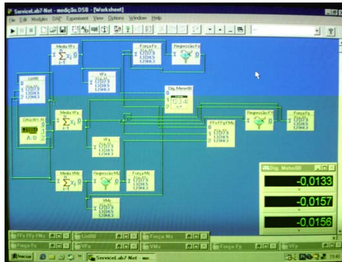
Figura 28 – Representação modular do programa DASyLab ® VERSÃO 7.0
