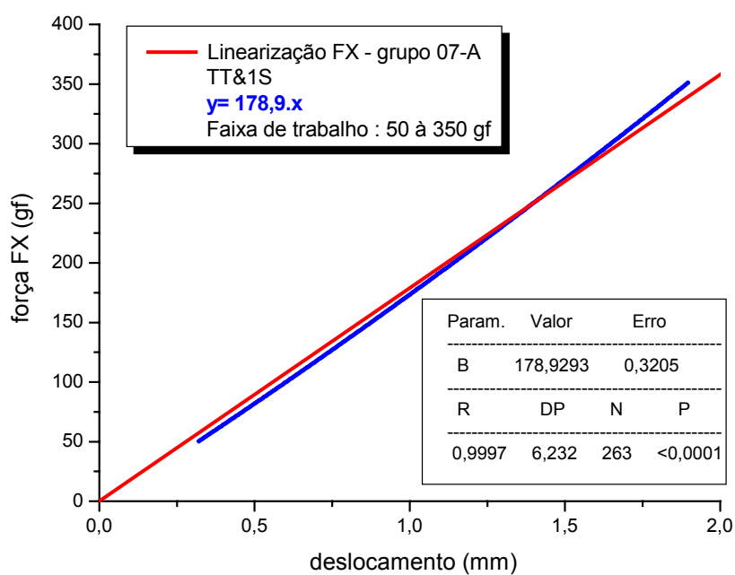
Figura 86 – Comportamento elástico em FX do grupo 07-A – TT&1S ( 50 \leq FX \leq 350 gf)
