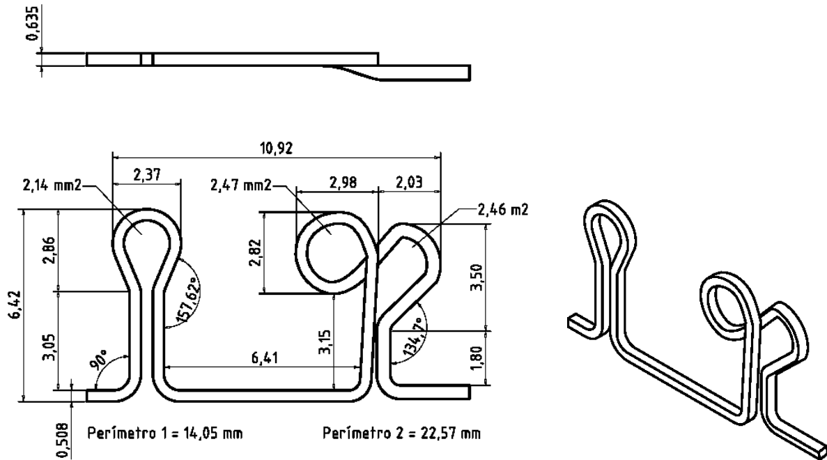
Figura 35 – Medidas lineares, angulares e de área das alças do grupo 04
