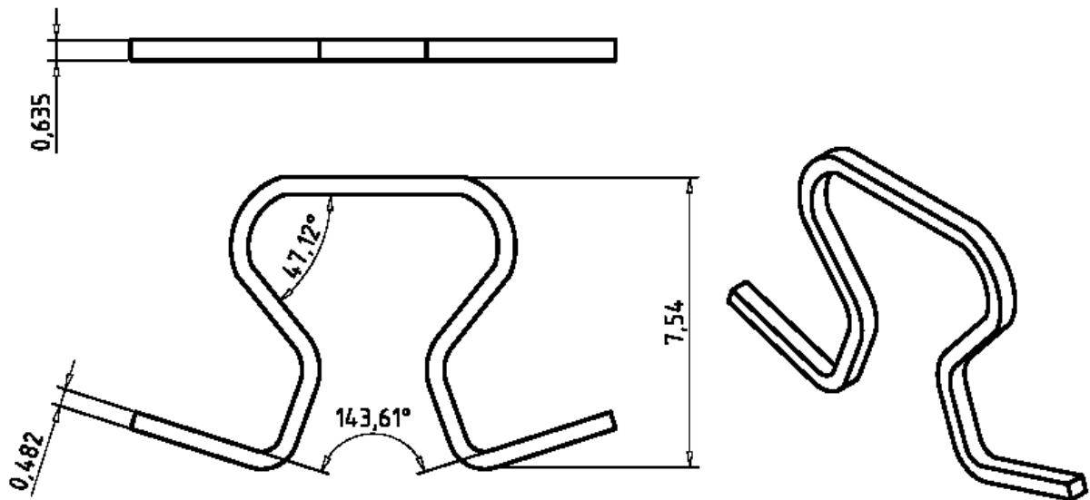
Figura 39 – Medidas lineares, angulares e de área das alças do grupo 06-B
