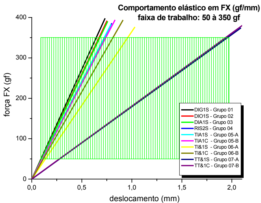
Figura 98 – Comportamento elástico em FX para os grupos 01 ao 07-B para a faixa de trabalho entre 50 e 350 gf – Comparativo
