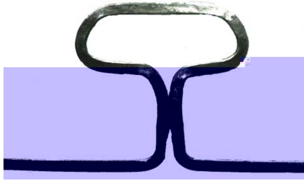
Figura 13 – Alça em “T” – ADITEK
