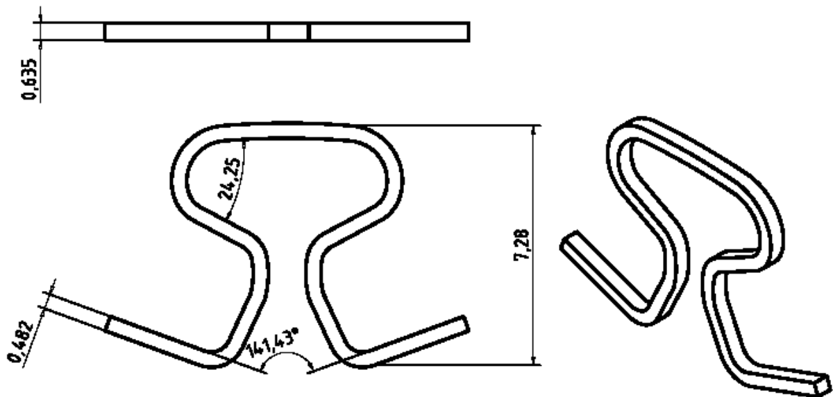
Figura 37 – Medidas lineares, angulares e de área das alças do grupo 05-B
