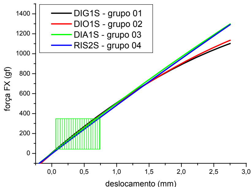
Figura 59 – Regressões gerais de FX para os grupos 01 ao 04 - Comparativo
