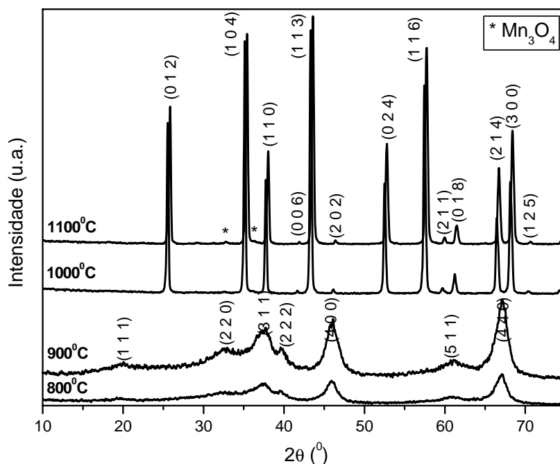
FIGURA 4.16 - Difratomogramas de raios X das amostras de Al 2 O 3 /4%Mn.
