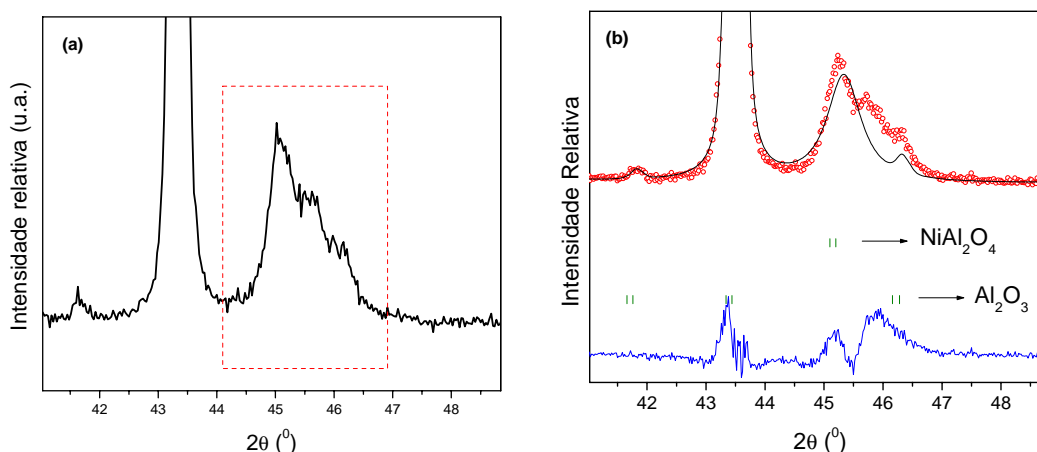
FIGURA 4.23 - Difratomogramas de raios X, ampliado de 41 a 49^{\circ} ( 2\theta ), da amostra de \text{Al}_2\text{O}_3/8\%\text{Ni} calcinada a 1100^{\circ}\text{C} por 2h (a) difratograma observado e (b) gráfico parcial de Rietveld.
