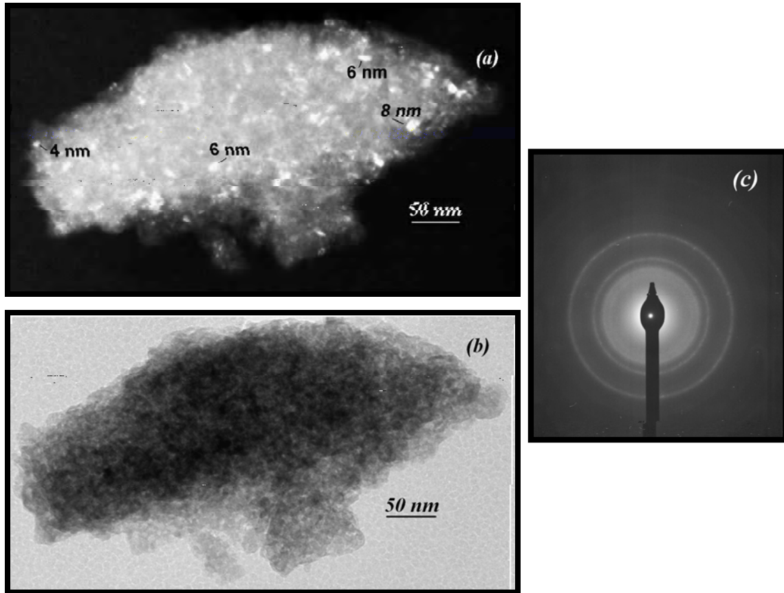
FIGURA 4.42 - Imagens obtidas por Microscopia Eletrônica de Transmissão (MET) da amostra de \text{Al}_2\text{O}_3/2\%\text{Mn} calcinada a 900^\circ\text{C} por 2h (a) campo escuro (b) campo claro (c) padrão de difração de elétrons.
