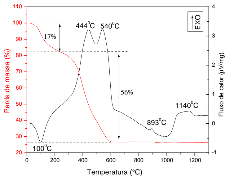
FIGURA 4.3 - Curvas de análise térmica (TG/DTA) da amostra \text{Al}_2\text{O}_3/2\%\text{Ni} .
