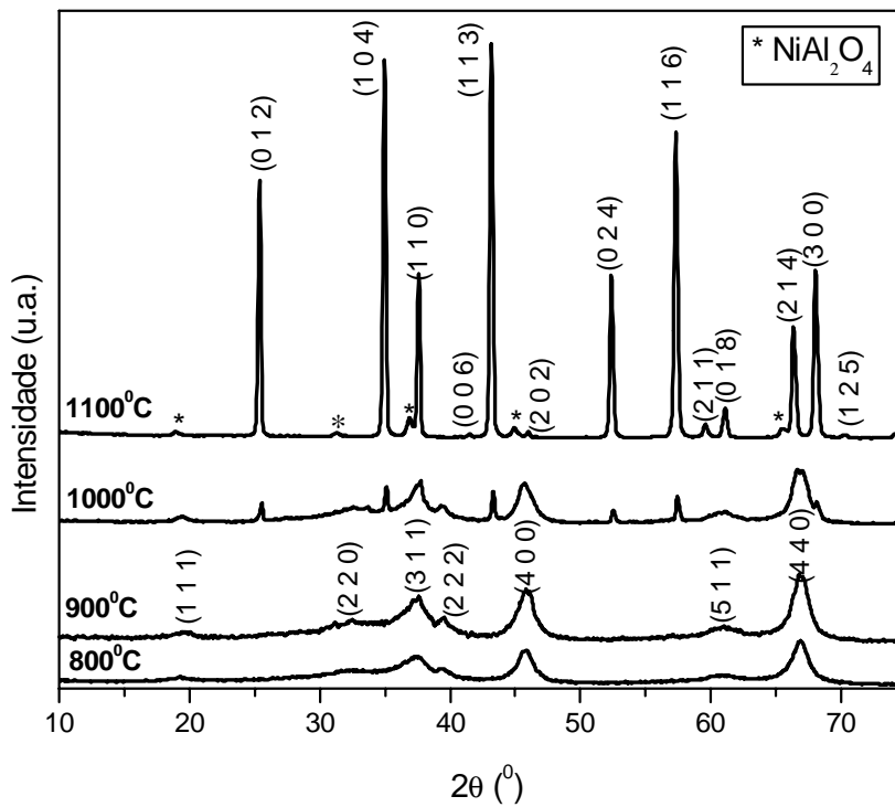
FIGURA 4.12 - Difratogramas de raios X das amostras de Al 2 O 3 /2%Ni.
