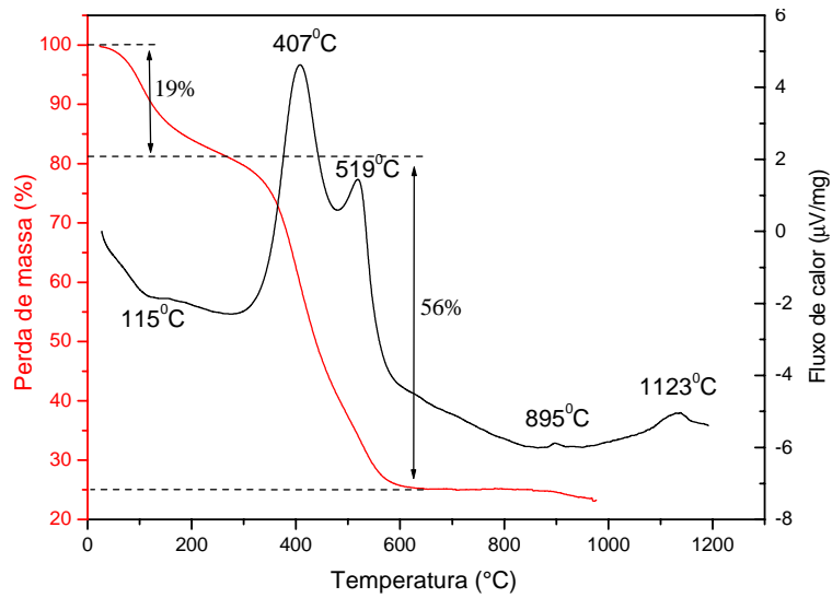
FIGURA 4.5 - Curvas de análise térmica (TG/DTA) da amostra Al 2 O 3 /2%Mn.
