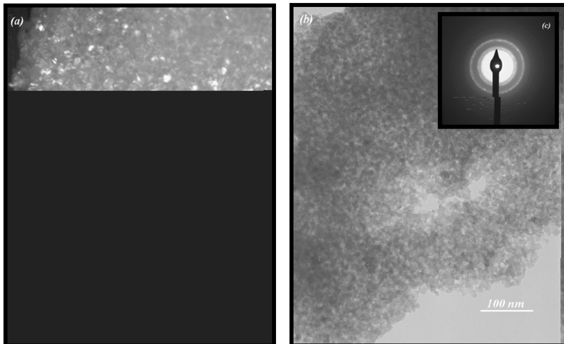
FIGURA 4.35 - Imagens obtidas por Microscopia Eletrônica de Transmissão (MET) da amostra de \text{Al}_2\text{O}_3/8\%\text{Fe} calcinada a 900^\circ\text{C} por 2h (a) campo escuro (b) campo claro (c) padrão de difração de elétrons.
