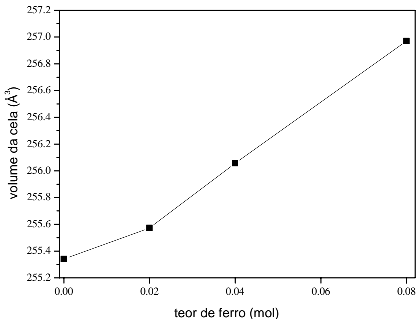
FIGURA 4.19 - Volume da célula em função da quantidade de ferro adicionado à rede da alumina para as amostras obtidas a 1100°C.
