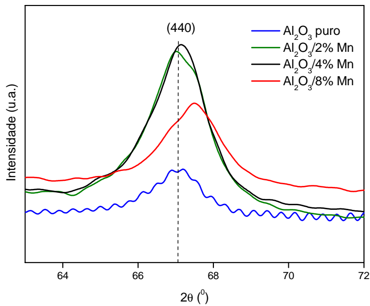
FIGURA 4.18 - Difratoformas de raios X das amostras de Al 2 O 3 puro e dopado com 2, 4 e 8% em mol de manganês obtidas a 900°C (região ampliada com 2θ entre 63 e 72°).
