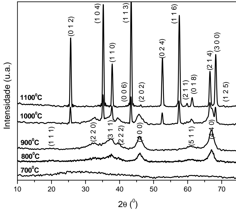
FIGURA 4.9 - Difratomogramas de raios X das amostras de Al 2 O 3 /4%Fe.
