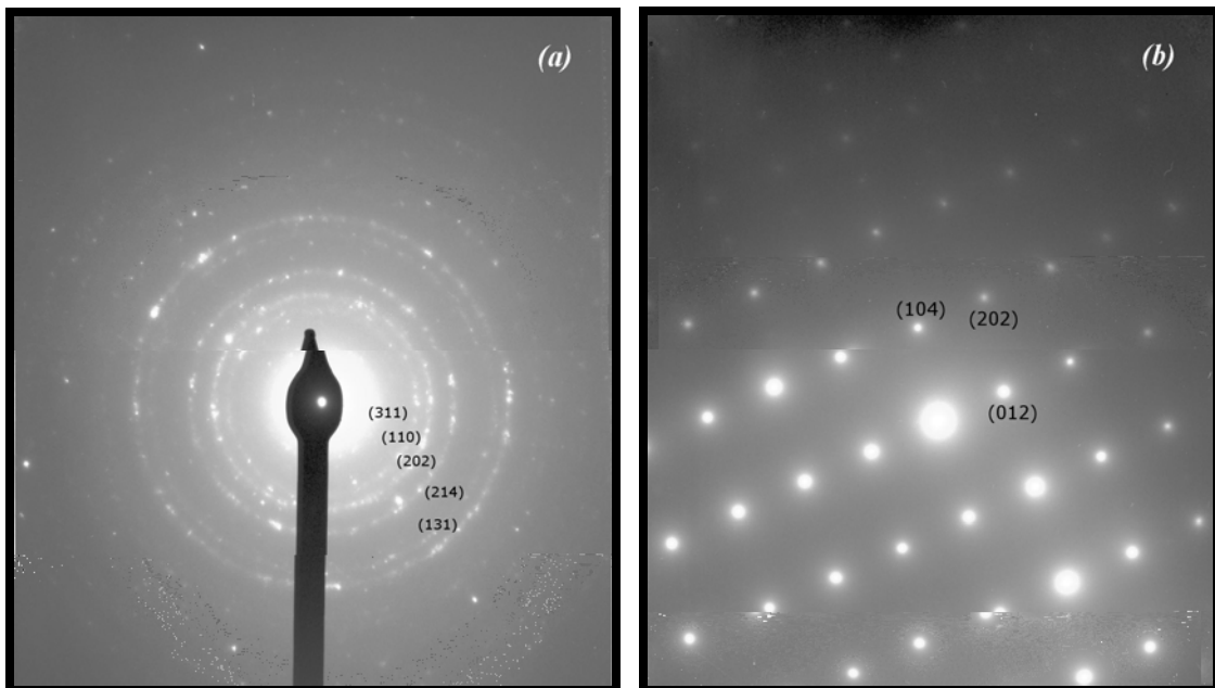
FIGURA 4.41 - Padrões de difração de elétrons obtidas por MET em regiões diferentes da amostra de \text{Al}_2\text{O}_3/8\%\text{Ni} calcinada a 1100^\circ\text{C} por 2h (a) \text{NiAl}_2\text{O}_4 (b) \alpha\text{-Al}_2\text{O}_3 .
