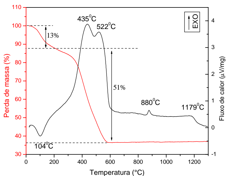
FIGURA 4.4 - Curvas de análise térmica (TG/DTA) da amostra \text{Al}_2\text{O}_3/8\%\text{Ni} .
