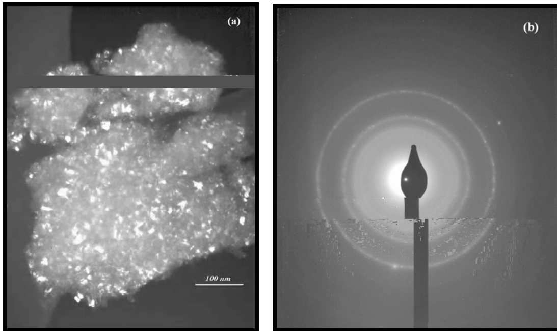
FIGURA 4.34 - Imagens obtidas por Microscopia Eletrônica de Transmissão (MET) da amostra de \text{Al}_2\text{O}_3/2\%\text{Fe} calcinada a 900^\circ\text{C} por 2h (a) campo escuro (b) padrão de difração de elétrons.
