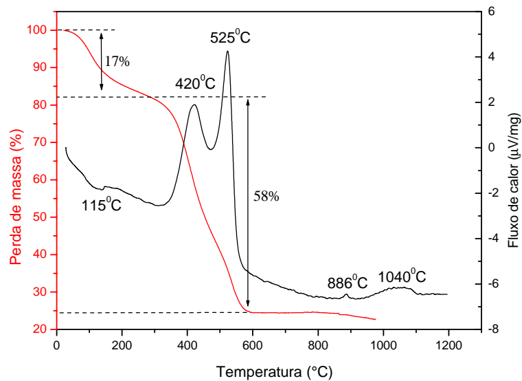
FIGURA 4.6 - Curvas de análise térmica (TG/DTA) da amostra Al 2 O 3 /8%Mn.
