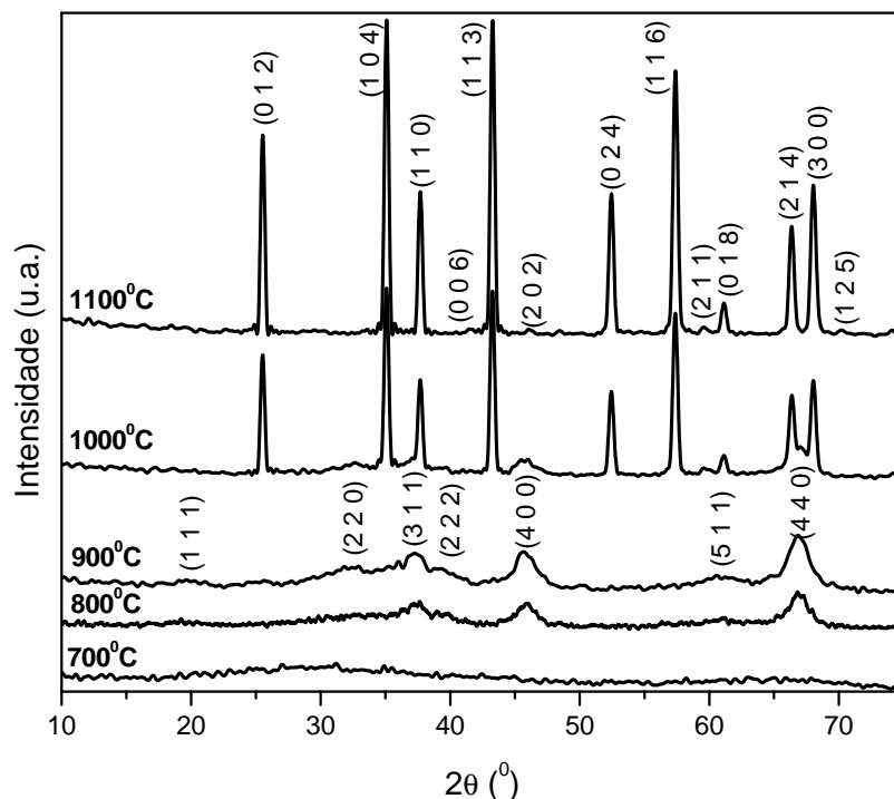
FIGURA 4.10 - Difratomogramas de raios X das amostras de \text{Al}_2\text{O}_3/8\%\text{Fe} .
