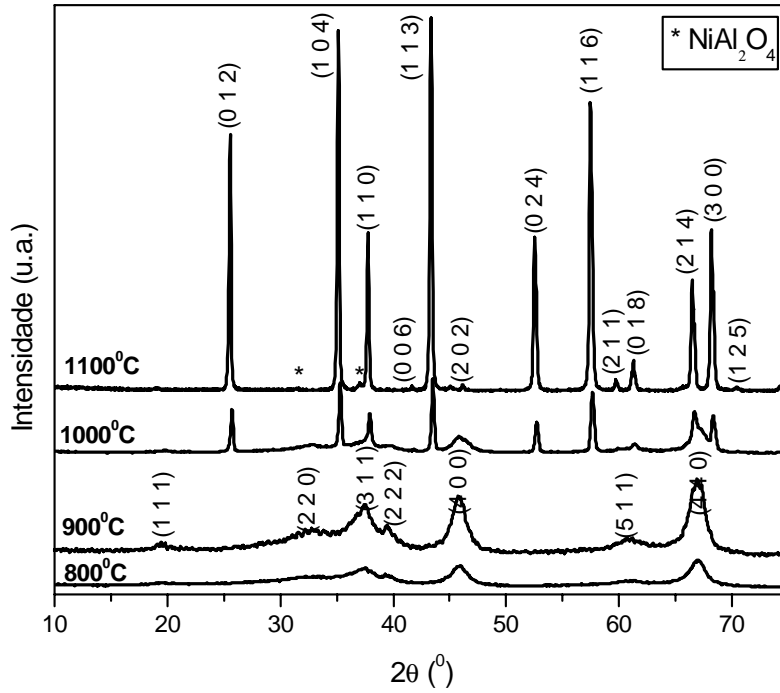
FIGURA 4.11 - Difratogramas de raios X das amostras de Al 2 O 3 /1%Ni.
