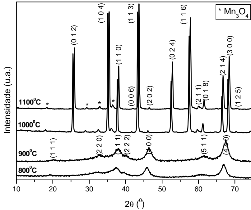
FIGURA 4.17 - Difratoformas de raios X das amostras de Al 2 O 3 /8%Mn.
