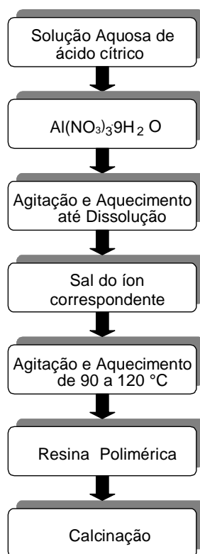
FIGURA 3.1 - Fluxograma utilizado na obtenção dos pigmentos de alumina dopada com ferro, níquel e manganês.
