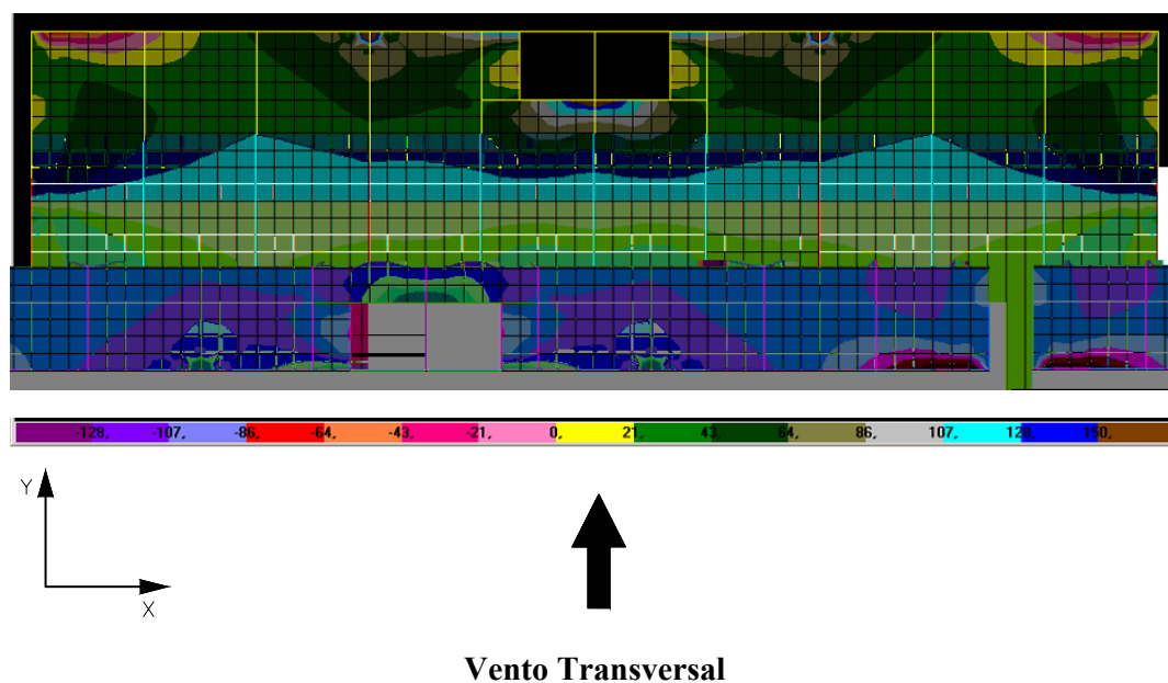
FIGURA 6.50 – Distribuição de tensões \sigma_x na face superior dos elementos de laje do 2º andar do modelo TRANSIÇÃO 2 (N/cm 2 )
