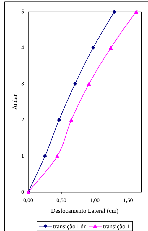
FIGURA 8.4 – Deslocamentos laterais U_y no ponto ( X = 15,00 m; Y = 4,50 m) - 1º ao 5º andares
