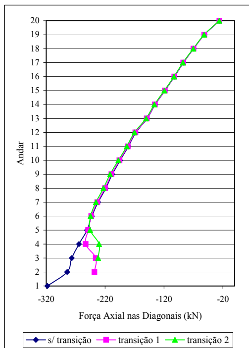
FIGURA 7.13 – Forças axiais nas diagonais comprimidas do contraventamento central
