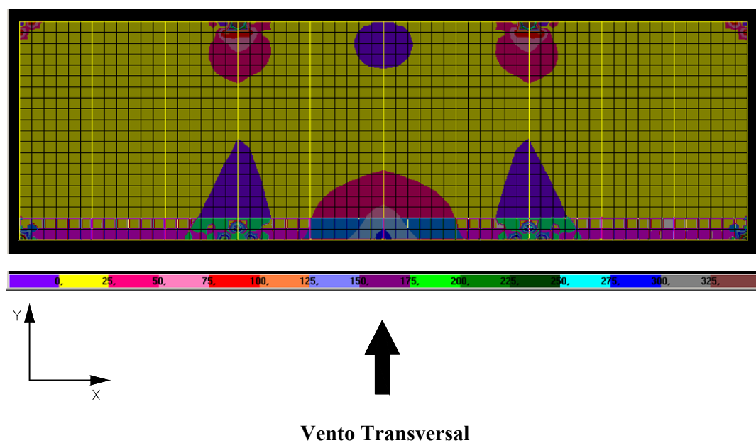
FIGURA 6.35 – Distribuição de tensões \sigma_{\text{máx}} na face superior dos elementos de laje do 20º andar do modelo SEM TRANSIÇÃO (N/cm 2 )
