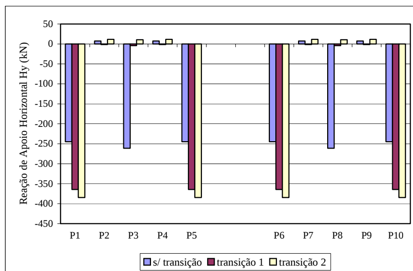
FIGURA 7.1 - Reações de apoio horizontais H_y na fundação dos pilares P1 a P10
