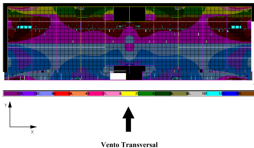
FIGURA 6.51 – Distribuição de tensões \sigma_x na face superior dos elementos de laje do 3º andar do modelo TRANSIÇÃO 2 (N/cm 2 )
