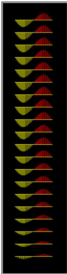
FIGURA 7.28 – Momento fletor M_3 devido às forças de vento transversal nas vigas do eixo X = 6,00 m do modelo TRANSICÃO 1
