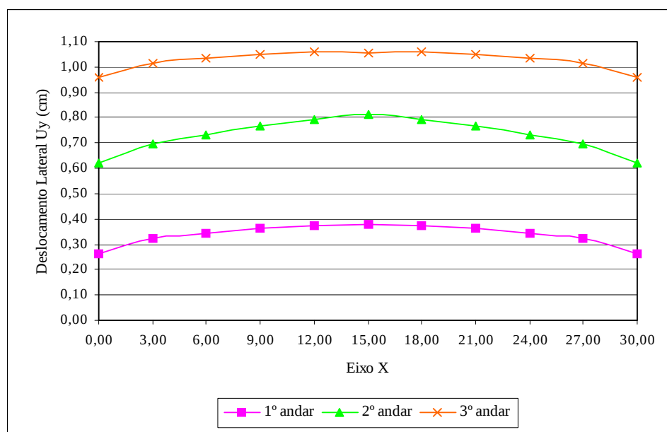
FIGURA 7.8 - Deslocamentos laterais U_y ao longo do eixo Y = 4,50 m nos 1º, 2º e 3º andares do modelo TRANSIÇÃO 2
