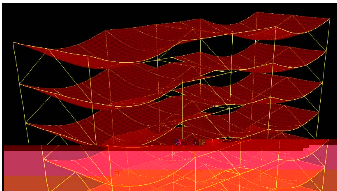
FIGURA 6.74 – Deformação das lajes, vigas e pilares dos andares superiores do modelo TRANSIÇÃO 1 devido às cargas gravitacionais nominais
