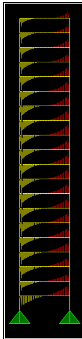
FIGURA 7.29 – Momento fletor M_3 devido às forças de vento transversal nas vigas do eixo X = 9,00 m do modelo TRANSICÃO 1
