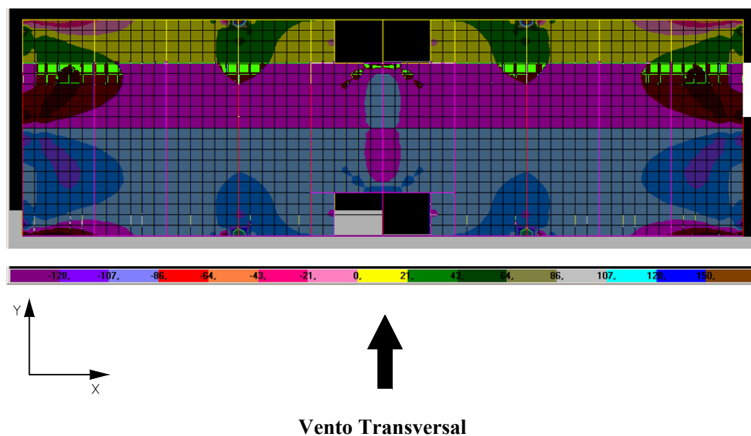
FIGURA 6.52 – Distribuição de tensões \sigma_x na face superior dos elementos de laje do 4º andar do modelo TRANSIÇÃO 2 ( \text{N/cm}^2 )
