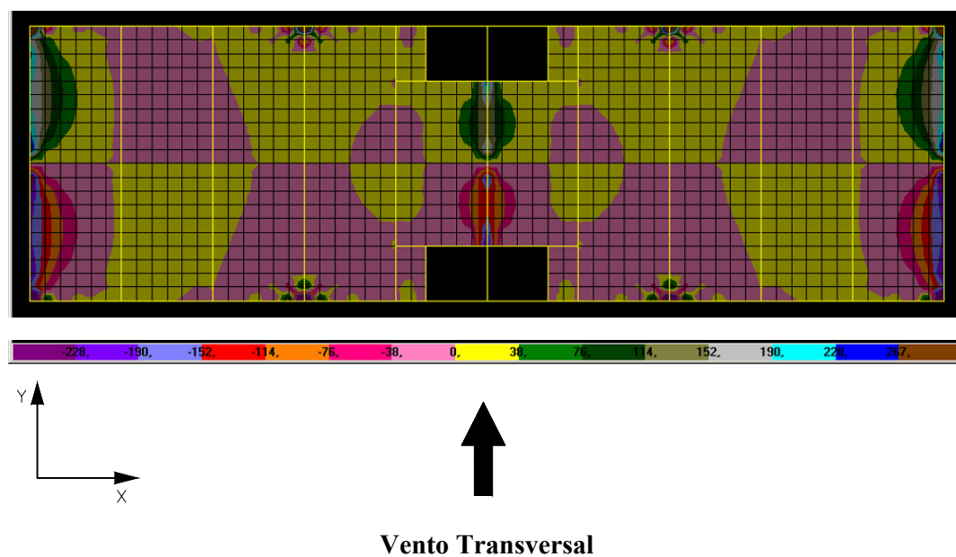
FIGURA 6.15 – Distribuição de tensões \sigma_y na face superior dos elementos de laje do 2º andar do modelo SEM TRANSIÇÃO ( \text{N/cm}^2 )
