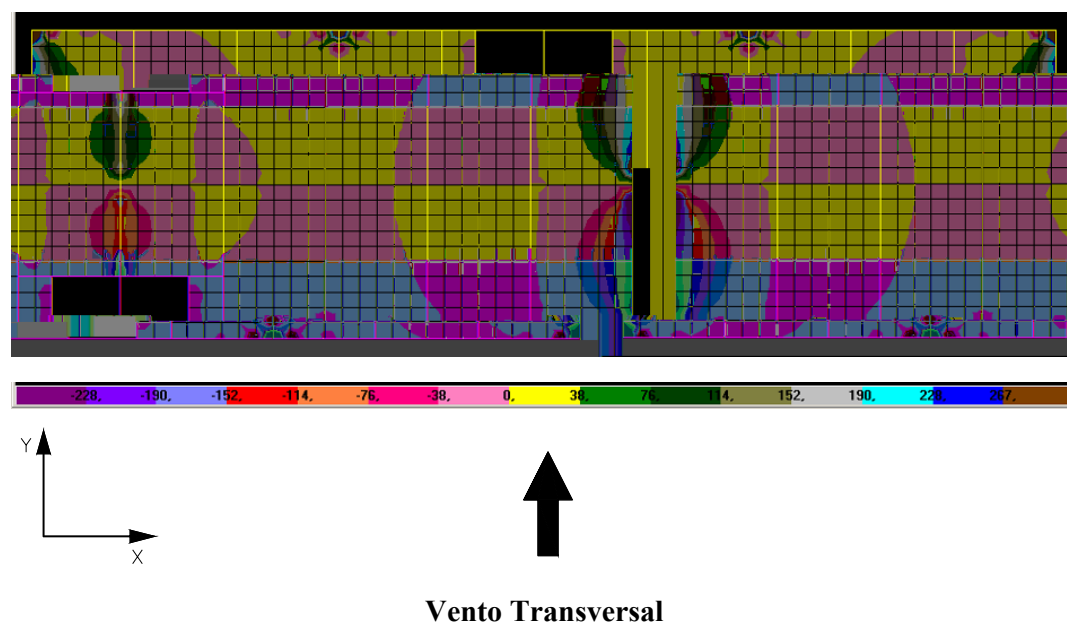
FIGURA 6.42 – Distribuição de tensões \sigma_y na face superior dos elementos de laje do 2º andar do modelo TRANSIÇÃO 1 ( \text{N/cm}^2 )
