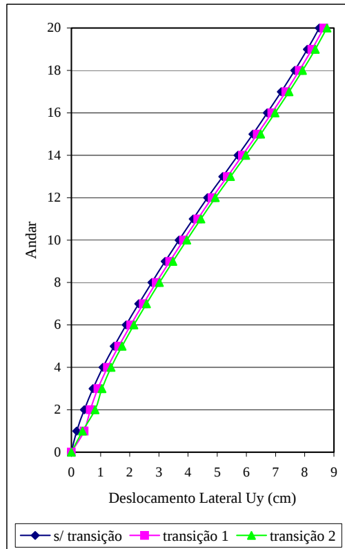
FIGURA 7.3 – Deslocamentos laterais U_y no ponto ( X = 15,00 m; Y = 4,50 m)
