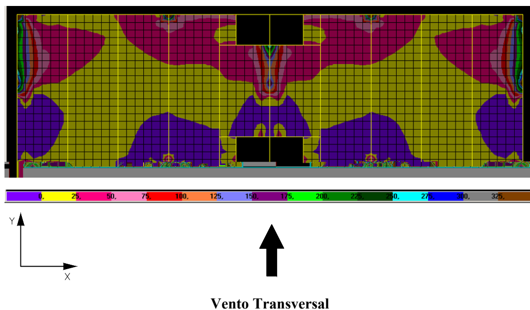
FIGURA 6.46 – Distribuição de tensões \sigma_{\text{máx}} na face superior dos elementos de laje do 2º andar do modelo TRANSIÇÃO 1 ( \text{N/cm}^2 )
