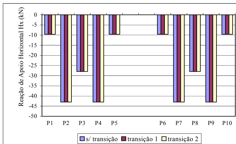
FIGURA 7.36 - Reações de apoio horizontais Hx na fundação dos pilares P1 a P10
