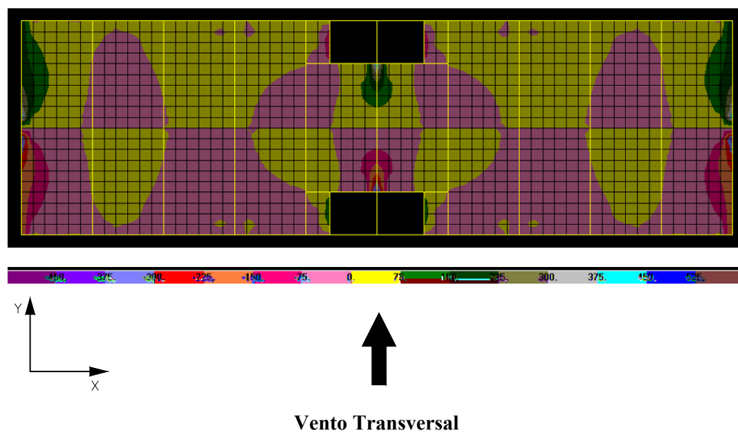
FIGURA 5.4 – Distribuição de tensões \sigma_y na face inferior dos elementos de laje do modelo SIMPLIFICADO ( \text{N/cm}^2 )
