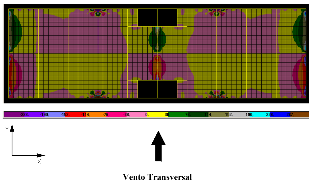
FIGURA 6.20 – Distribuição de tensões \sigma_y na face inferior dos elementos de laje do 10º andar do modelo SEM TRANSIÇÃO (N/cm 2 )
