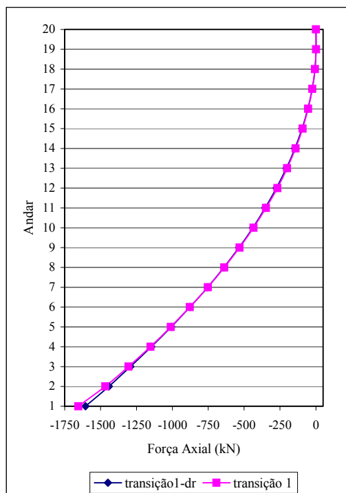
FIGURA 8.13 – Forças axiais no pilar P6
