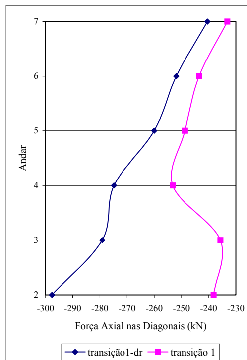
FIGURA 8.11 – Forças axiais nas diagonais comprimidas do contraventamento central - 2º ao 7º andares
