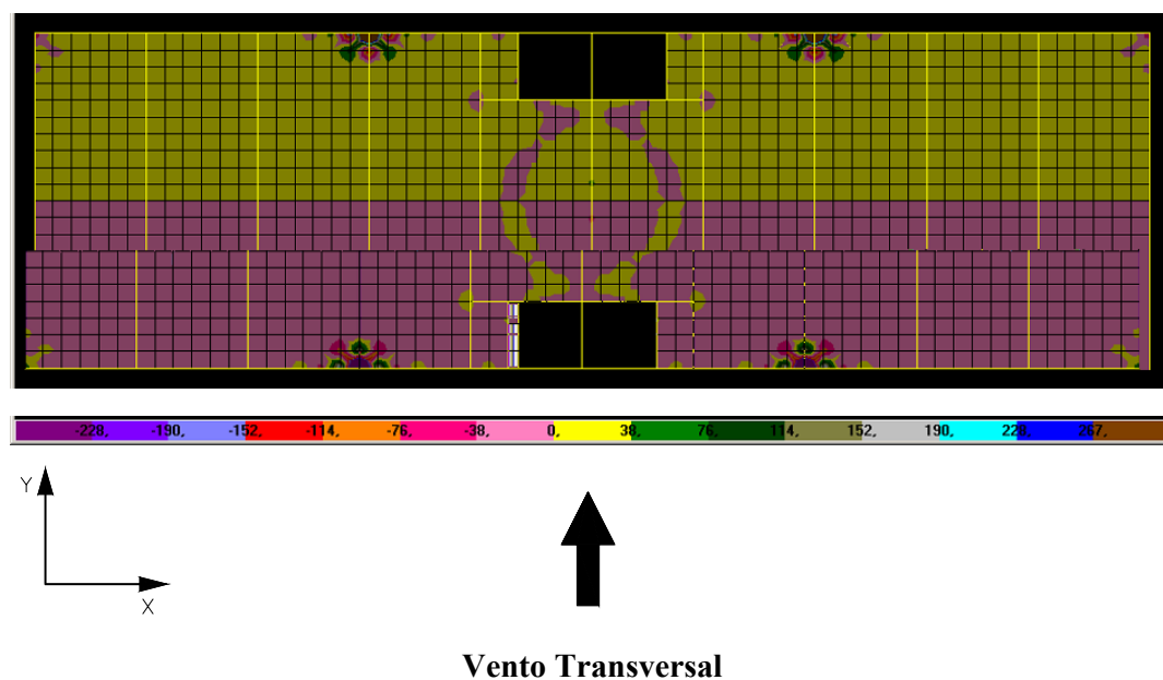
FIGURA 6.21 – Distribuição de tensões \sigma_y na face superior dos elementos de laje do 19º andar do modelo SEM TRANSIÇÃO ( \text{N/cm}^2 )
