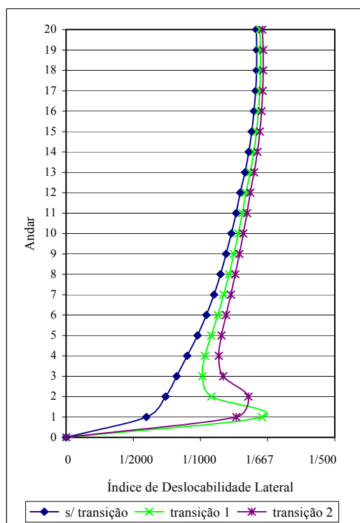
FIGURA 7.9 – Índice de deslocabilidade lateral - ponto (X = 15,00m; Y = 4,50m)
