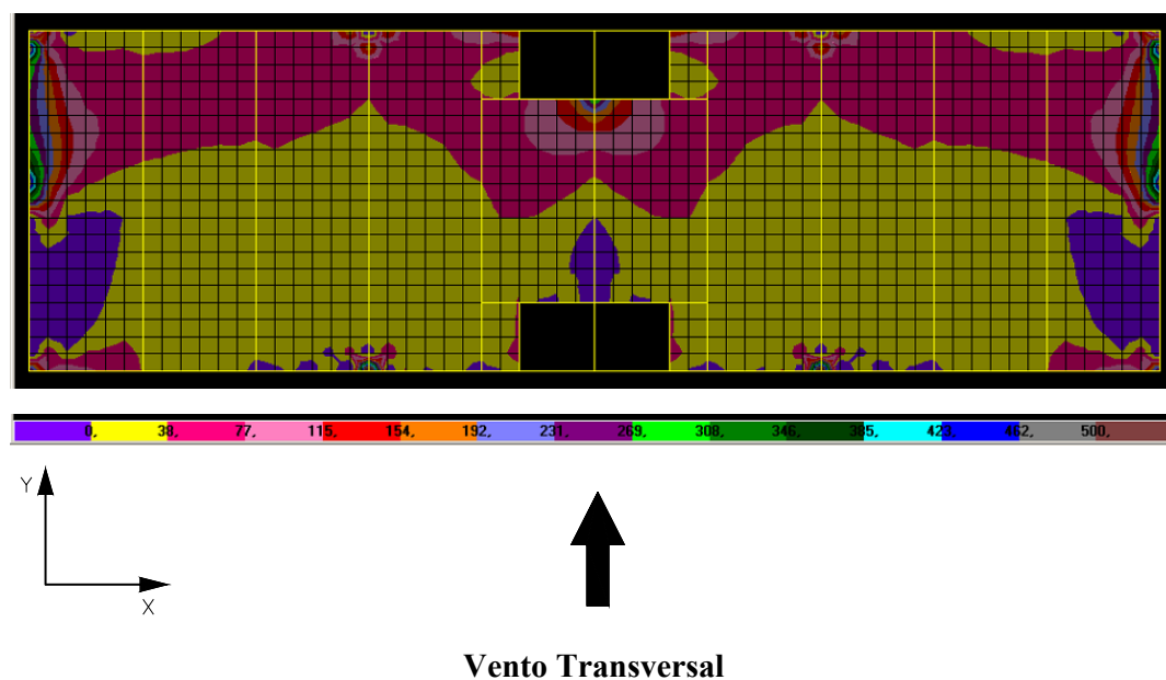
FIGURA 6.67 – Distribuição de tensões \sigma_{\text{máx}} na face inferior dos elementos de laje do 1º andar do modelo TRANSIÇÃO 1 (N/cm 2 )
