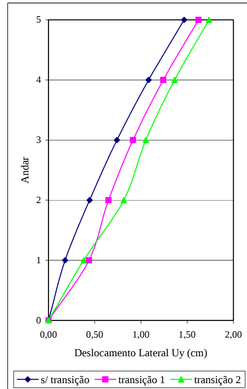
FIGURA 7.4 – Deslocamentos laterais U_y no ponto ( X = 15,00 m; Y = 4,50 m) - 1º ao 5º andares
