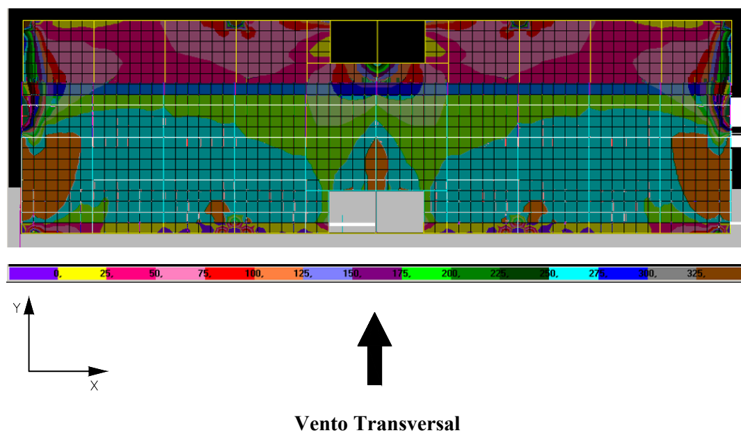
FIGURA 6.64 – Distribuição de tensões \sigma_{\max} na face superior dos elementos de laje do 1º andar do modelo TRANSIÇÃO 1 (N/cm 2 )
