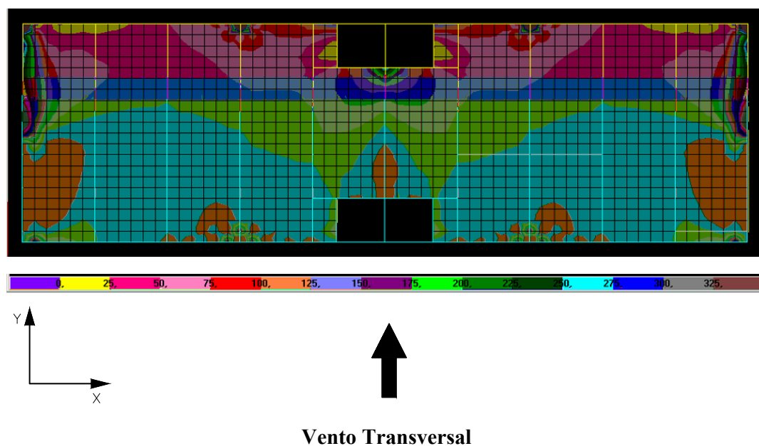
FIGURA 6.60 – Distribuição de tensões \sigma_{\max} na face superior dos elementos de laje do 2º andar do modelo TRANSIÇÃO 2 ( \text{N/cm}^2 )
