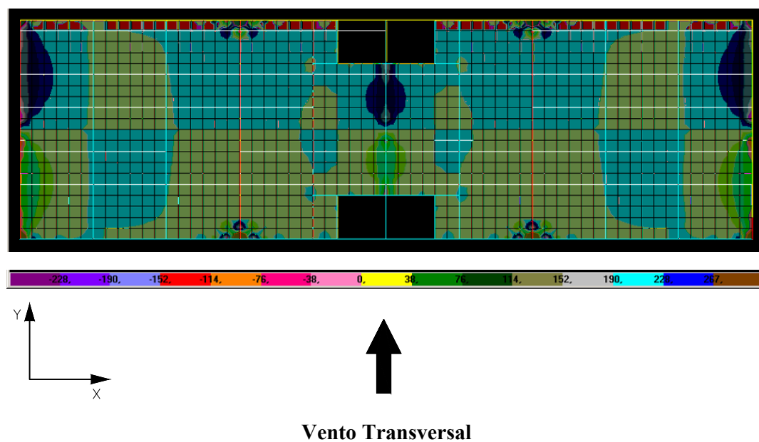
FIGURA 6.19 – Distribuição de tensões \sigma_y na face superior dos elementos de laje do 10º andar do modelo SEM TRANSIÇÃO (N/cm 2 )
