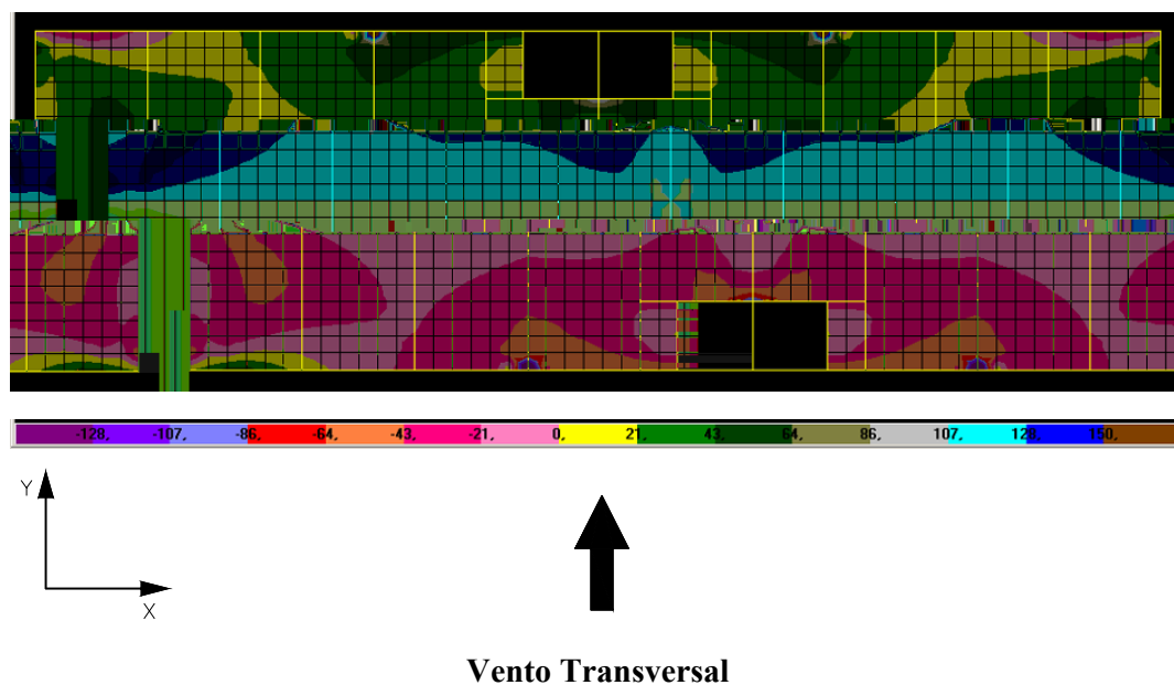
FIGURA 6.38 – Distribuição de tensões \sigma_x na face superior dos elementos de laje do 2º andar do modelo TRANSIÇÃO 1 (N/cm 2 )
