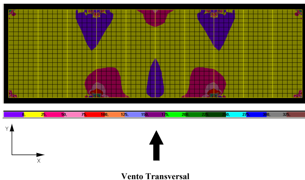
FIGURA 6.36 – Distribuição de tensões \sigma_{\text{máx}} na face inferior dos elementos de laje do 20º andar do modelo SEM TRANSIÇÃO (N/cm 2 )
