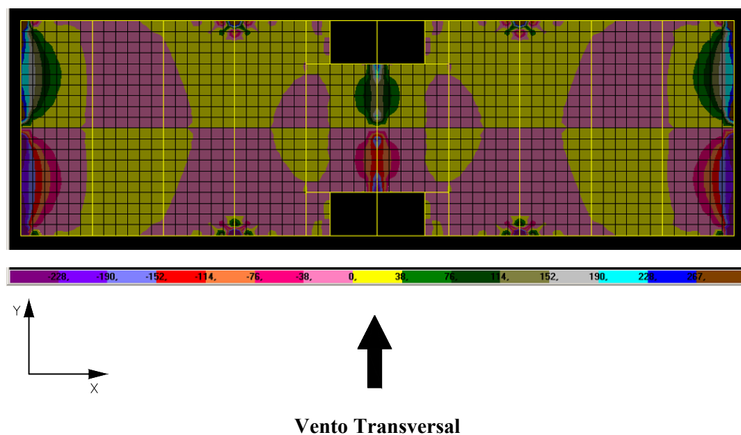
FIGURA 6.43 – Distribuição de tensões \sigma_y na face superior dos elementos de laje do 3º andar do modelo TRANSIÇÃO 1 (N/cm 2 )
