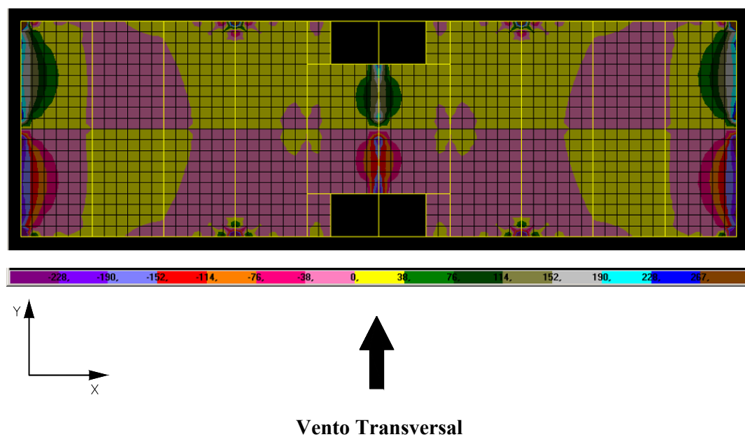
FIGURA 6.13 – Distribuição de tensões \sigma_y na face superior dos elementos de laje do 1º andar do modelo SEM TRANSIÇÃO (N/cm 2 )
