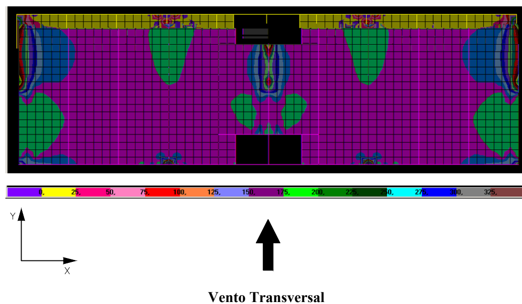
FIGURA 6.28 – Distribuição de tensões \sigma_{\text{máx}} na face inferior dos elementos de laje do 2º andar do modelo SEM TRANSIÇÃO (N/cm 2 )
