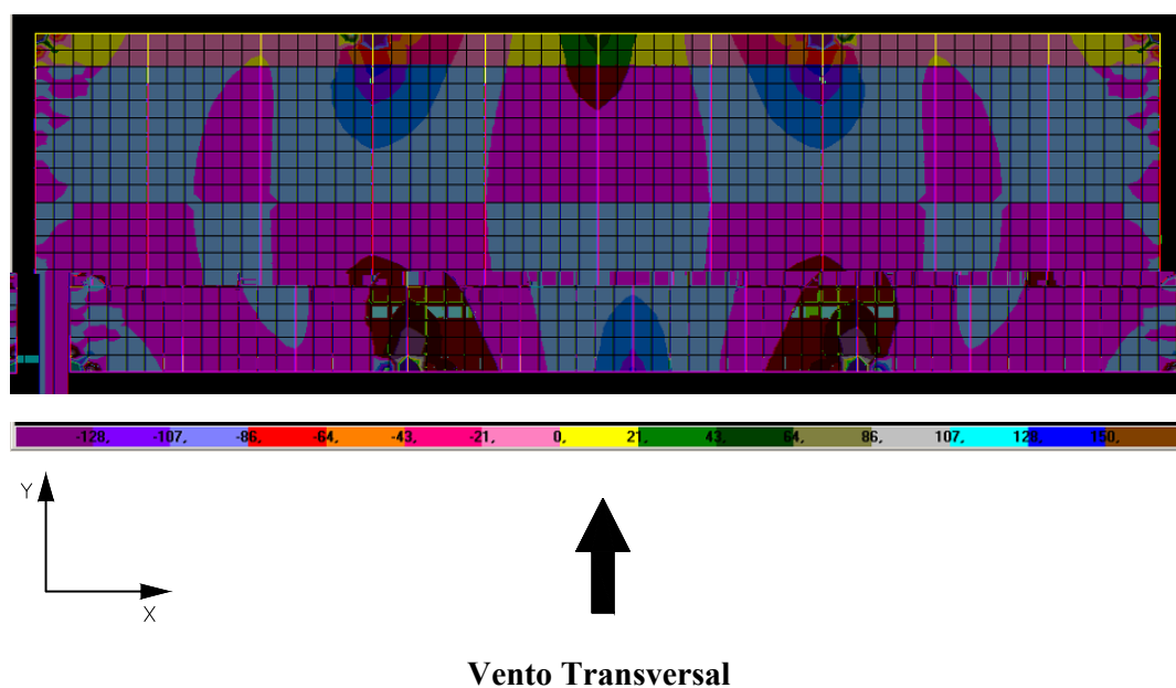
FIGURA 6.12 – Distribuição de tensões \sigma_x na face inferior dos elementos de laje do 20º andar do modelo SEM TRANSIÇÃO ( \text{N/cm}^2 )
