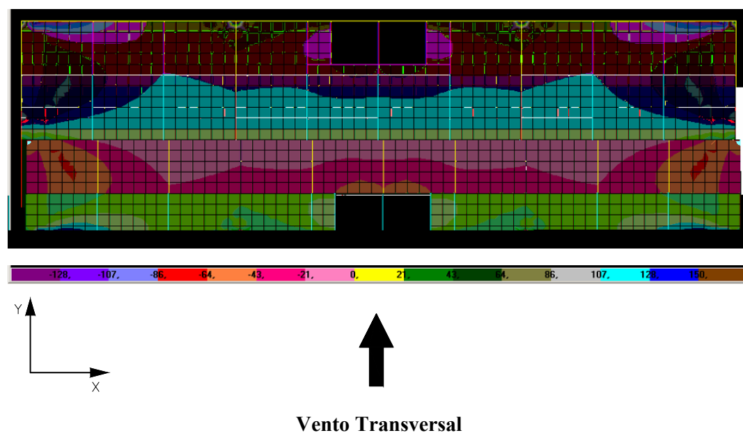
FIGURA 6.49 – Distribuição de tensões \sigma_x na face superior dos elementos de laje do 1º andar do modelo TRANSIÇÃO 2 (N/cm 2 )
