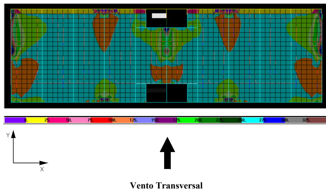
FIGURA 6.32 – Distribuição de tensões \sigma_{\text{máx}} na face inferior dos elementos de laje do 10º andar do modelo SEM TRANSIÇÃO (N/cm 2 )
