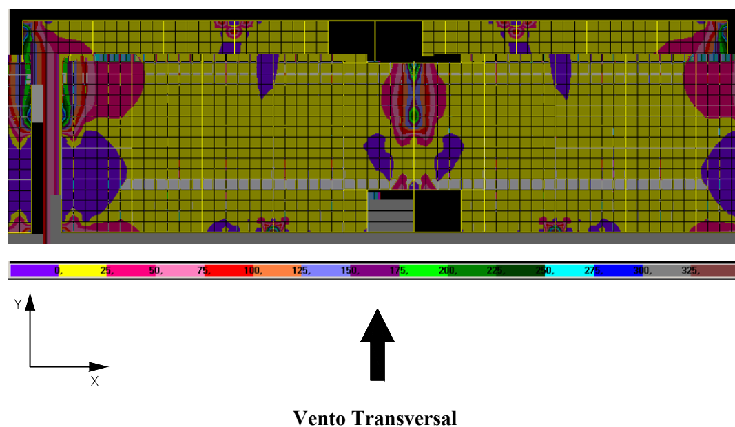
FIGURA 6.26 – Distribuição de tensões \sigma_{\text{máx}} na face inferior dos elementos de laje do 1º andar do modelo SEM TRANSIÇÃO (N/cm 2 )
