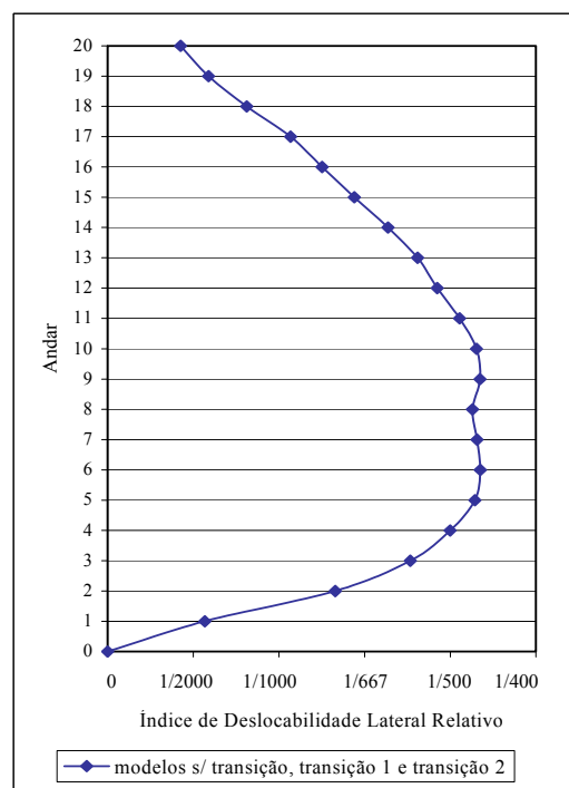
FIGURA 7.41 – Índice de deslocabilidade lateral relativo - ponto (X = 15,00m; Y = 4,50m)
