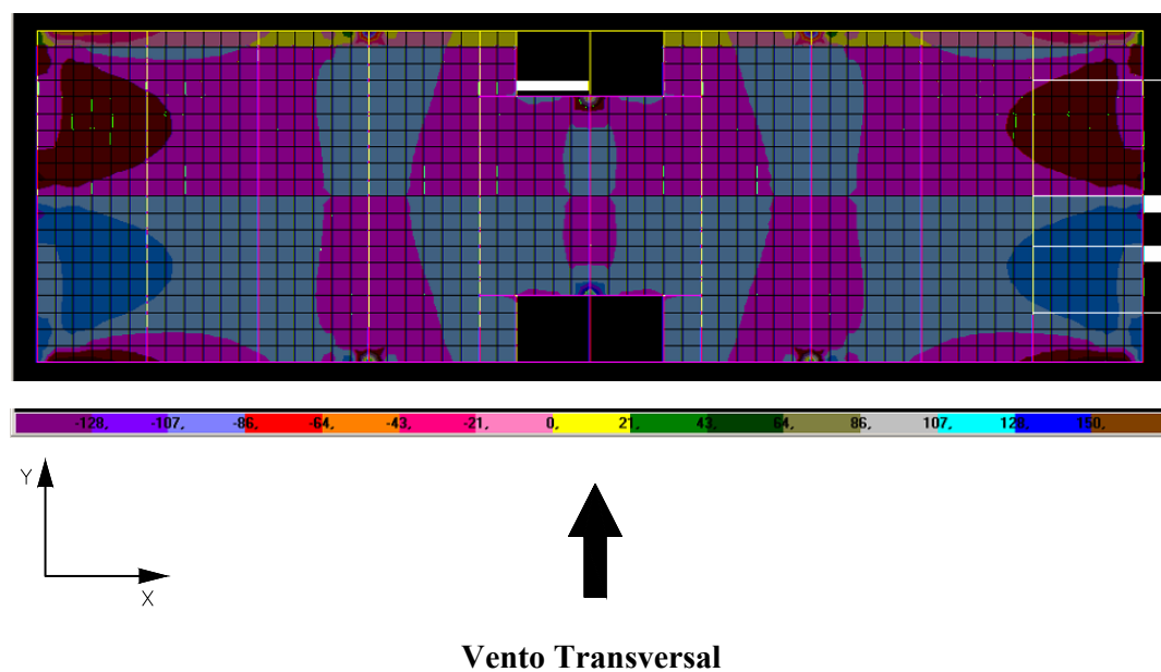
FIGURA 6.4 – Distribuição de tensões \sigma_x na face inferior dos elementos de laje do 2º andar do modelo SEM TRANSIÇÃO (N/cm 2 )
