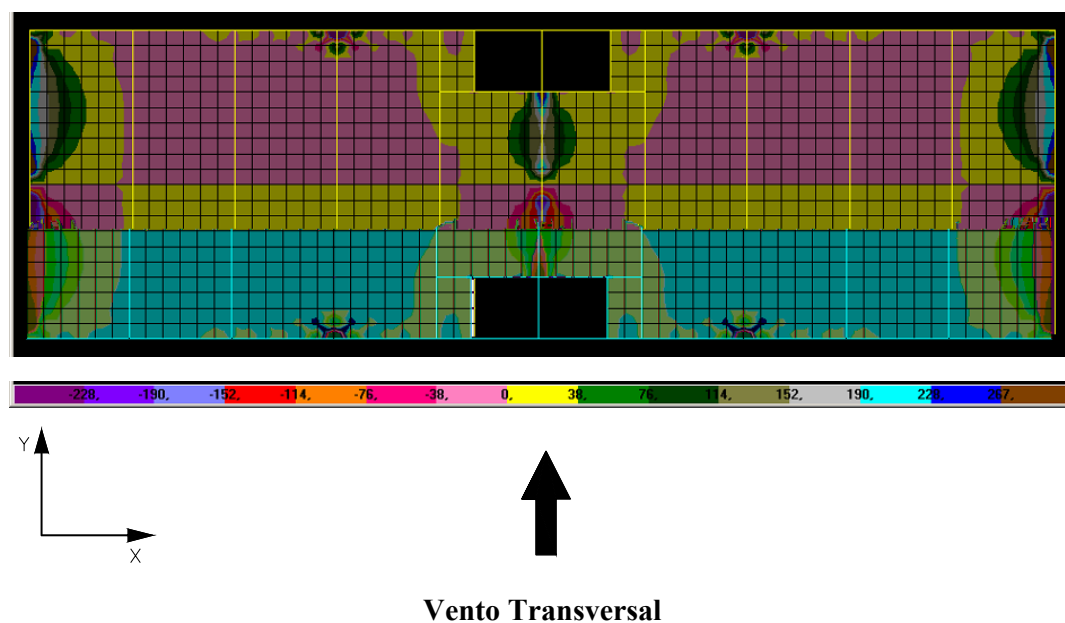
FIGURA 6.18 – Distribuição de tensões \sigma_y na face inferior dos elementos de laje do 3º andar do modelo SEM TRANSIÇÃO (N/cm 2 )
