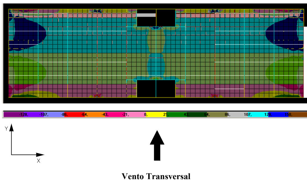
FIGURA 6.1 – Distribuição de tensões \sigma_x na face superior dos elementos de laje do 1º andar do modelo SEM TRANSIÇÃO (N/cm 2 )
