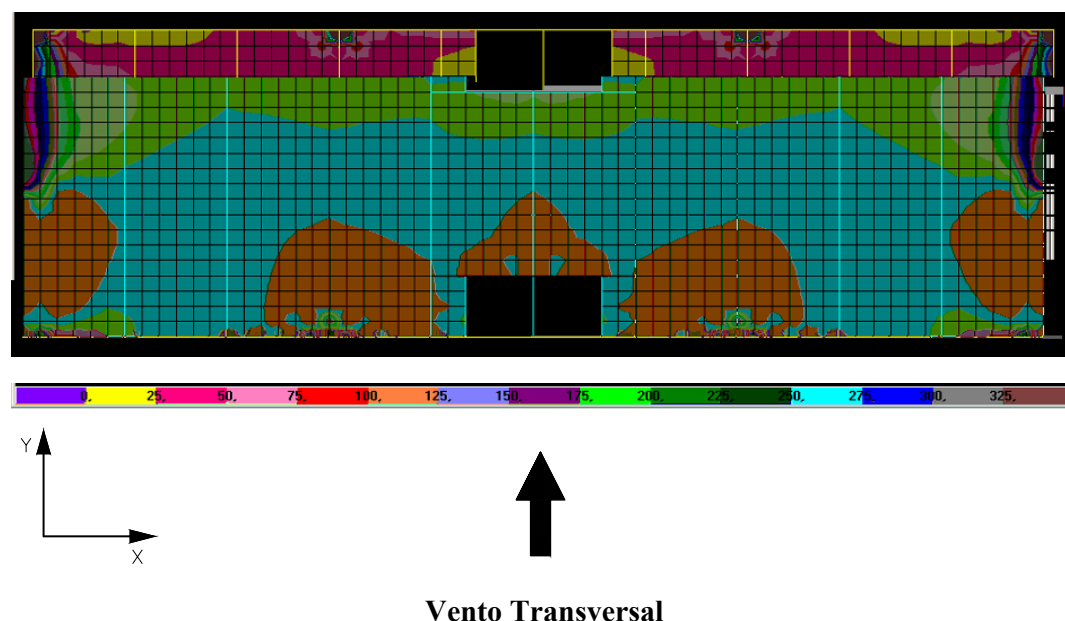
FIGURA 6.59 – Distribuição de tensões \sigma_{\text{máx}} na face superior dos elementos de laje do 1º andar do modelo TRANSIÇÃO 2 ( \text{N}/\text{cm}^2 )
