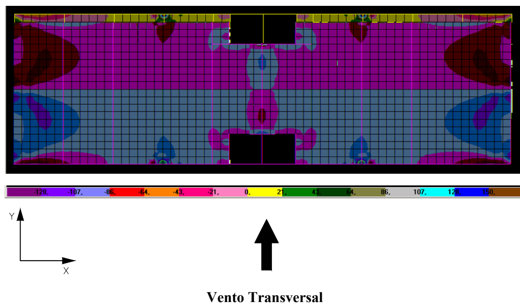
FIGURA 6.5 – Distribuição de tensões \sigma_x na face superior dos elementos de laje do 3º andar do modelo SEM TRANSIÇÃO (N/cm 2 )
