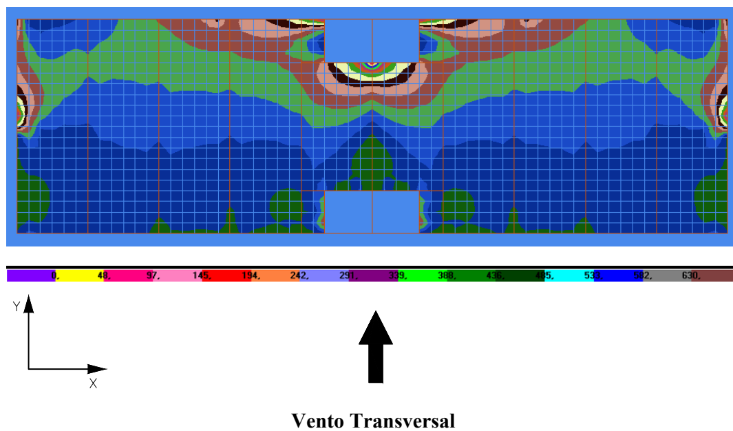
FIGURA 5.6 – Distribuição de tensões \sigma_{\text{máx}} na face inferior dos elementos de laje do modelo SIMPLIFICADO (N/cm 2 )
