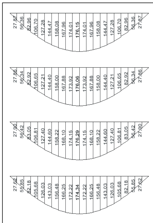
FIGURA 7.34 – Momento fletor M3 devido às cargas gravitacionais nas vigas do eixo X = 6,00 m do modelo TRANSIÇÃO 1 – 1º ao 4º andares
