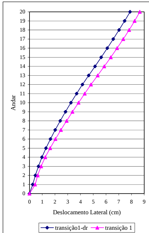
FIGURA 8.3 – Deslocamentos laterais U_y no ponto ( X = 15,00 m; Y = 4,50 m)
