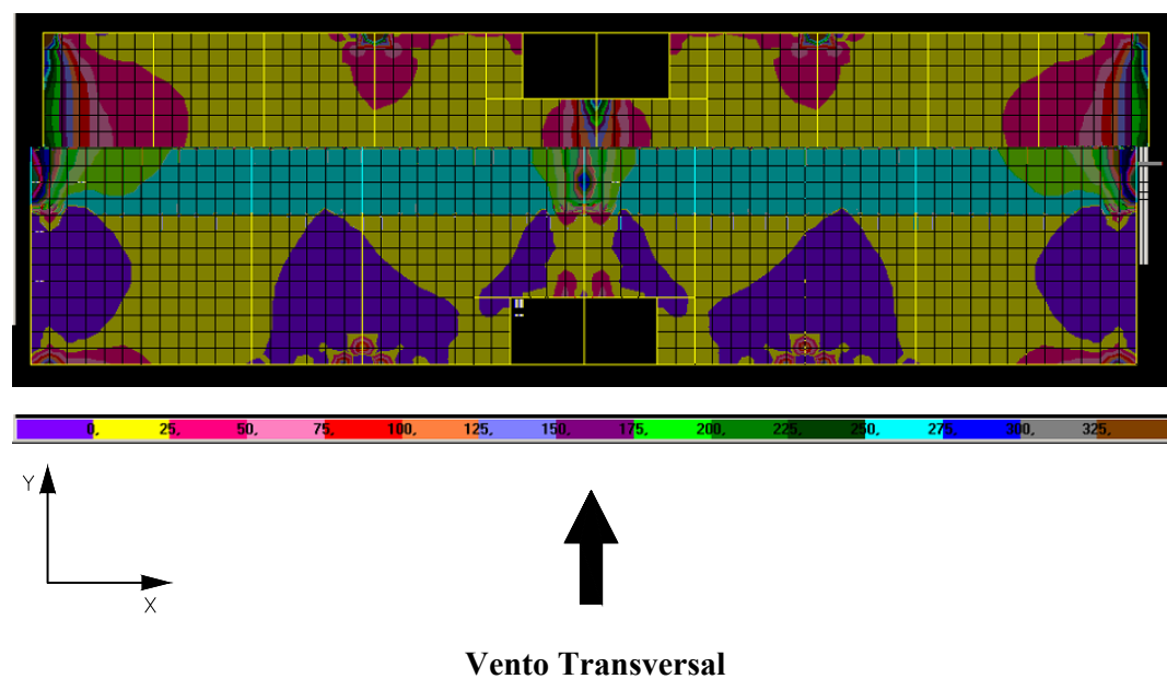
FIGURA 6.47 – Distribuição de tensões \sigma_{\max} na face superior dos elementos de laje do 3º andar do modelo TRANSIÇÃO 1 ( \text{N}/\text{cm}^2 )
