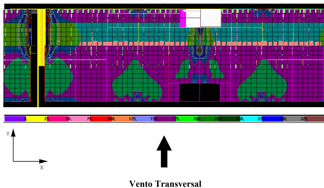
FIGURA 6.27 – Distribuição de tensões \sigma_{\text{máx}} na face superior dos elementos de laje do 2º andar do modelo SEM TRANSIÇÃO (N/cm 2 )
