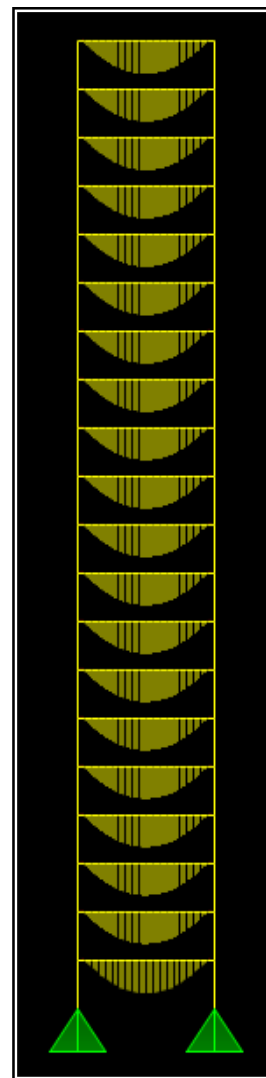
FIGURA 7.33 – Momento fletor M_3 devido às cargas gravitacionais nas vigas do eixo X = 9,00 m do modelo TRANSICÃO 1
