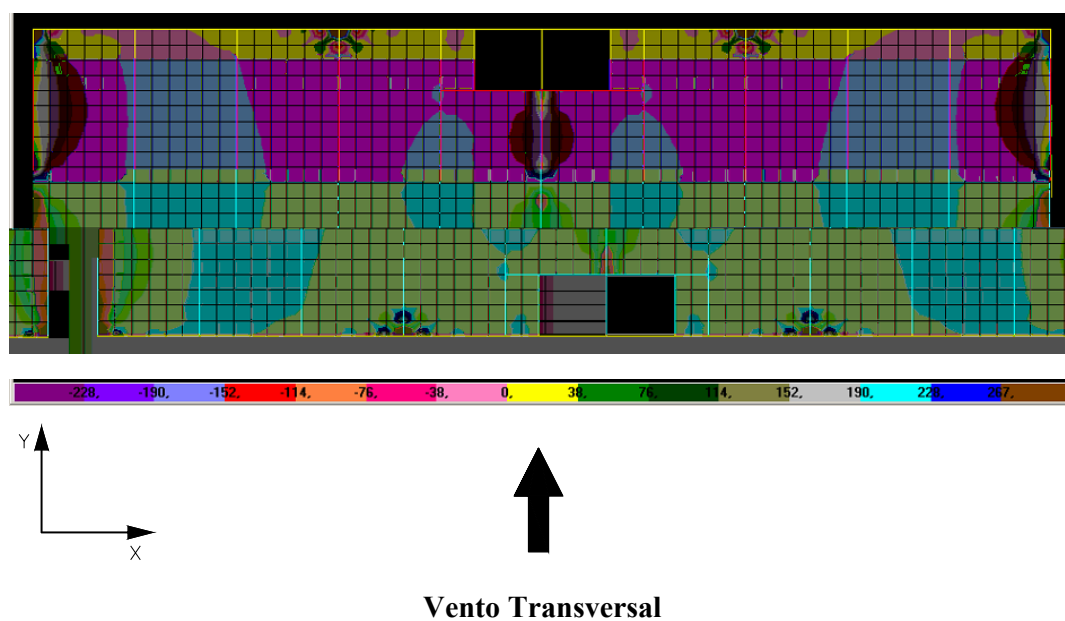
FIGURA 6.58 – Distribuição de tensões \sigma_y na face superior dos elementos de laje do 5º andar do modelo TRANSIÇÃO 2 (N/cm 2 )
