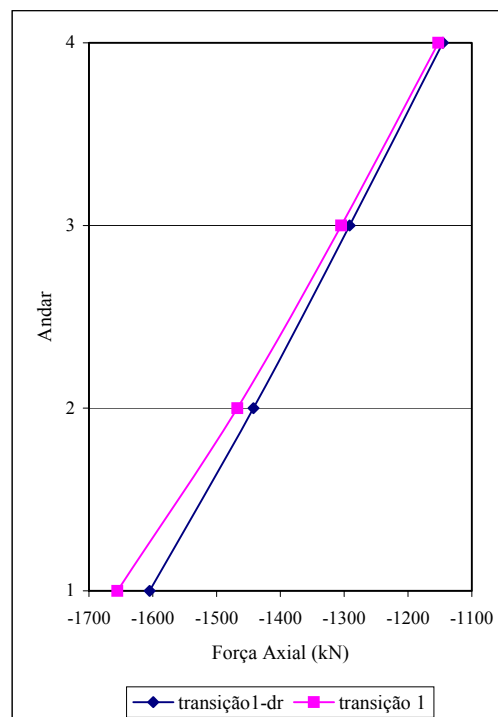
FIGURA 8.14 – Forças axiais no pilar P6 - 1º ao 4º andares
