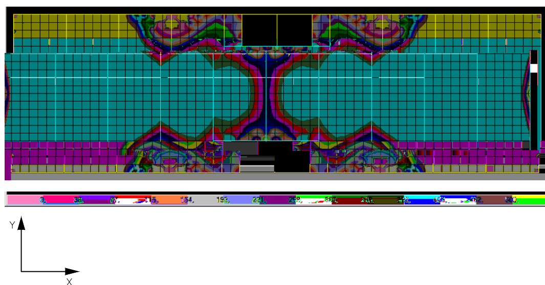
FIGURA 6.73 – Distribuição de tensões \sigma_{\text{máx}} < 500 \text{ N/cm}^2 devido às forças gravitacionais nominais na face inferior dos elementos de laje do 1º andar do modelo TRANSIÇÃO 1 (N/cm 2 )
