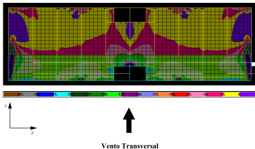
FIGURA 6.65 – Distribuição de tensões \sigma_{\min} na face superior dos elementos de laje do 1º andar do modelo TRANSIÇÃO 1 (N/cm 2 )
