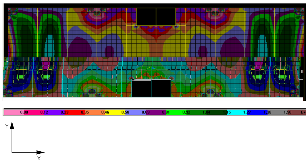
FIGURA 6.69 – Distribuição de tensões \sigma_{\text{máx}} devido às forças gravitacionais nominais na face inferior dos elementos de laje do 1º andar do modelo TRANSIÇÃO 1 (N/cm 2 )
