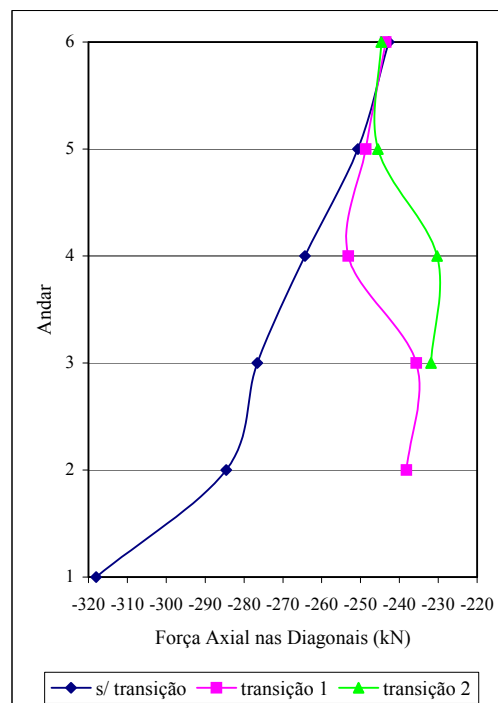
FIGURA 7.14 – Forças axiais nas diagonais comprimidas do contraventamento central - 1º ao 6º andares
