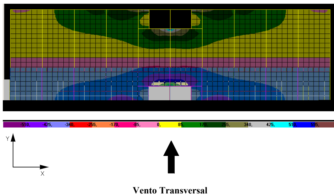
FIGURA 5.2 – Distribuição de tensões \sigma_x na face inferior dos elementos de laje do modelo SIMPLIFICADO ( \text{N/cm}^2 )
