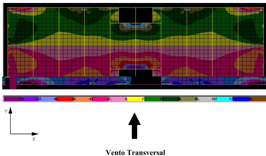
FIGURA 6.37 – Distribuição de tensões \sigma_x na face superior dos elementos de laje do 1º andar do modelo TRANSIÇÃO 1 (N/cm 2 )
