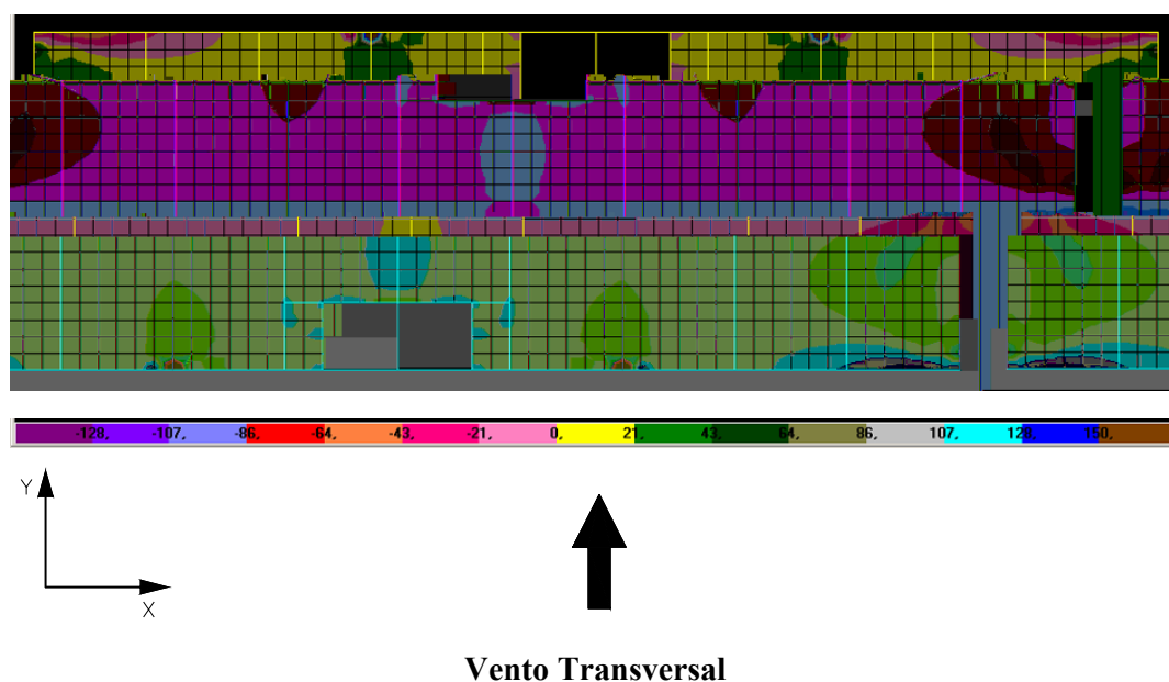
FIGURA 6.40 – Distribuição de tensões \sigma_x na face superior dos elementos de laje do 4º andar do modelo TRANSIÇÃO 1 (N/cm 2 )
