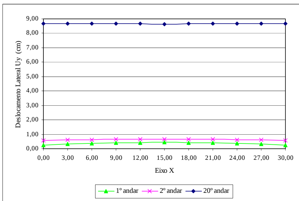
FIGURA 7.5 - Deslocamentos laterais U_y ao longo do eixo Y = 4,50 m nos 1º, 2º e 20º andares do modelo TRANSIÇÃO 1
