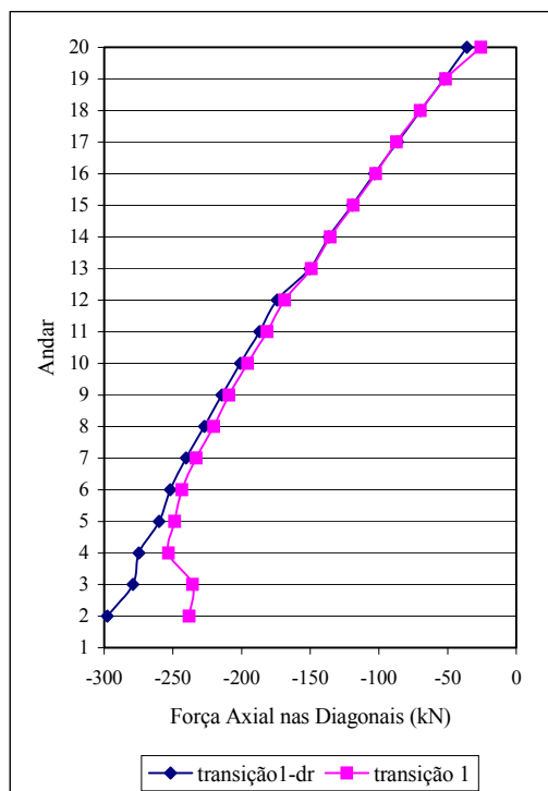
FIGURA 8.10 – Forças axiais nas diagonais comprimidas do contraventamento central
