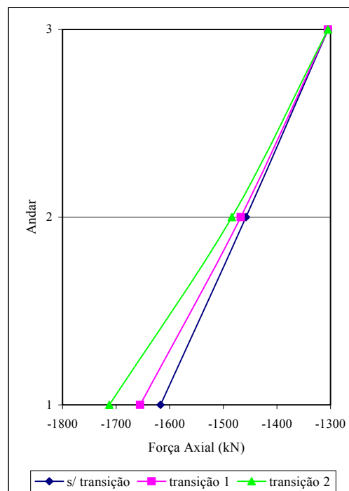
FIGURA 7.18 – Forças axiais no pilar P6 - 1º ao 3º andares
