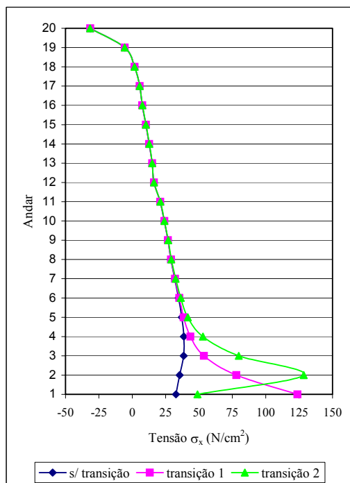
FIGURA 6.77 – Tensão \sigma_x no ponto A do elemento analisado
