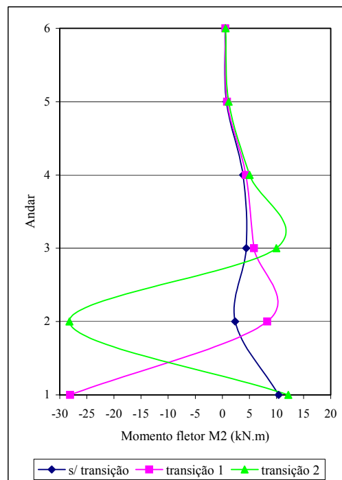
FIGURA 7.25 – Momento fletor M_2 (sistema local) nos nós superiores do pilar P7 em cada andar - 1º ao 6º andares
