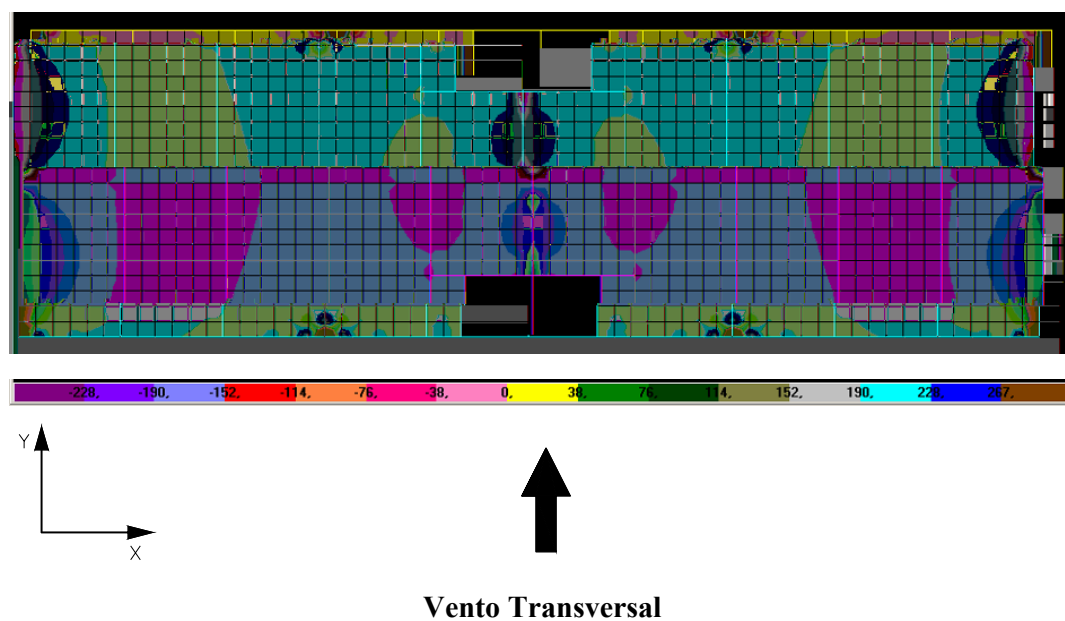
FIGURA 6.44 – Distribuição de tensões \sigma_y na face superior dos elementos de laje do 4º andar do modelo TRANSIÇÃO 1 (N/cm 2 )
