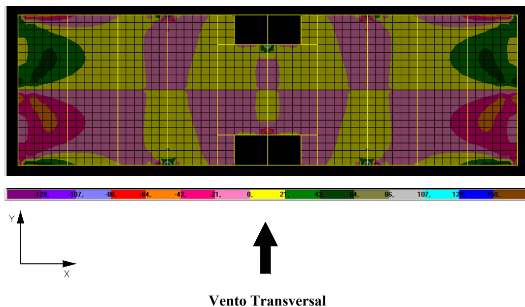
FIGURA 6.6 – Distribuição de tensões \sigma_x na face inferior dos elementos de laje do 3º andar do modelo SEM TRANSIÇÃO (N/cm 2 )
