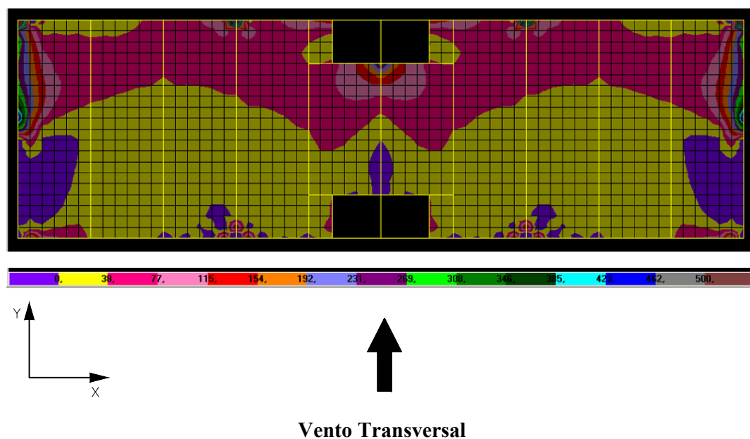
FIGURA 6.66 – Distribuição de tensões \sigma_{\text{máx}} na face superior dos elementos de laje do 1º andar do modelo TRANSIÇÃO 1 (N/cm 2 )
