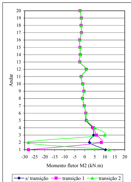
FIGURA 7.24 – Momento fletor M_2 (sistema local) nos nós superiores do pilar P7 em cada andar
