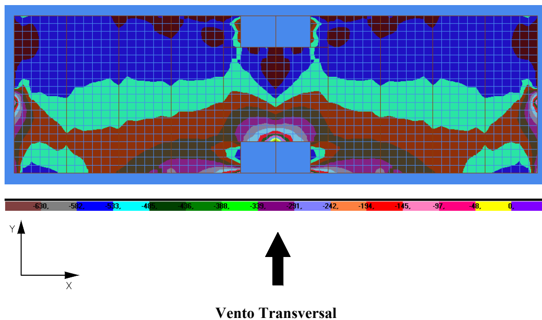
FIGURA 5.7 – Distribuição de tensões \sigma_{\min} na face superior dos elementos de laje do modelo SIMPLIFICADO ( \text{N/cm}^2 )
