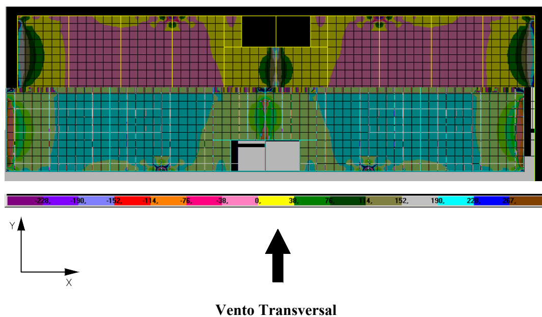
FIGURA 6.14 – Distribuição de tensões \sigma_y na face inferior dos elementos de laje do 1º andar do modelo SEM TRANSIÇÃO (N/cm 2 )
