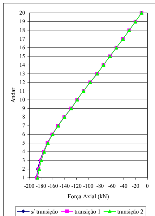
FIGURA 7.19 – Forças axiais no pilar P7
