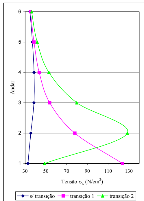
FIGURA 6.78 – Tensão \sigma_x no ponto A do elemento analisado – 1º ao 6º andares
