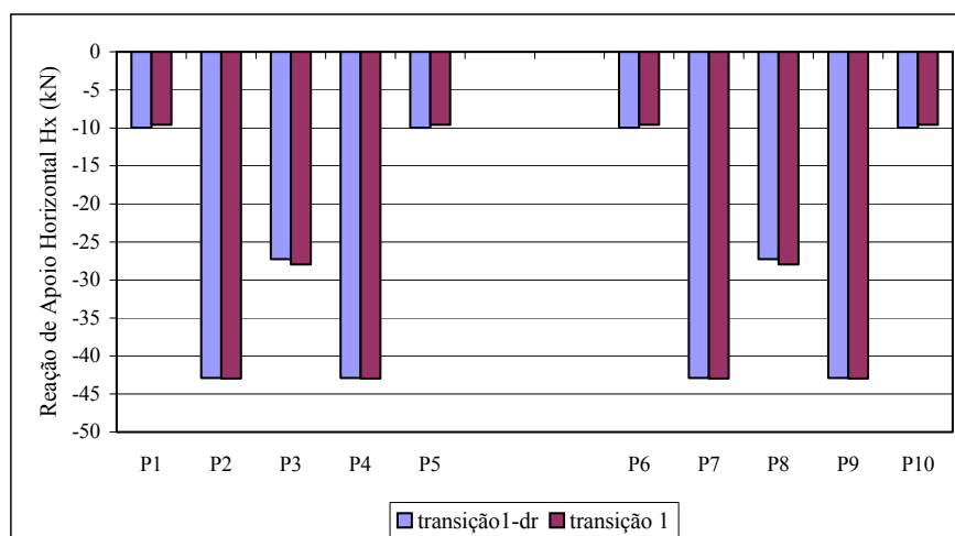
FIGURA 8.18 - Reações de apoio horizontais Hx na fundação dos pilares P1 a P10
