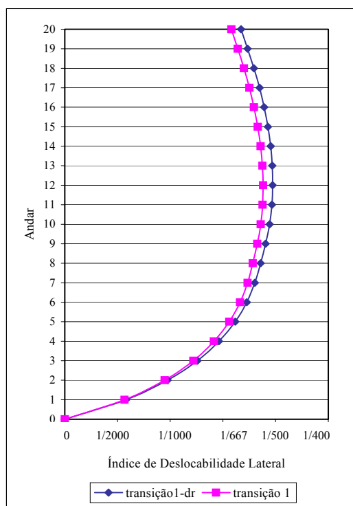
FIGURA 8.22 – Índice de deslocabilidade lateral - ponto (X = 15,00m; Y = 4,50m)
