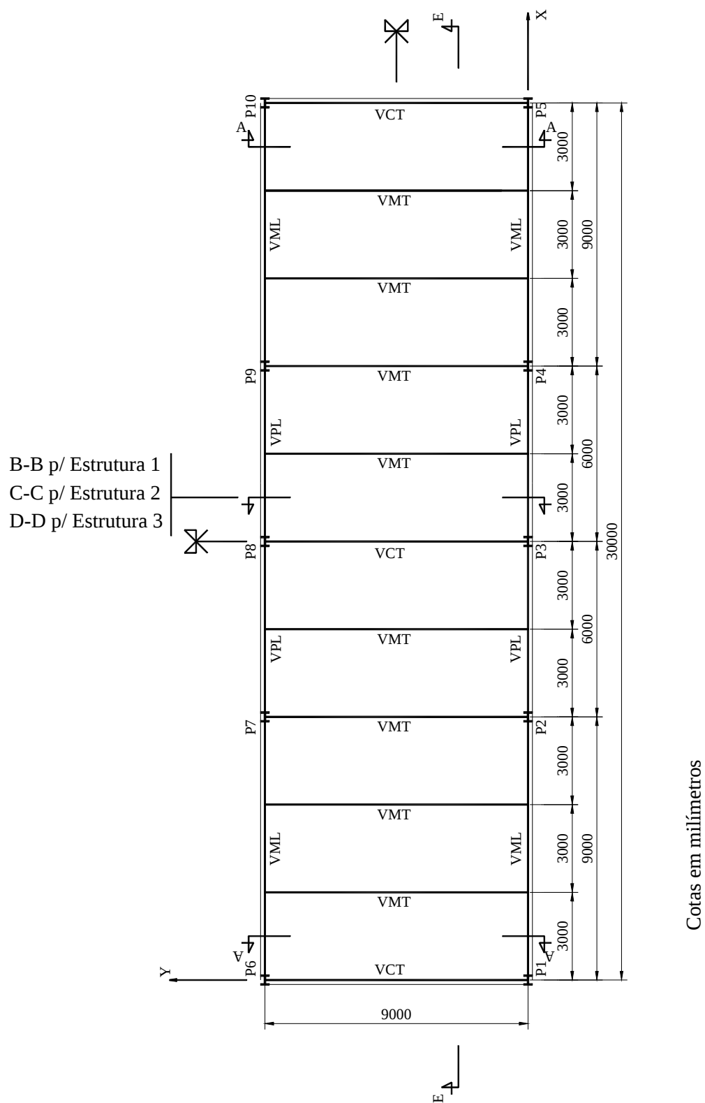
FIGURA 3.2 – Planta do 20º Andar das Estruturas 1, 2 e 3
