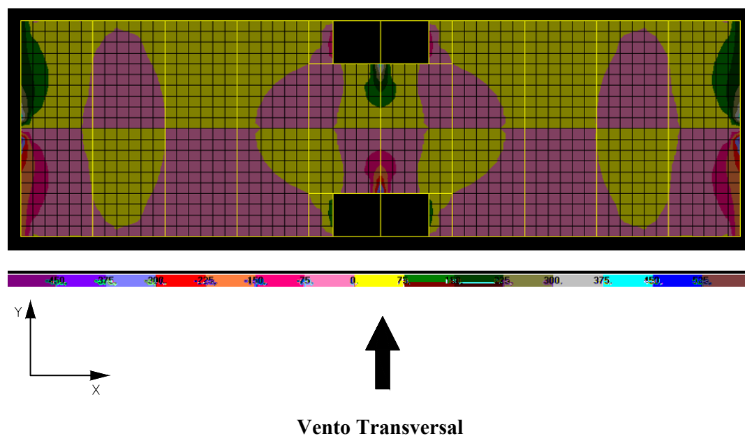
FIGURA 5.3 – Distribuição de tensões \sigma_y na face superior dos elementos de laje do modelo SIMPLIFICADO ( \text{N/cm}^2 )
