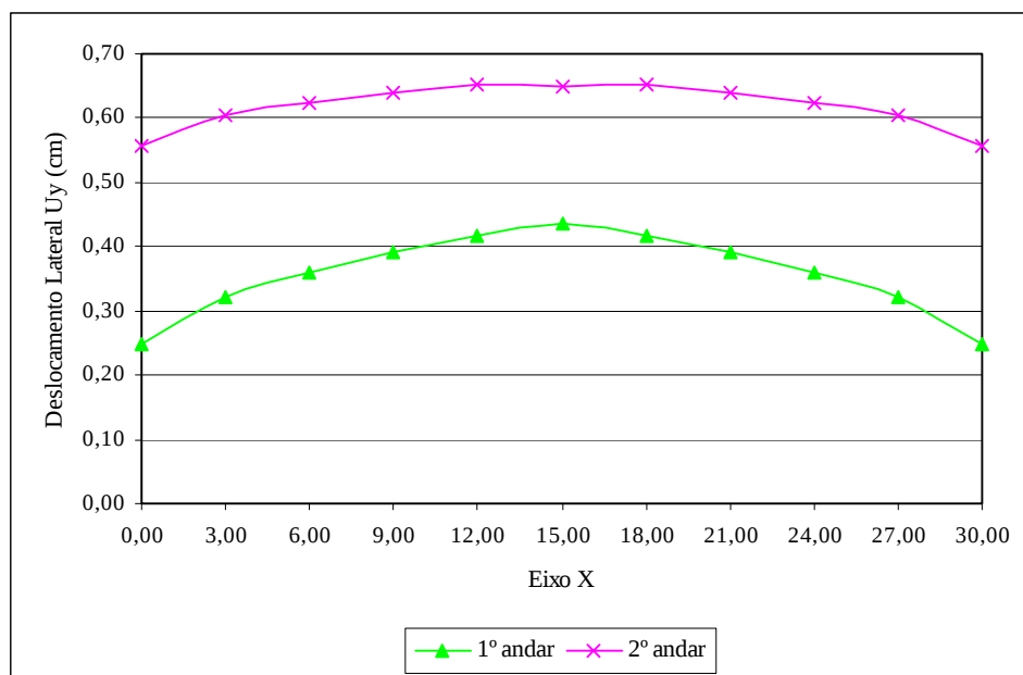
FIGURA 7.6 - Deslocamentos laterais U_y ao longo do eixo Y = 4,50 m nos 1º e 2º andares do modelo TRANSIÇÃO 1
