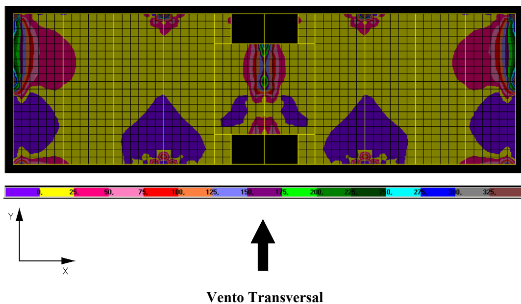
FIGURA 6.29 – Distribuição de tensões \sigma_{\max} na face superior dos elementos de laje do 3º andar do modelo SEM TRANSIÇÃO ( \text{N/cm}^2 )
