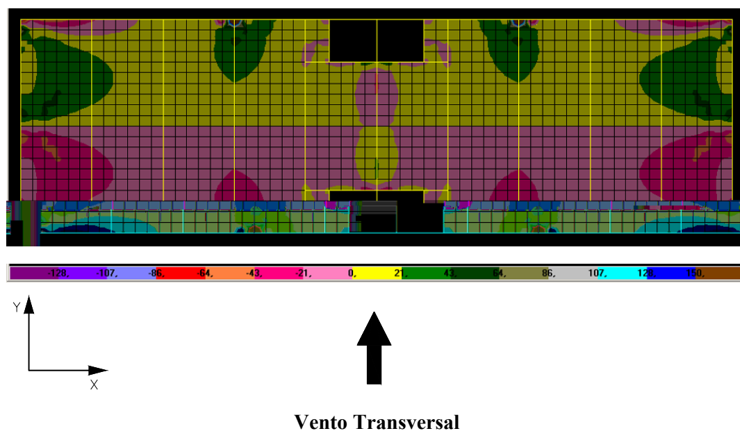
FIGURA 6.53 – Distribuição de tensões \sigma_x na face superior dos elementos de laje do 5º andar do modelo TRANSIÇÃO 2 ( \text{N/cm}^2 )
