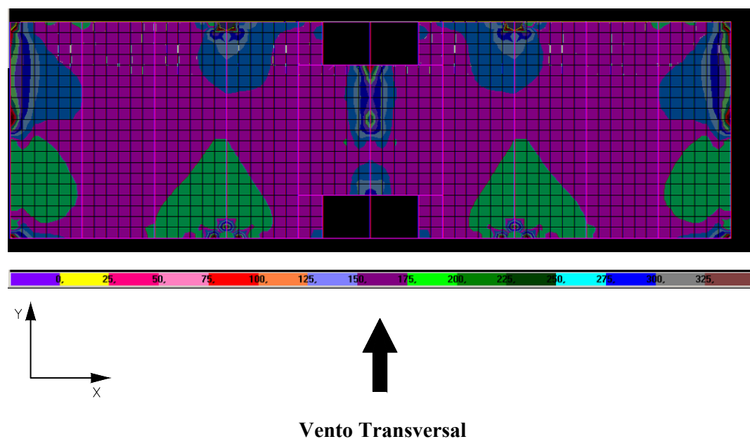
FIGURA 6.31 – Distribuição de tensões \sigma_{\text{máx}} na face superior dos elementos de laje do 10º andar do modelo SEM TRANSIÇÃO (N/cm 2 )
