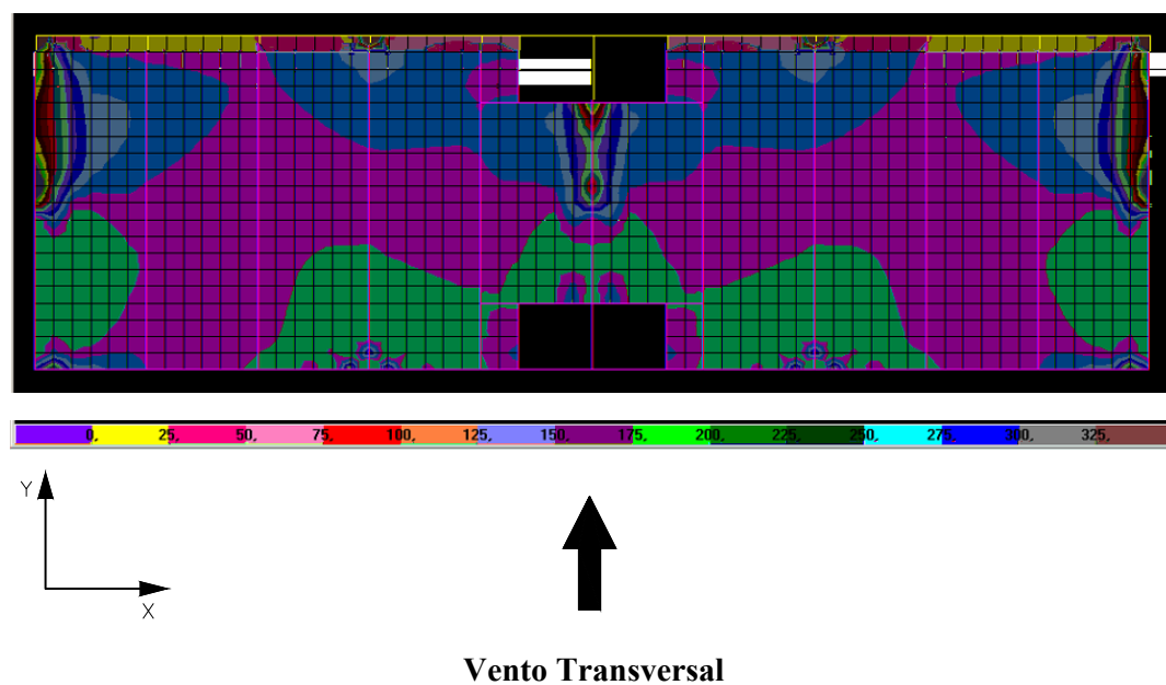
FIGURA 6.61 – Distribuição de tensões \sigma_{\max} na face superior dos elementos de laje do 3º andar do modelo TRANSIÇÃO 2 ( \text{N/cm}^2 )
