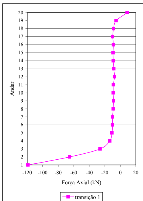
FIGURA 8.12 – Forças axiais nas vigas longitudinais junto ao pilar P3 no eixo Y = 0,00 m
