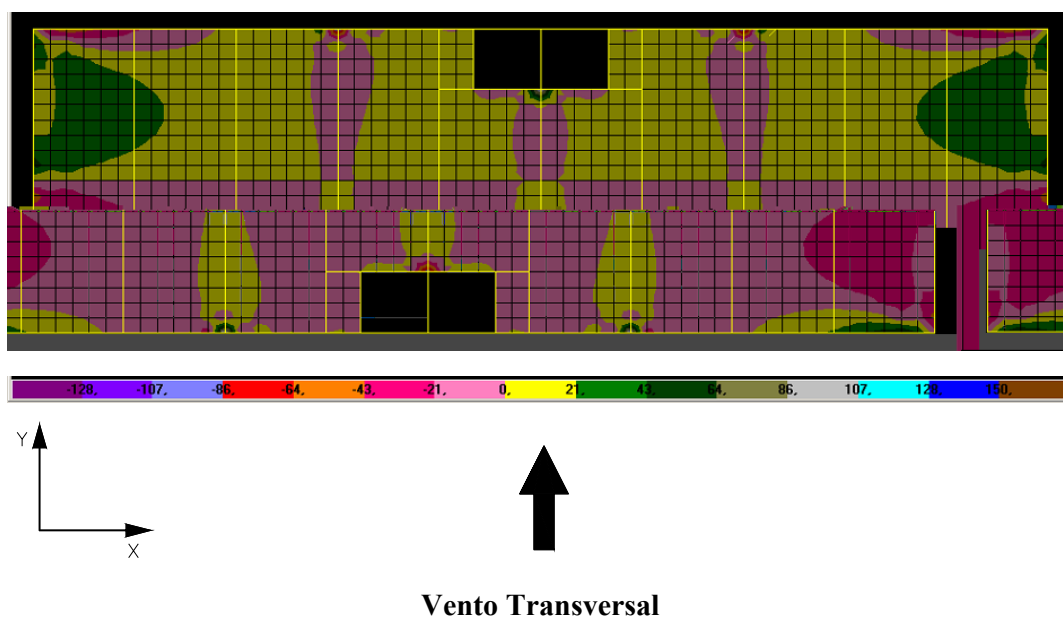
FIGURA 6.2 – Distribuição de tensões \sigma_x na face inferior dos elementos de laje do 1º andar do modelo SEM TRANSIÇÃO (N/cm 2 )
