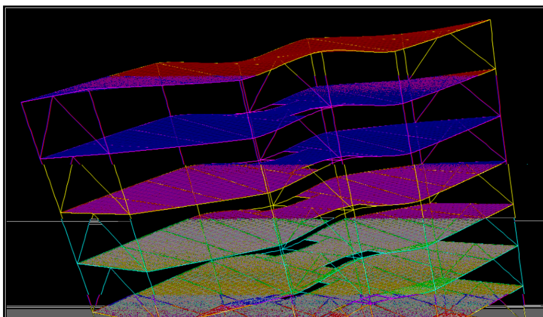
FIGURA 6.75 – Deformação das lajes, vigas e pilares dos andares superiores do modelo TRANSIÇÃO 1 devido às forças de vento transversal
