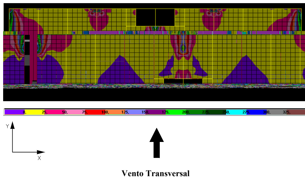
FIGURA 6.63 – Distribuição de tensões \sigma_{\text{máx}} na face superior dos elementos de laje do 5º andar do modelo TRANSIÇÃO 2 ( \text{N/cm}^2 )
