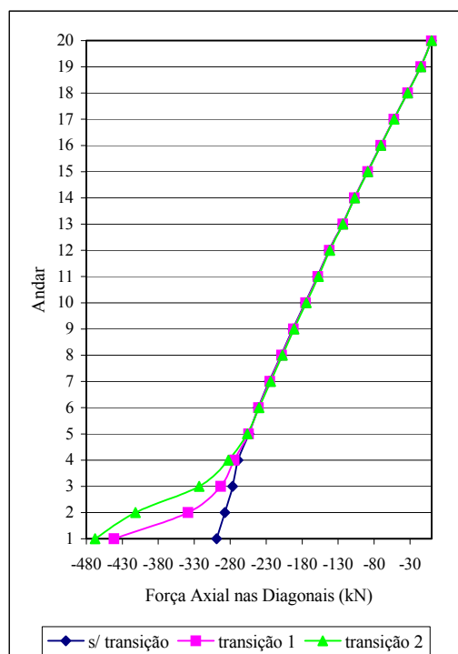
FIGURA 7.11 – Forças axiais nas diagonais comprimidas dos contraventamentos das extremidades
