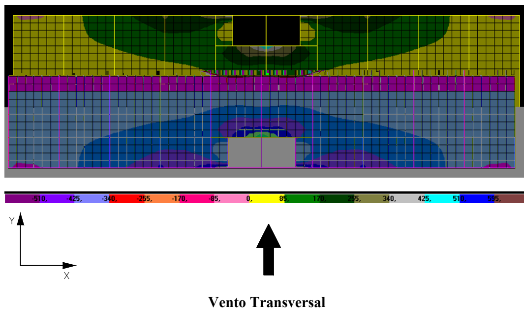
FIGURA 5.1 – Distribuição de tensões \sigma_x na face superior dos elementos de laje do modelo SIMPLIFICADO ( \text{N/cm}^2 )
