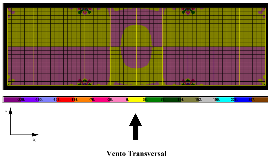
FIGURA 6.23 – Distribuição de tensões \sigma_y na face superior dos elementos de laje do 20º andar do modelo SEM TRANSIÇÃO (N/cm 2 )
