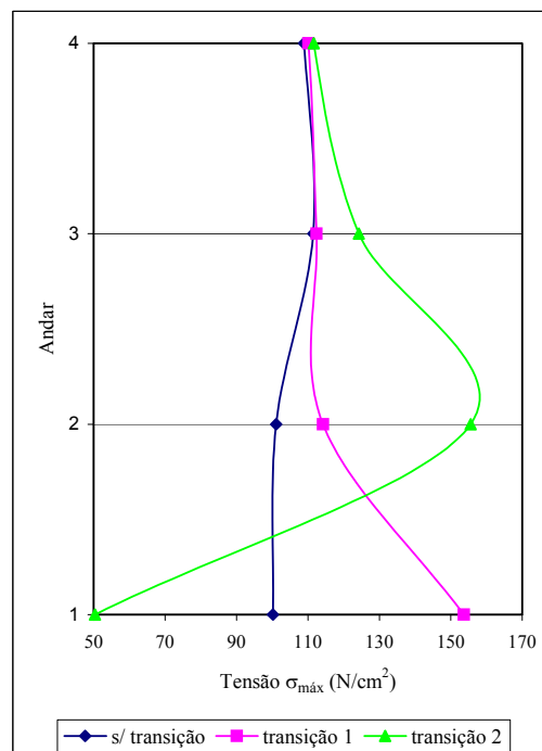
FIGURA 6.82 – Tensão \sigma_{\max} no ponto A do elemento analisado – 1º ao 4º andares
