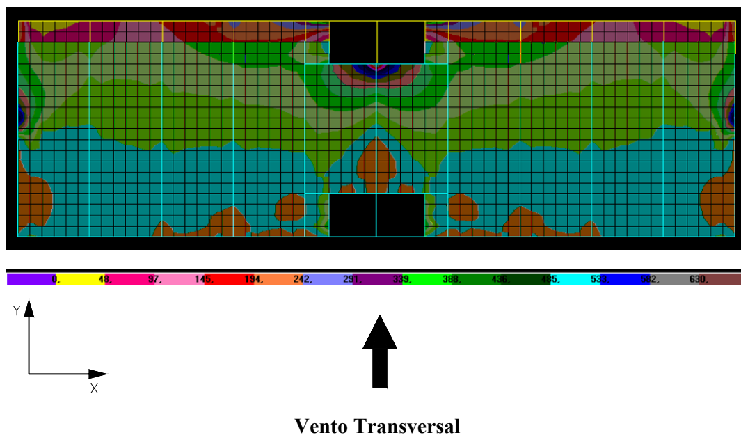
FIGURA 5.5 – Distribuição de tensões \sigma_{\text{máx}} na face superior dos elementos de laje do modelo SIMPLIFICADO (N/cm 2 )
