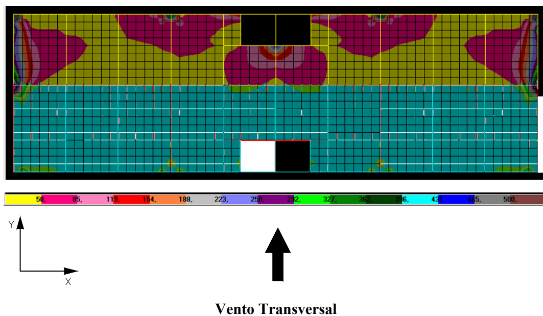
FIGURA 6.70 – Distribuição de tensões \sigma_{\max} > 50 \text{ N/cm}^2 na face superior dos elementos de laje do 1º andar do modelo TRANSIÇÃO 1 ( \text{N/cm}^2 )
