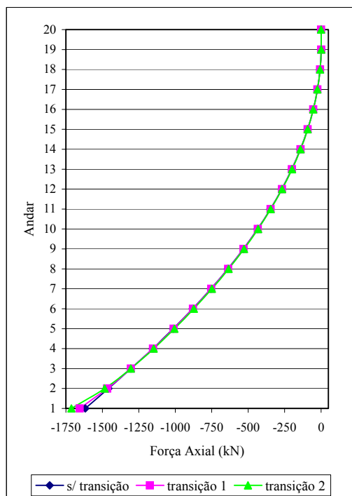
FIGURA 7.17 – Forças axiais no pilar P6
