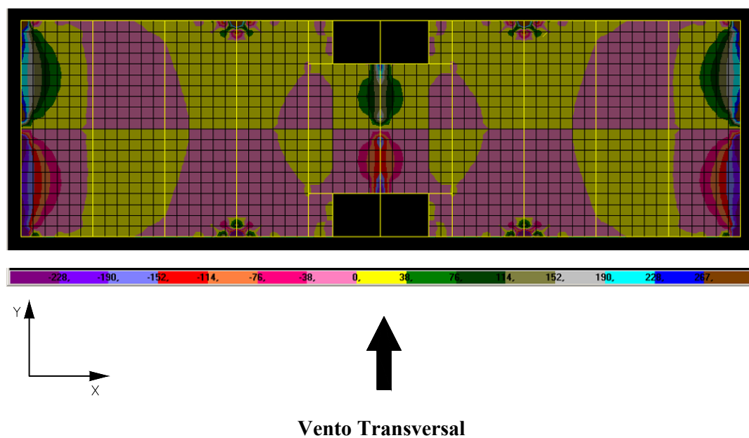
FIGURA 6.57 – Distribuição de tensões \sigma_y na face superior dos elementos de laje do 4º andar do modelo TRANSIÇÃO 2 (N/cm 2 )
