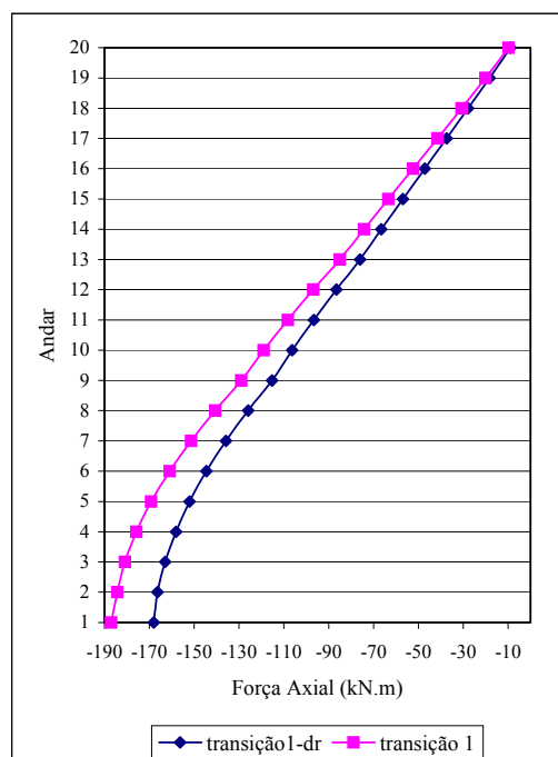
FIGURA 8.15 – Forças axiais no pilar P7
