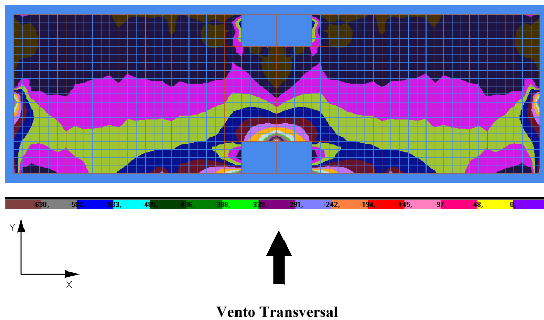
FIGURA 5.8 – Distribuição de tensões \sigma_{\min} na face inferior dos elementos de laje do modelo SIMPLIFICADO ( \text{N/cm}^2 )
