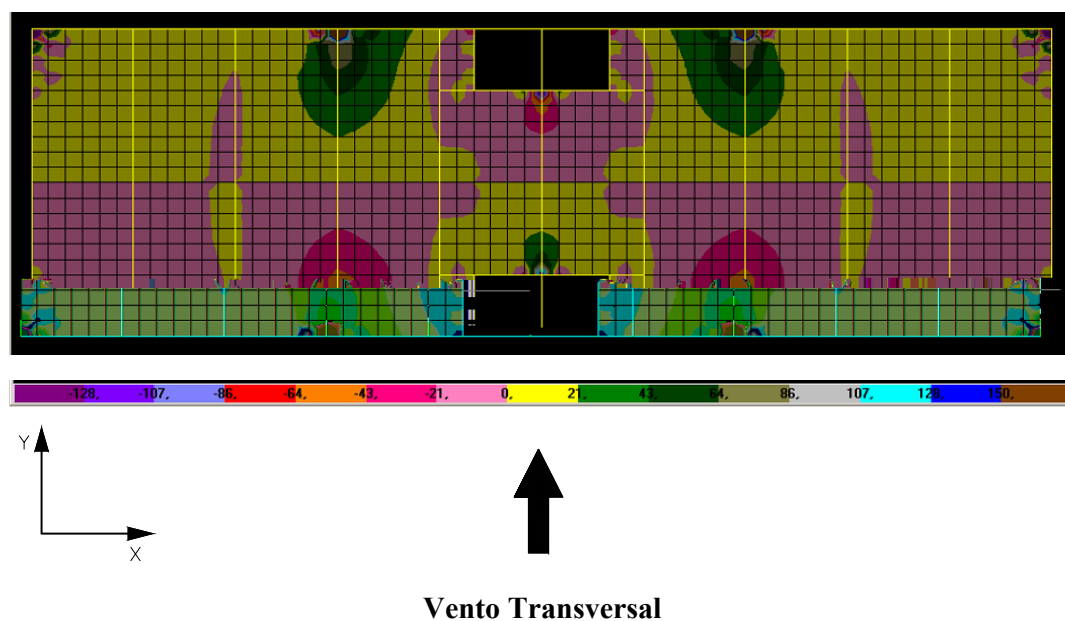
FIGURA 6.9 – Distribuição de tensões \sigma_x na face superior dos elementos de laje do 19º andar do modelo SEM TRANSIÇÃO (N/cm 2 )
