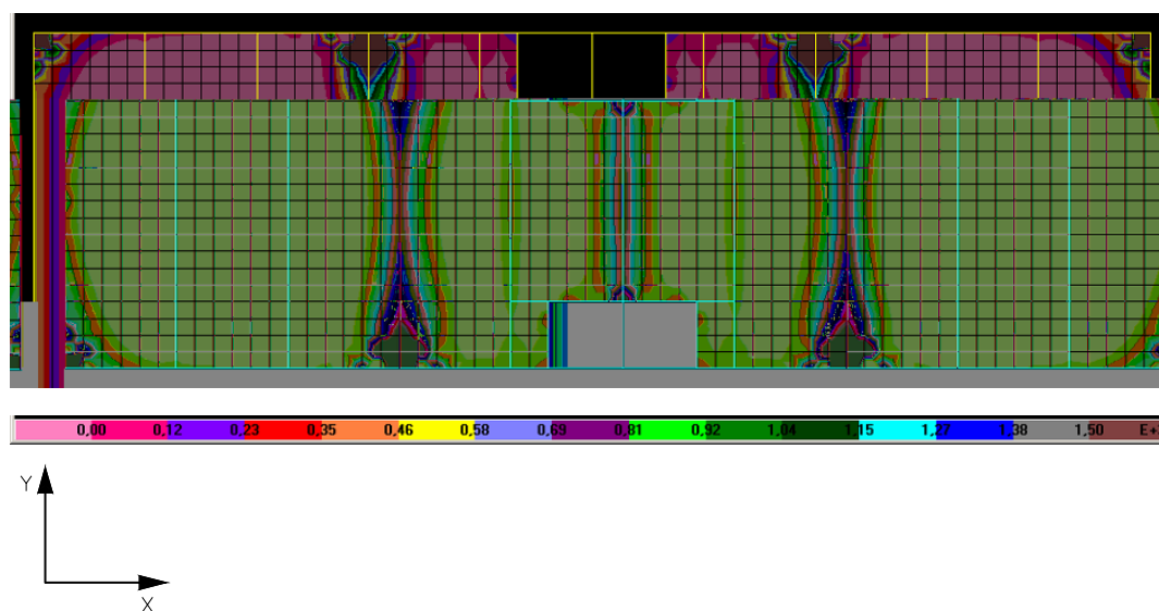
FIGURA 6.68 – Distribuição de tensões \sigma_{\text{máx}} devido às forças gravitacionais nominais na face superior dos elementos de laje do 1º andar do modelo TRANSIÇÃO 1 (N/cm 2 )
