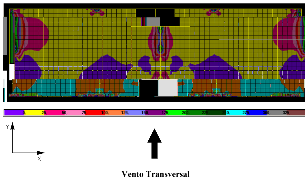
FIGURA 6.25 – Distribuição de tensões \sigma_{\text{máx}} na face superior dos elementos de laje do 1º andar do modelo SEM TRANSIÇÃO (N/cm 2 )
