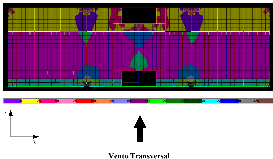
FIGURA 6.34 – Distribuição de tensões \sigma_{\text{máx}} na face inferior dos elementos de laje do 19º andar do modelo SEM TRANSIÇÃO (N/cm 2 )
