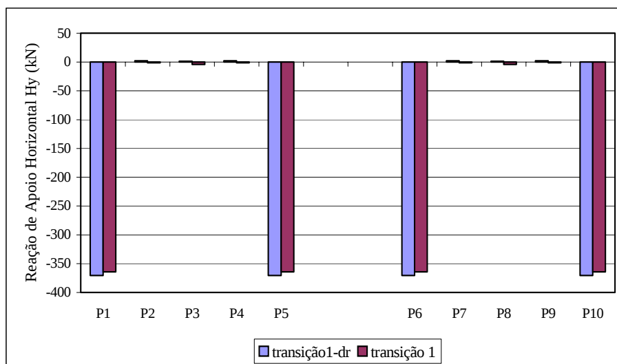
FIGURA 8.1 - Reações de apoio horizontais H_y na fundação dos pilares P1 a P10
