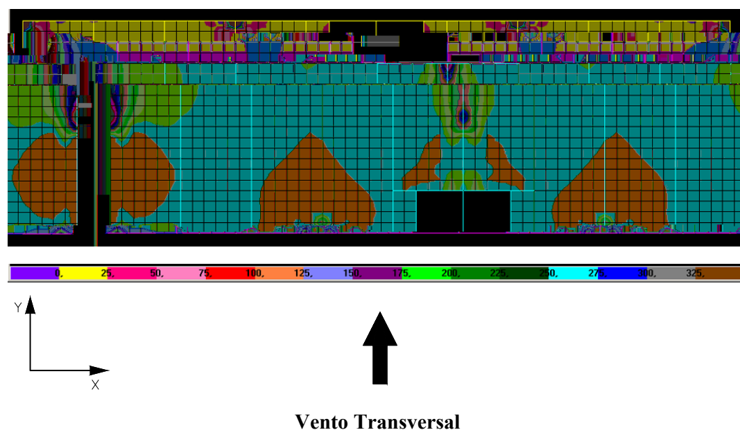
FIGURA 6.48 – Distribuição de tensões \sigma_{\max} na face superior dos elementos de laje do 4º andar do modelo TRANSIÇÃO 1 ( \text{N}/\text{cm}^2 )
