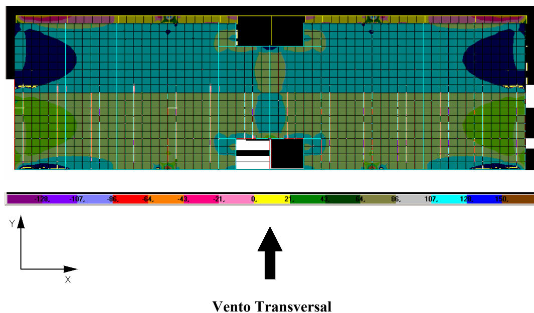
FIGURA 6.3 – Distribuição de tensões \sigma_x na face superior dos elementos de laje do 2º andar do modelo SEM TRANSIÇÃO (N/cm 2 )
