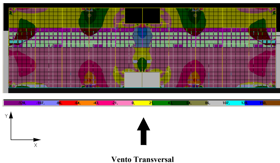
FIGURA 6.7 – Distribuição de tensões \sigma_x na face superior dos elementos de laje do 10º andar do modelo SEM TRANSIÇÃO (N/cm 2 )
