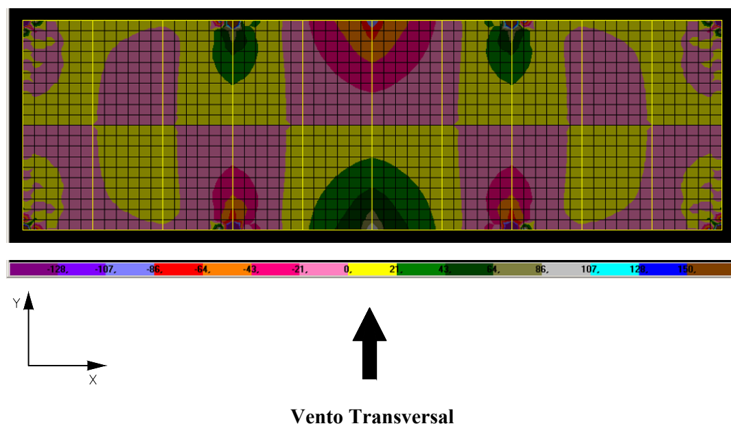
FIGURA 6.11 – Distribuição de tensões \sigma_x na face superior dos elementos de laje do 20º andar do modelo SEM TRANSIÇÃO ( \text{N/cm}^2 )
