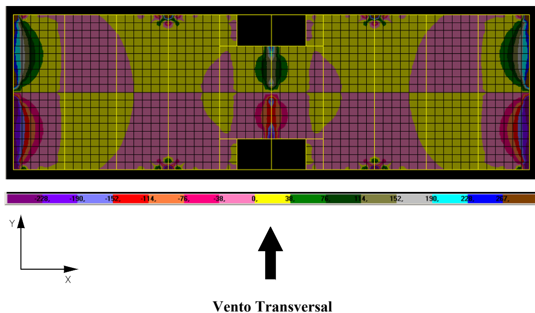
FIGURA 6.56 – Distribuição de tensões \sigma_y na face superior dos elementos de laje do 3º andar do modelo TRANSIÇÃO 2 ( \text{N/cm}^2 )
