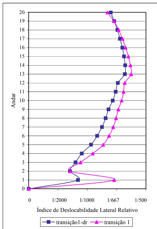
FIGURA 8.6 – Índice de deslocabilidade lateral - ponto ( X = 15,00 m; Y = 4,50 m)
