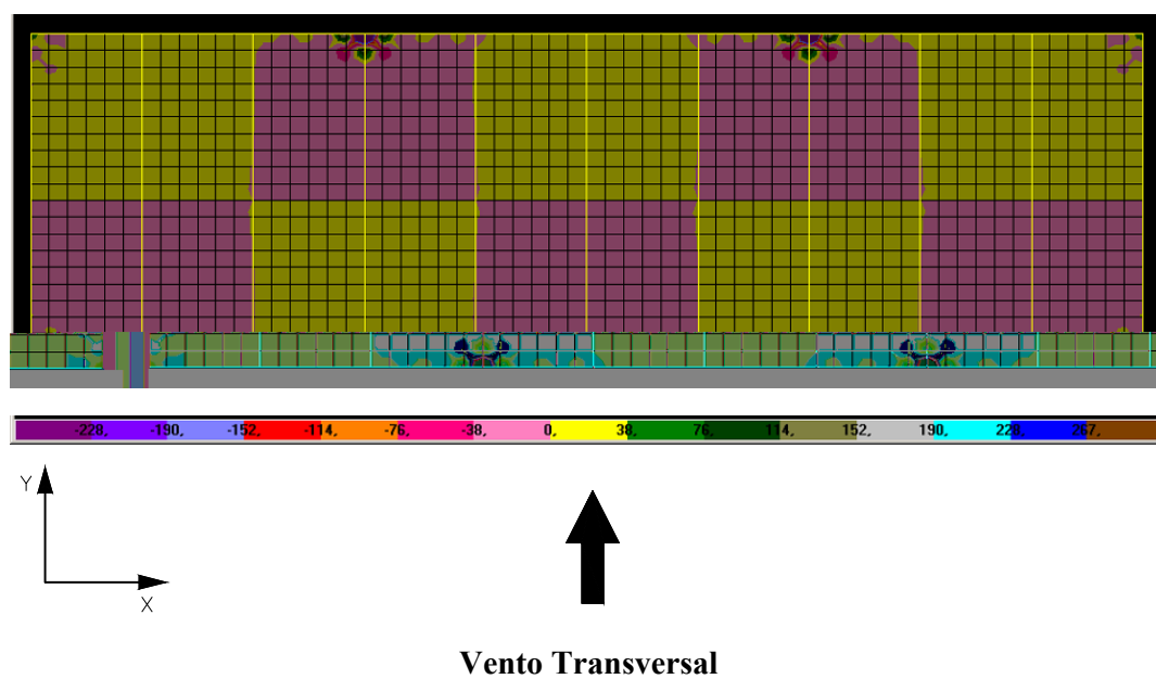
FIGURA 6.24 – Distribuição de tensões \sigma_y na face inferior dos elementos de laje do 20º andar do modelo SEM TRANSIÇÃO (N/cm 2 )
