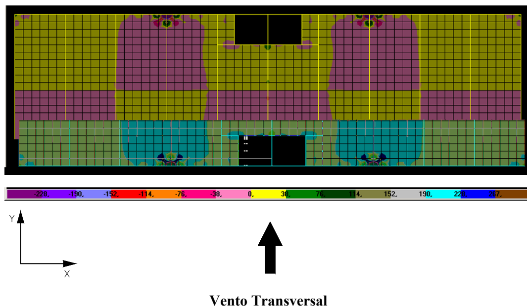
FIGURA 6.22 – Distribuição de tensões \sigma_y na face inferior dos elementos de laje do 19º andar do modelo SEM TRANSIÇÃO ( \text{N/cm}^2 )
