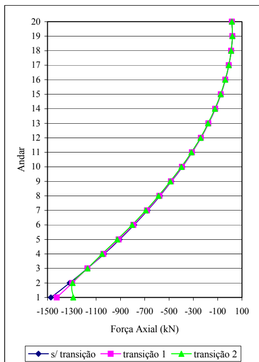
FIGURA 7.20 – Forças axiais no pilar P8
