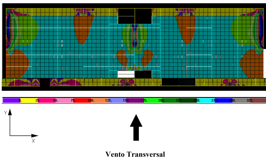
FIGURA 6.30 – Distribuição de tensões \sigma_{\max} na face inferior dos elementos de laje do 3º andar do modelo SEM TRANSIÇÃO ( \text{N/cm}^2 )
