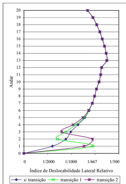
FIGURA 7.10 – Índice de deslocabilidade lateral relativo - ponto (X = 15,00m; Y = 4,50m)
