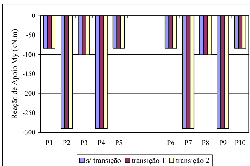
FIGURA 7.38 - Reações de apoio My na fundação dos pilares P1 a P10
