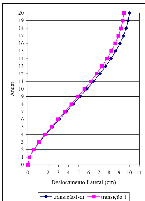
FIGURA 8.21 – Deslocamentos laterais U_x no ponto ( X = 15,00 m; Y = 4,50 m)
