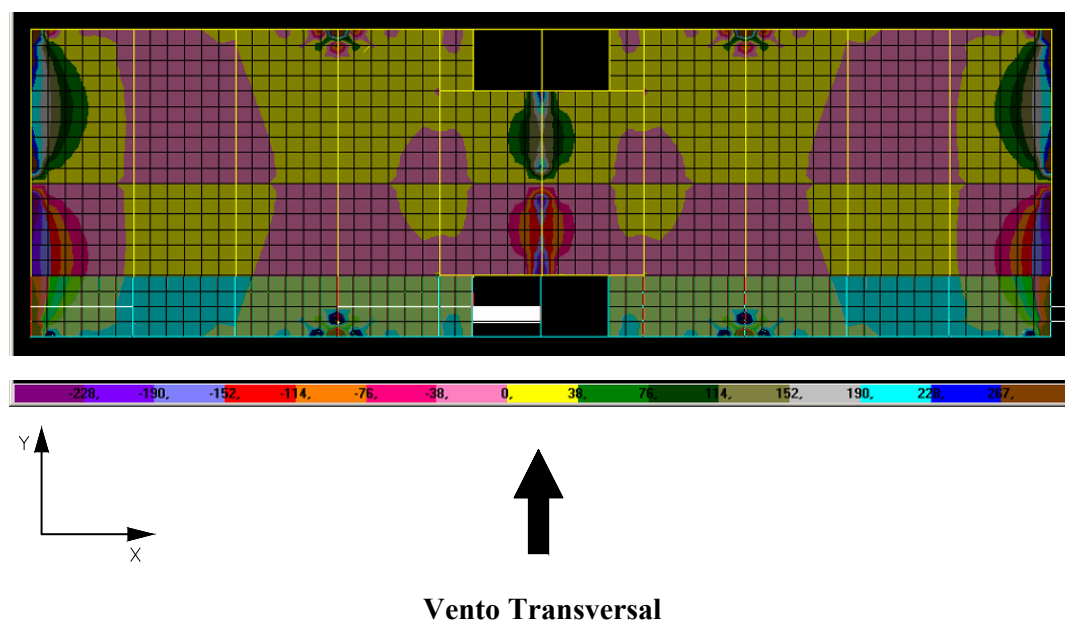
FIGURA 6.17 – Distribuição de tensões \sigma_y na face superior dos elementos de laje do 3º andar do modelo SEM TRANSIÇÃO (N/cm 2 )
