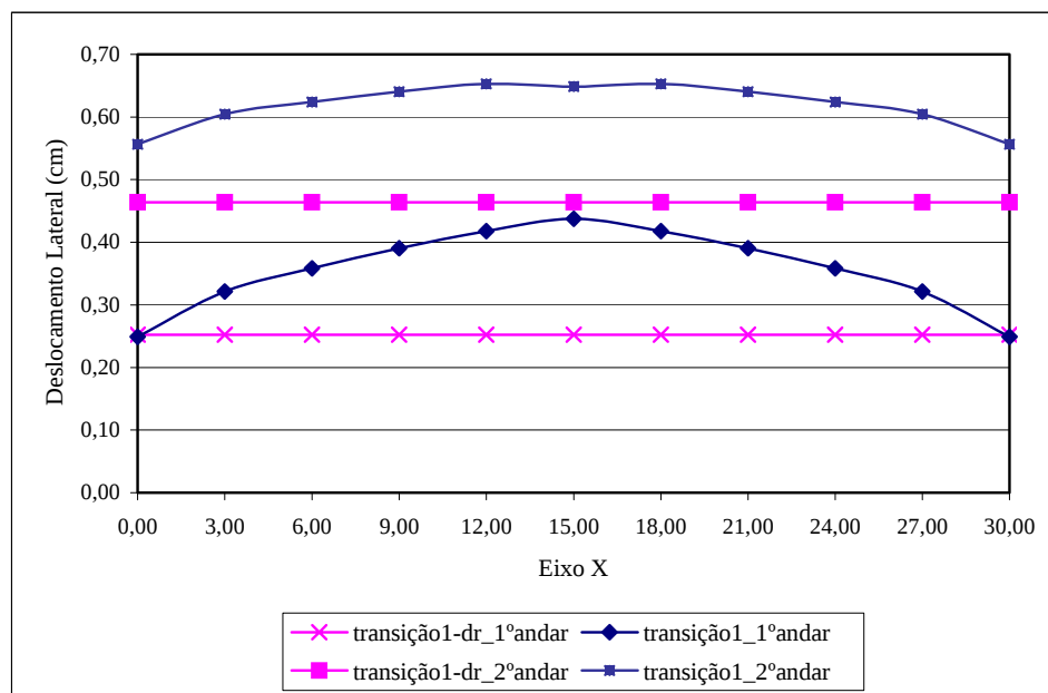
FIGURA 8.5 - Deslocamentos laterais U_y no eixo Y = 4,50 m nos 1º e 2º andares dos modelos TRANSIÇÃO 1 e TRANSIÇÃO 1 - DR
