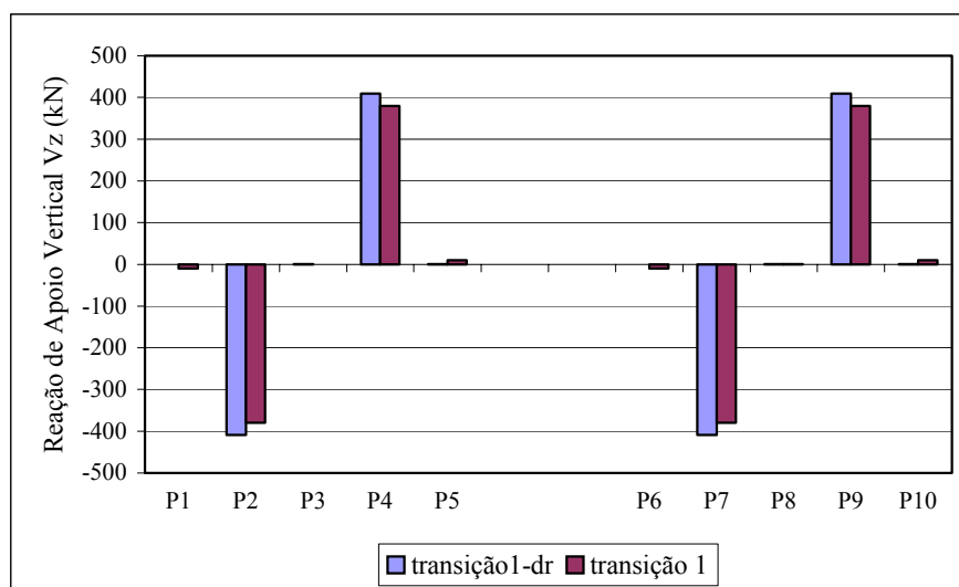
FIGURA 8.19 - Reações de apoio verticais na fundação dos pilares P1 a P10
