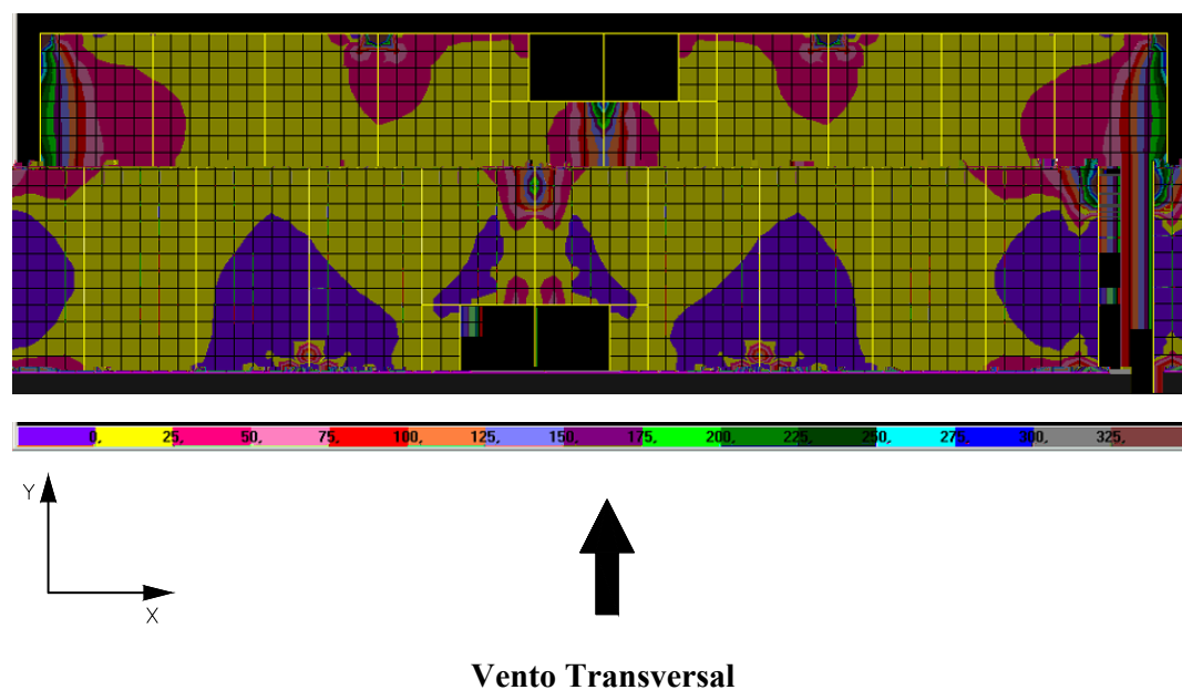
FIGURA 6.62 – Distribuição de tensões \sigma_{\text{máx}} na face superior dos elementos de laje do 4º andar do modelo TRANSIÇÃO 2 ( \text{N/cm}^2 )
