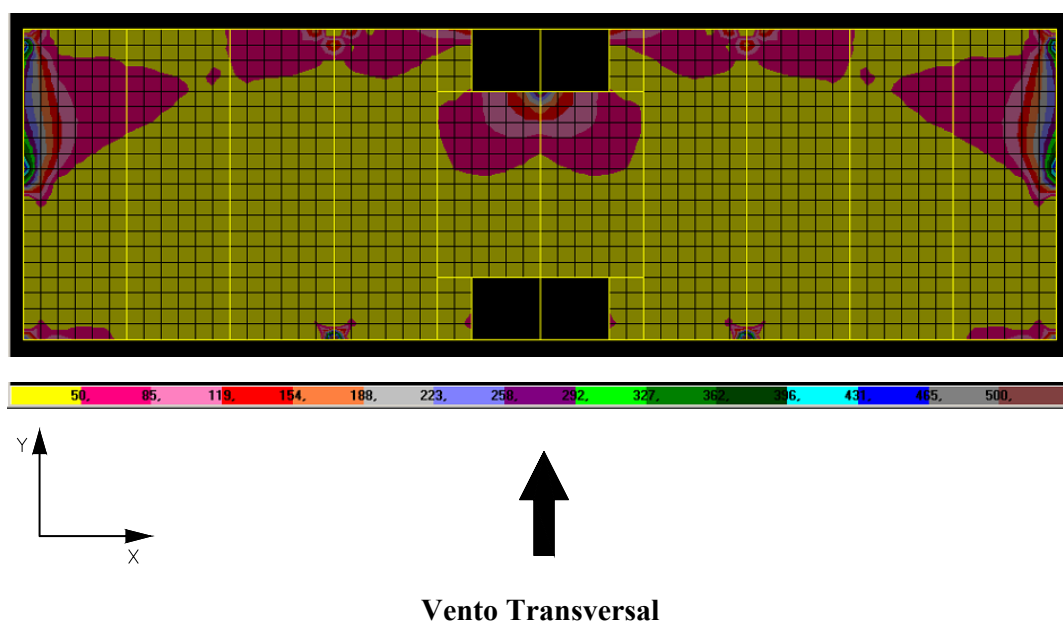
FIGURA 6.71 – Distribuição de tensões \sigma_{\max} > 50 \text{ N/cm}^2 na face inferior dos elementos de laje do 1º andar do modelo TRANSIÇÃO 1 ( \text{N/cm}^2 )
