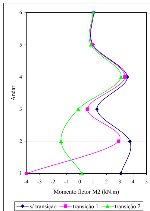
FIGURA 7.23 – Momento fletor M2 (sistema local) nos nós superiores do pilar P6 em cada andar - 1º ao 6º andares
