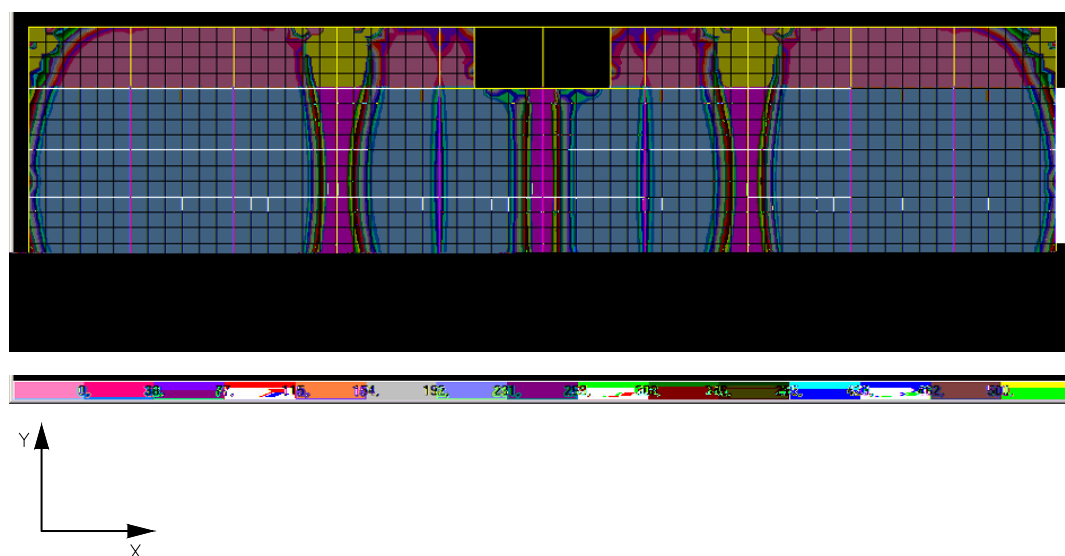
FIGURA 6.72 – Distribuição de tensões \sigma_{\text{máx}} < 500 \text{ N/cm}^2 devido às forças gravitacionais nominais na face superior dos elementos de laje do 1º andar do modelo TRANSIÇÃO 1 (N/cm 2 )
