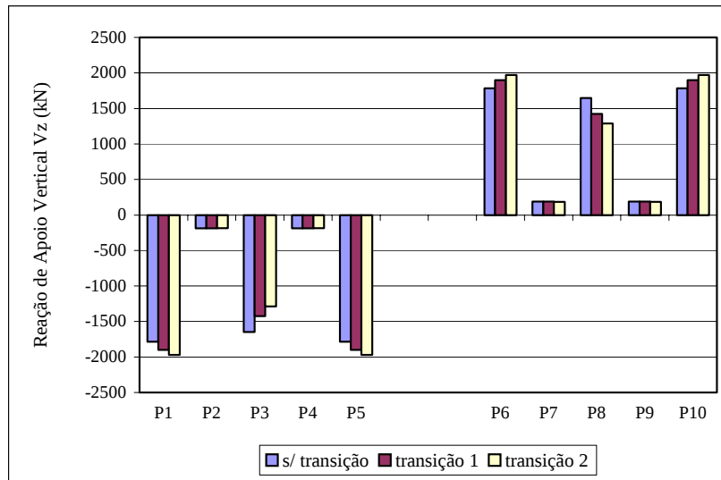
FIGURA 7.2 - Reações de apoio verticais Vz na fundação dos pilares P1 a P10
