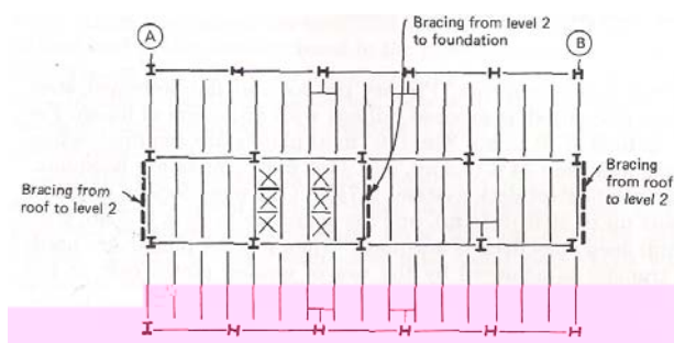
FIGURA 2.1 – Planta do pavimento tipo do edifício
