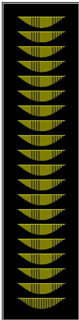
FIGURA 7.32 – Momento fletor M_3 devido às cargas gravitacionais nas vigas do eixo X = 6,00 m do modelo TRANSICÃO 1
