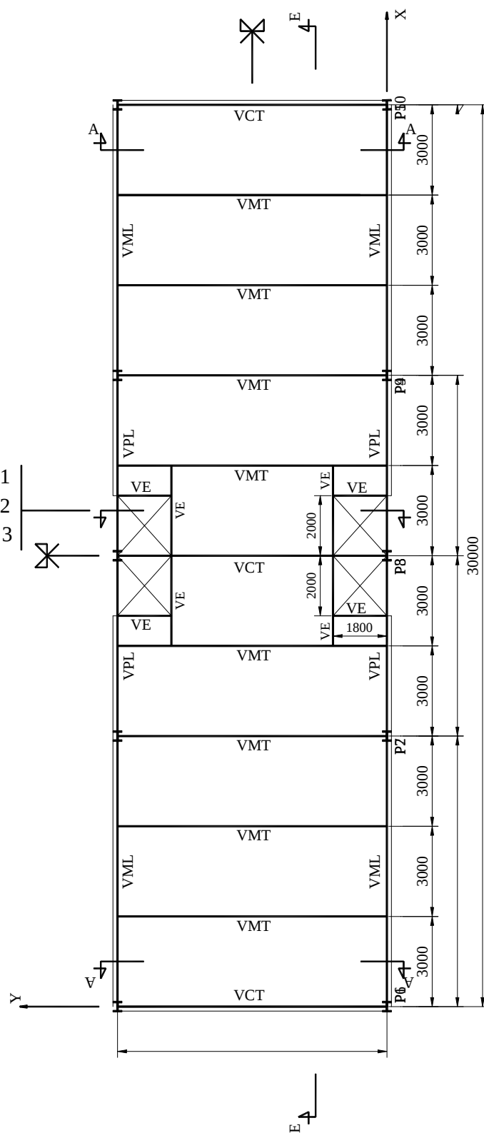
FIGURA 3.1 – Planta do Andar Tipo das Estruturas 1, 2 e 3
