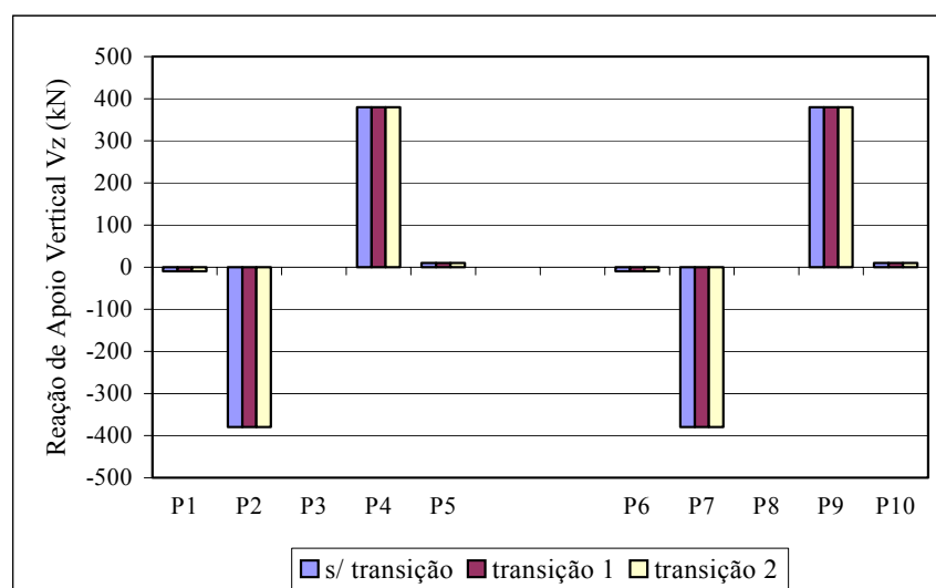
FIGURA 7.37 - Reações de apoio verticais Vz na fundação dos pilares P1 a P10
