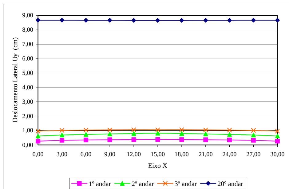
FIGURA 7.7 - Deslocamentos laterais U_y ao longo do eixo Y = 4,50 m nos 1º, 2º, 3º e 20º andares do modelo TRANSIÇÃO 2
