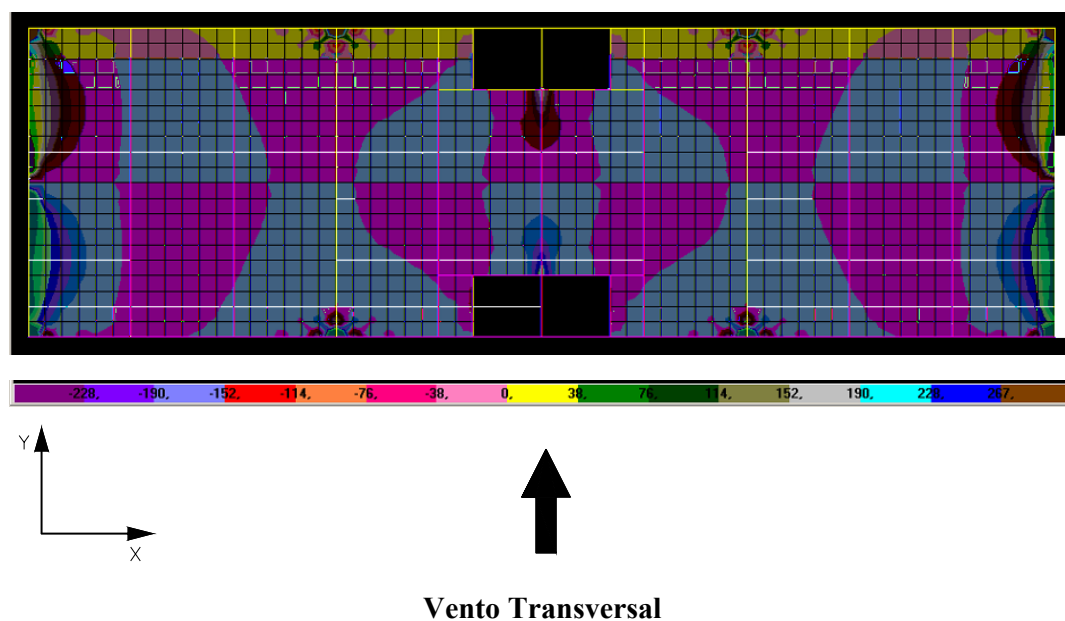
FIGURA 6.55 – Distribuição de tensões \sigma_y na face superior dos elementos de laje do 2º andar do modelo TRANSIÇÃO 2 ( \text{N/cm}^2 )
