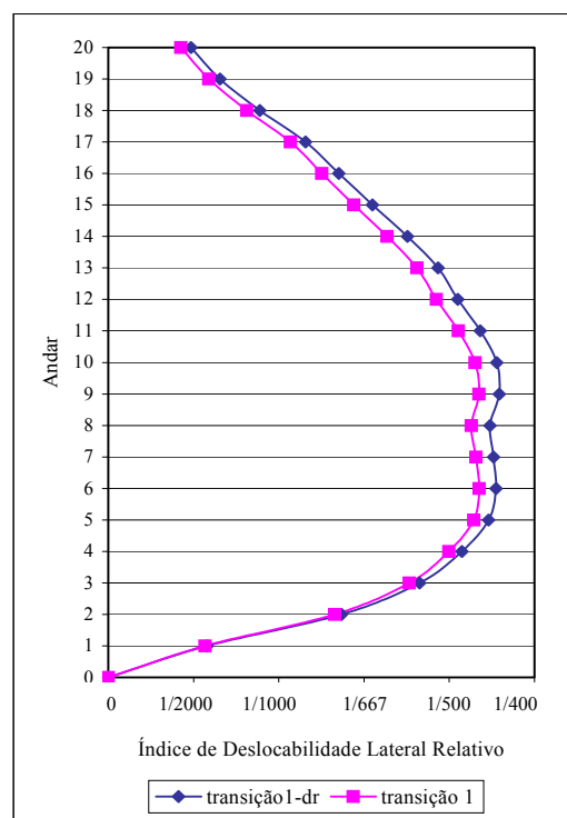
FIGURA 8.23 – Índice de deslocabilidade lateral relativo - ponto (X = 15,00m; Y = 4,50m)
