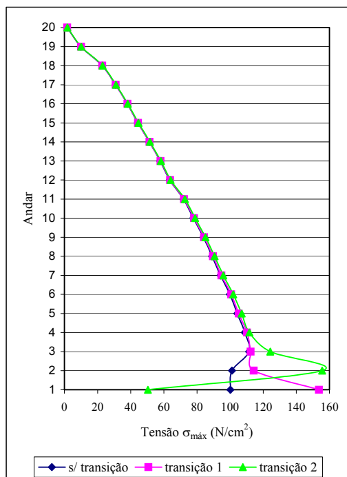
FIGURA 6.81 – Tensão \sigma_{\max} no ponto A do elemento analisado
