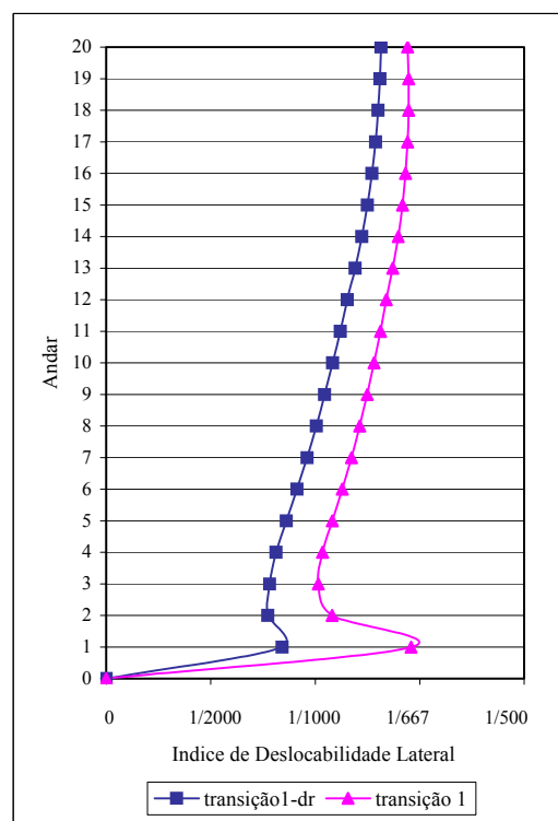
FIGURA 8.7 – Índice de deslocabilidade lateral relativo - ponto ( X = 15,00 m; Y = 4,50 m)
