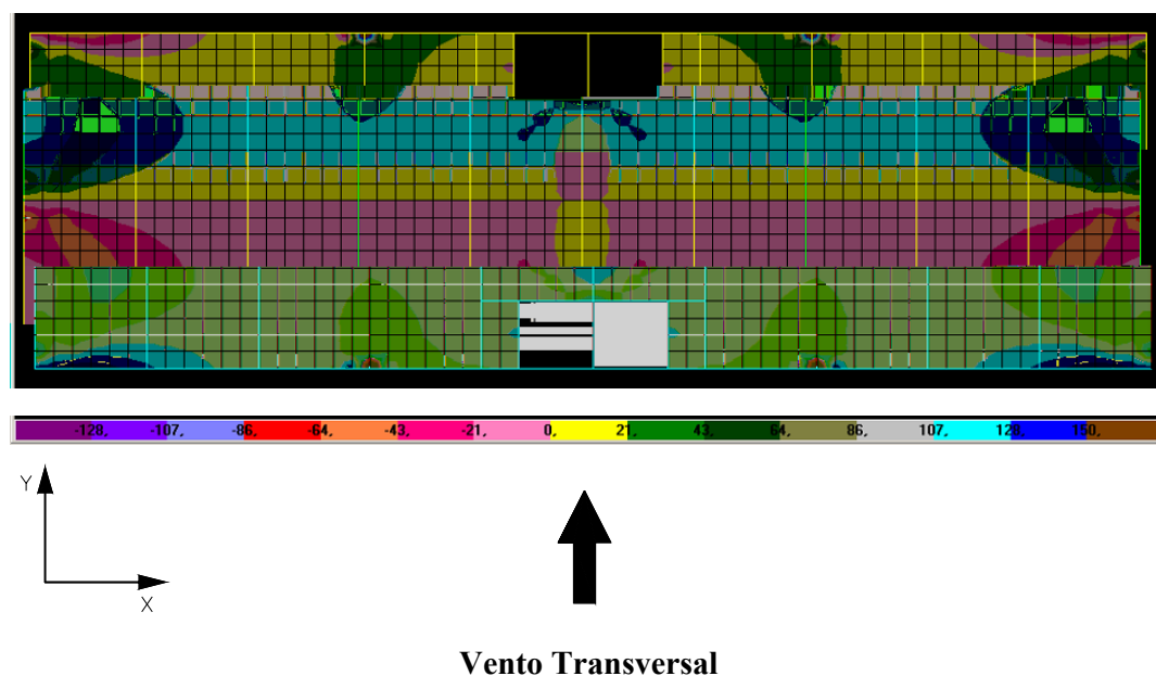
FIGURA 6.39 – Distribuição de tensões \sigma_x na face superior dos elementos de laje do 3º andar do modelo TRANSIÇÃO 1 (N/cm 2 )
