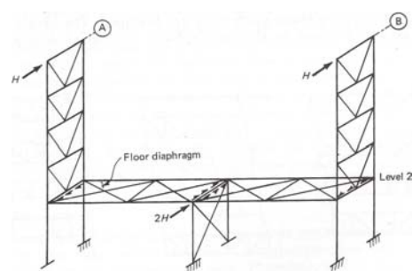
FIGURA 2.2 – Esquema de transferência de forças entre os contraventamentos do edifício
