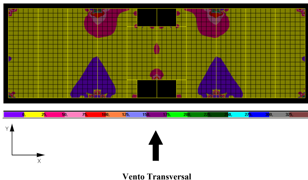
FIGURA 6.33 – Distribuição de tensões \sigma_{\text{máx}} na face superior dos elementos de laje do 19º andar do modelo SEM TRANSIÇÃO (N/cm 2 )
