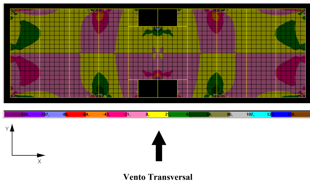
FIGURA 6.8 – Distribuição de tensões \sigma_x na face inferior dos elementos de laje do 10º andar do modelo SEM TRANSIÇÃO (N/cm 2 )
