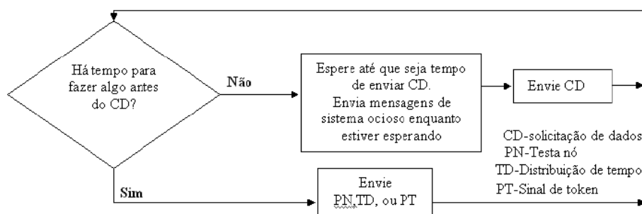
Figura 29: Fluxograma do algoritmo de escalonamento
