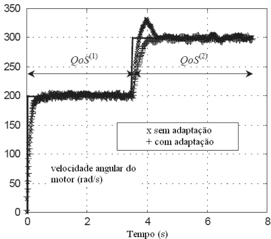
Figura 27: Resposta ao degrau de um sistema de controle de velocidade de um motor DC na metodologia baseada em adaptação do controle do usuário final; x: sem adaptação, +:com adaptação
