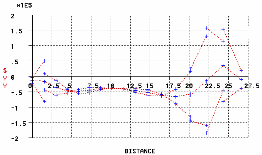
Figura 51.3 – Análise Linear – Tensões ao longo da diagonal perpendicular aos apoios – (kgf/m 2 ) – (tração = +)
