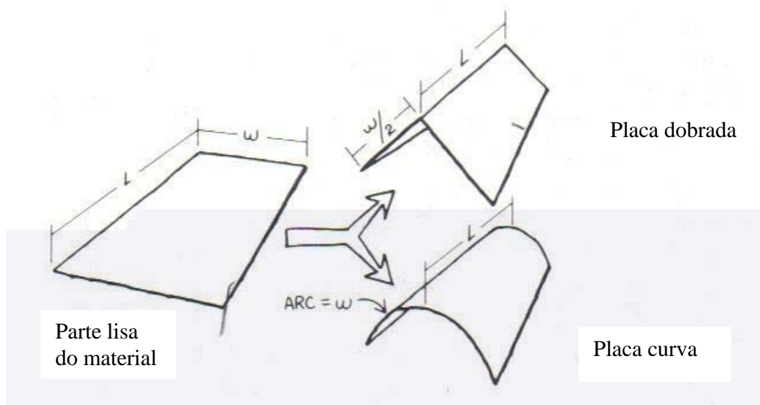
Figura 35.3– Superfície desenvolvível
