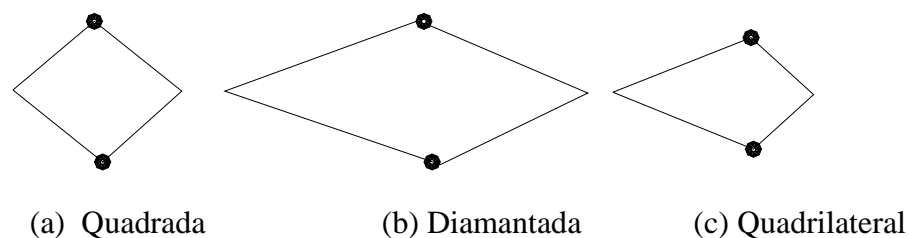
Figura 17.3 – Tipos de casca PH em planta
