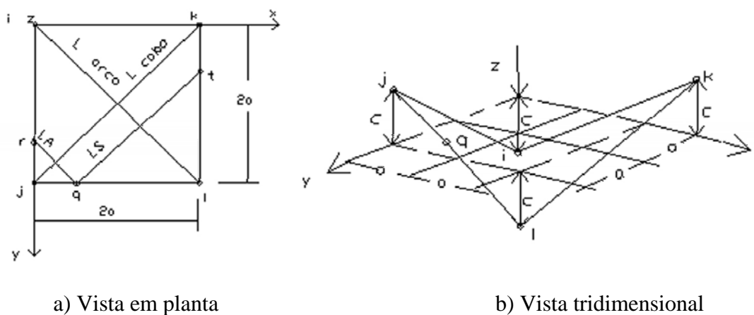
Figura25.3 – Casca PH quadrada com L_1 = L_2 = L e c_1 = c_2 = c
