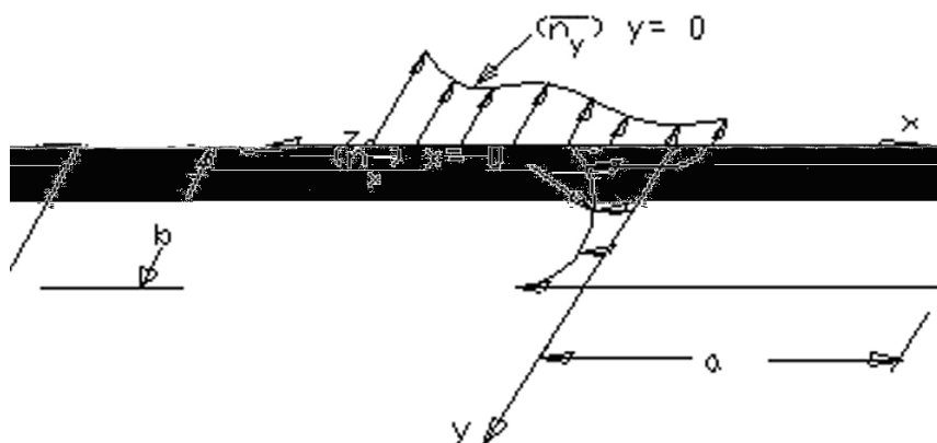
Figura 33.3– Tensões de bordo em x = 0 e y = 0
