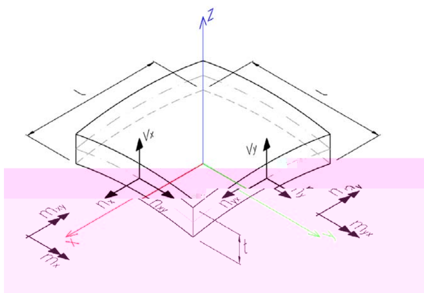
Figura 6.2 - Elemento de casca
