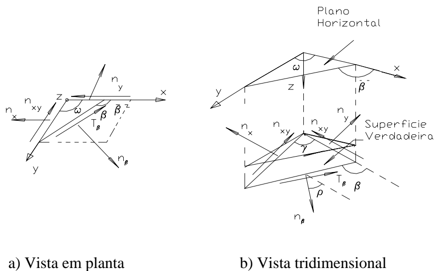
Figura 34.3 – Tensões normal e de corte, n_\beta e T_\beta , num plano arbitrário na superfície verdadeira da casca
