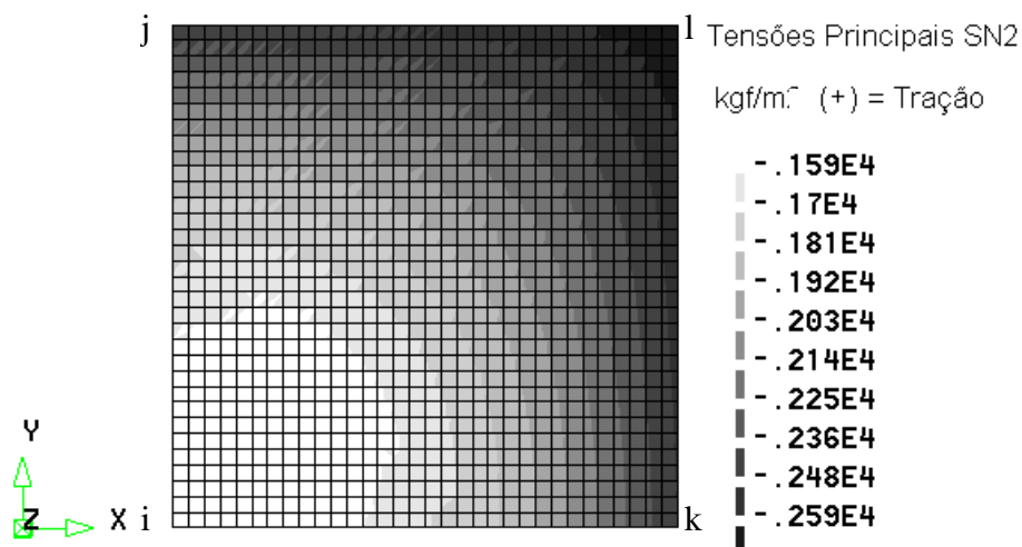
Figura 46.3 – Tensões principais de membrana nos arcos comprimidos
