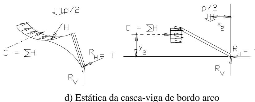
Figura 30.3 - Estática dos sistemas de apoio das vigas de bordo da casca tipo sela
