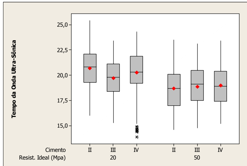
FIGURA 5.7: para o Tempo da Onda Ultra-Sônica ( \mu\text{s} ) Estratificado por Resistência Ideal (MPa) e Tipo de Cimento.
