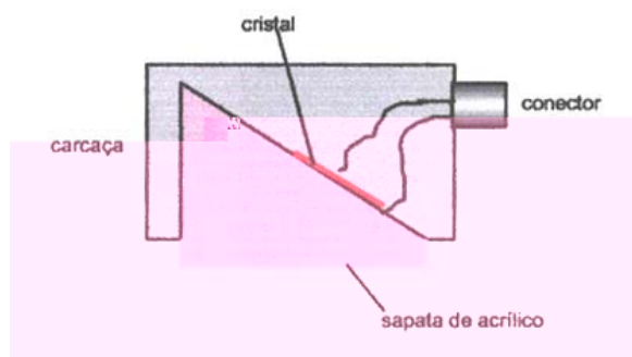
FIGURA 3.6 – Transdutor angular. (ANDREUCCI, 2002)
