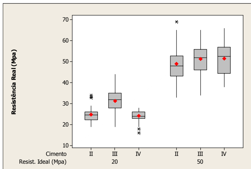
FIGURA 5.3: para a Resistência Real (MPa) Estratificado por Resistência Ideal (MPa) e Tipo de Cimento.
