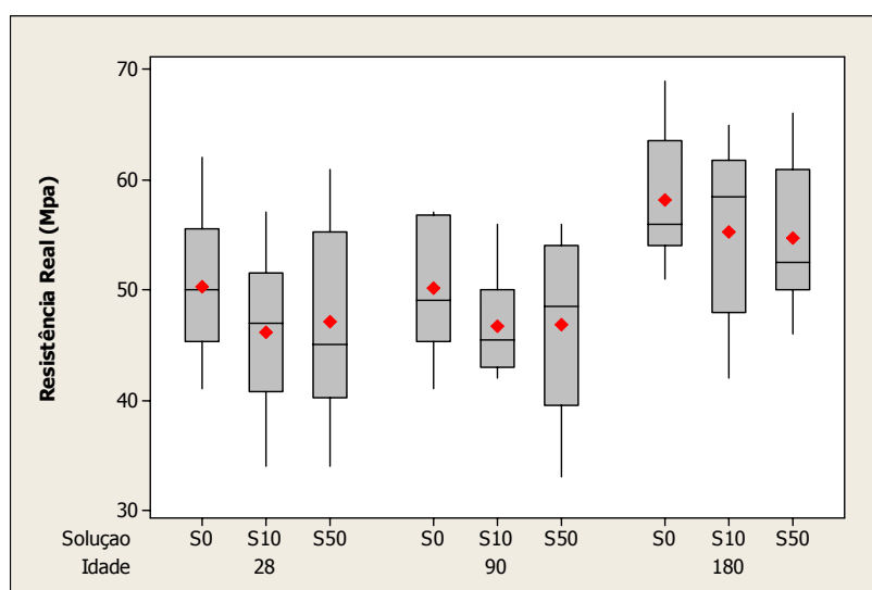
FIGURA 5.6: para a Resistência Real (MPa) Estratificado por Idade e Solução (Resistência Ideal igual a 50 MPa).
