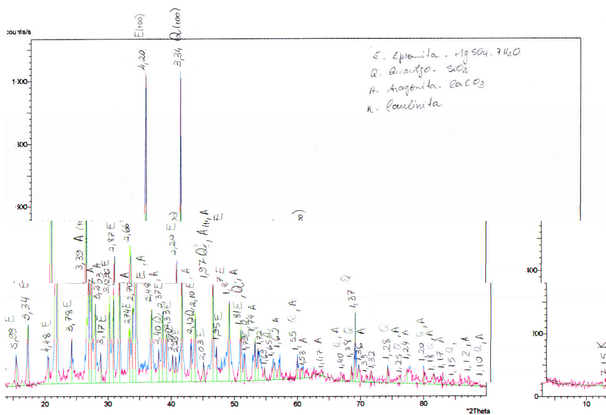
FIGURA C.16: Análise de Difração de Raios-X do Pó Acumulado no Fundo da Caixa D'água da Solução S50.
