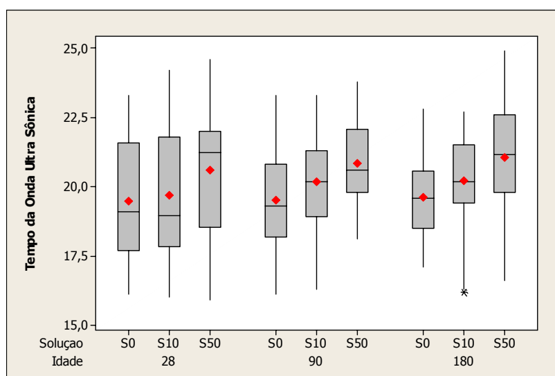
FIGURA 5.20: para o Tempo da Onda Ultra-Sônica ( \mu\text{s} ) Estratificado por Solução e Idade (Resistência Ideal igual a 20 MPa).
