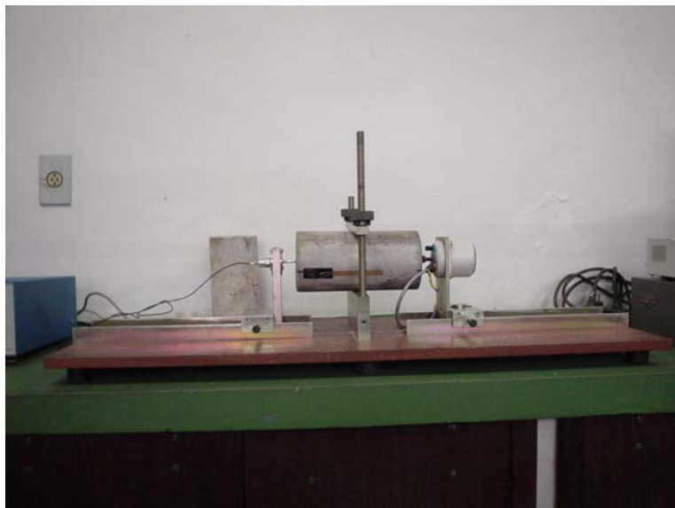
FOTO B.3: Aparelho Utilizado para a Determinação do Módulo de Elasticidade Dinâmico.
