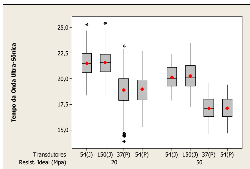
FIGURA 5.11: para o Tempo da Onda Ultra-Sônica ( \mu\text{s} ) Estratificado por Resistência Ideal (MPa) e Transdutores.
