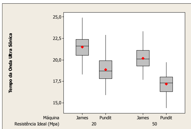
FIGURA 5.23: para o Tempo da Onda Ultra-Sônica ( \mu\text{s} ) Estratificado por Resistência Ideal (MPa) e Máquina.
