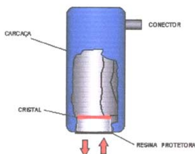
FIGURA 3.5 – Transdutor normal ou reto. (ANDREUCCI, 2002)
