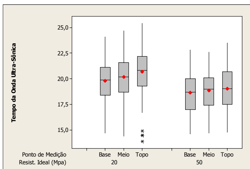
FIGURA 5.13: para o Tempo da Onda Ultra-Sônica ( \mu\text{s} ) Estratificado por Resistência Ideal (MPa) e Ponto de Medição.
