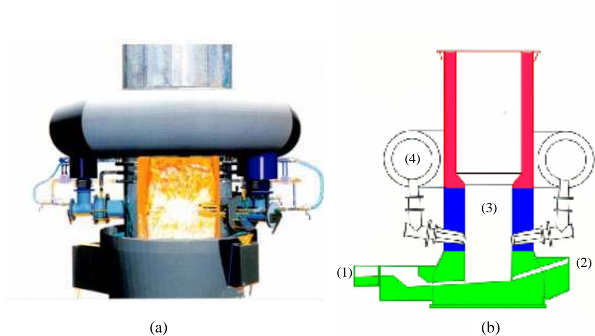
Figura 2.3 - Fotografia (a) e desenho esquemático (b) de forno tipo cubilô. Canal de vazamento de ferro líquido (1), canal de vazamento de escória (2), interior do forno (3), sistema de refrigeração (4).
