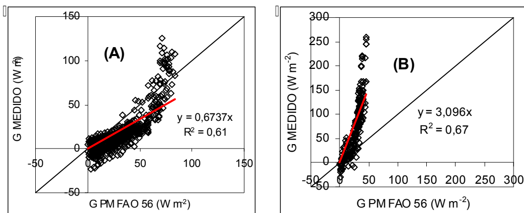
Figura 24 - Gráficos das correlações entre os valores do fluxo de calor no solo ( G ) medidos pelos fluxímetros e estimados pela Equação de Penmam-Monteith FAO 56, nos pixels da cana-de-açúcar (A) e do coqueiro anão (B), em W m^{-2} .
