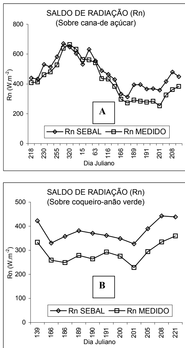
Figura 18 - Distribuição temporal dos valores do saldo de radiação medidos por saldo radiômetros e estimados pelo SEBAL sobre as culturas da cana-de-açúcar (A) e do coqueiro-anão verde (B), em W\ m^{-2} .
