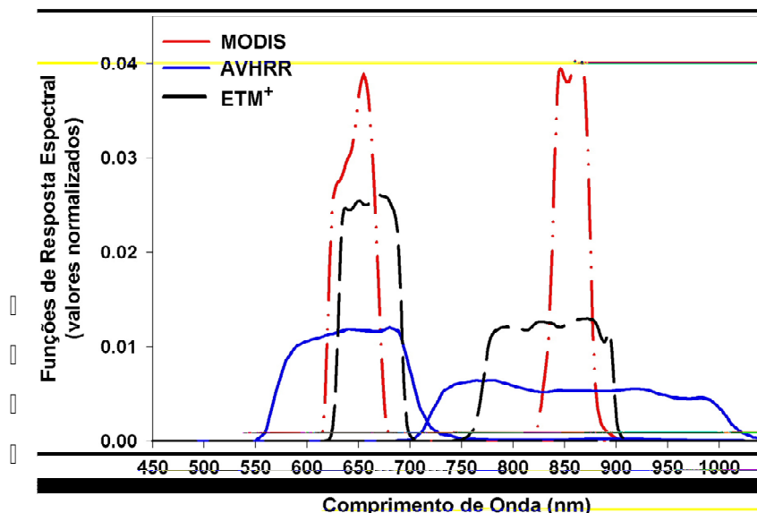
Figura 1 - Disposição e largura de bandas do sensor MODIS em relação aos sensores ETM+ e AVHRR. Fonte: Adaptada de Justice et al. (1998).
