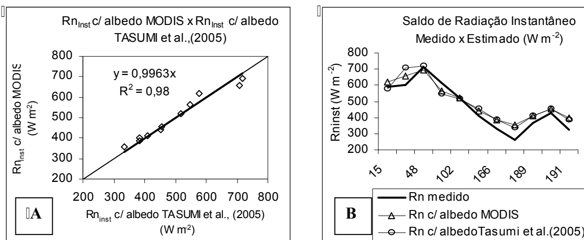
Figura 14 - Gráfico da correlação entre os valores do saldo de radiação, em \text{mm dia}^{-1} estimados com o albedo obtido pelo método de Tasumi et al. e com o albedo produto MODIS (A) e da distribuição temporal dos valores medidos e estimados pelas duas metodologias (B)
