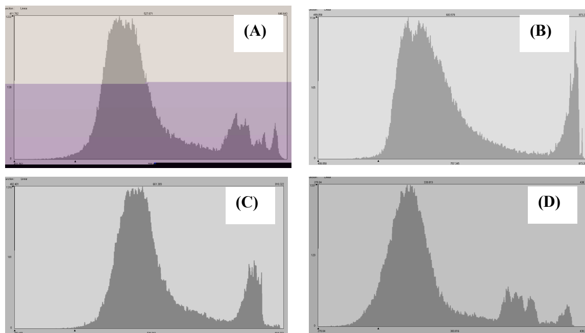
Figura 20 - Histogramas correspondentes às cartas do saldo de radiação, na região Norte Fluminense, RJ, nos dias 2005241 (A), 2005320 (B), 2006036 (C) e 2006166 (D), em \text{W m}^{-2} .
