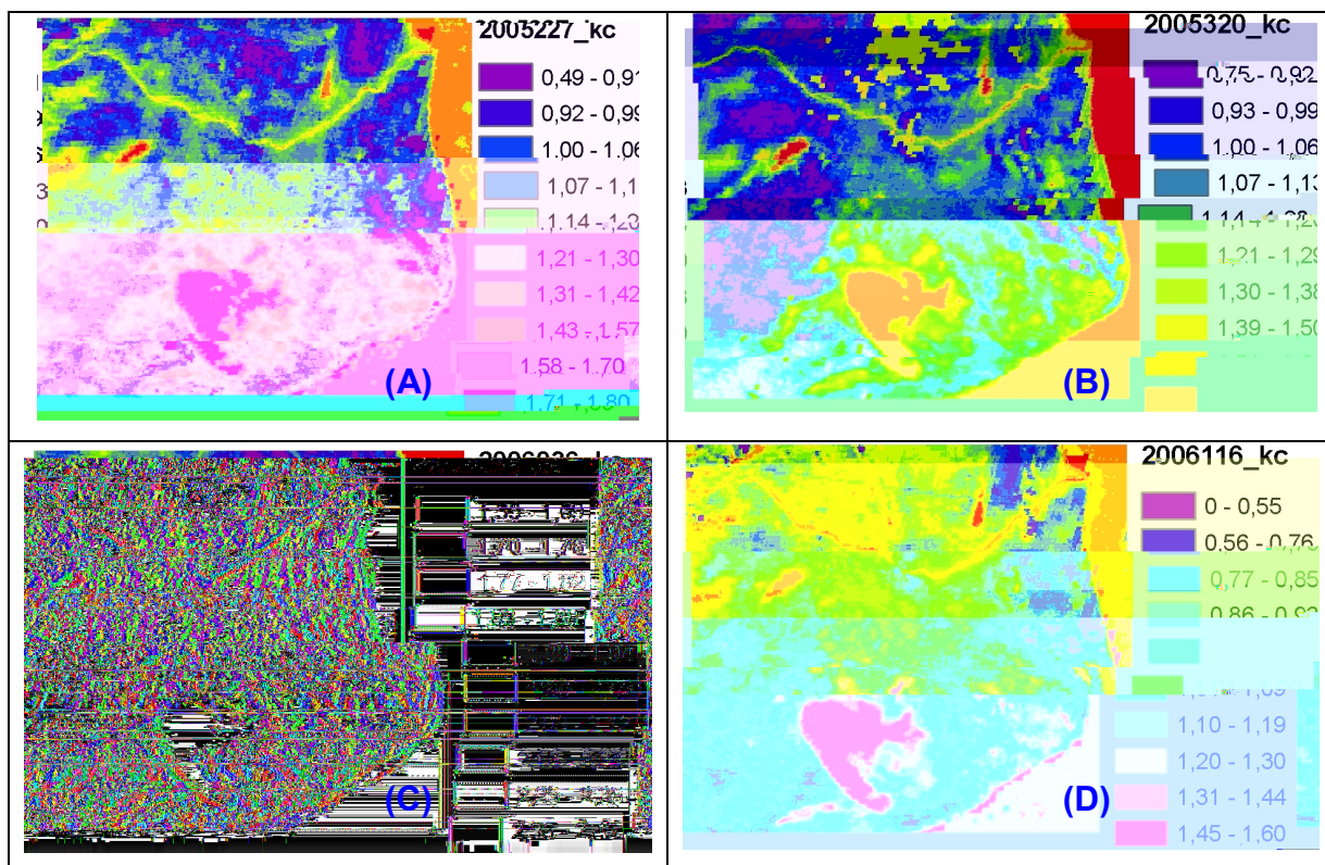
Figura 42 - Variação espacial do coeficiente cultural (Kc), estimado pelo SEBAL, na região Norte Fluminense, RJ nos dias julianos 2005227 (A), 2005320 (B), 2006036 (C) e 2006116 (D).
