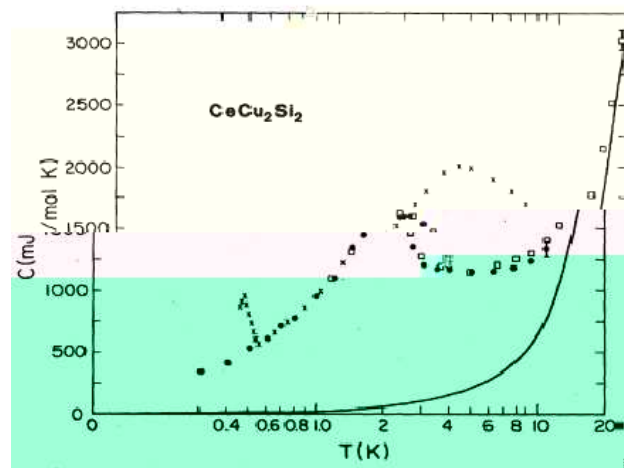
Figura 1.8: Medida de calor específico versus temperatura para o composto \text{CeCu}_2\text{Si}_2 obtido por Steglich et. al. [20].
