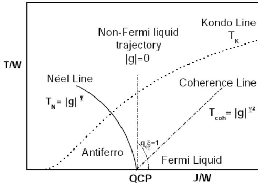
Figura 1.3: Diagrama de fases para a rede Kondo [28]
