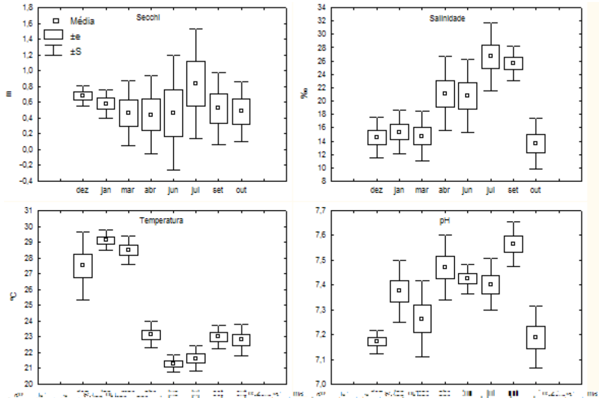
Figura 2. Variação nos dias amostrados das médias da visibilidade da água (Secchi), salinidade, temperatura da água e pH.
